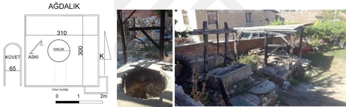
Şekil 4.56. Yalnızdam, Ağdalık (Orijinal 2018)
