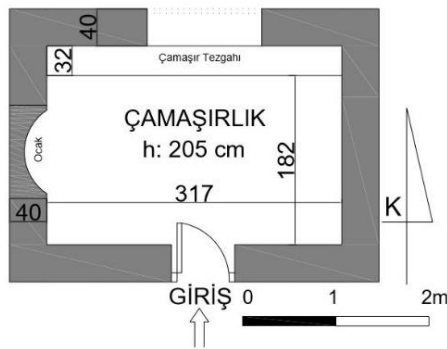
Şekil 4.44. Armutlu, Çamaşırlık yapısı plan görüntüsü (Oriinal 2018)
