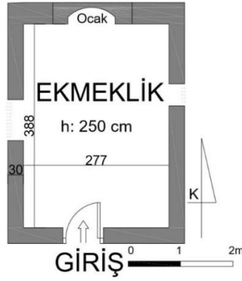
Şekil 4.30. Düden, Ekmeklik yapısı (Orijinal 2018)
