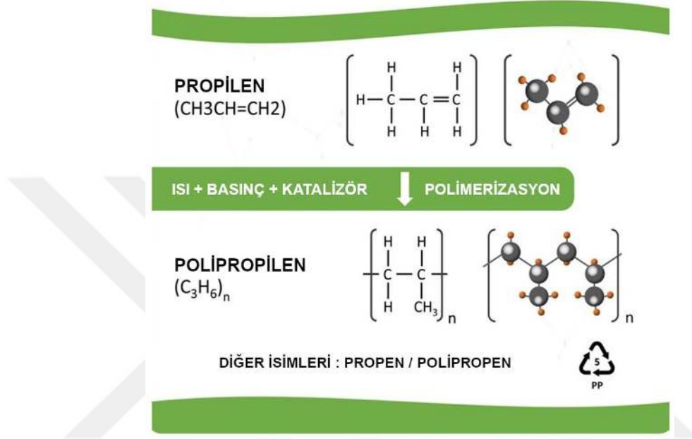
Şekil 2.15. Polipropilen Formül Yapısı
