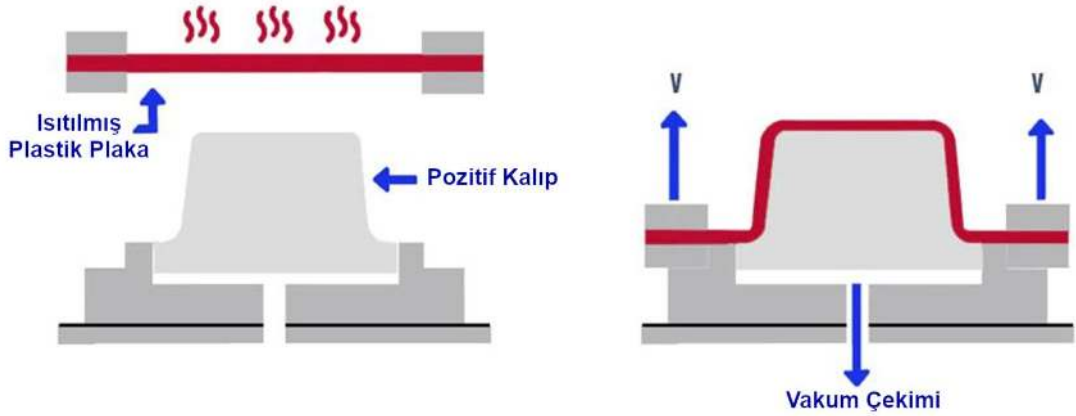
Şekil 2.7. Vakum Şekillendirme
