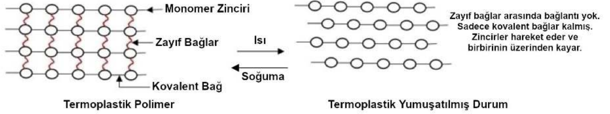
Şekil 2.11. Termoplastik Polimerler
