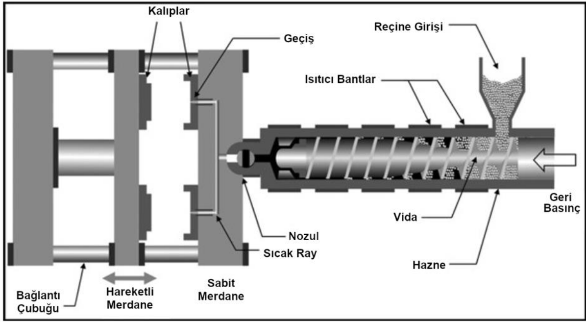
Şekil 2.8. Enjeksiyon Kalıplama
