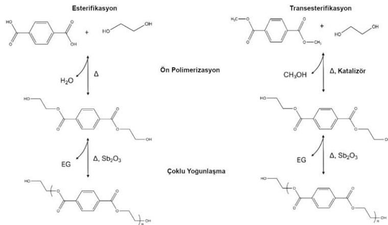
Şekil 2.17. PET Polimerizasyon Yapısı
