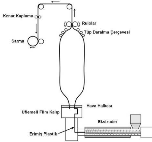
Şekil 2.4. Üflemlî Film Ekstrüzyonu
