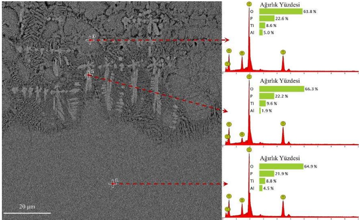
Şekil 5.8. LATP-C numunesinde soğuma esnasında meydana gelen farklı yapılarıdaki katılaşma ürünlerinin enerji dağılımlı x-ışını tekniği ile elementel analizi. (1) camı faz, (2) dendritik kristalleşme, (3) yöne bağlı olmayan kristalleşme
