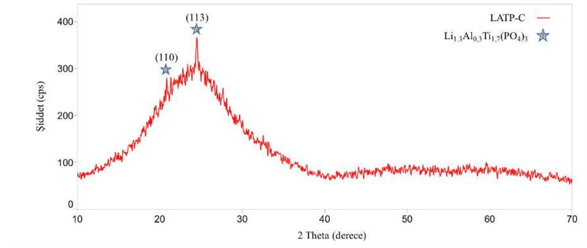
Şekil 5.2. LATP-C numunesinin XRD deseni
