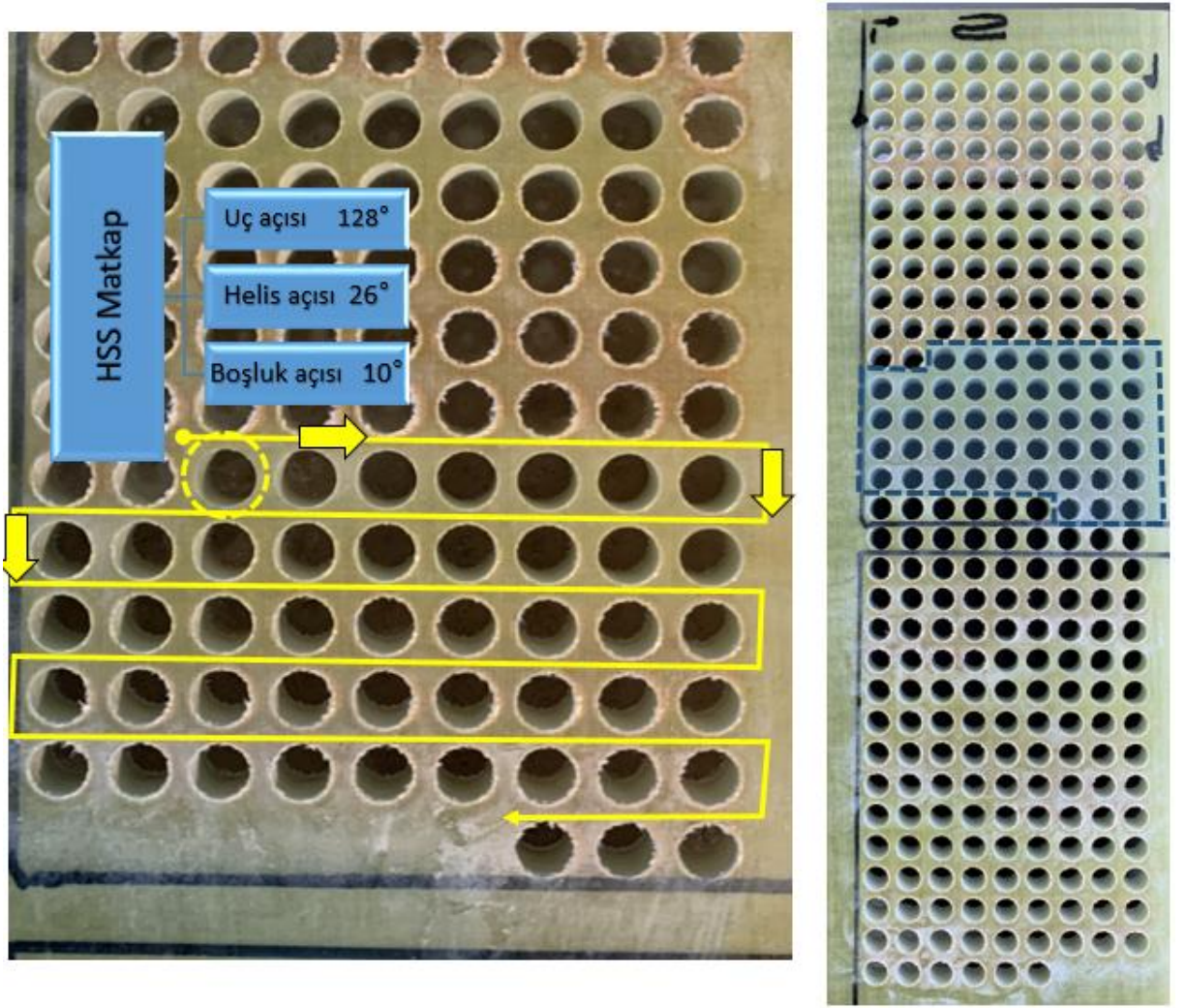
Şekil 4.129. HSS matkap ile delinen kompozit iş parçası
