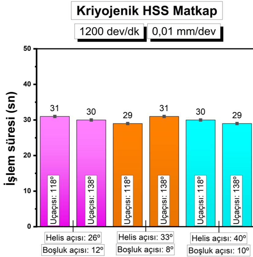
Şekil 4.111. Kriyojenik HSS matkapların 1200 dev/dk ve 0,01 ilerleme hızındaki işleme süreleri
