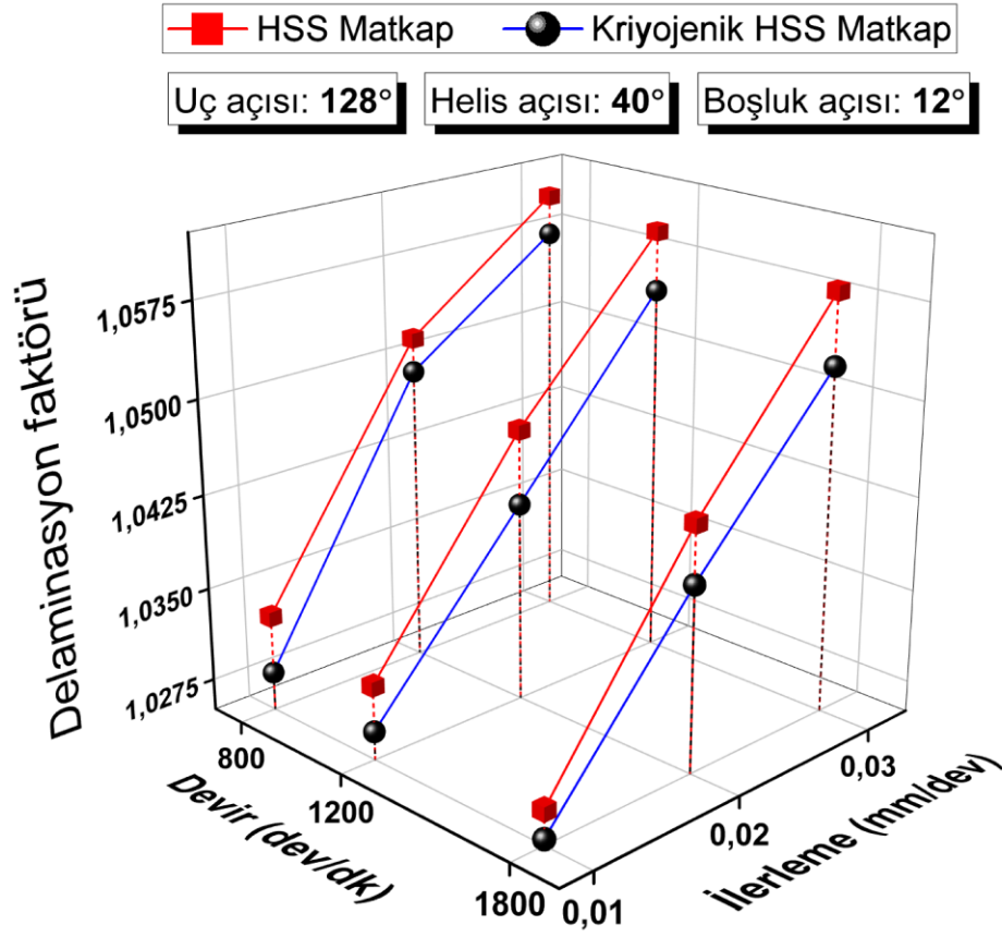
Şekil 4.86. 128° uç açısı, 40° helis açısı ve 12° boşluk açılı matkaplar ile işlemede delaminasyon faktörü
