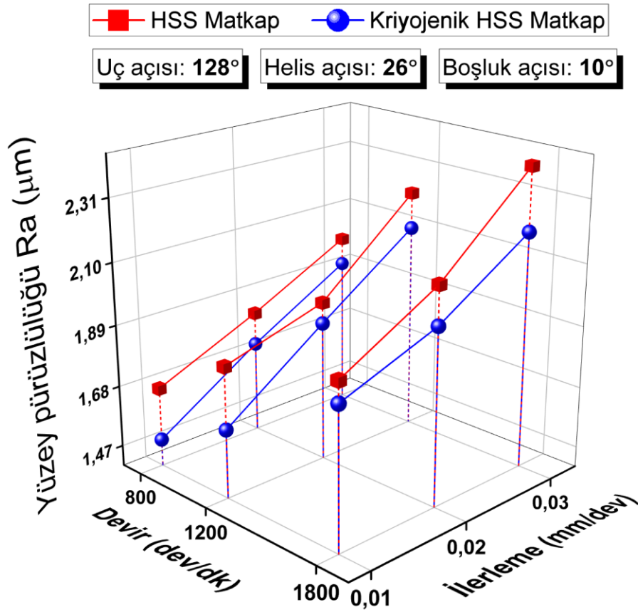
Şekil 4.47. 128° uç açısı, 26° helis açısı ve 10° boşluk açılı matkaplar ile işlemede yüzey pürüzlülüğü
