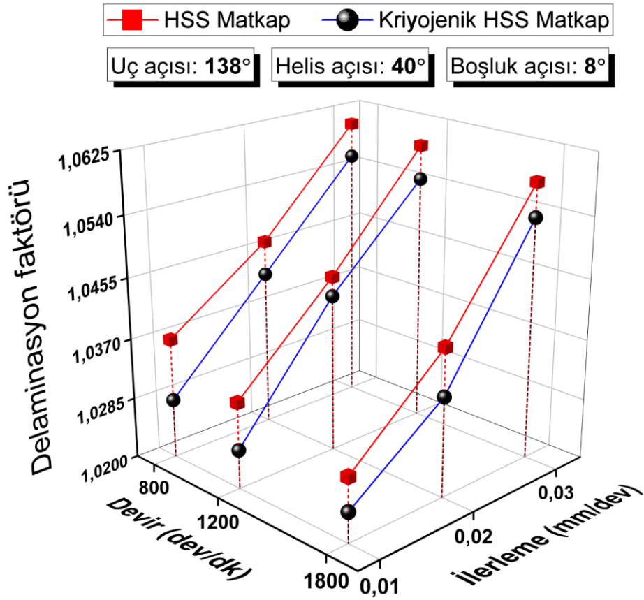
Şekil 4.93. 138° uç açısı, 40° helis açısı ve 8° boşluk açılı matkaplar ile işlemede delaminasyon faktörü
