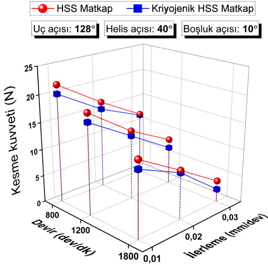
Şekil 4.22. 128° uç açısı, 40° helis açısı ve 10° boşluk açısına sahip matkaplarda kesme kuvveti
