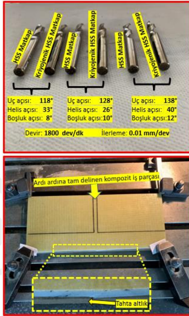
Şekil 4.116. Takım ömrü deneyleri için kullanılan kesici takımlar ve kompozit iş parçası
