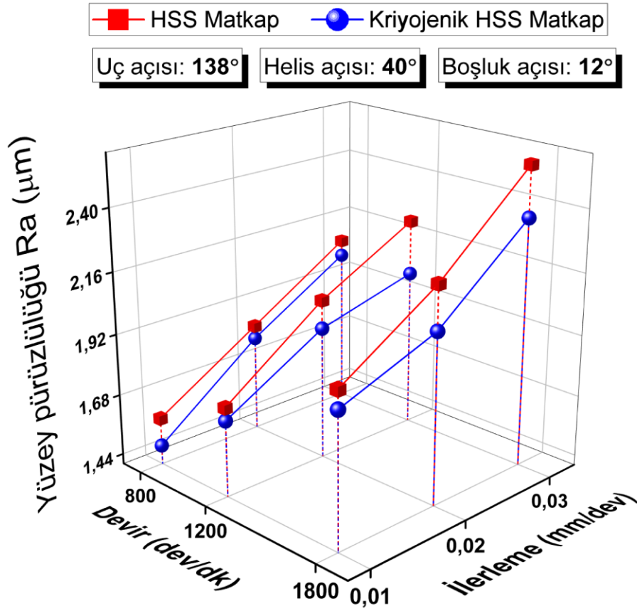
Şekil 4.63. 138^\circ uç açısı, 40^\circ helis açısı ve 12^\circ boşluk açılı matkaplar ile işlemede yüzey pürüzlülüğü
