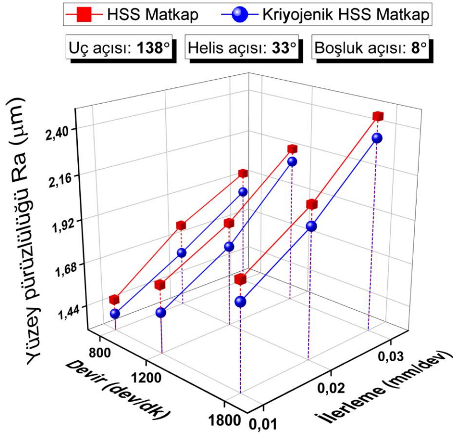
Şekil 4.58. 138^\circ uç açısı, 33^\circ helis açısı ve 8^\circ boşluk açılı matkaplar ile işlemede yüzey pürüzlülüğü
