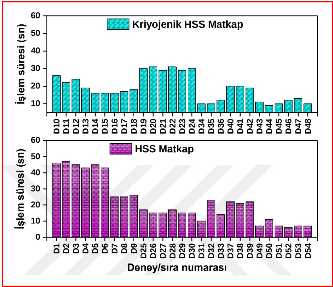
Şekil 4.106. HSS matkaplar ile kriyojenik ve temperlenmiş HSS matkapların işlem süreleri
