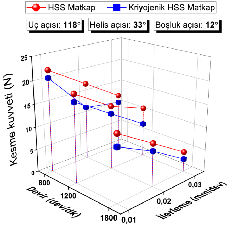
Şekil 4.11. 118° uç açısı, 33° helis açısı ve 12° boşluk açısına sahip matkaplarda kesme kuvveti
