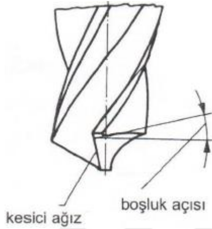
Şekil 1.24. Kesici takım matkabın boşluk açısı (Şahin, 2008)
