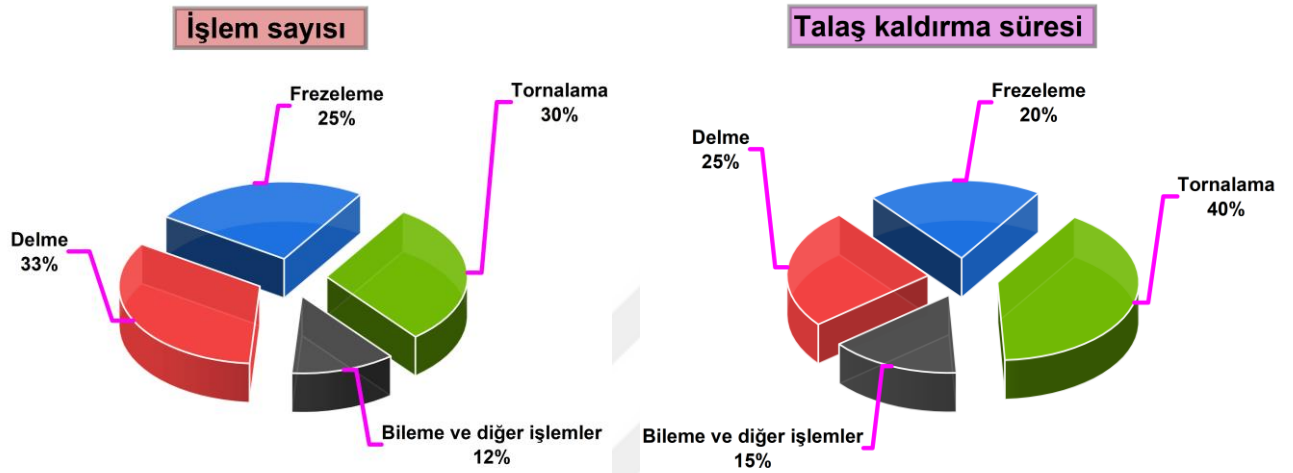
Şekil 1.10. İşlem sayısı ve talaş kaldırma süresinin karşılaştırması (Tönshoff ve ark., 1994)
