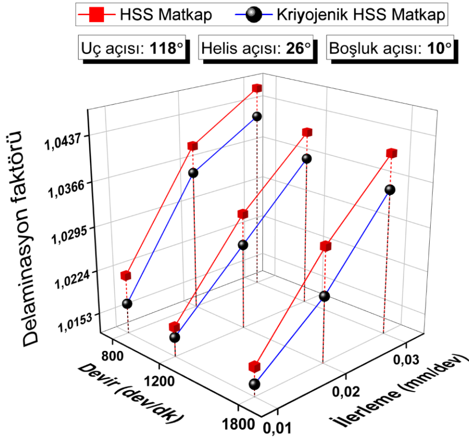
Şekil 4.70. 118° uç açısı, 26° helis açısı ve 10° boşluk açılı matkaplar ile işlemede delaminasyon faktörü
