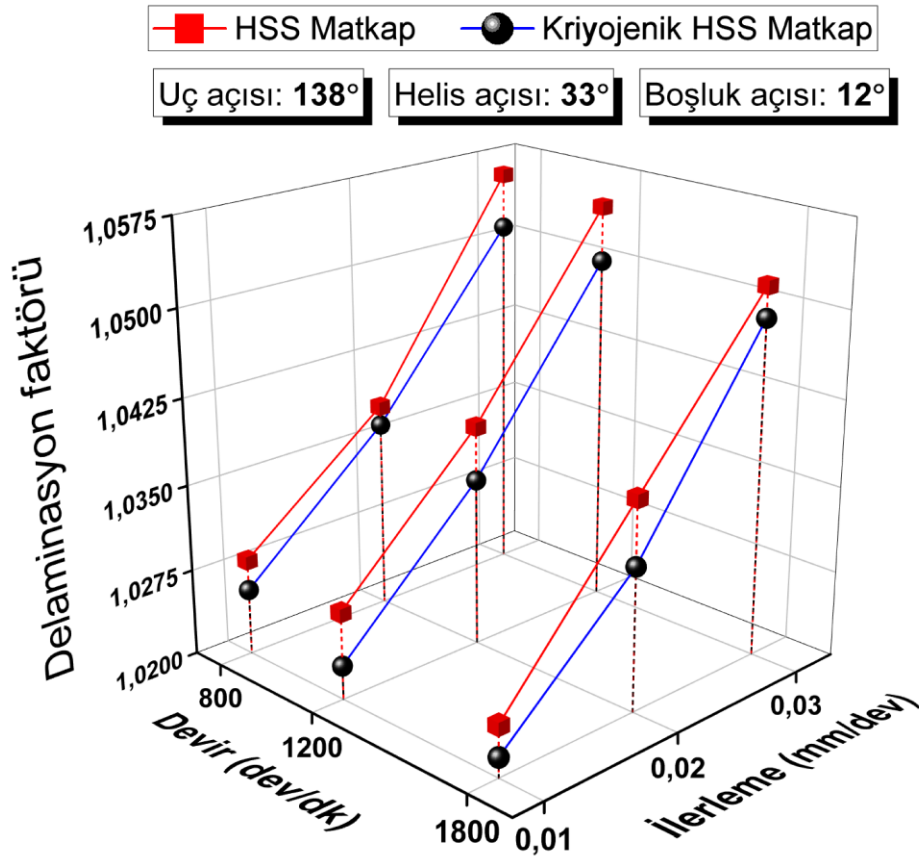
Şekil 4.92. 138° uç açısı, 33° helis açısı ve 12° boşluk açılı matkaplar ile işlemede delaminasyon faktörü
