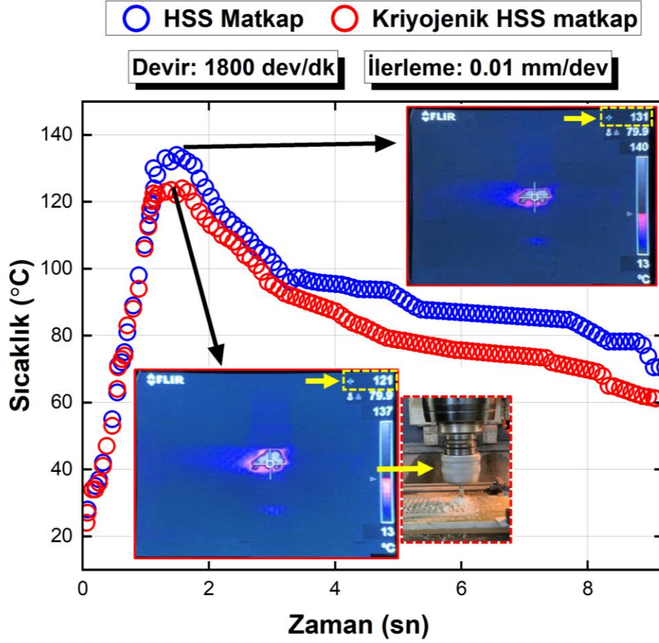
Şekil 4.125. Aşınma testleri sırasında çıkan talaşların sıcaklıkları
