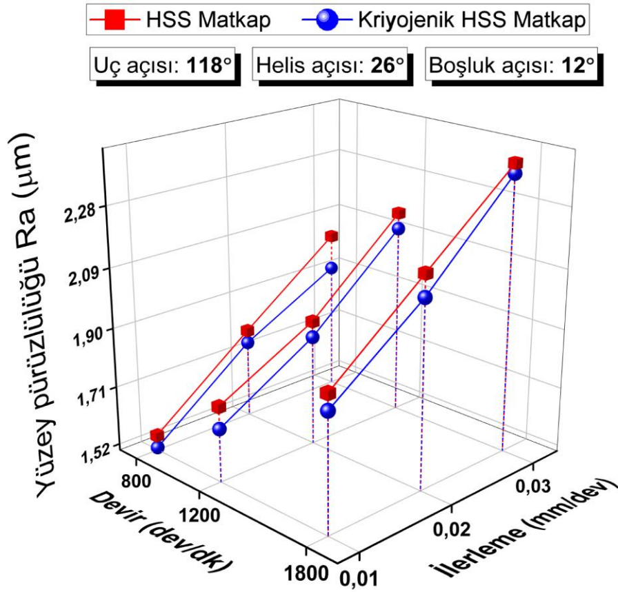
Şekil 4.39. 118° uç açısı, 26° helis açısı ve 12° boşluk açılı matkaplar ile işlemede yüzey pürüzlülüğü
