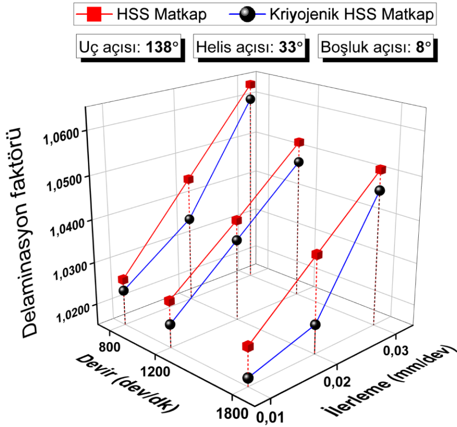
Şekil 4.90. 138° uç açısı, 33° helis açısı ve 8° boşluk açılı matkaplar ile işlemede delaminasyon faktörü
