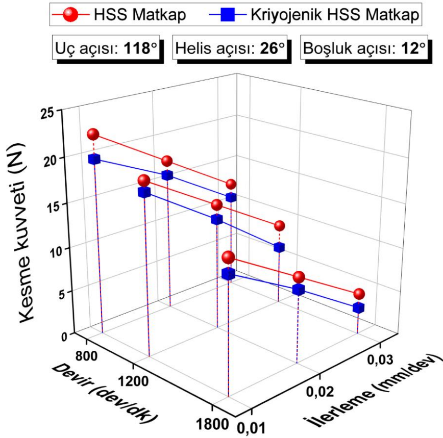
Şekil 4.8. 118° uç açısı, 26° helis açısı ve 12° boşluk açısına sahip matkaplarda kesme kuvveti
