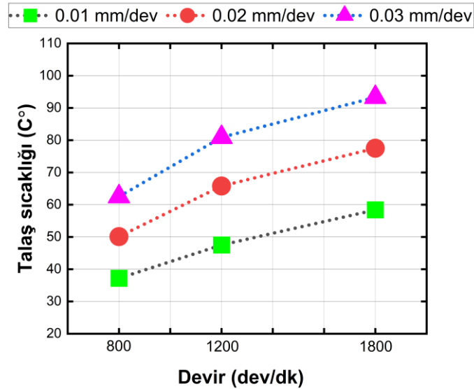
Şekil 4. 124. Devir sayısı ve ilerlemeye bağlı değişimde talaş sıcaklıkları
