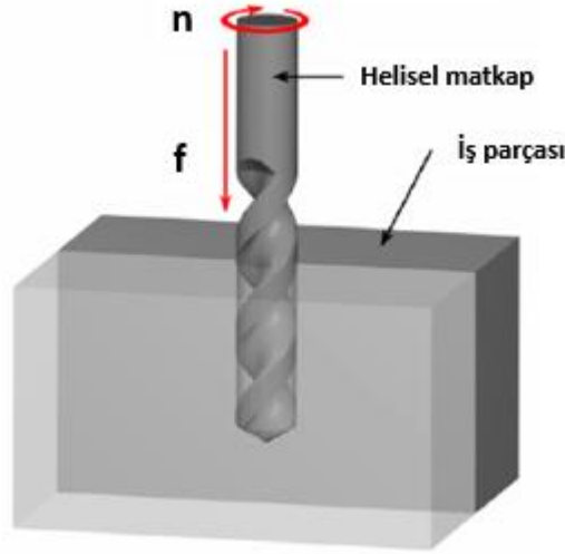
Şekil 1.20. Delik delme işleminde dönme ve ilerleme hareketi (Patel ve Verma, 2015)
