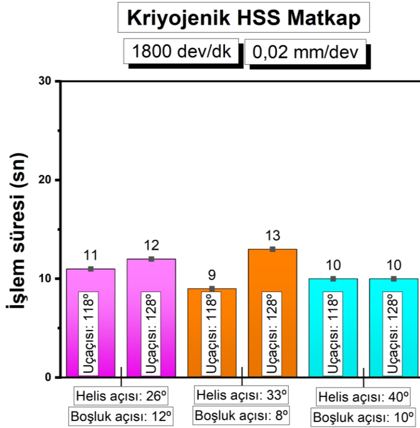
Şekil 4.112. Kriyojenik HSS matkapların 1800 dev/dk ve 0,02 ilerleme hızındaki işleme süreleri
