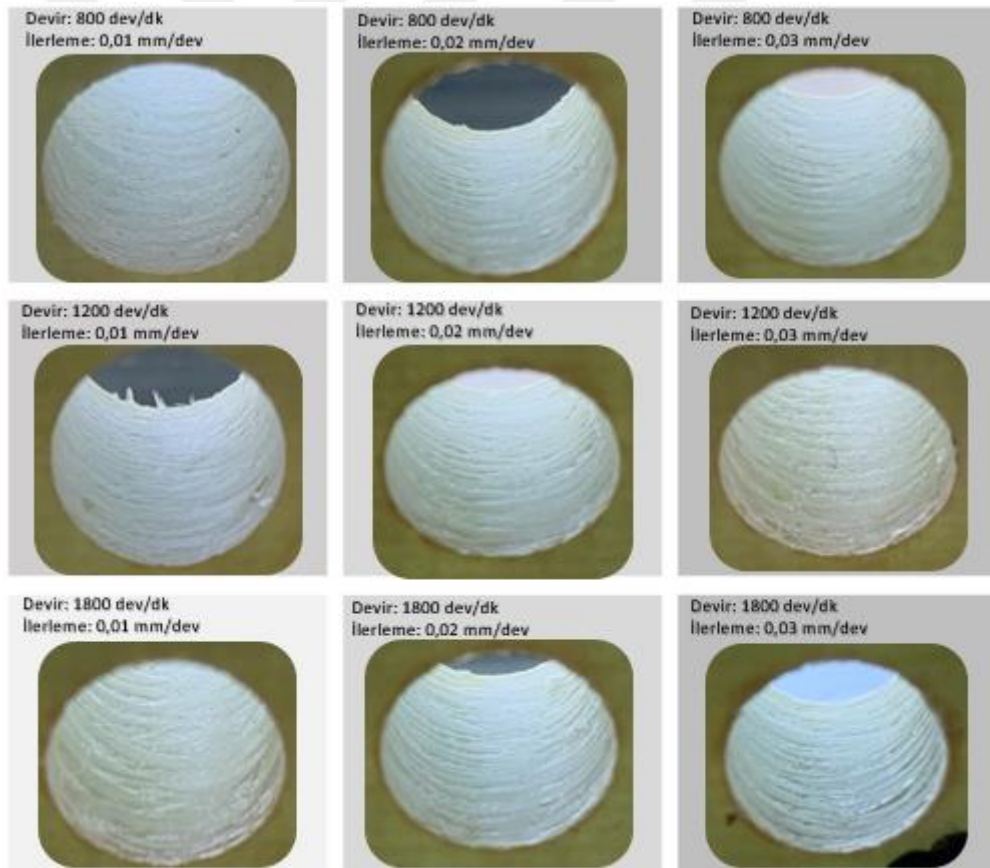
Şekil 4.64. Devir ve ilerleme artışına bağlı yüzey pürüzlülükleri değişimleri
