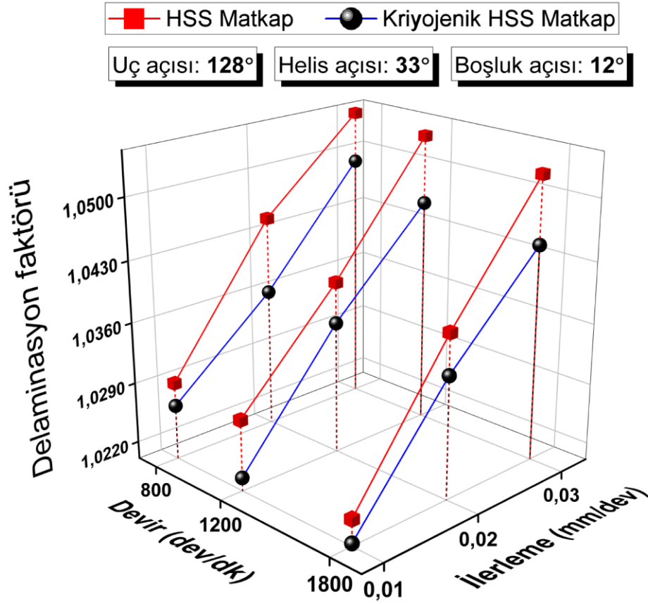
Şekil 4.83. 128° uç açısı, 33° helis açısı ve 12° boşluk açılı matkaplar ile işlemede delaminasyon faktörü
