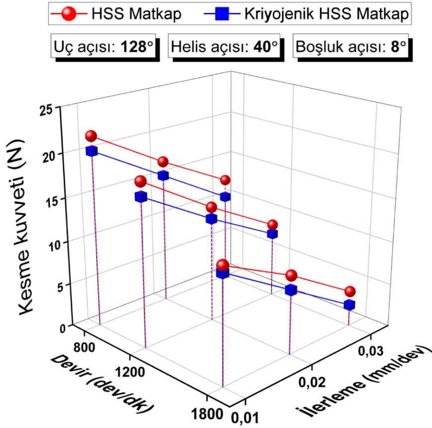
Şekil 4.21. 128° uç açısı, 40° helis açısı ve 8° boşluk açısına sahip matkaplarda kesme kuvveti
