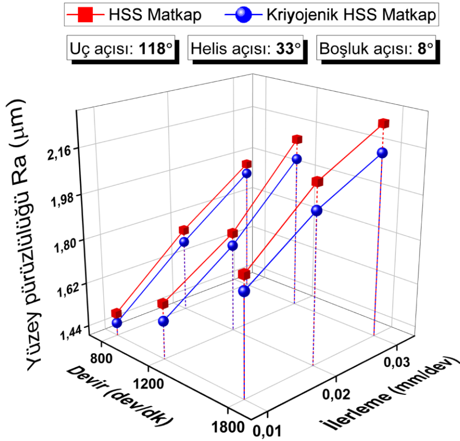
Şekil 4.40. 118° uç açısı, 33° helis açısı ve 8° boşluk açılı matkaplar ile işlemede yüzey pürüzlülüğü
