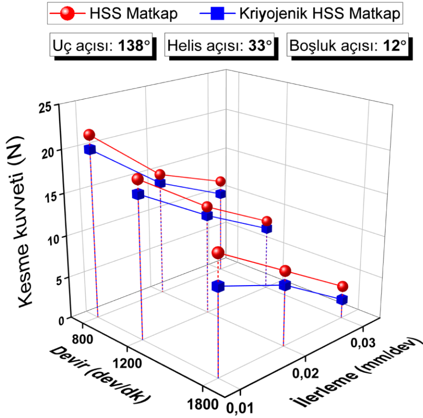
Şekil 4.29. 138° uç açısı, 33° helis açısı ve 12° boşluk açısına sahip matkaplarda kesme kuvveti
