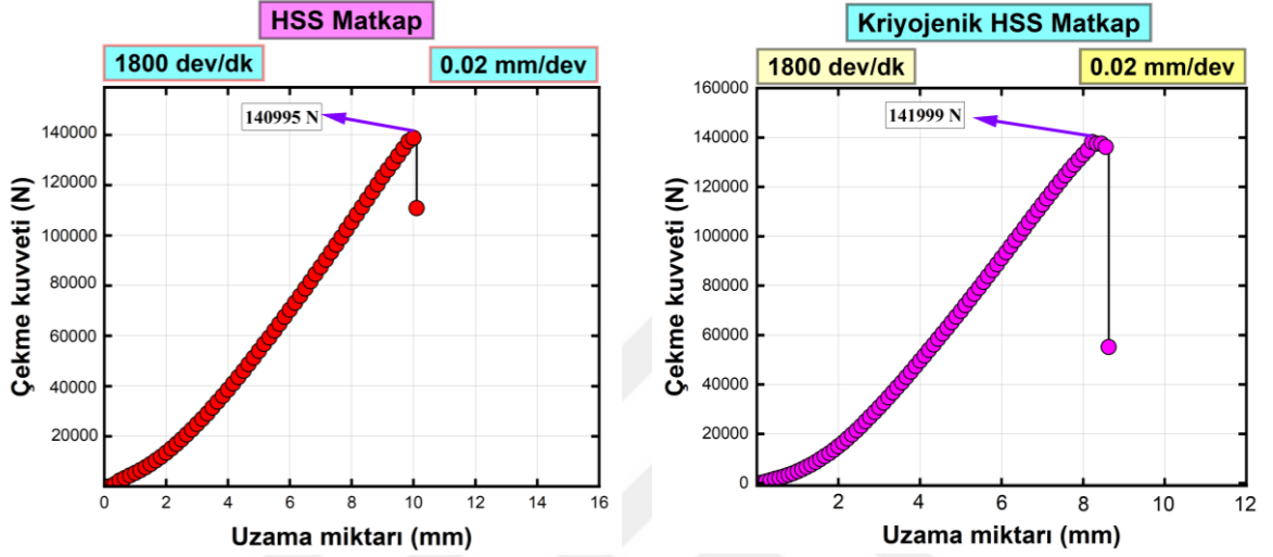
Şekil 4.134. 0,02 mm/dev ilerleme ile delik açılan numunelerin çekme grafikleri
