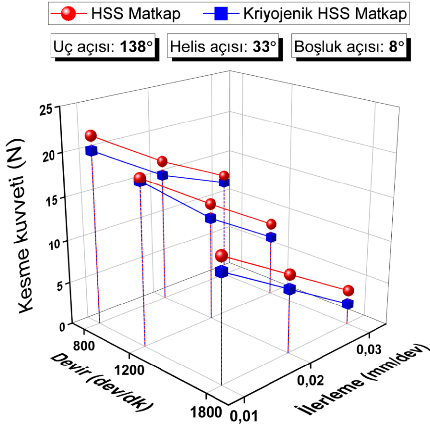
Şekil 4.27. 138° uç açısı, 33° helis açısı ve 8° boşluk açısına sahip matkaplarda kesme kuvveti
