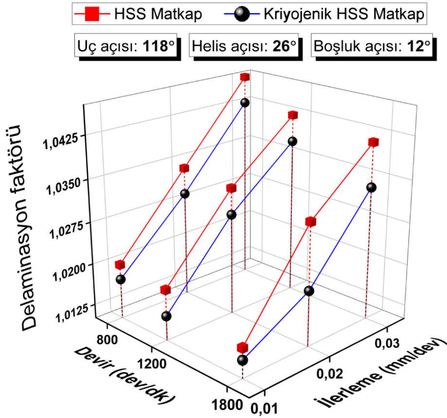
Şekil 4.71. 118° uç açısı, 26° helis açısı ve 12° boşluk açılı matkaplar ile işlemede delaminasyon faktörü
