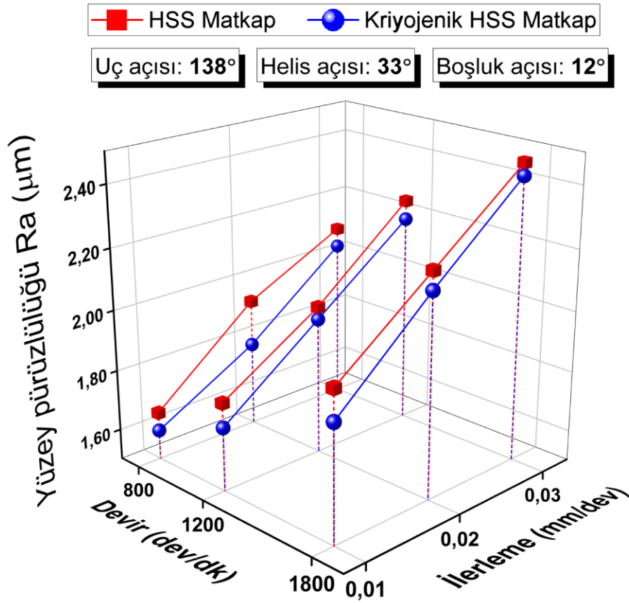
Şekil 4.60. 138^\circ uç açısı, 33^\circ helis açısı ve 12^\circ boşluk açılı matkaplar ile işlemede yüzey pürüzlülüğü
