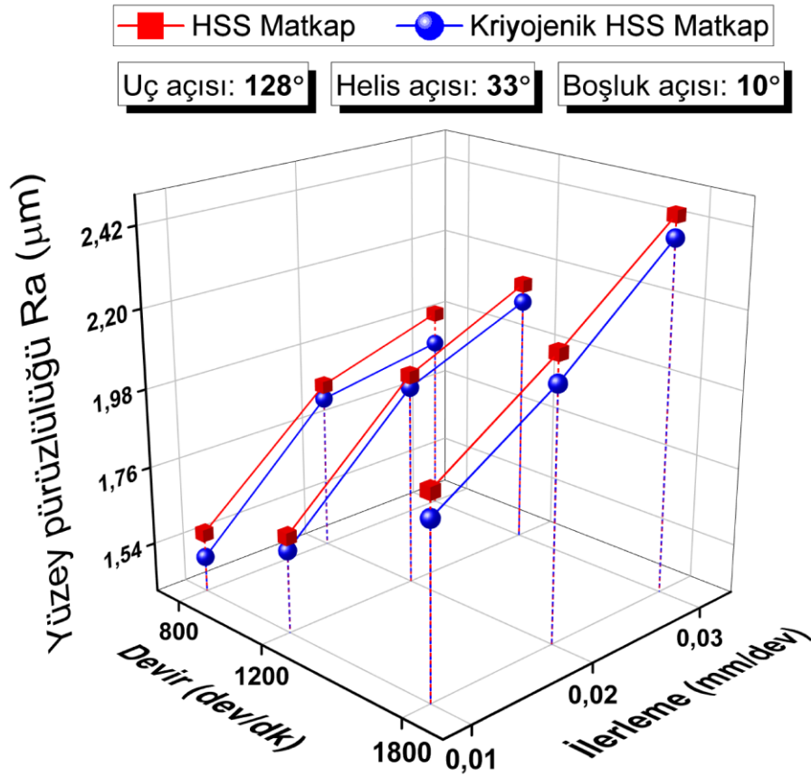
Şekil 4.50. 128° uç açısı, 33° helis açısı ve 10° boşluk açılı matkaplar ile işlemede yüzey pürüzlülüğü
