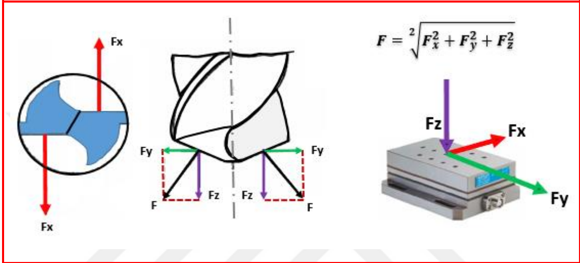
Şekil 3.13. Matkabı etkileyen kuvvetler (Kıvak, 2007; Yenigün, 2018)
