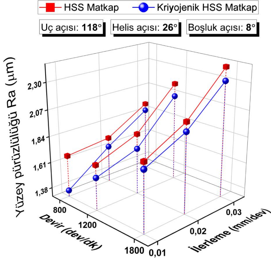
Şekil 4.37. 118° uç açısı, 26° helis açısı ve 8° boşluk açılı matkaplar ile işlemede yüzey pürüzlülüğü
