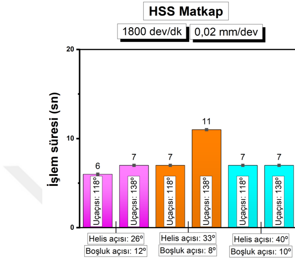
Şekil 4.109. HSS matkapların 1800 dev/dk ve 0,02 ilerleme hızındaki işleme süreleri
