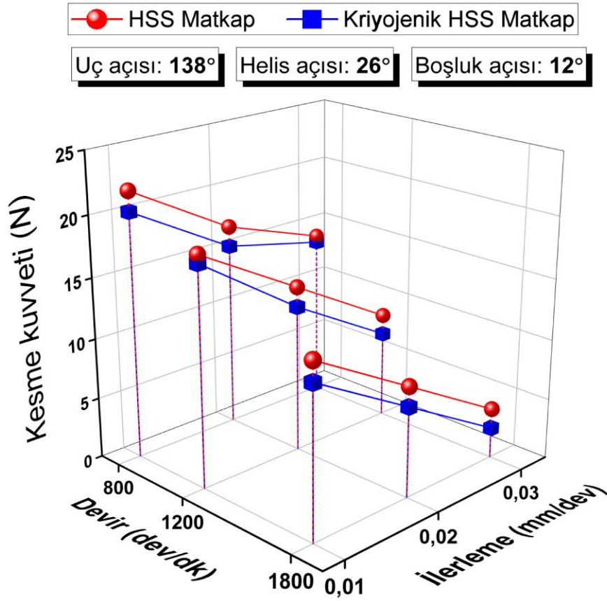
Şekil 4.26. 138° uç açısı, 26° helis açısı ve 12° boşluk açısına sahip matkaplarda kesme kuvveti
