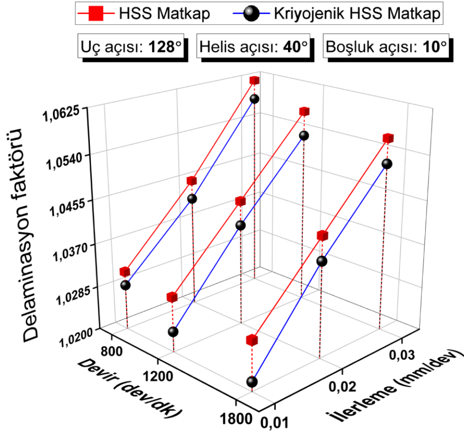
Şekil 4.85. 128° uç açısı, 40° helis açısı ve 10° boşluk açılı matkaplar ile işlemede delaminasyon faktörü
