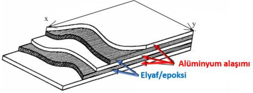
Şekil 1.8. Hibrit kompozitin temel yapısı (Botelho ve ark., 2006)
