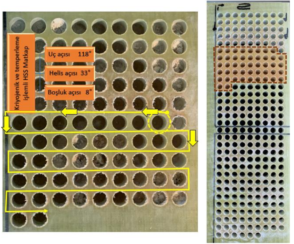
Şekil 4.128. Kriyojenik ve temperleme işlemi görmüş HSS matkap ile delinen kompozit iş parçası
