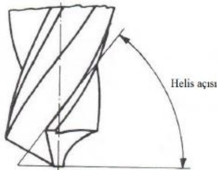
Şekil 1.25. Kesici takım matkabın helis açısı (Şahin, 2008)
