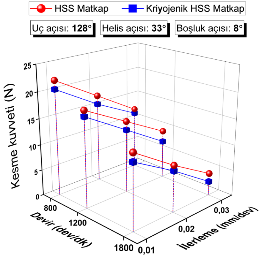
Şekil 4.18. 128° uç açısı, 33° helis açısı ve 8° boşluk açısına sahip matkaplarda kesme kuvveti
