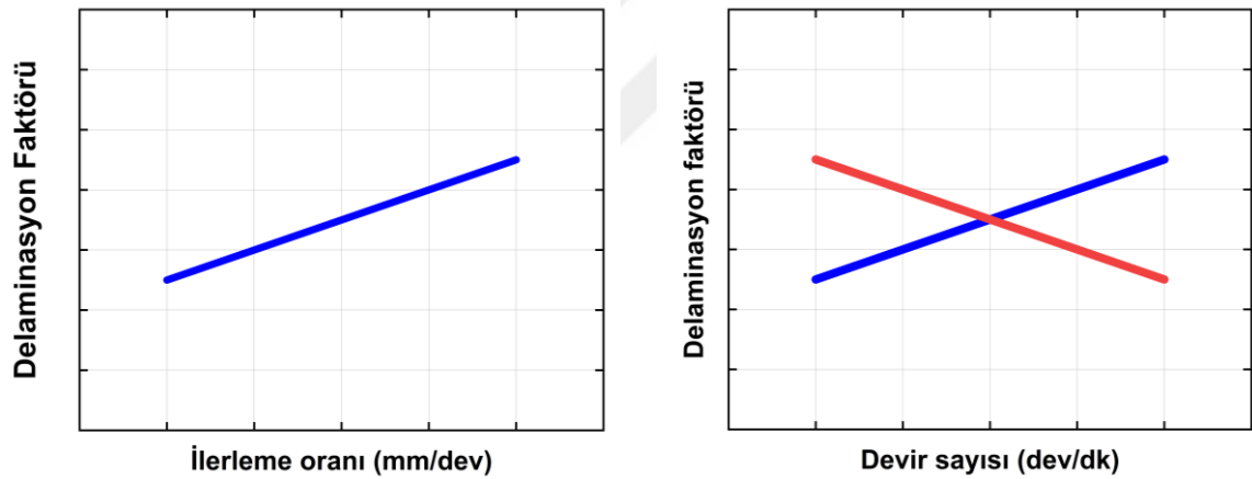
Şekil 4.68. Literatürdeki devir sayısı ve ilerlemelere göre delaminasyon faktörleri (Yenigün, 2018)
