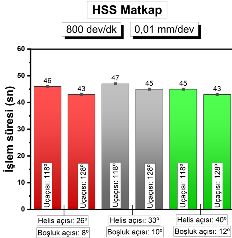
Şekil 4.107. HSS matkapların 800 dev/dk ve 0,01 ilerleme hızındaki işleme süreleri
