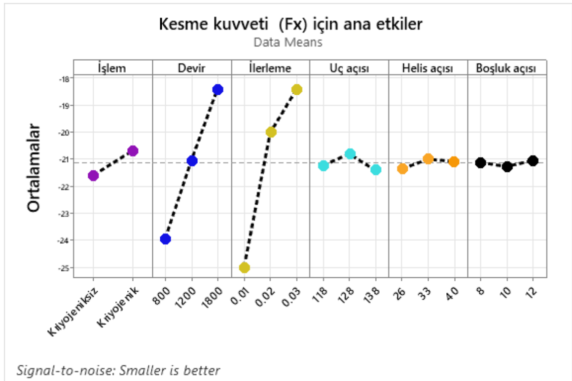
Şekil 4.4. Faktörlerin kesme kuvvetleri (Fx) üzerindeki ana etkileri
