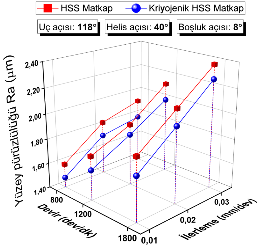
Şekil 4.43. 118° uç açısı, 40° helis açısı ve 8° boşluk açılı matkaplar ile işlemede yüzey pürüzlülüğü
