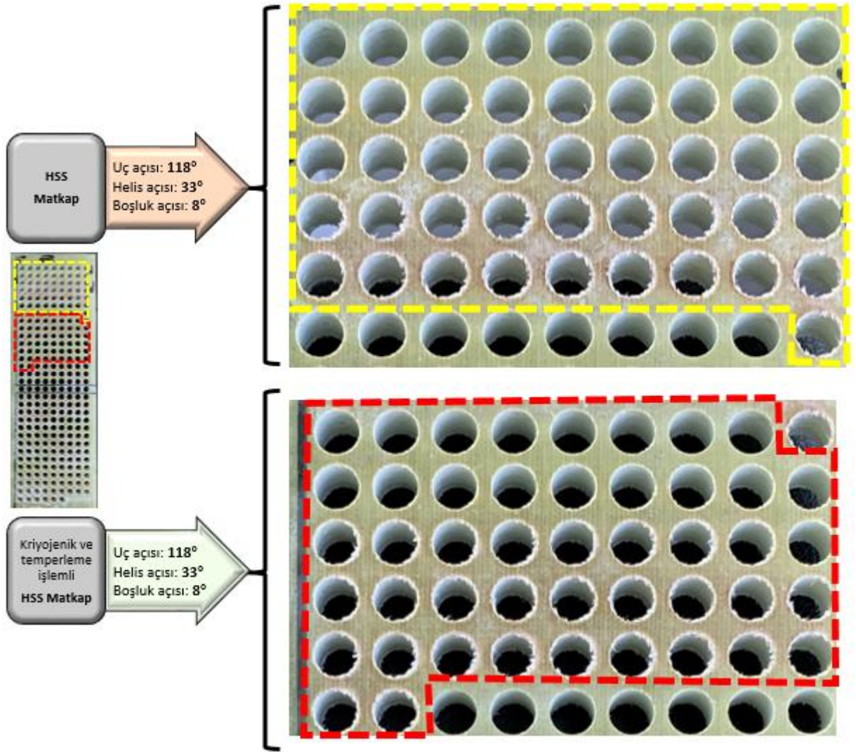
Şekil 4.131. İki matkap türünün ardı ardına delik delme görüntüleri
