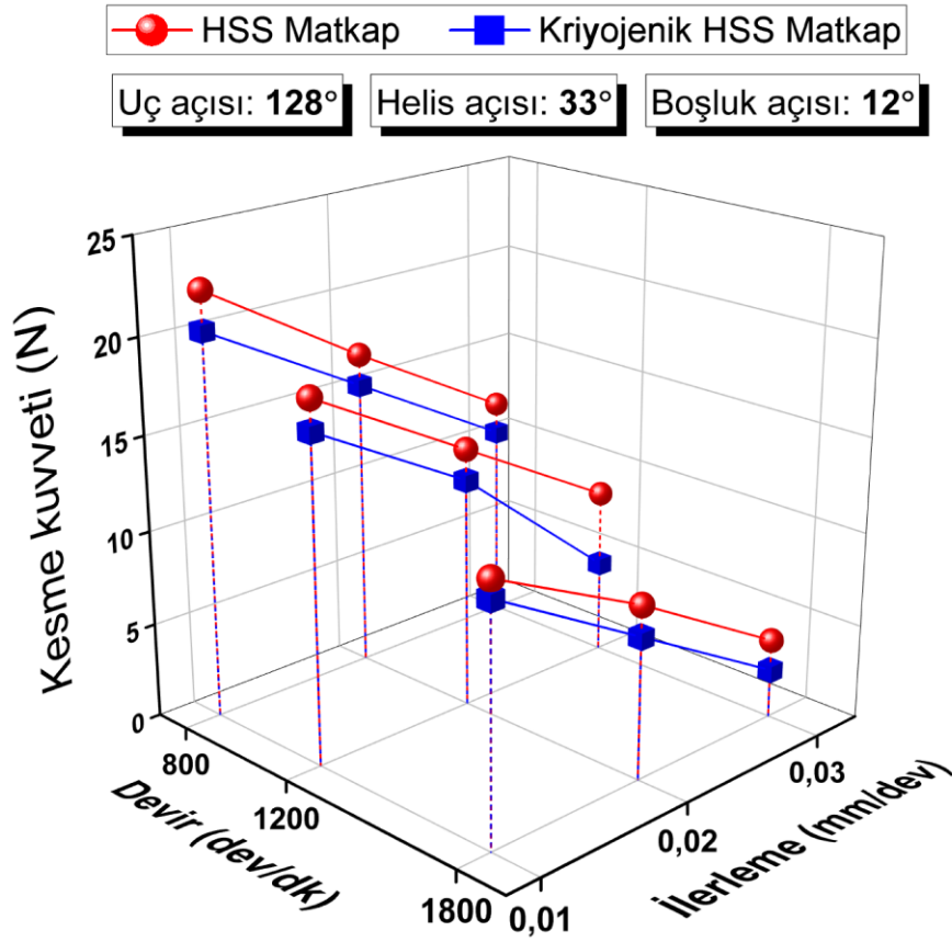
Şekil 4.20. 128° uç açısı, 33° helis açısı ve 12° boşluk açısına sahip matkaplarda kesme kuvveti
