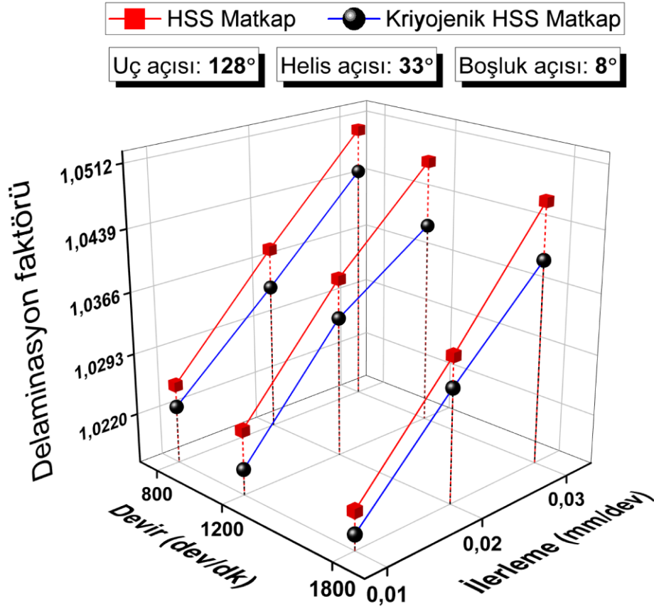
Şekil 4.81. 128° uç açısı, 33° helis açısı ve 8° boşluk açılı matkaplar ile işlemede delaminasyon faktörü
