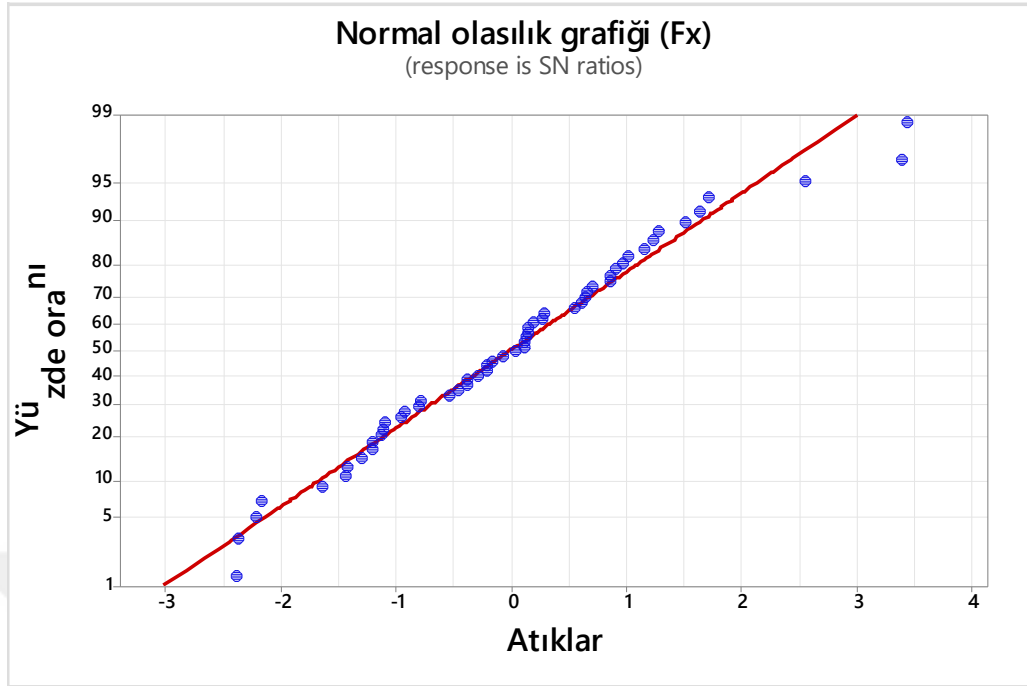
Şekil 4.5. Kesme kuvvetleri (Fx) için normal olasılık grafiği
