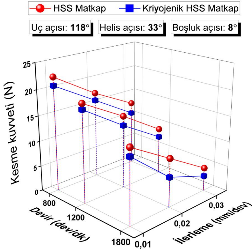
Şekil 4.9. 118° uç açısı, 33° helis açısı ve 8° boşluk açısına sahip matkaplarda kesme kuvveti
