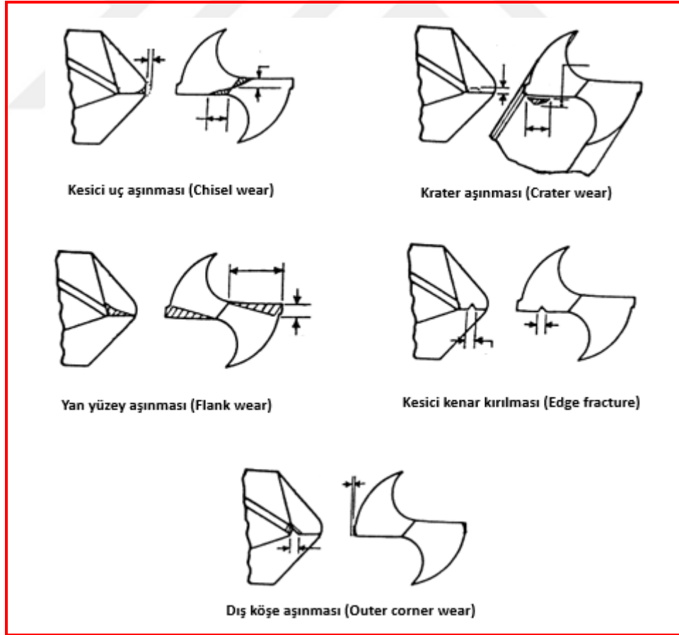
Şekil 4.118. Kesici takım matkapta meydana gelen aşınmaların türleri (Abu-Mahfouz, 2003)
