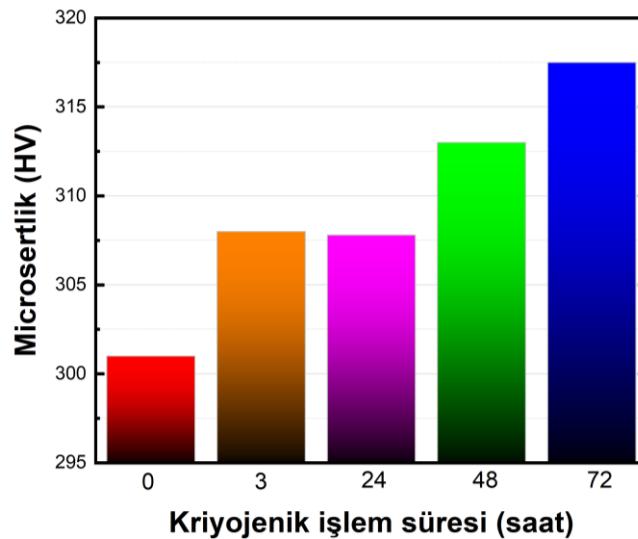
Şekil 1.27. Kriyojenik işlem sürelerinin mikrosertlik değerine etkisi (Gu ve ark., 2014)
