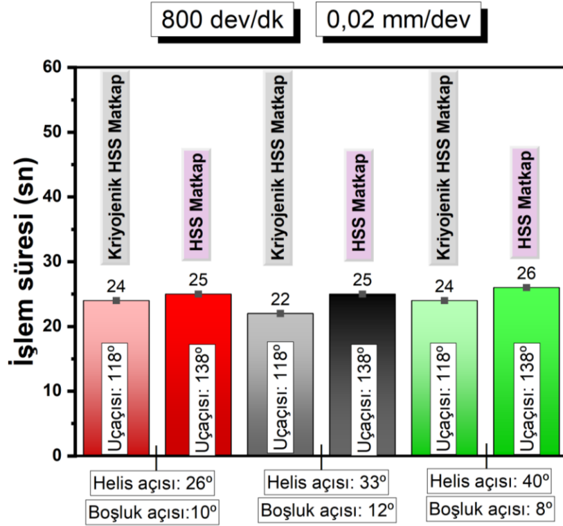
Şekil 4.113. HSS ve kriyojenik HSS matkapların aynı devir ve ilerlemedeki işleme süreleri
