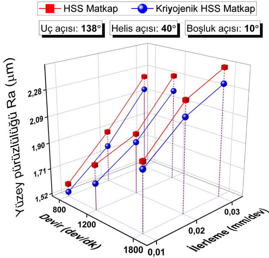
Şekil 4.62. 138^\circ uç açısı, 40^\circ helis açısı ve 10^\circ boşluk açılı matkaplar ile işlemede yüzey pürüzlülüğü
