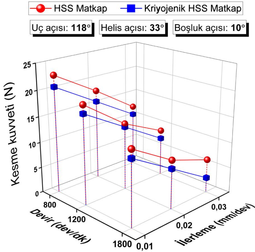
Şekil 4.10. 118° uç açısı, 33° helis açısı ve 10° boşluk açısına sahip matkaplarda kesme kuvveti
