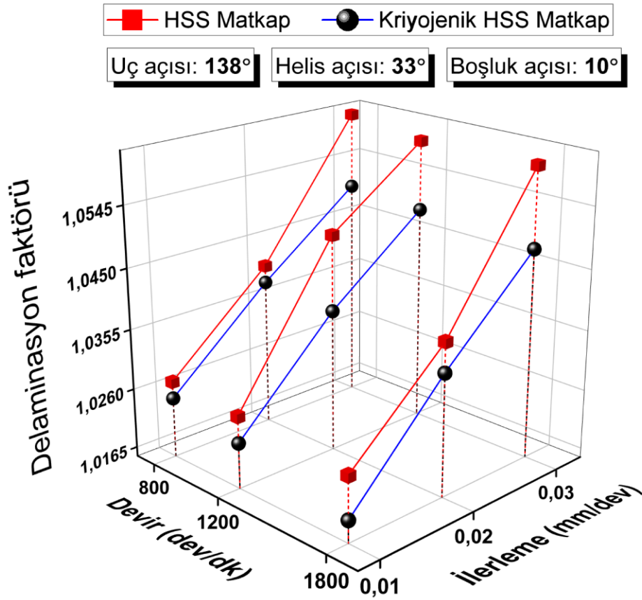
Şekil 4.91. 138^\circ uç açısı, 33^\circ helis açısı ve 10^\circ boşluk açılı matkaplar ile işlemede delaminasyon faktörü
