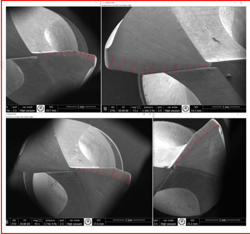
Şekil 4.120. Imagej programı ile kesici takımlar üzerinde hesaplanan aşınma değerleri
