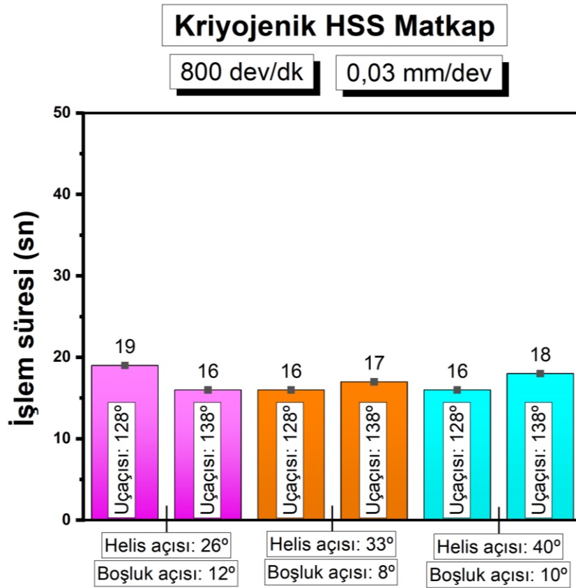
Şekil 4.110. Kriyojenik HSS matkapların 800 dev/dk ve 0,03 ilerleme hızındaki işleme süreleri
