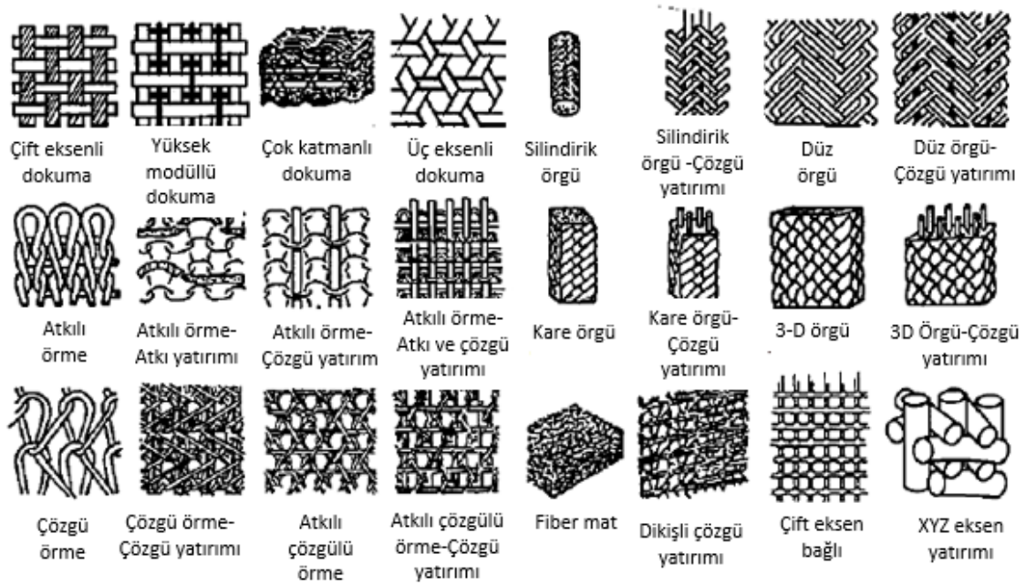
Şekil 1.6. Kompozit malzemelerde kullanılan elyaf dokumalarının çeşitleri (Buckley ve Edie, 1993)
