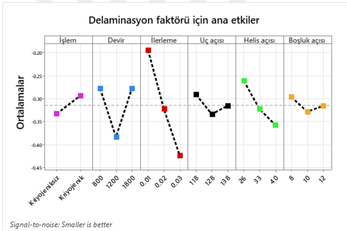
Şekil 4.66. Parametrelerin delaminasyon faktörü üzerindeki ana etkileri
