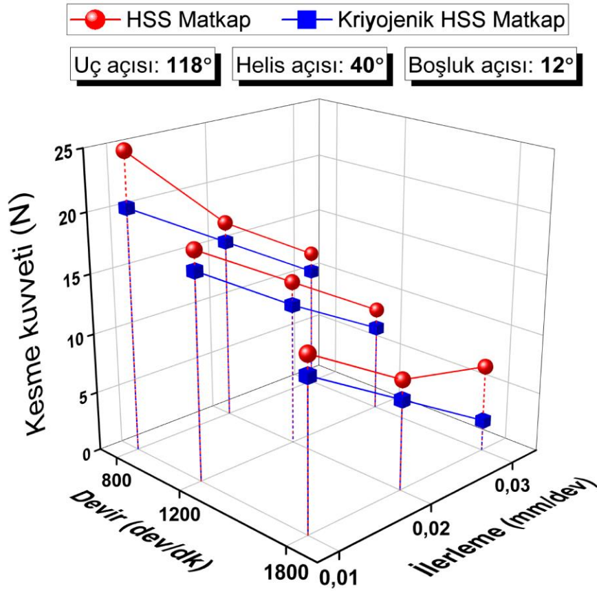
Şekil 4.14. 118° uç açısı, 40° helis açısı ve 12° boşluk açısına sahip matkaplarda kesme kuvveti
