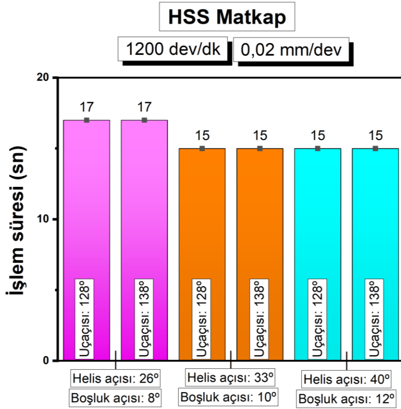
Şekil 4.108. HSS matkapların 1200 dev/dk ve 0,02 ilerleme hızındaki işleme süreleri
