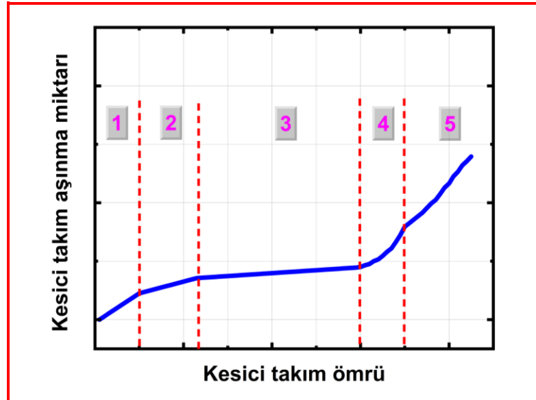
Şekil 4.117. Aşınma evreleri (Ertunç ve Sevim, 2011; Liu ve Anantharaman, 1994)
