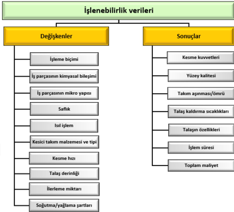
Şekil 1.9. Talaşlı üretimde işlenebilirlik verileri (Tinga, 2019)
