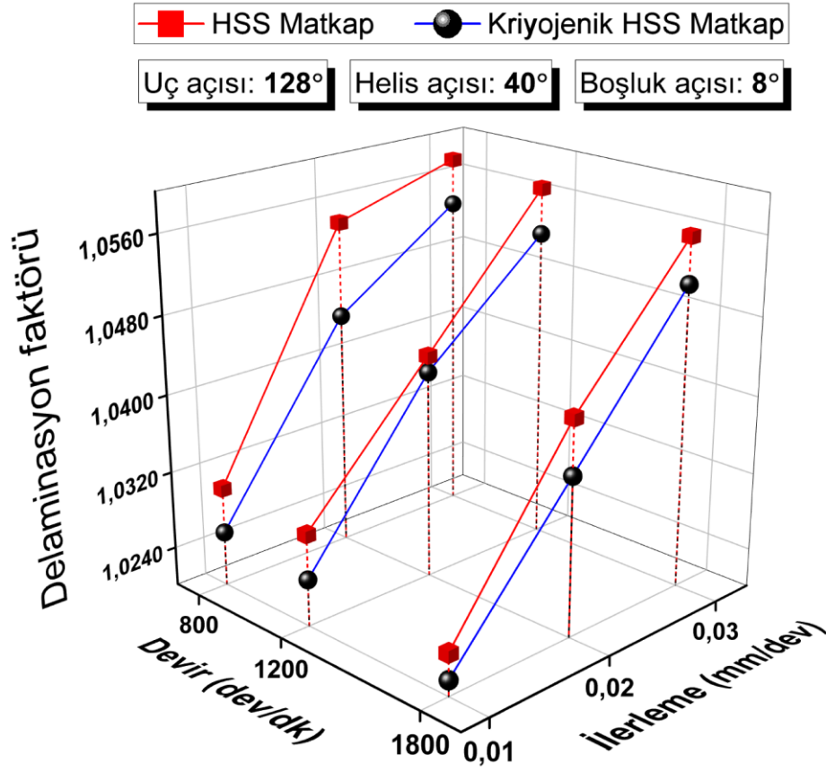
Şekil 4.84. 128° uç açısı, 40° helis açısı ve 8° boşluk açılı matkaplar ile işlemede delaminasyon faktörü
