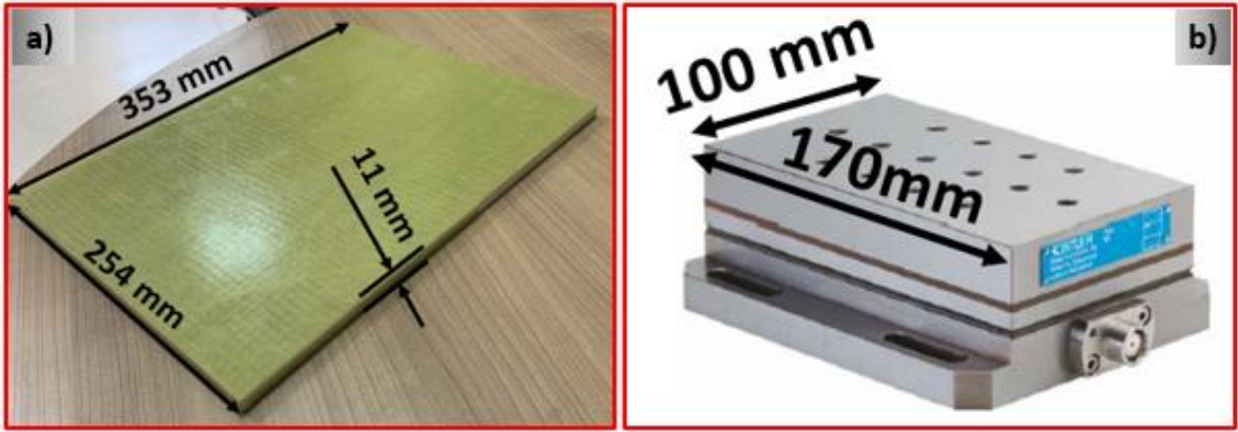
Şekil 3.1. Kompozit iş parçası (a) ve dinamometre (b) ebatları
