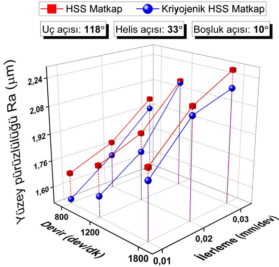
Şekil 4.41. 118^\circ uç açısı, 33^\circ helis açısı ve 10^\circ boşluk açılı matkaplar ile işlemede yüzey pürüzlülüğü
