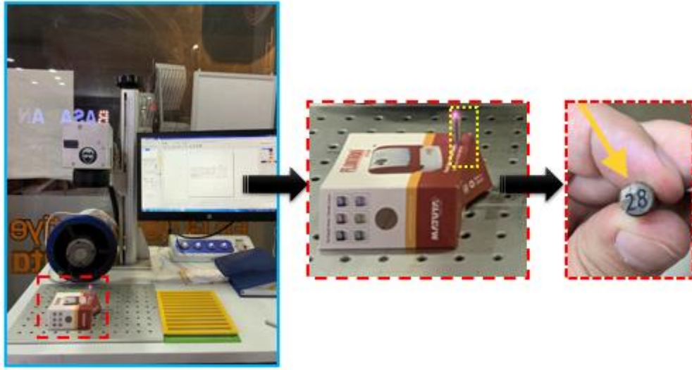
Şekil 3.4. Lazer sayı yazım cihazı
