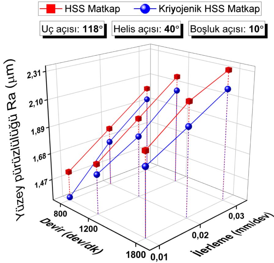
Şekil 4.44. 118° uç açısı, 40° helis açısı ve 10° boşluk açılı matkaplar ile işlemede yüzey pürüzlülüğü
