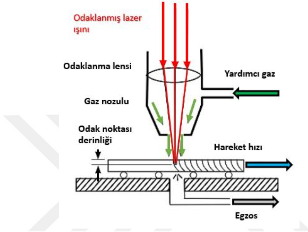
Şekil 1.13. Lazer ile delik delme işleminin şeması (Sheikh-Ahmad, 2009)
