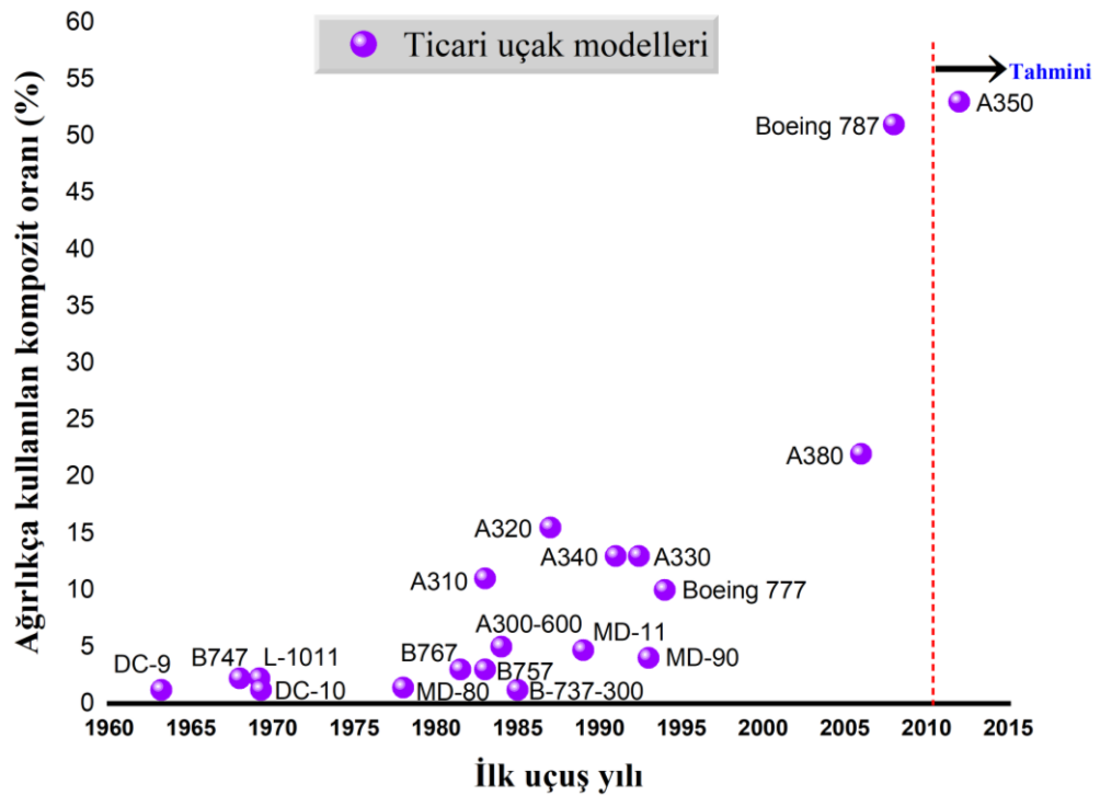
Şekil 1.2. Yolcu uçaklarında kullanılan kompozit malzemelerin yüzdelikleri (Safety, 2011)
