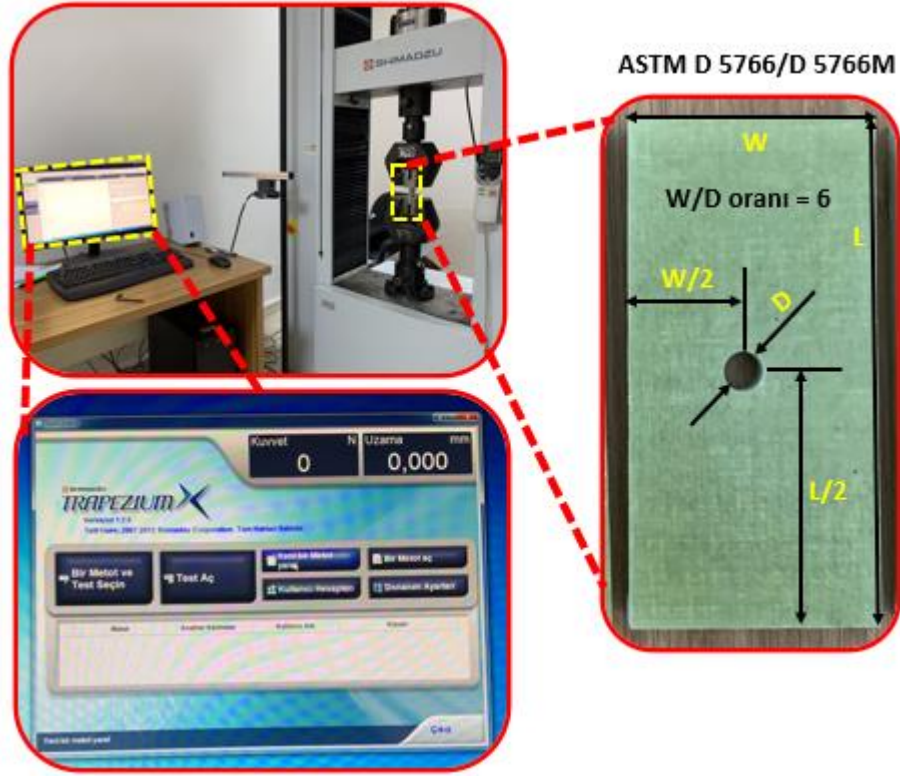
Şekil 3.20. Çekme testi cihazı, ASTM standardına göre numune ve Trapezium yazılımı
