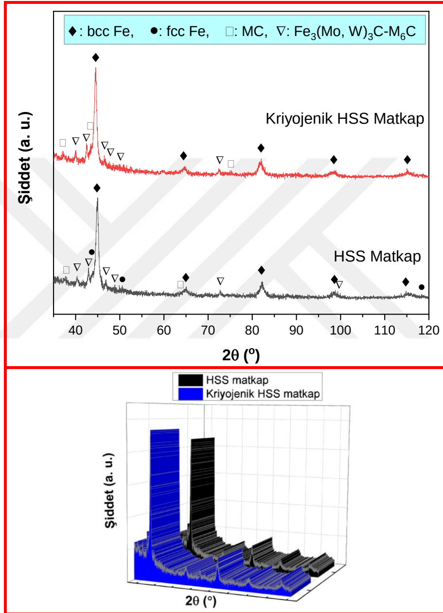
Şekil 4.2. XRD analizi sonuçları
