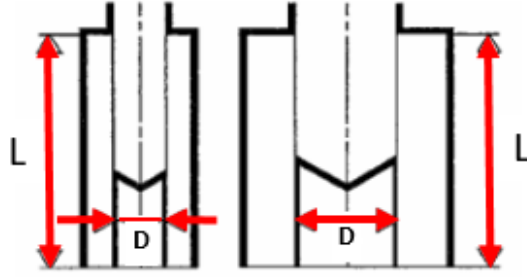
Şekil 1.21. Delik boyu ve delik çapı gösterimi (Çakır, 2000)
