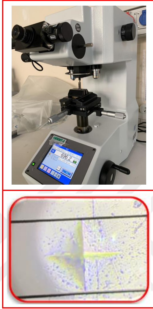
Şekil 3.10. Mikrosertlik ölçüm cihazı ve ölçüm esnasındaki görüntüsü
