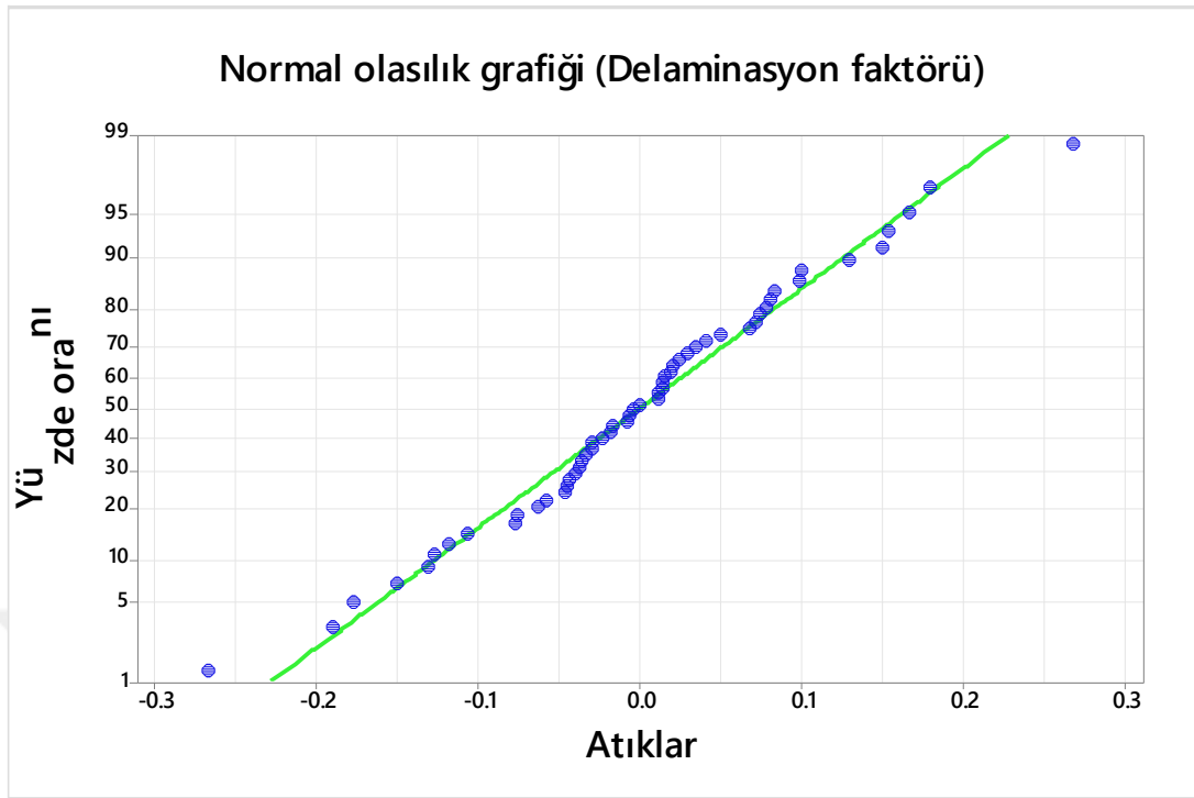
Şekil 4.67. Parametrelerin delaminasyon faktörü için normal olasılık grafiği
