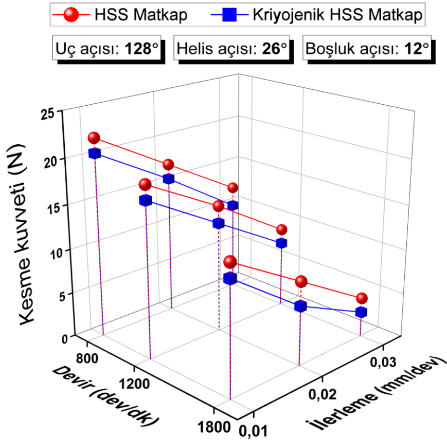
Şekil 4.17. 128° uç açısı, 26° helis açısı ve 12° boşluk açısına sahip matkaplarda kesme kuvveti
