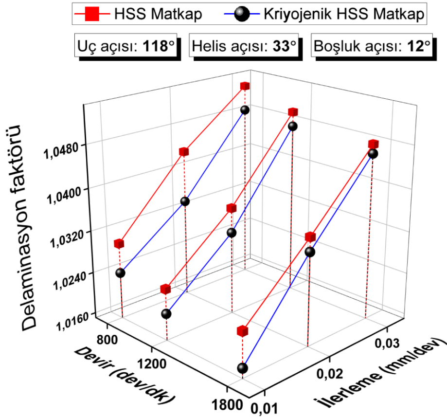
Şekil 4.74. 118^\circ uç açısı, 33^\circ helis açısı ve 12^\circ boşluk açılı matkaplar ile işlemede delaminasyon faktörü
