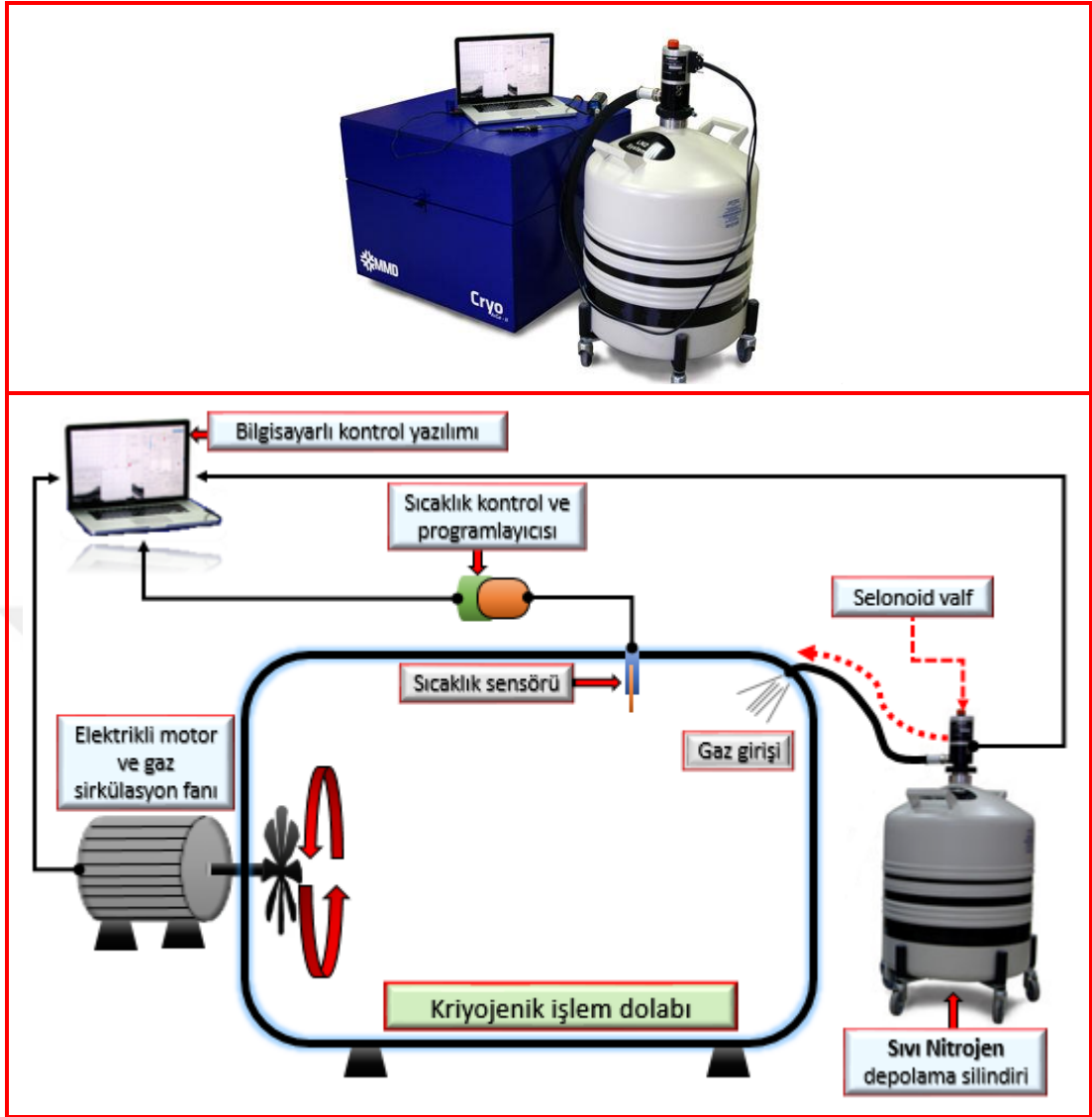
Şekil 3.9. Kriyojenik işlem cihazı ve işlem şeması
