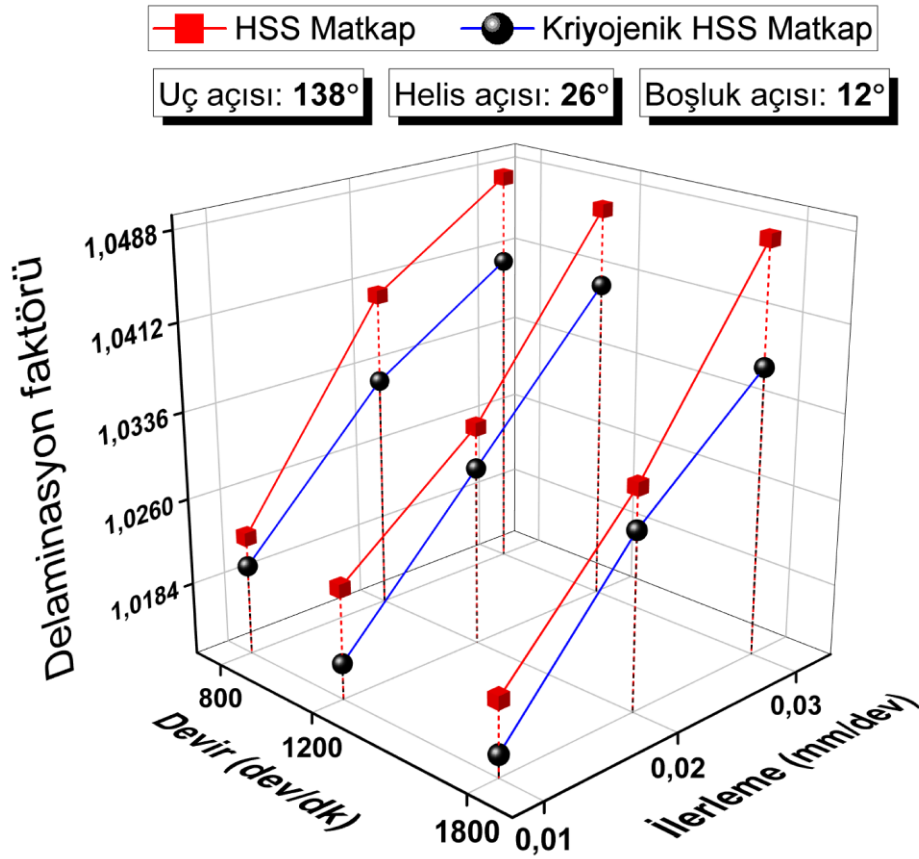
Şekil 4.89. 138° uç açısı, 26° helis açısı ve 12° boşluk açılı matkaplar ile işlemede delaminasyon faktörü
