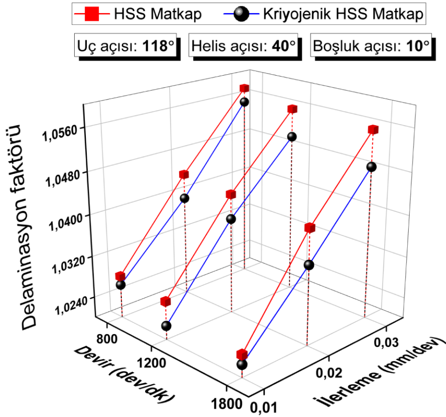
Şekil 4.76. 118° uç açısı, 40° helis açısı ve 10° boşluk açılı matkaplar ile işlemede delaminasyon faktörü
