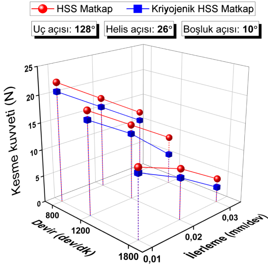
Şekil 4.16. 128° uç açısı, 26° helis açısı ve 10° boşluk açısına sahip matkaplarda kesme kuvveti
