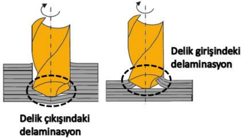
Şekil 1.17. Kompozit iş parçasında meydana gelen delaminasyonlar (Sheikh-Ahmad, 2009)
