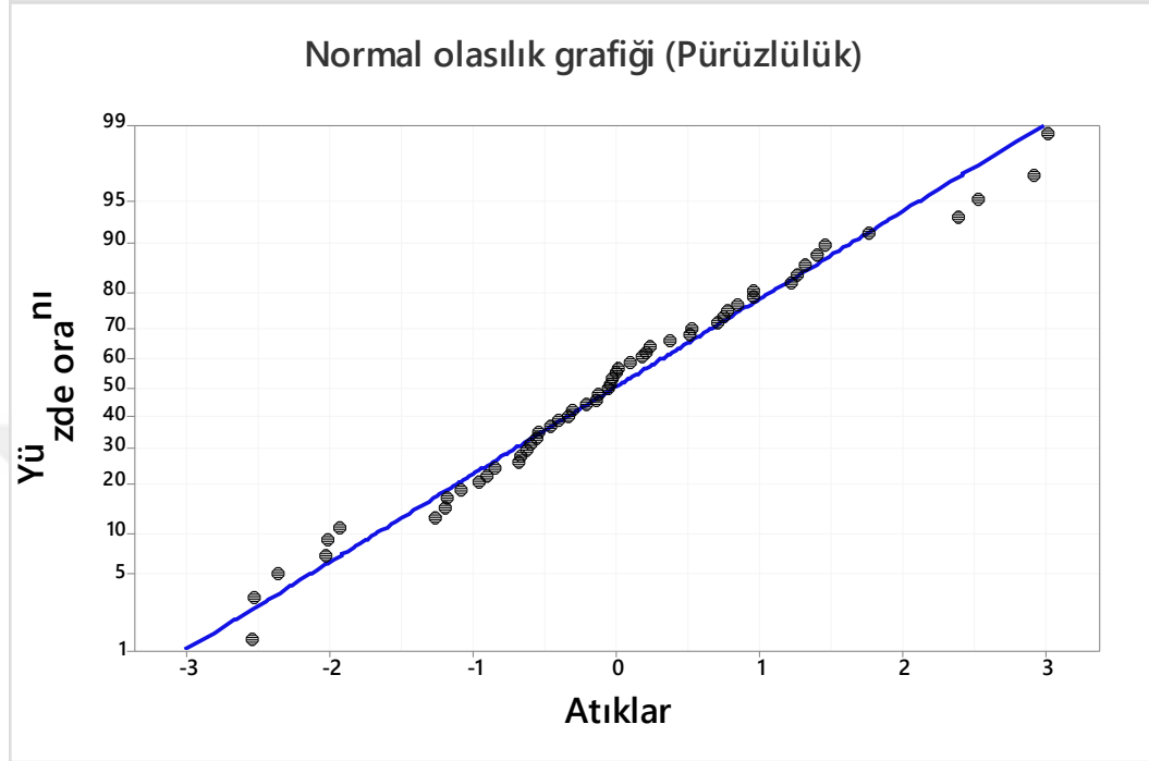
Şekil 4.35. Faktörlerin Yüzey pürüzlülüğü (Ra) için normal olasılık grafiği
