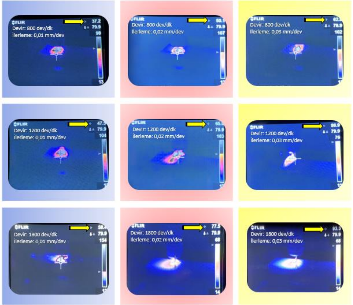
Şekil 4.33. Devir ve ilerleme artışına bağlı sıcaklık değişimleri
