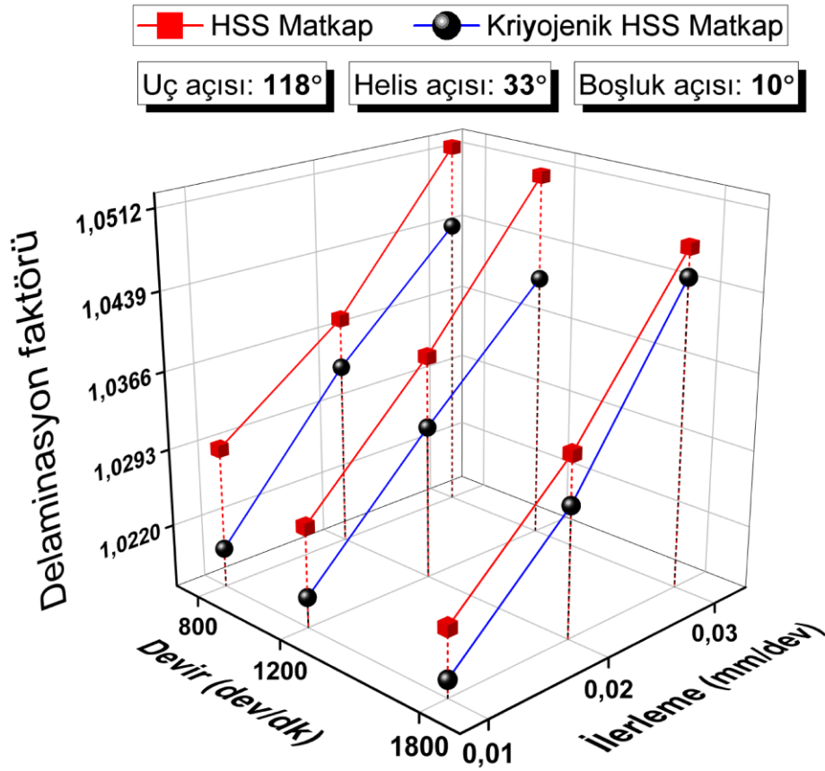
Şekil 4.73. 118° uç açısı, 33° helis açısı ve 10° boşluk açılı matkaplar ile işlemede delaminasyon faktörü
