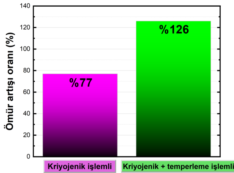
Şekil 1.29. Kriyojenik ve temperleme işlemlerinin takım ömrüne etkisi (Firouzdor ve ark., 2008)
