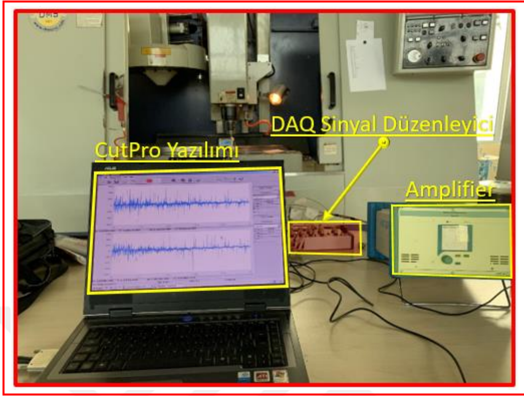
Şekil 3.15. Amplifier, DAQ sinyal düzenleyici ve CutPro yazılım programı
