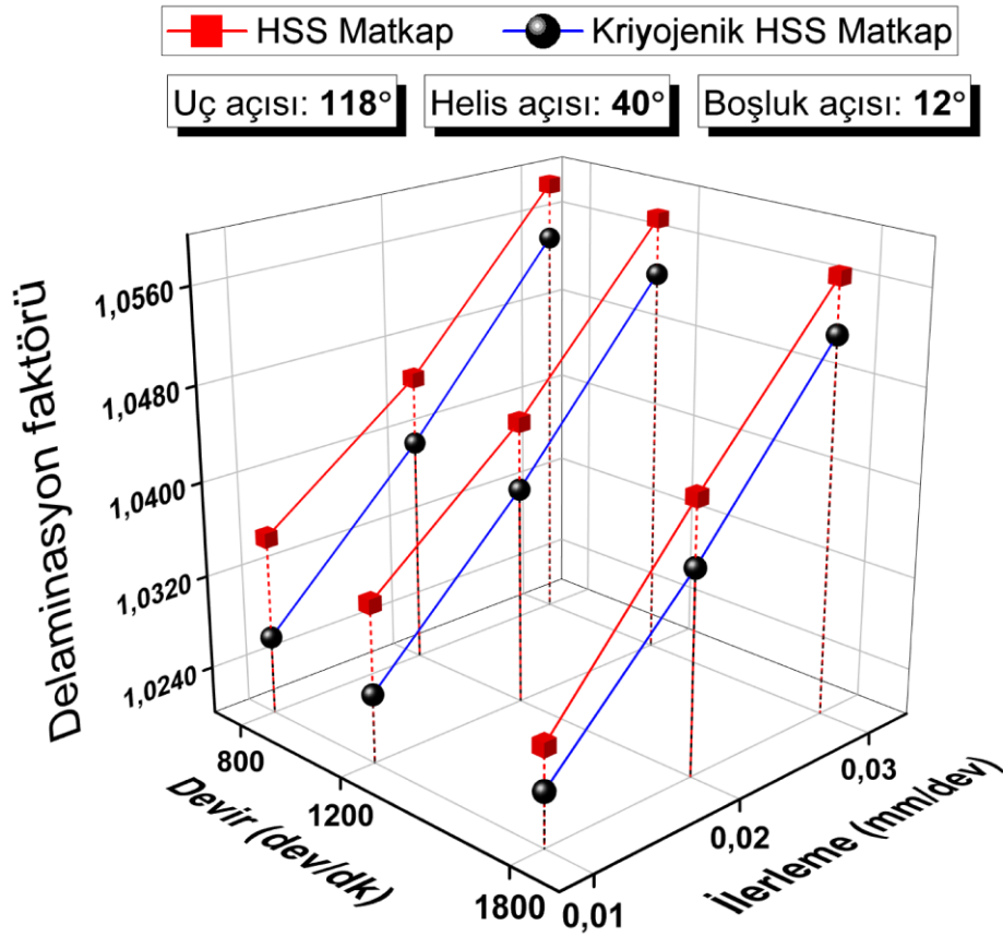
Şekil 4.77. 118° uç açısı, 40° helis açısı ve 12° boşluk açılı matkaplar ile işlemede delaminasyon faktörü
