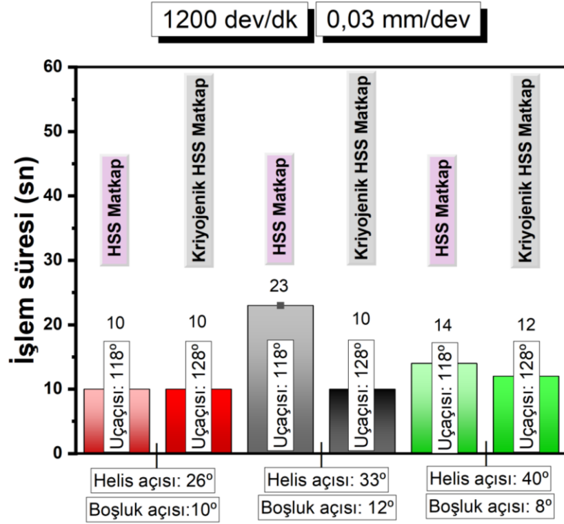
Şekil 4.114. HSS ve kriyojenik HSS matkapların aynı devir ve ilerlemedeki işleme süreleri
