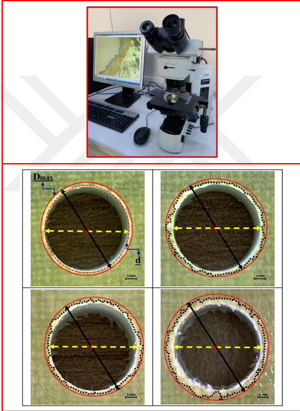
Şekil 3.17. Mikroskop cihazı ve delaminasyon faktörü ölçümü
