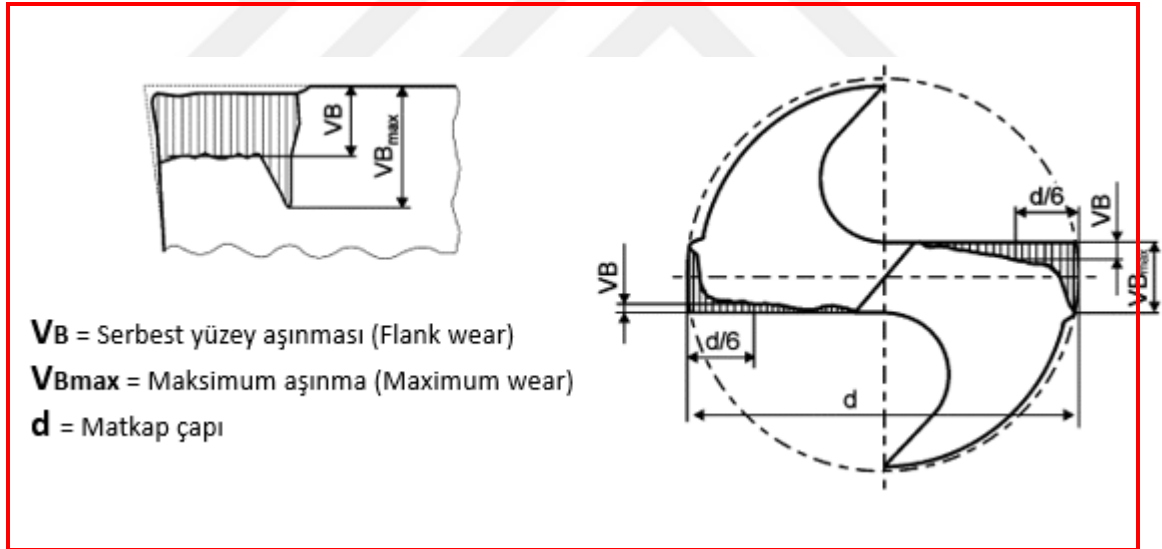
Şekil 4.119. Matkapta serbest yüzey aşınmasını ölçme şeması (Dolinšek ve ark., 2001)
