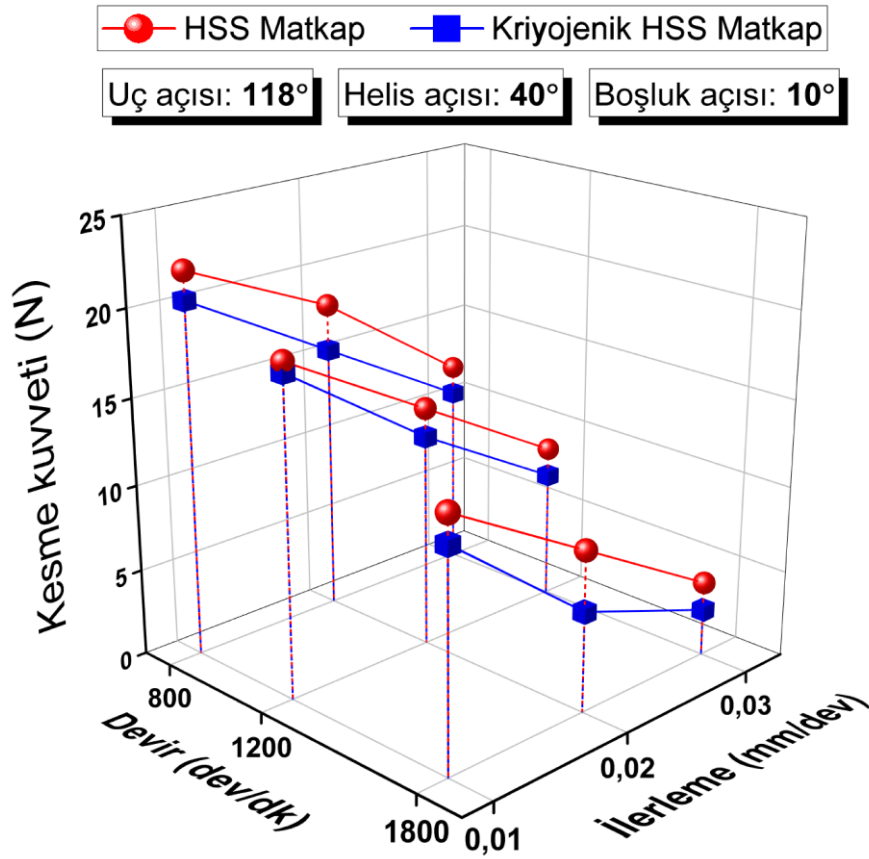
Şekil 4.13. 118° uç açısı, 40° helis açısı ve 10° boşluk açısına sahip matkaplarda kesme kuvveti
