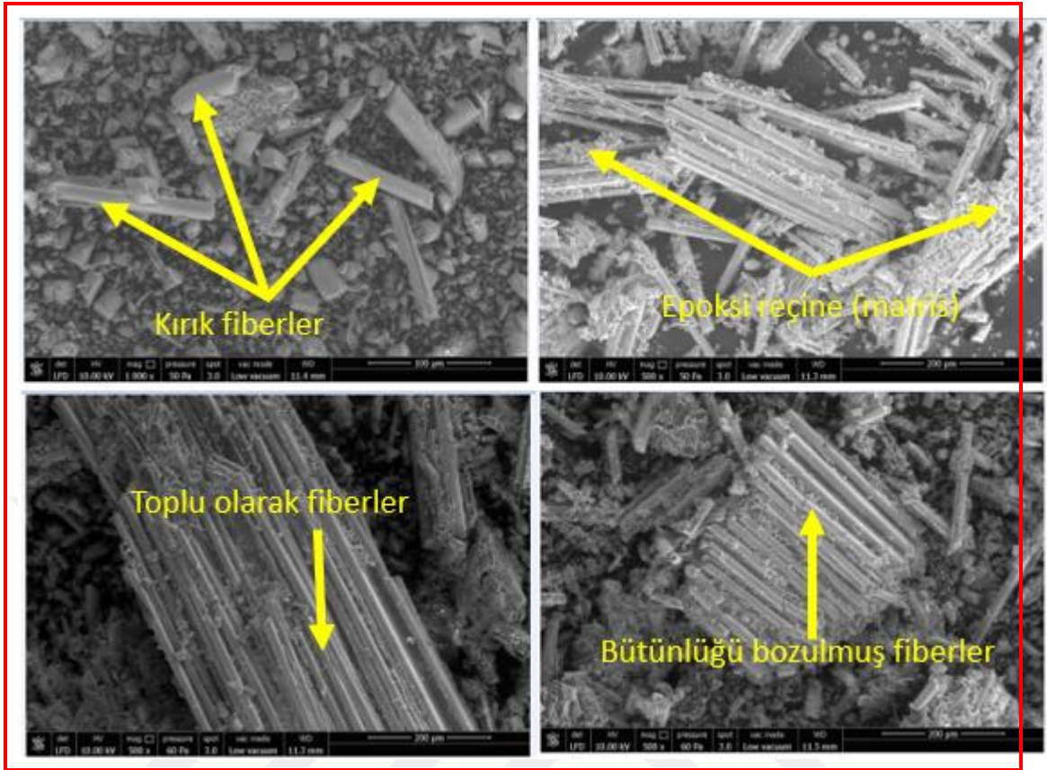
Şekil 4.102. Farklı parametrelerde açılmış deliklerden çıkan talaşların SEM görüntüleri
