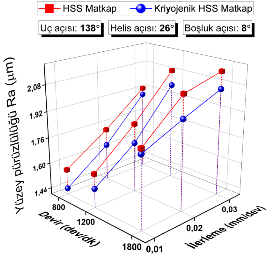
Şekil 4.55. 138° uç açısı, 26° helis açısı ve 8° boşluk açılı matkaplar ile işlemede yüzey pürüzlülüğü
