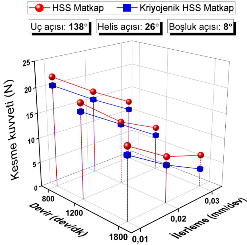
Şekil 4.24. 138° uç açısı, 26° helis açısı ve 8° boşluk açısına sahip matkaplarda kesme kuvveti
