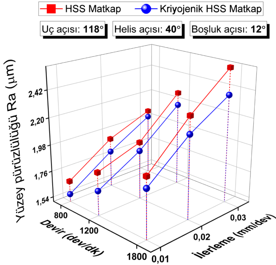
Şekil 4.45. 118° uç açısı, 40° helis açısı ve 12° boşluk açılı matkaplar ile işlemede yüzey pürüzlülüğü
