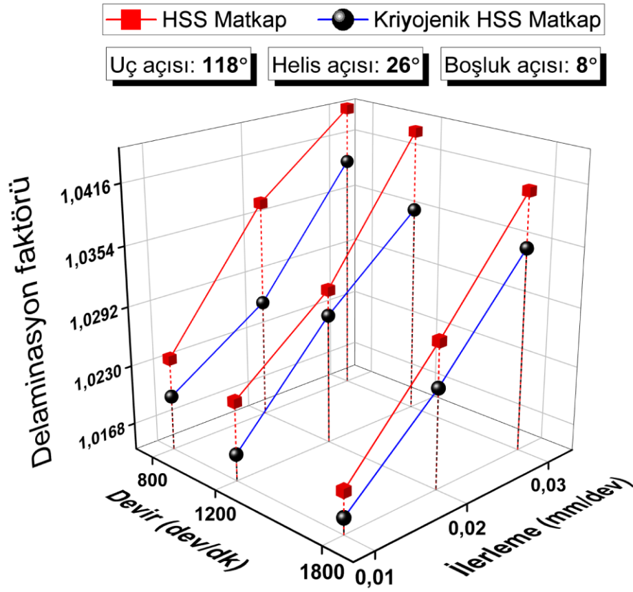
Şekil 4.69. 118^\circ uç açısı, 26^\circ helis açısı ve 8^\circ boşluk açılı matkaplar ile işlemede delaminasyon faktörü
