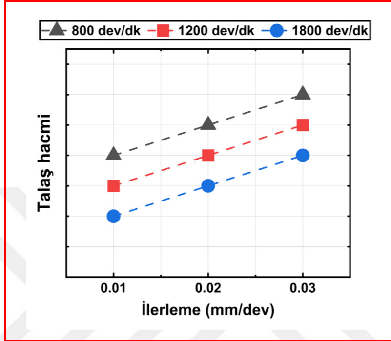
Şekil 4.101. Devir ve ilerleme hızına bağlı olarak talaş hacmi değişimi
