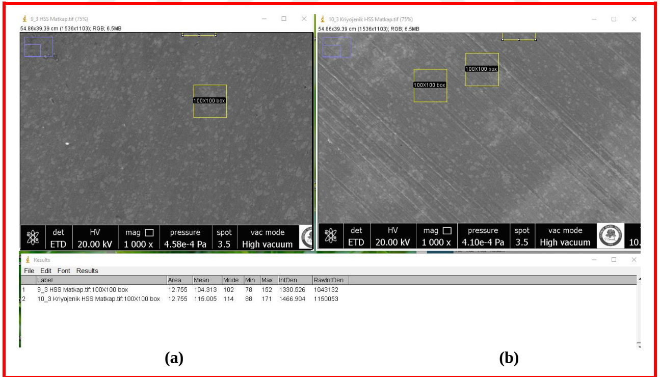
Şekil 4.1. HSS matkap (a) ile kriyojenik ve temperleme işlemleri görmüş HSS matkap (b) SEM görüntüleri
