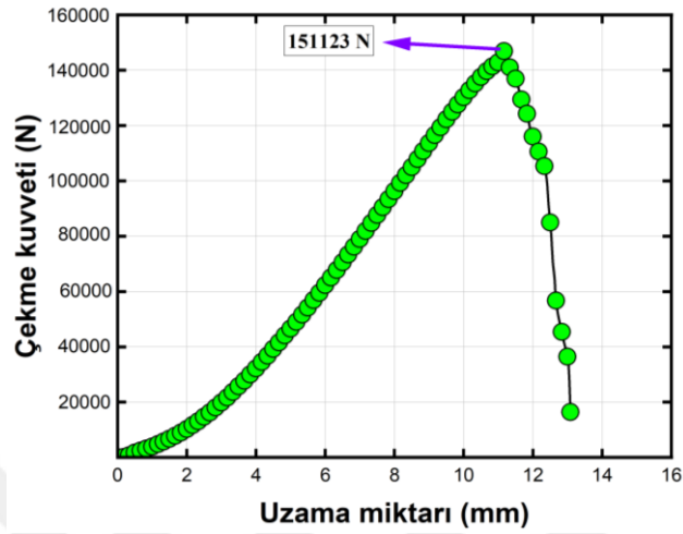
Şekil 4.132. Delik açılmayan numunenin çekme grafiği
