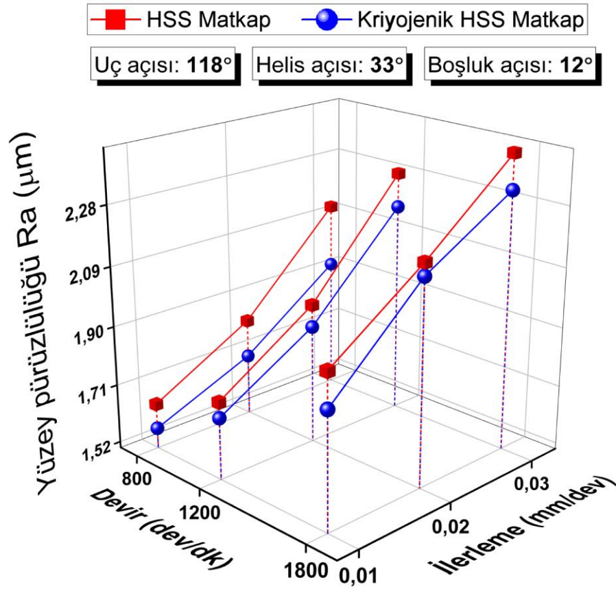
Şekil 4.42. 118° uç açısı, 33° helis açısı ve 12° boşluk açılı matkaplar ile işlemede yüzey pürüzlülüğü
