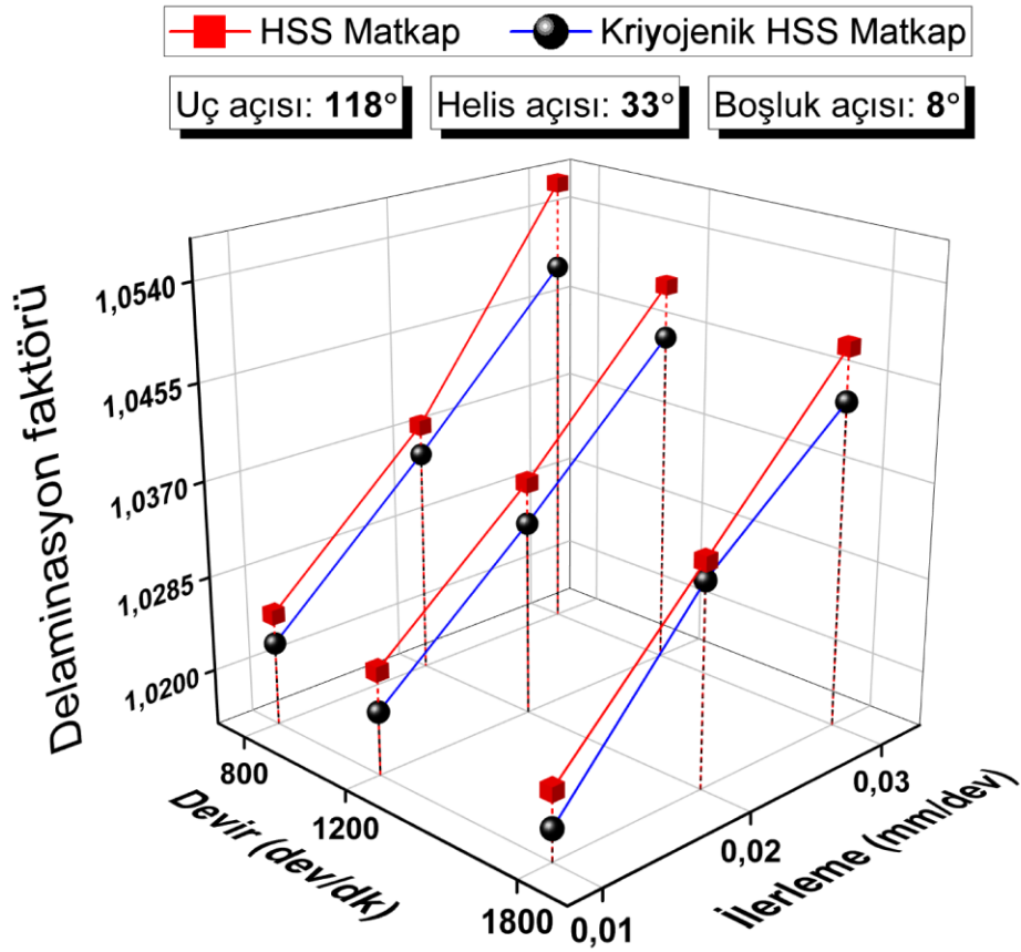
Şekil 4.72. 118° uç açısı, 33° helis açısı ve 8° boşluk açılı matkaplar ile işlemede delaminasyon faktörü
