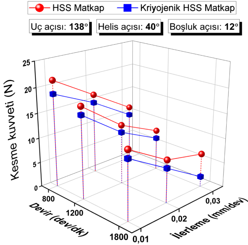
Şekil 4.32. 138° uç açısı, 40° helis açısı ve 12° boşluk açısına sahip matkaplarda kesme kuvveti
