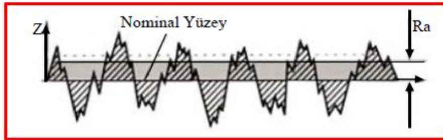
Şekil 4.36. Ortalama yüzey pürüzlülüğü (Ra) (Demir ve Toktaş, 2014)
