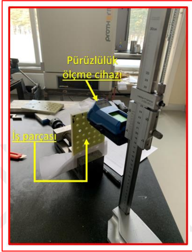
Şekil 3.16. Yüzey pürüzlüğü ölçme cihazı
