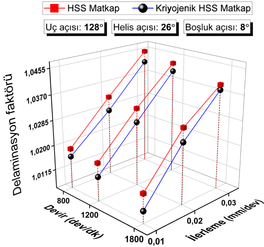
Şekil 4.78. 128° uç açısı, 26° helis açısı ve 8° boşluk açılı matkaplar ile işlemede delaminasyon faktörü
