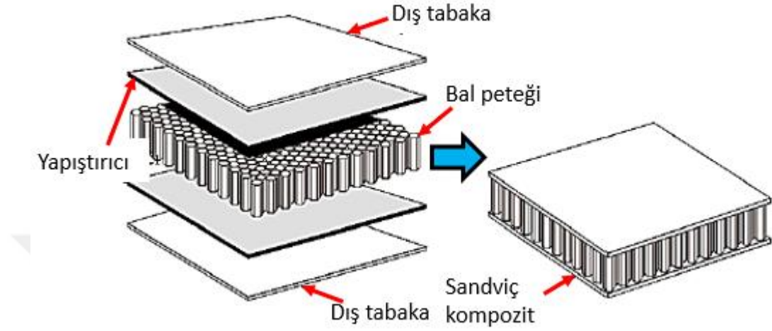
Şekil 1.7. Sandviç kompozitin temel yapısı (Sheehan, 1987)
