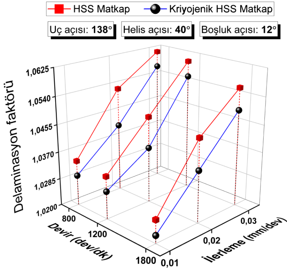
Şekil 4.95. 138° uç açısı, 40° helis açısı ve 12° boşluk açılı matkaplar ile işlemede delaminasyon faktörü
