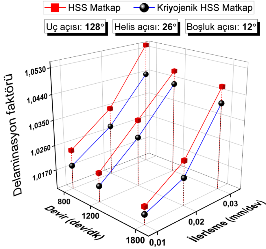
Şekil 4.80. 128° uç açısı, 26° helis açısı ve 12° boşluk açılı matkaplar ile işlemede delaminasyon faktörü
