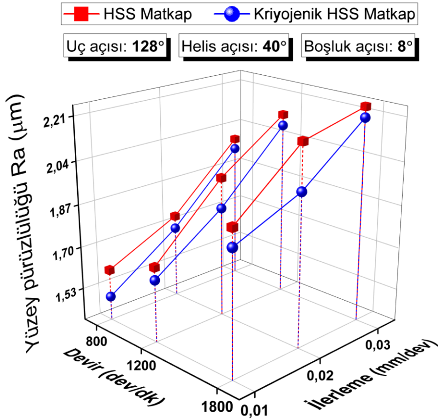
Şekil 4.52. 128° uç açısı, 40° helis açısı ve 8° boşluk açılı matkaplar ile işlemede yüzey pürüzlülüğü
