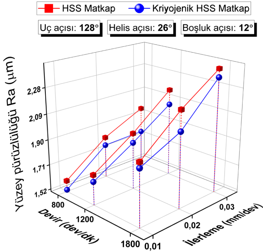
Şekil 4.48. 128° uç açısı, 26° helis açısı ve 12° boşluk açılı matkaplar ile işlemede yüzey pürüzlülüğü
