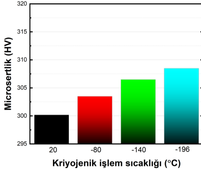
Şekil 1.28. Kriyojenik işlem sıcaklıklarının mikrosertlik değerine etkisi (Gu ve ark., 2014)
