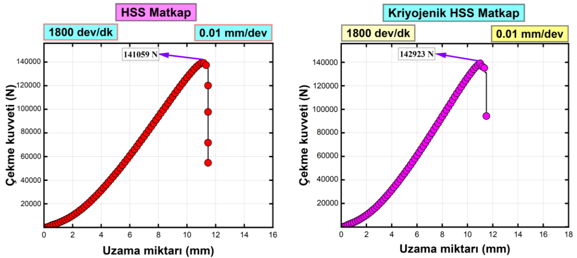
Şekil 4.133. 0,01 mm/dev ilerleme ile delik açılan numunelerin çekme grafikleri
