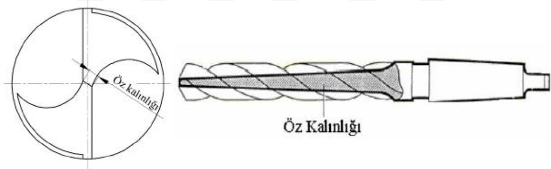
Şekil 1.23. Matkap öz kalınlığı (Kaynak, 2006)
