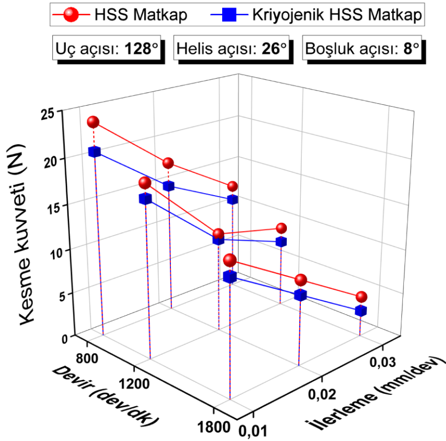
Şekil 4.15. 128° uç açısı, 26° helis açısı ve 8° boşluk açısına sahip matkaplarda kesme kuvveti
