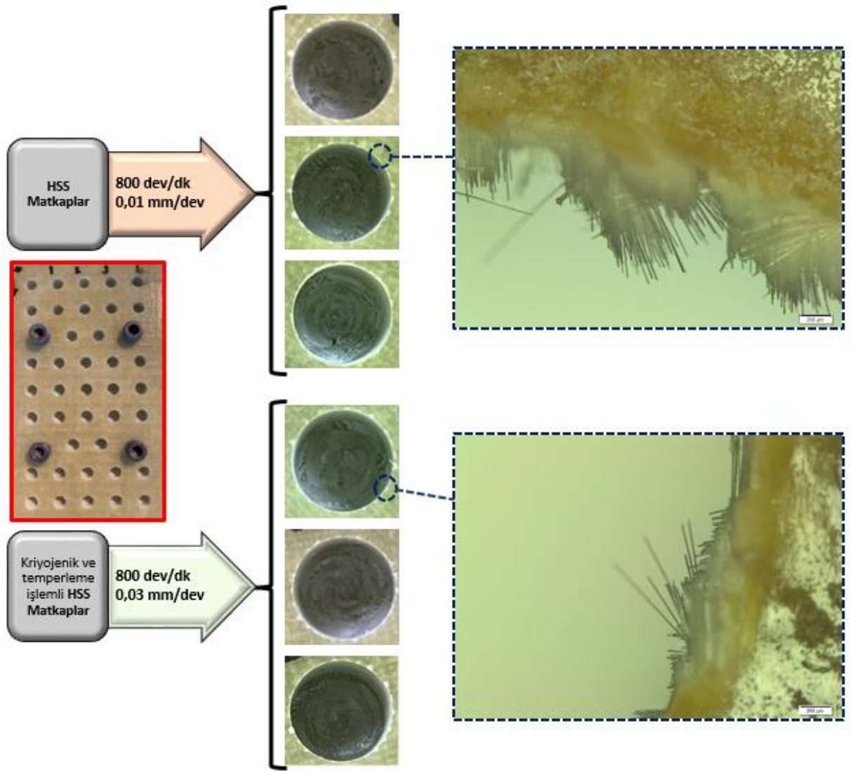
Şekil 4.96. Farklı matkaplar ile açılan deliklerin kenarlarının makro ve mikro resimleri
