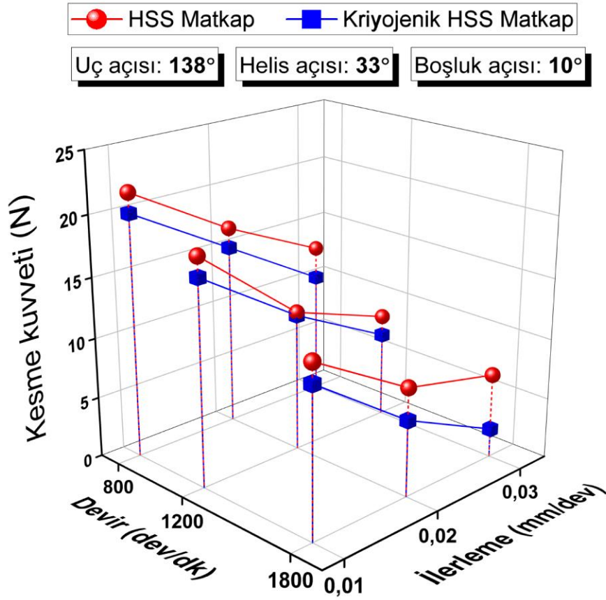
Şekil 4.28. 138° uç açısı, 33° helis açısı ve 10° boşluk açısına sahip matkaplarda kesme kuvveti
