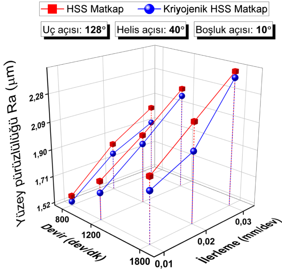
Şekil 4.53. 128° uç açısı, 40° helis açısı ve 10° boşluk açılı matkaplar ile işlemede yüzey pürüzlülüğü
