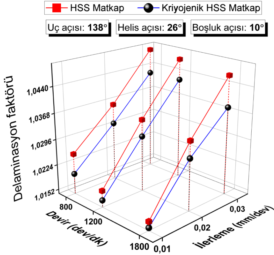
Şekil 4.88. 138° uç açısı, 26° helis açısı ve 10° boşluk açılı matkaplar ile işlemede delaminasyon faktörü
