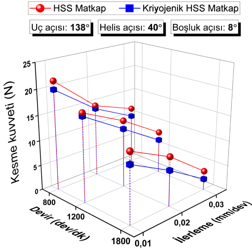
Şekil 4.30. 138° uç açısı, 40° helis açısı ve 8° boşluk açısına sahip matkaplarda kesme kuvveti
