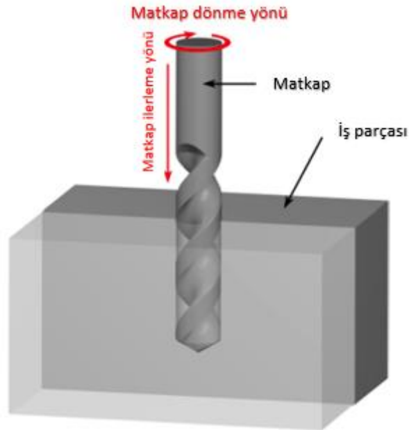
Şekil 1.11. Geleneksel delik delme işleminin mekanizması (Patel ve Verma, 2015)
