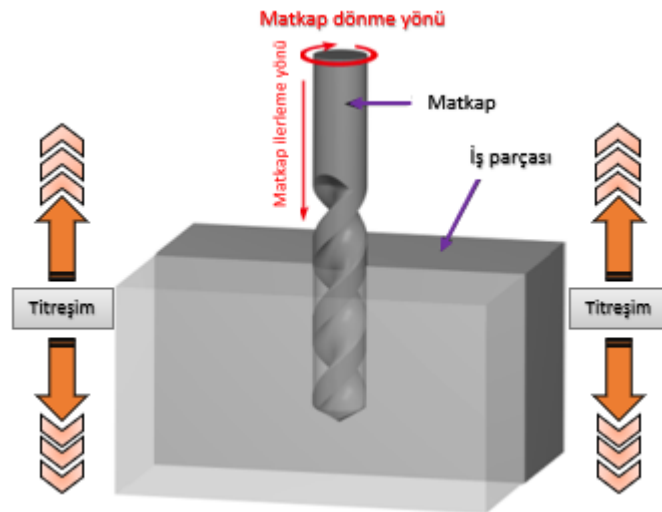
Şekil 1.15. Ultrasonik titreşim desteği yöntemi ile delme (Patel ve Verma, 2015; Xu ve ark., 2009)
