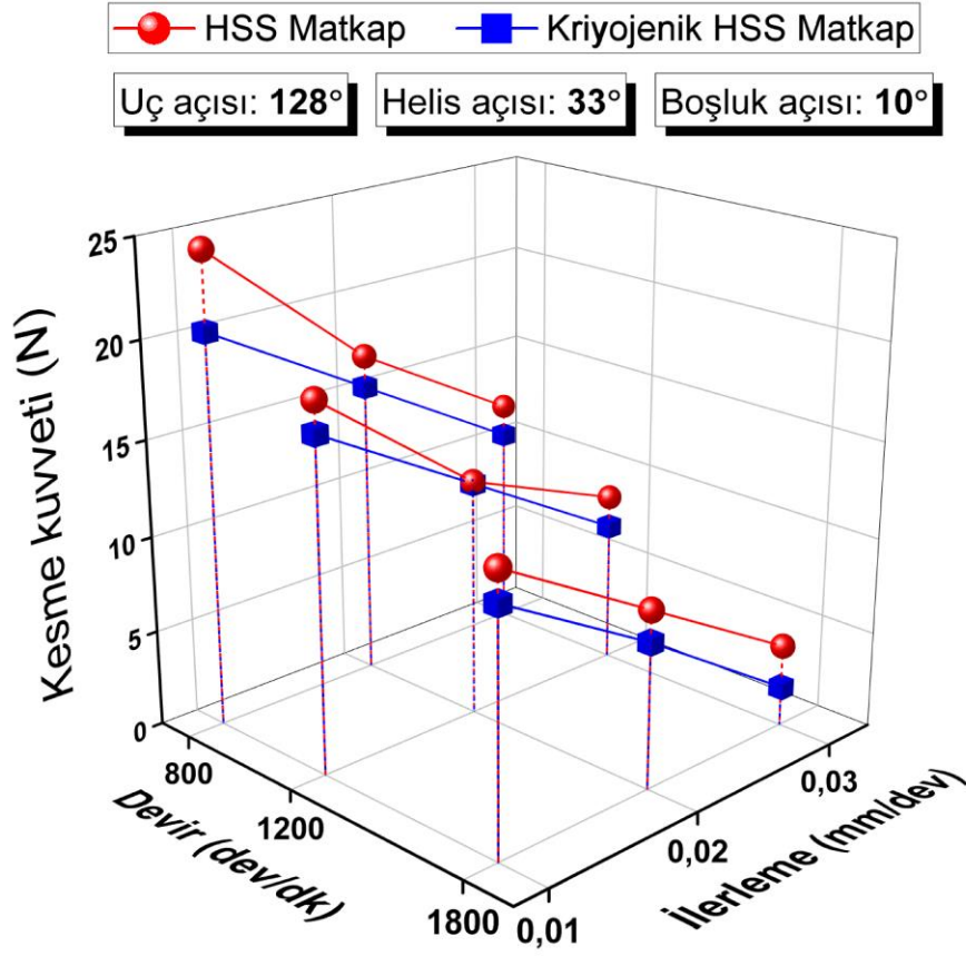
Şekil 4.19. 128° uç açısı, 33° helis açısı ve 10° boşluk açısına sahip matkaplarda kesme kuvveti
