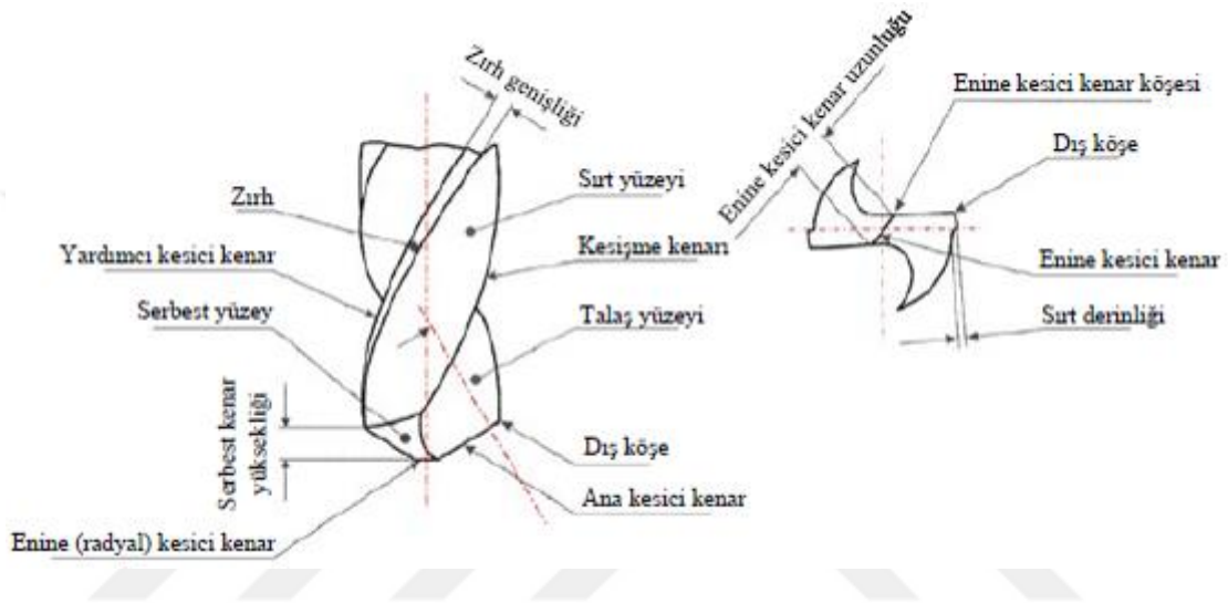
Şekil 1.22. Matkapta bulunan kesici kenar ve yüzeyler (Çakır ve ark., 2014)
