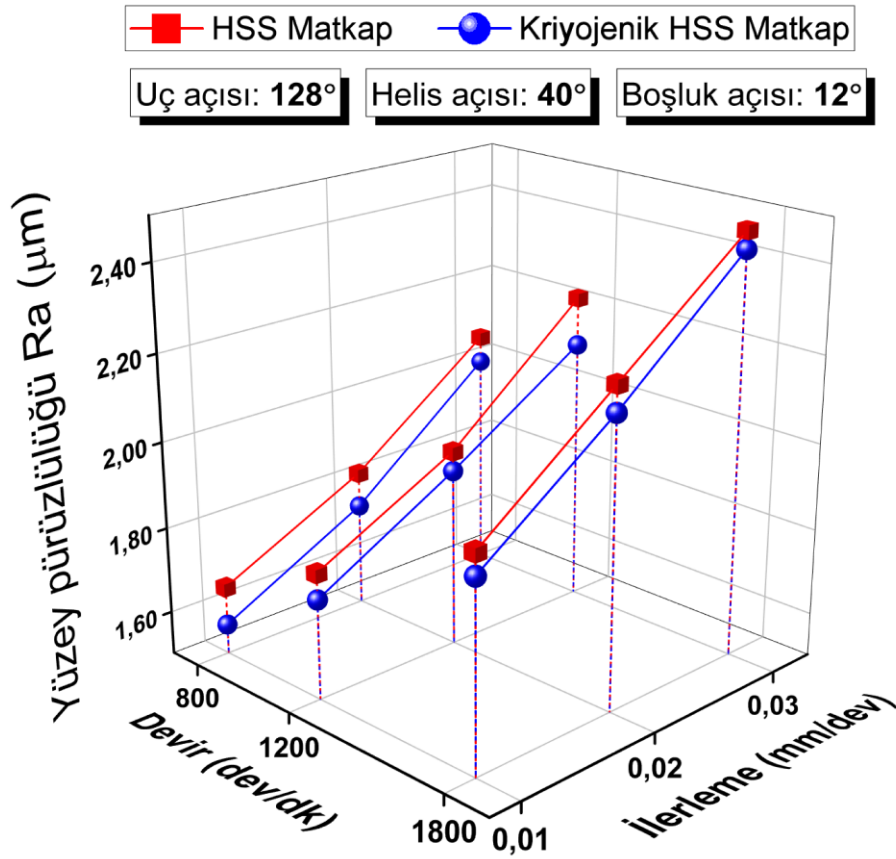
Şekil 4.54. 128^\circ uç açısı, 40^\circ helis açısı ve 12^\circ boşluk açılı matkaplar ile işlemede yüzey pürüzlülüğü
