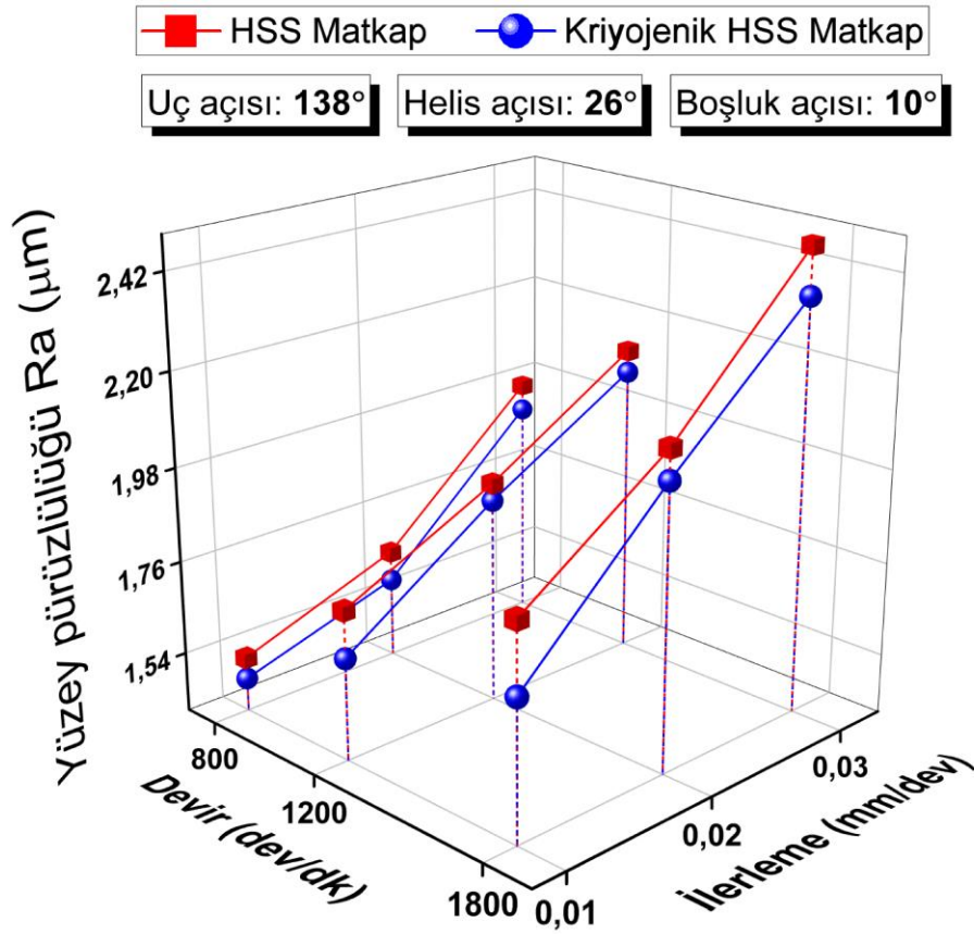
Şekil 4.56. 138^\circ uç açısı, 26^\circ helis açısı ve 10^\circ boşluk açılı matkaplar ile işlemede yüzey pürüzlülüğü
