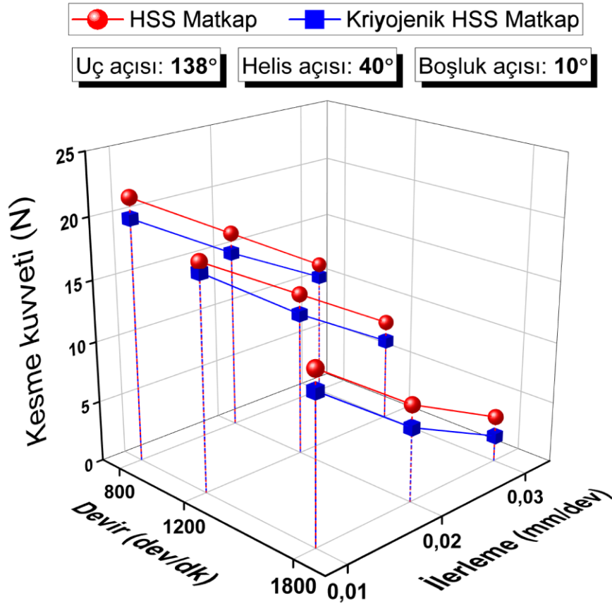
Şekil 4.31. 138° uç açısı, 40° helis açısı ve 10° boşluk açısına sahip matkaplarda kesme kuvveti
