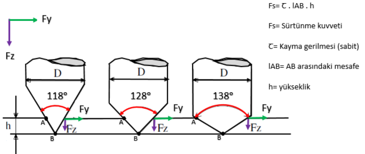
Şekil 4.99. Delik girişinde oluşan kuvvetler ve matkap uç açısının etkileri (Ekici, 2009)
