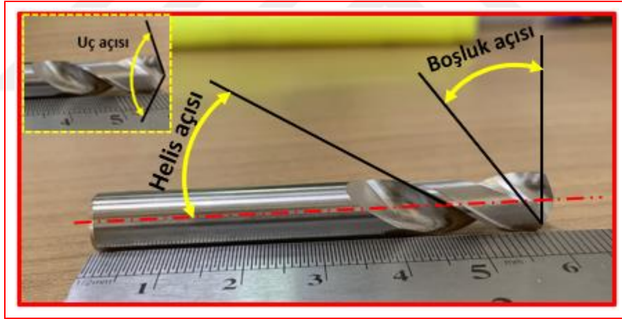
Şekil 3.6. Kesici takım matkabın geometrik ölçülerinin isimleri
