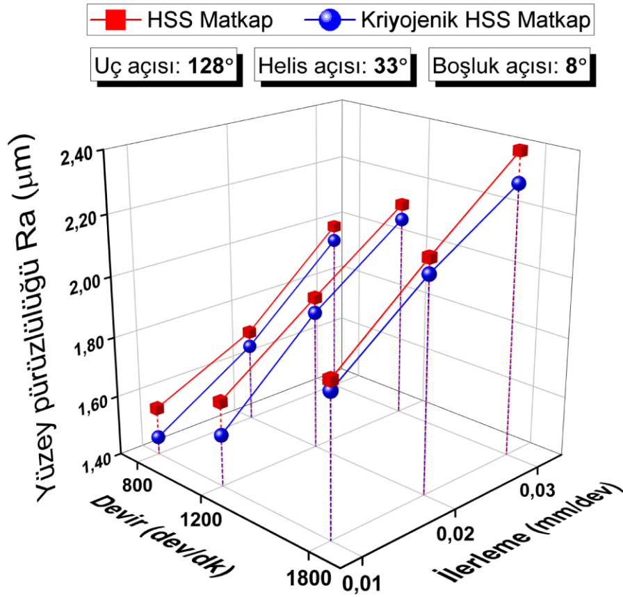
Şekil 4.49. 128^\circ uç açısı, 33^\circ helis açısı ve 8^\circ boşluk açılı matkaplar ile işlemede yüzey pürüzlülüğü
