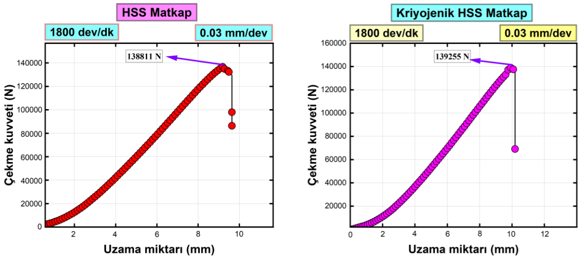
Şekil 4.135. 0,03 mm/dev ilerleme ile delik açılan numunelerin çekme grafikleri
