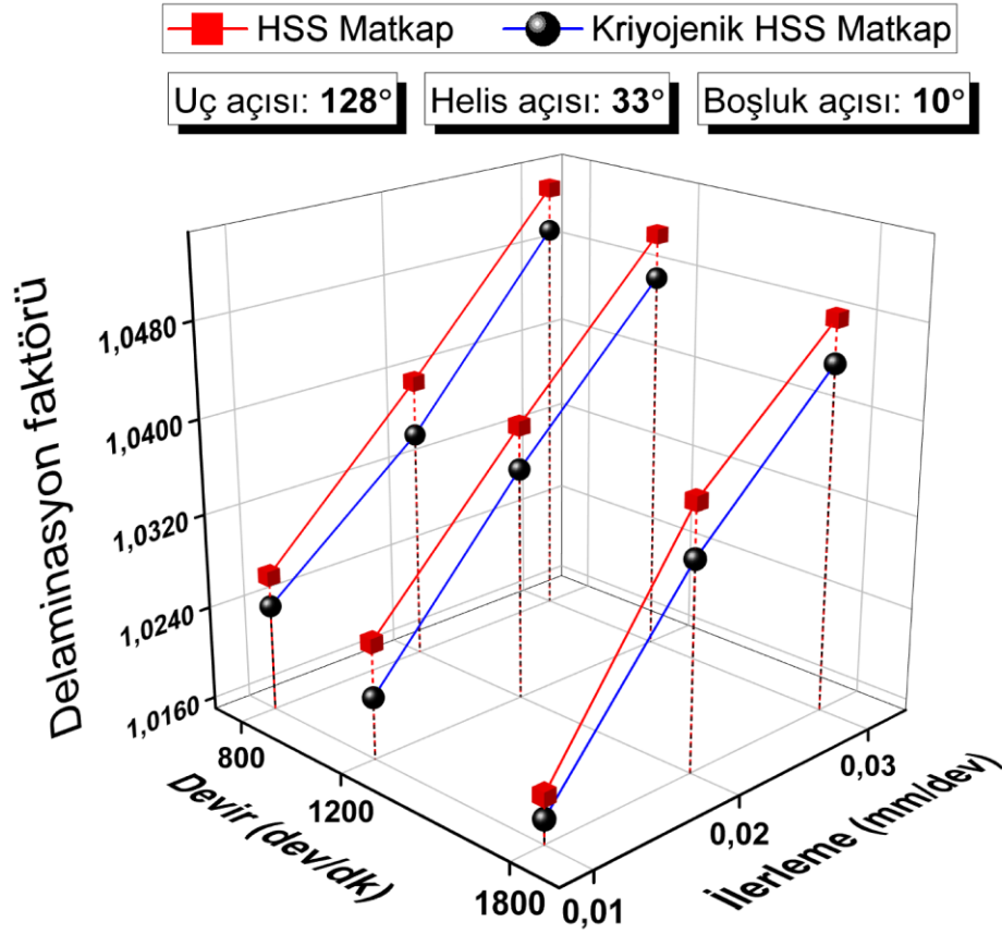
Şekil 4.82. 128° uç açısı, 33° helis açısı ve 10° boşluk açılı matkaplar ile işlemede delaminasyon faktörü
