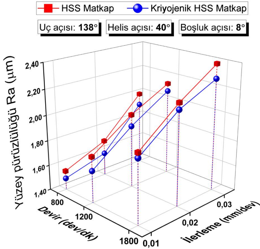
Şekil 4.61. 138^\circ uç açısı, 40^\circ helis açısı ve 8^\circ boşluk açılı matkaplar ile işlemede yüzey pürüzlülüğü
