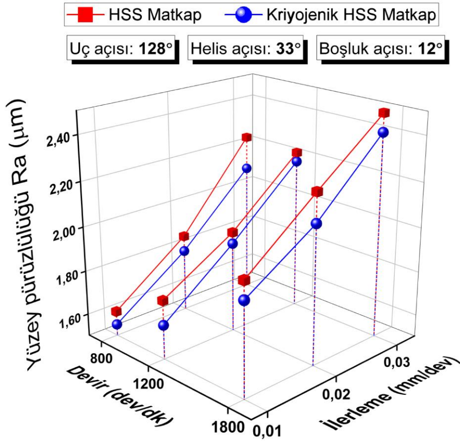
Şekil 4.51. 128° uç açısı, 33° helis açısı ve 12° boşluk açılı matkaplar ile işlemede yüzey pürüzlülüğü
