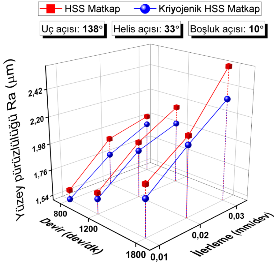
Şekil 4.59. 138° uç açısı, 33° helis açısı ve 10° boşluk açılı matkaplar ile işlemede yüzey pürüzlülüğü
