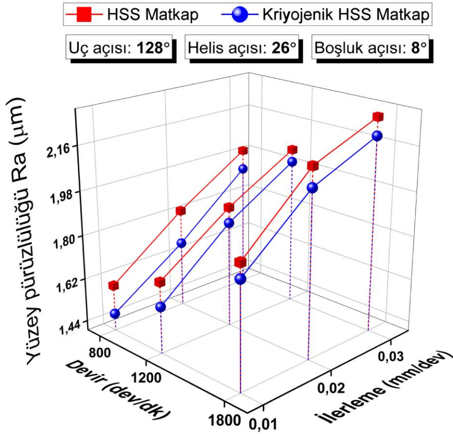
Şekil 4.46. 128° uç açısı, 26° helis açısı ve 8° boşluk açılı matkaplar ile işlemede yüzey pürüzlülüğü
