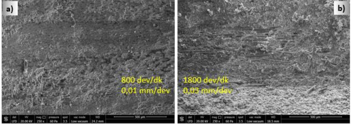
Şekil 4.65. Farklı devir ve ilerlemelerde delinen kompozitlerin delik duvarı SEM görüntüleri
