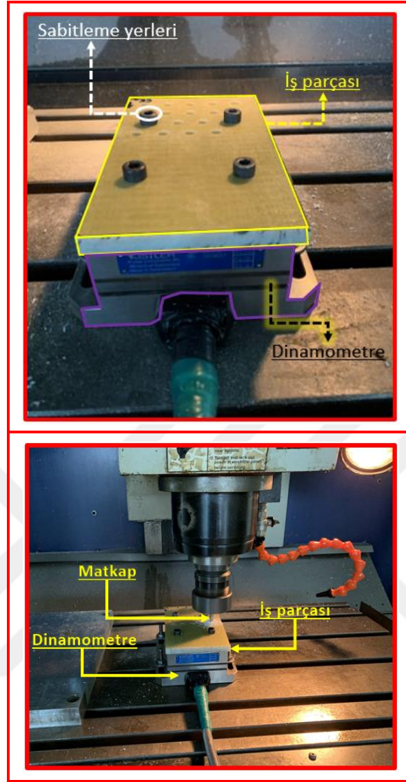
Şekil 3.14. İş parçasının dinamometreye bağlanmış hali
