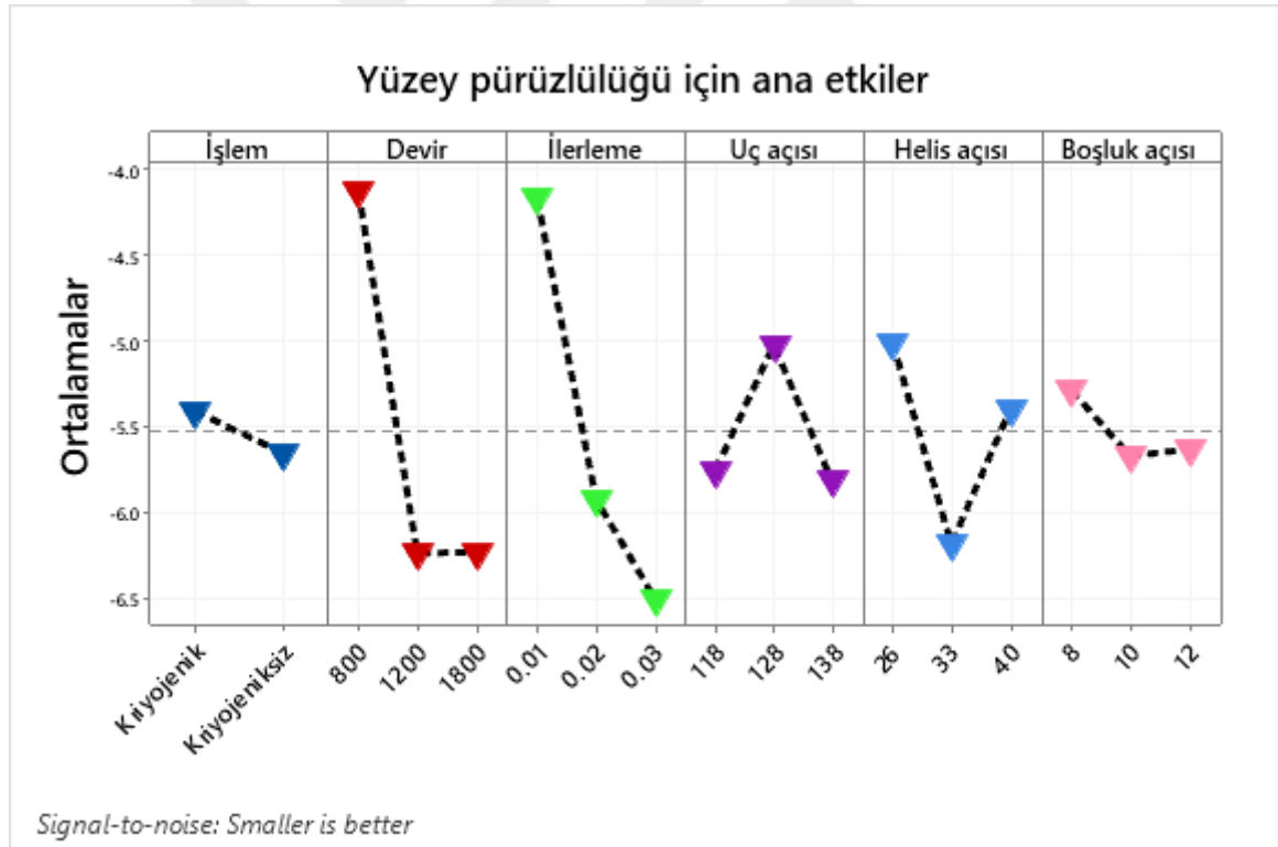
Şekil 4.34. Faktörlerin Yüzey pürüzlülüğü (Ra) üzerindeki ana etkileri
