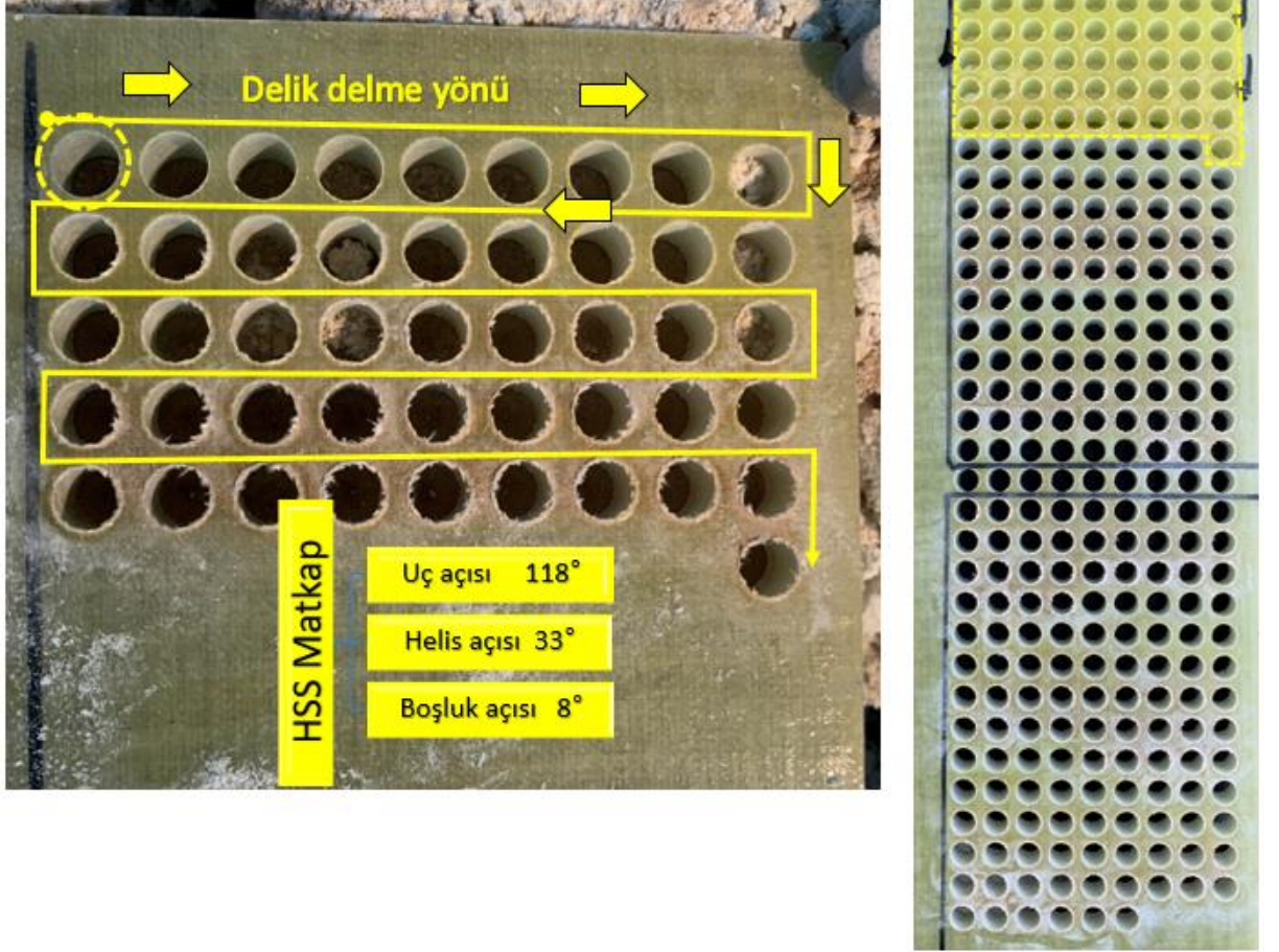
Şekil 4.127. HSS matkap ile delinen kompozit iş parçası
