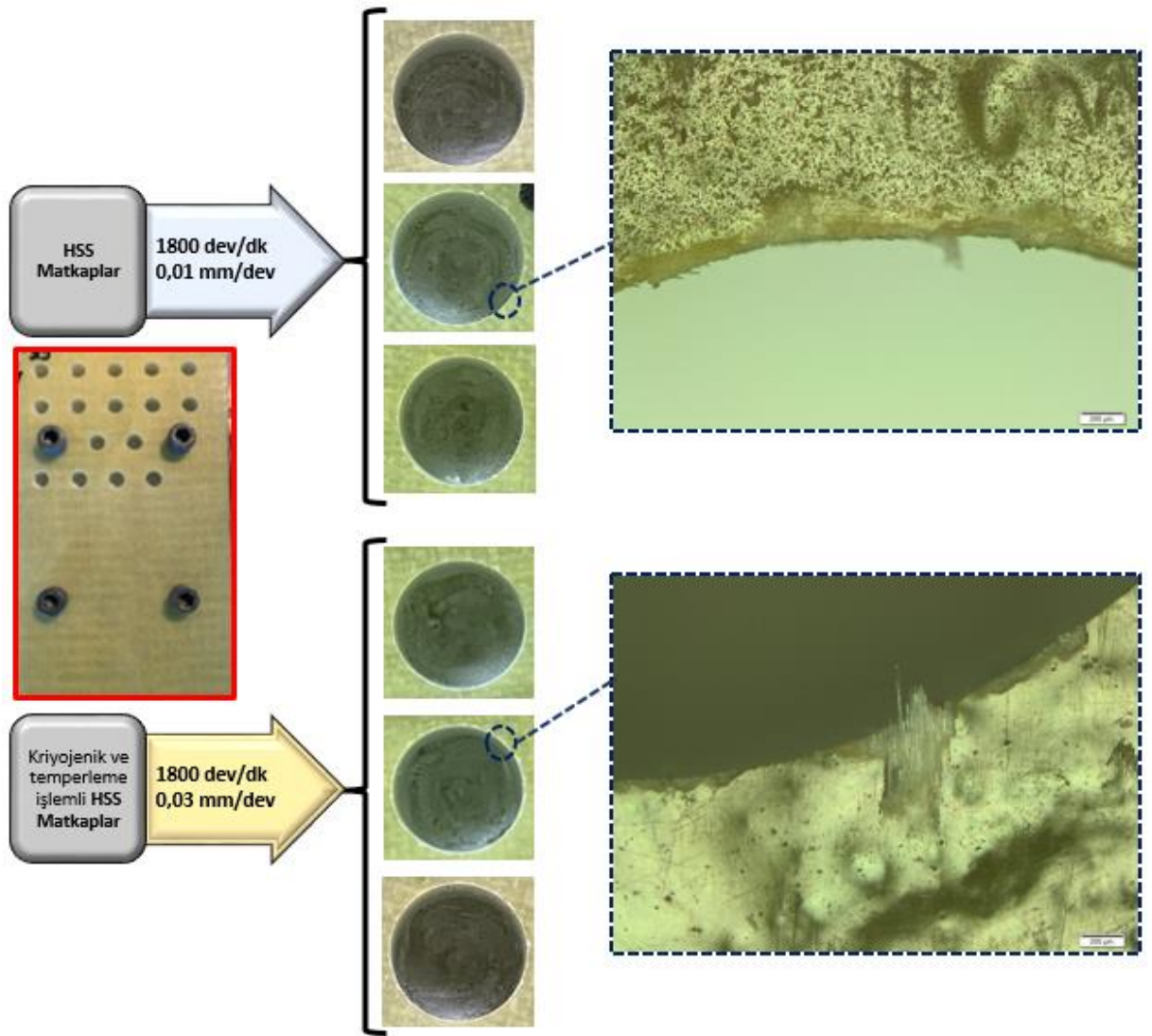
Şekil 4.97. Farklı matkaplar ile açılan deliklerin kenarlarının makro ve mikro resimleri
