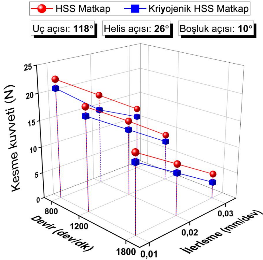
Şekil 4.7. 118° uç açısı, 26° helis açısı ve 10° boşluk açısına sahip matkaplarda kesme kuvveti
