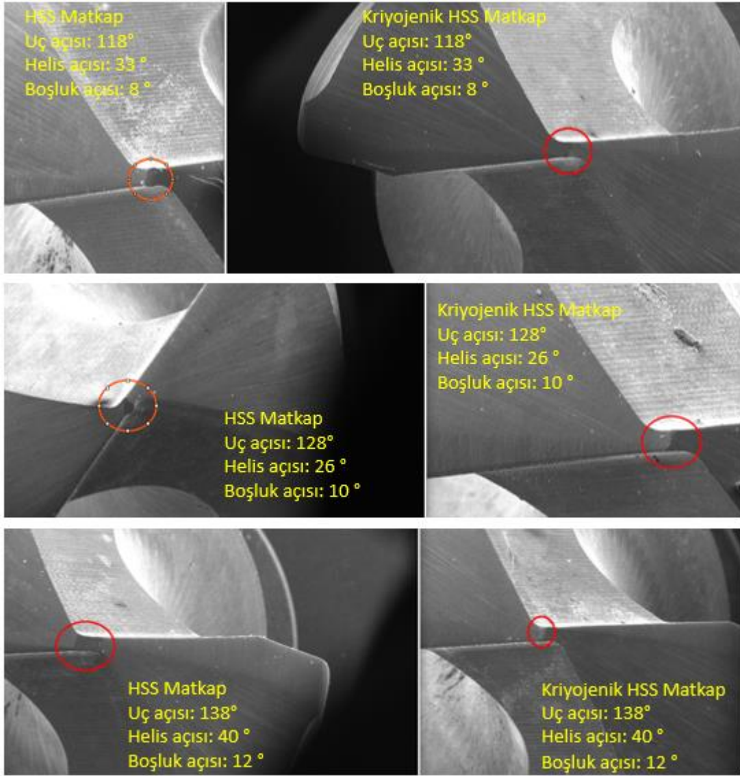
Şekil 4.121. Kesici takımlardaki radyal ağız aşınmalarının (daire içinde) SEM görüntüleri
