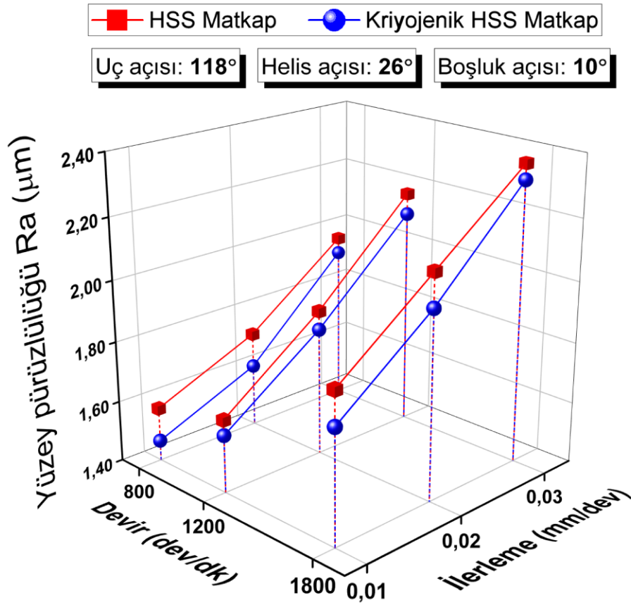
Şekil 4.38. 118° uç açısı, 26° helis açısı ve 10° boşluk açılı matkaplar ile işlemede yüzey pürüzlülüğü
