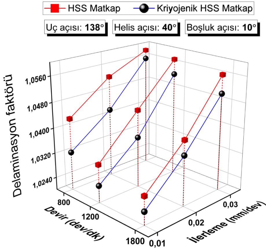
Şekil 4.94. 138° uç açısı, 40° helis açısı ve 10° boşluk açılı matkaplar ile işlemede delaminasyon faktörü
