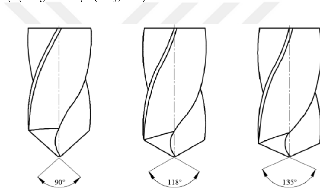
Şekil 1.26. Kesici takım matkabın uç açısı (Okay, 2020)
