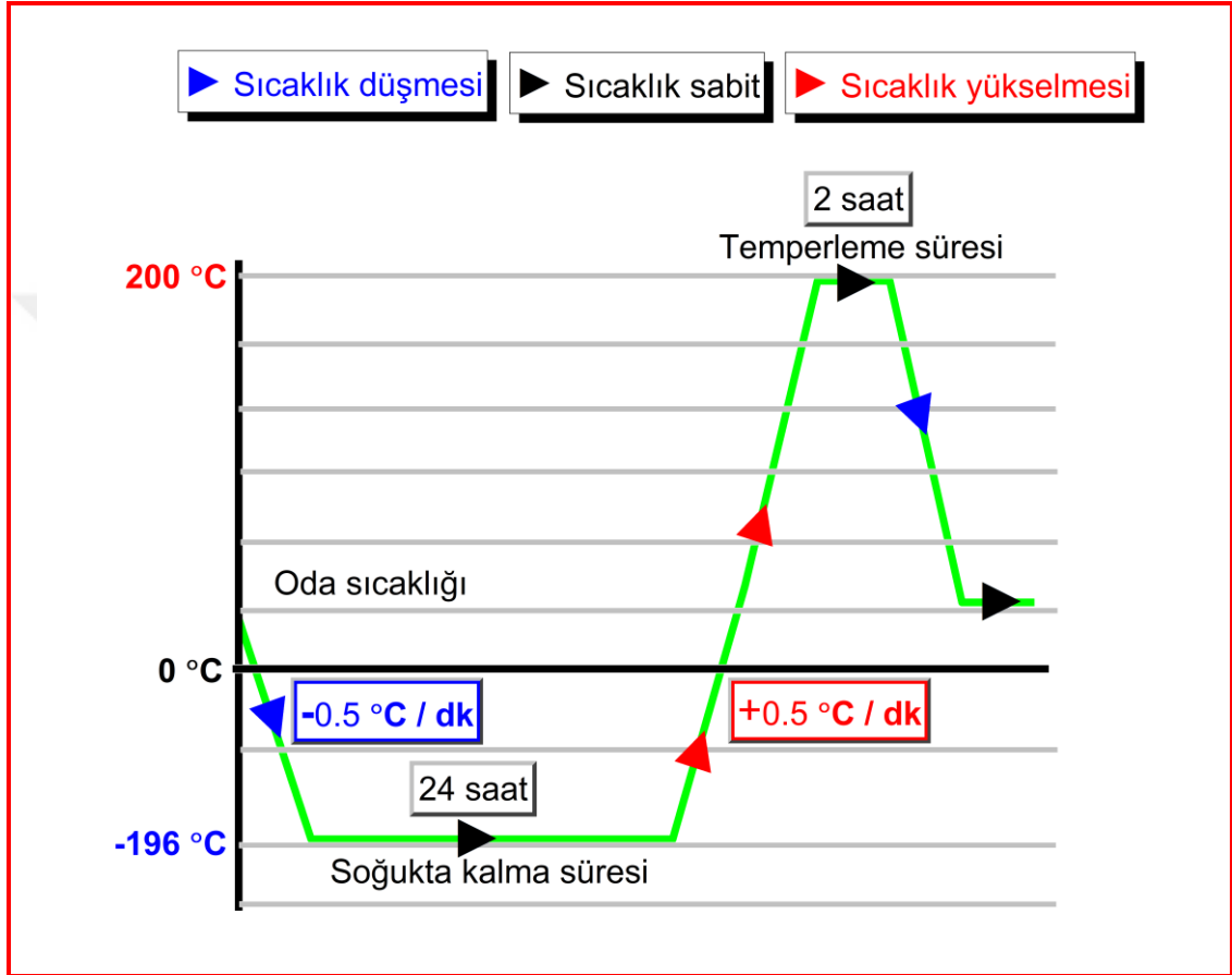
Şekil 3.8. Kriyojenik işlem süreçleri
