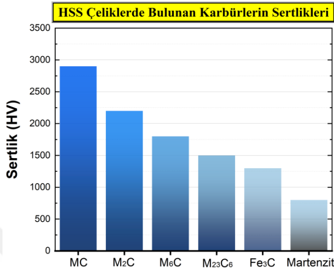
Şekil 4.3. HSS çeliklerde bulunan karbürlerin sertlikleri (Wells ve Lherbier, 1980)
