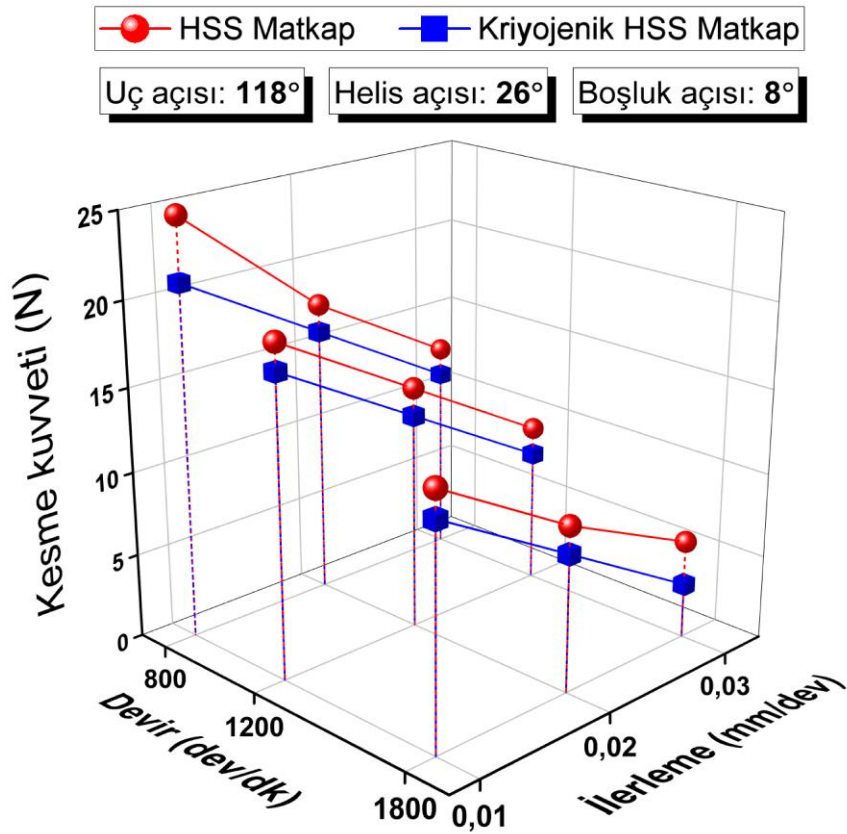
Şekil 4.6. 118° uç açısı, 26° helis açısı ve 8° boşluk açısına sahip matkaplarda kesme kuvveti
