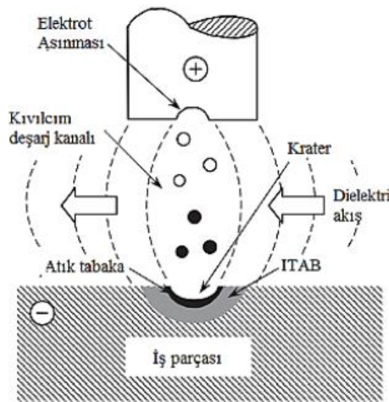
Şekil 1.16. Elektro-erozyon yöntemi ile delme işlemi şeması (Sheikh-Ahmad, 2009)
