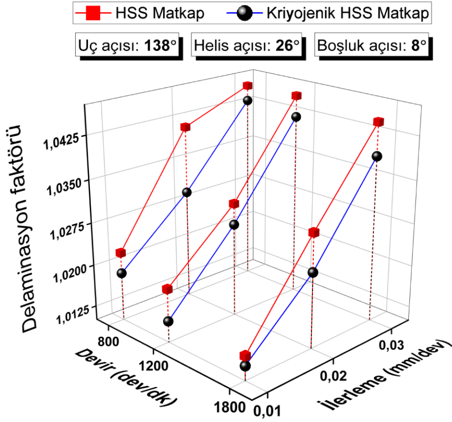
Şekil 4.87. 138° uç açısı, 26° helis açısı ve 8° boşluk açılı matkaplar ile işlemede delaminasyon faktörü
