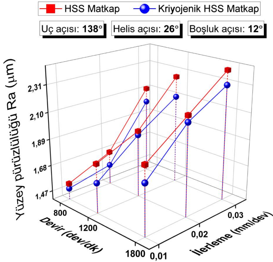
Şekil 4.57. 138^\circ uç açısı, 26^\circ helis açısı ve 12^\circ boşluk açılı matkaplar ile işlemede yüzey pürüzlülüğü
