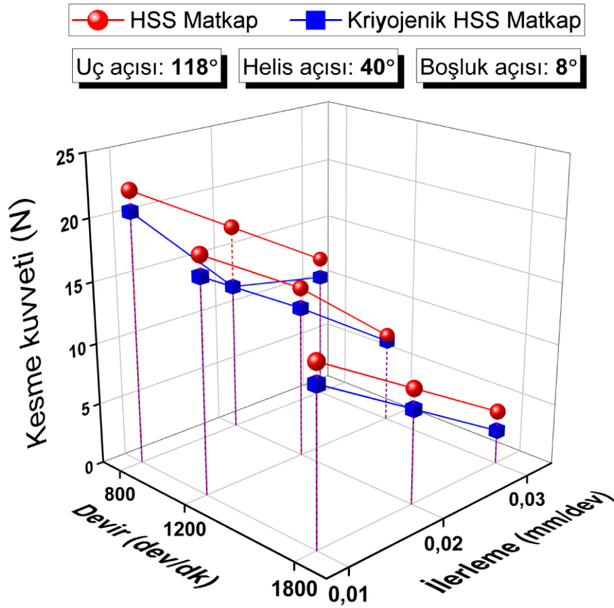
Şekil 4.12. 118° uç açısı, 40° helis açısı ve 8° boşluk açısına sahip matkaplarda kesme kuvveti
