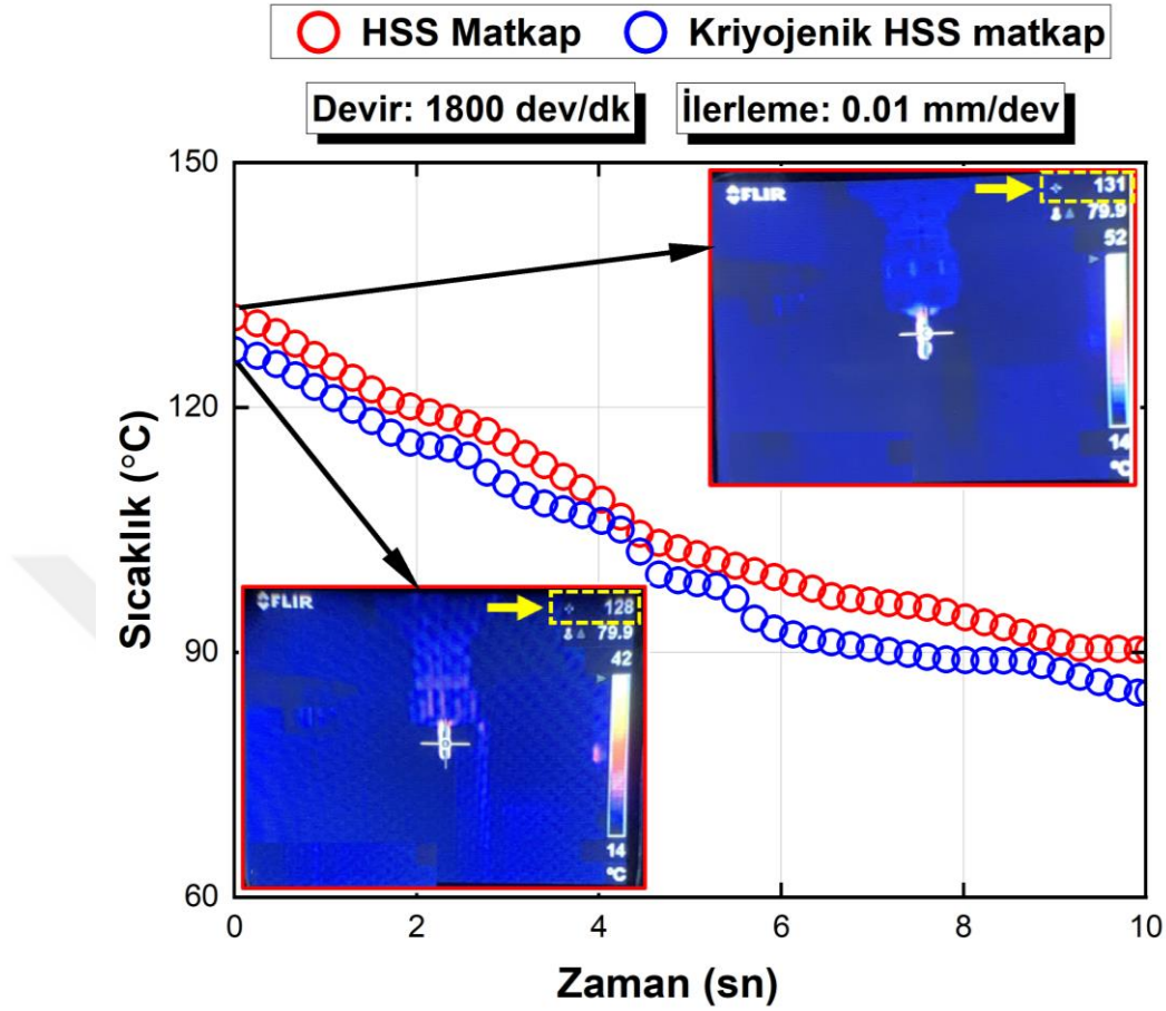
Şekil 4. 126. Ardı ardına delik işlemleri bitimi matkapların uç kısımlarının sıcaklıkları
