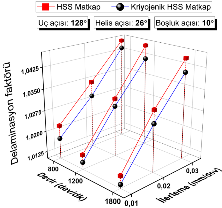
Şekil 4.79. 128° uç açısı, 26° helis açısı ve 10° boşluk açılı matkaplar ile işlemede delaminasyon faktörü
