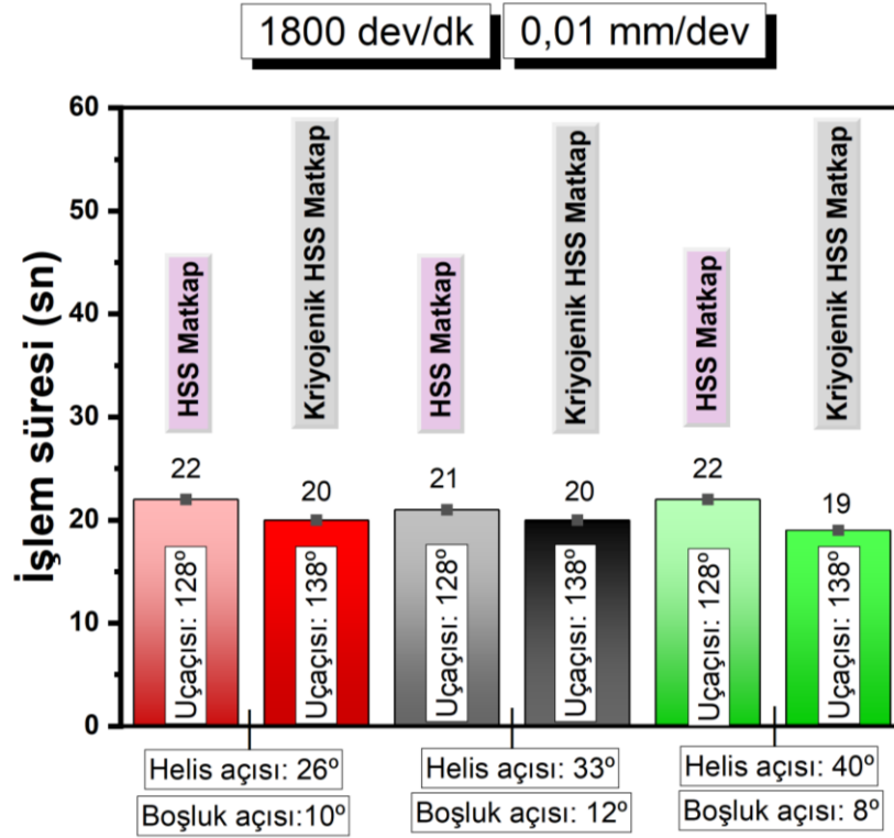
Şekil 4.115. HSS ve kriyojenik HSS matkapların aynı devir ve ilerlemedeki işleme süreleri
