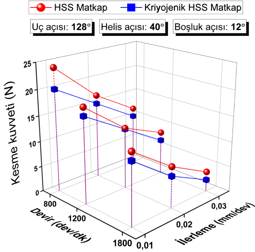
Şekil 4.23. 128° uç açısı, 40° helis açısı ve 12° boşluk açısına sahip matkaplarda kesme kuvveti
