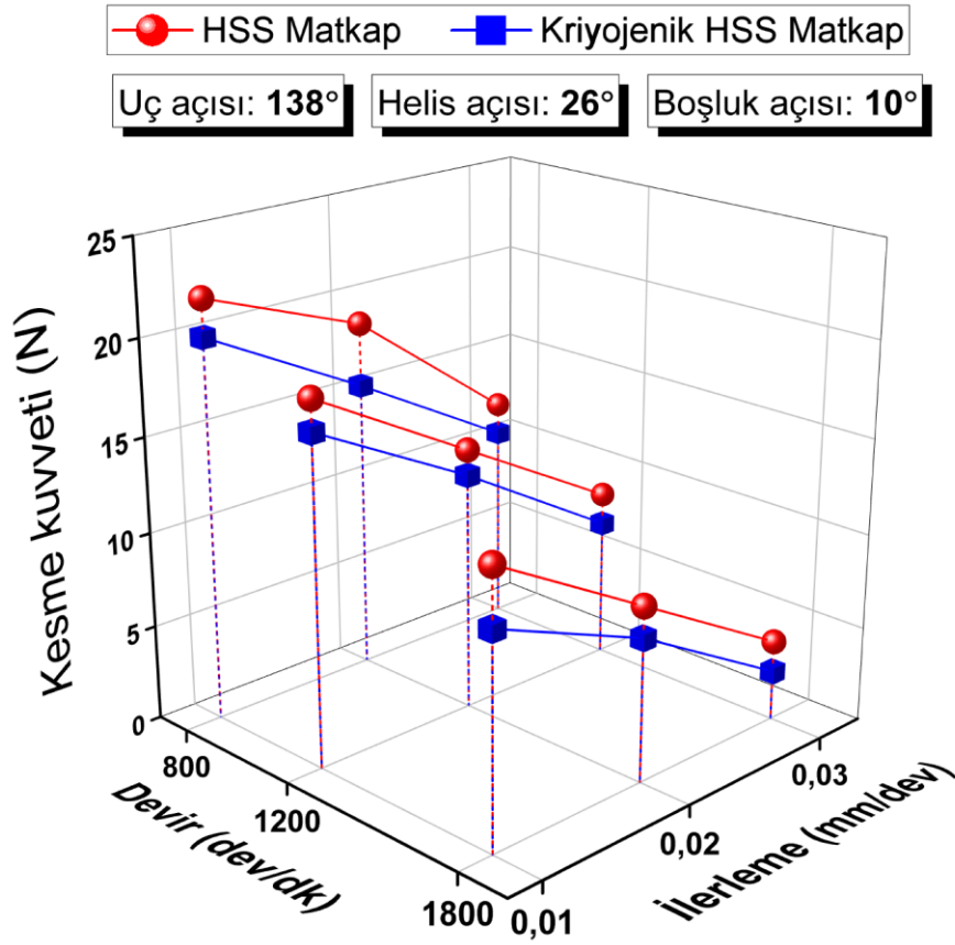
Şekil 4.25. 138° uç açısı, 26° helis açısı ve 10° boşluk açısına sahip matkaplarda kesme kuvveti
