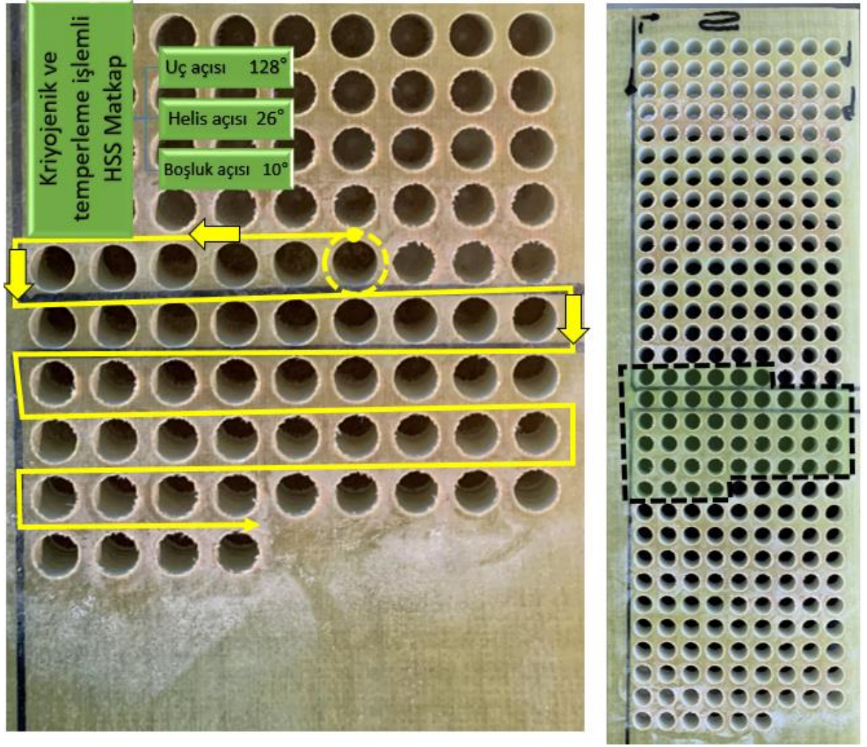
Şekil 4.130. Kriyojenik ve temperleme işlemi görmüş HSS matkap ile delinen kompozit iş parçası
