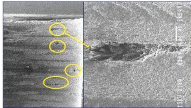
Şekil 1.18. Kompozit malzemelerde elyaf kopması (Davim, 2013)
