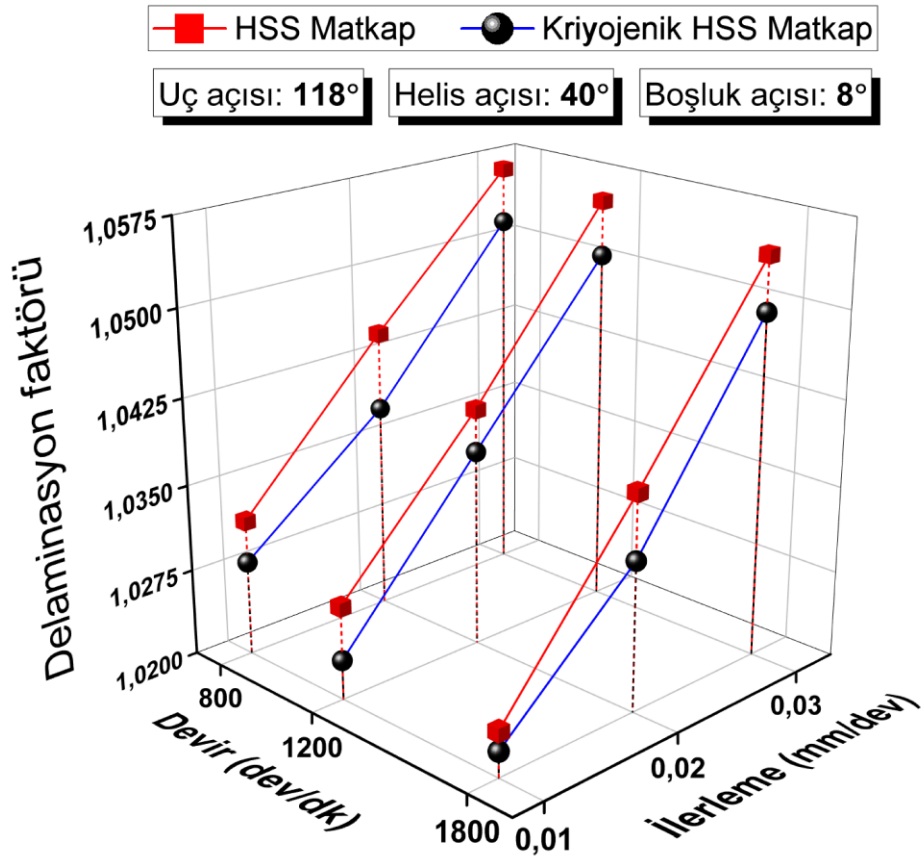
Şekil 4.75. 118° uç açısı, 40° helis açısı ve 8° boşluk açılı matkaplar ile işlemede delaminasyon faktörü
