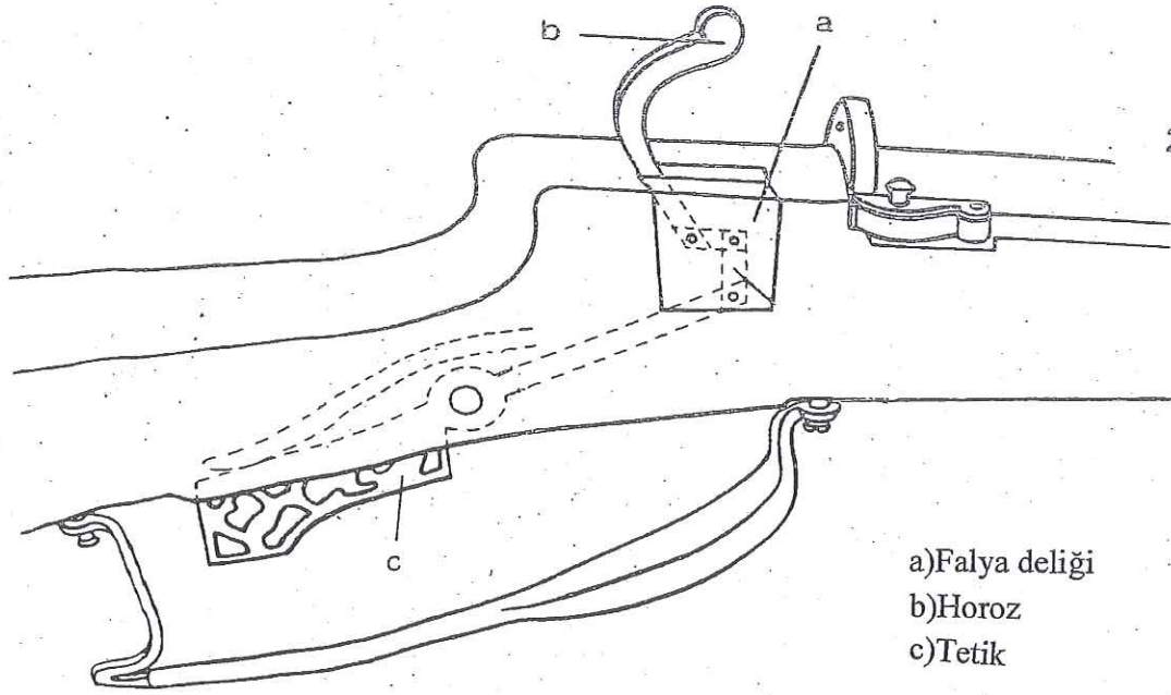
1: Osmanlı fitilli mekanizması
