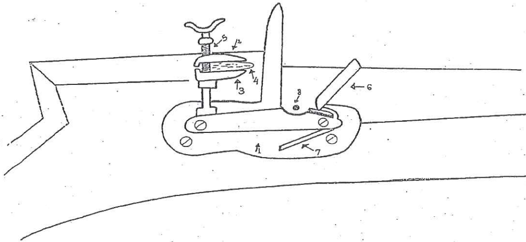
2: Osmanlı Çakmaklı Mekanizması (1. tesbit levhası, 2. horoz, 3. taş tutma dili, 4. çakmak taşı, 5. sıkıştırma vidası, 6. çakmak demiri, 7. kumma yayı, 8. falya deliği.)
