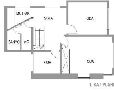
Şekil 3.31 1. Kat Planı
