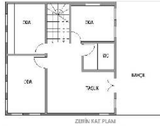
Şekil 3.16 Zemin Kat Planı
