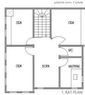
Şekil 3.29 1. Kat Planı
