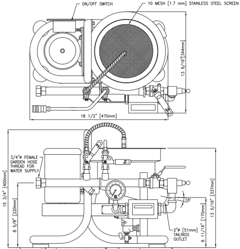
Şekil 2.5 Knelson Gravite Konsantratör görseli ve şematik görünümü (laboratuvar tip).
