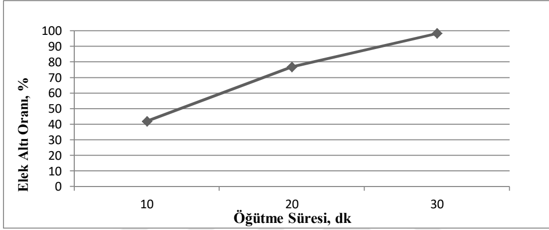
Şekil 3.7 Bilyalı değirmende öğütme sürelerine göre elek altı oranı grafiği.
