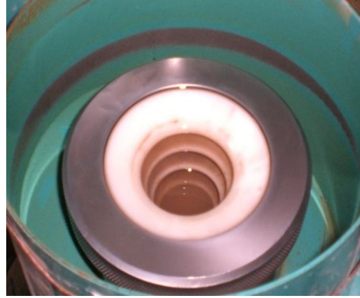
Şekil 2.7 Deneylerde kullanılan laboratuvar tip Knelson Gravite Seperator (MD3 Model).
