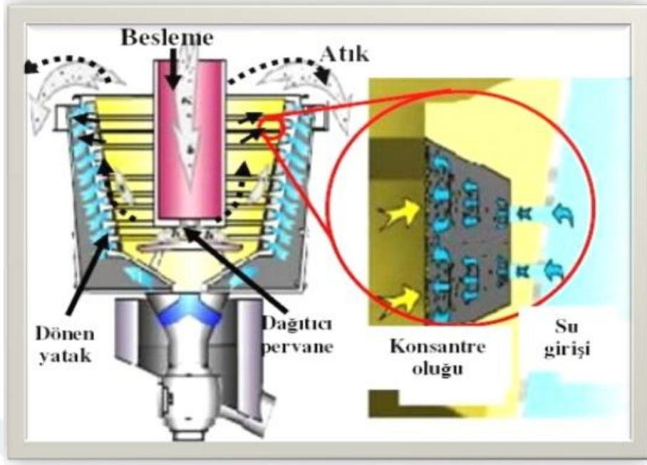
Şekil 2.6 Knelson Gravite Seperator düşey kesiti (Ling 1998).
