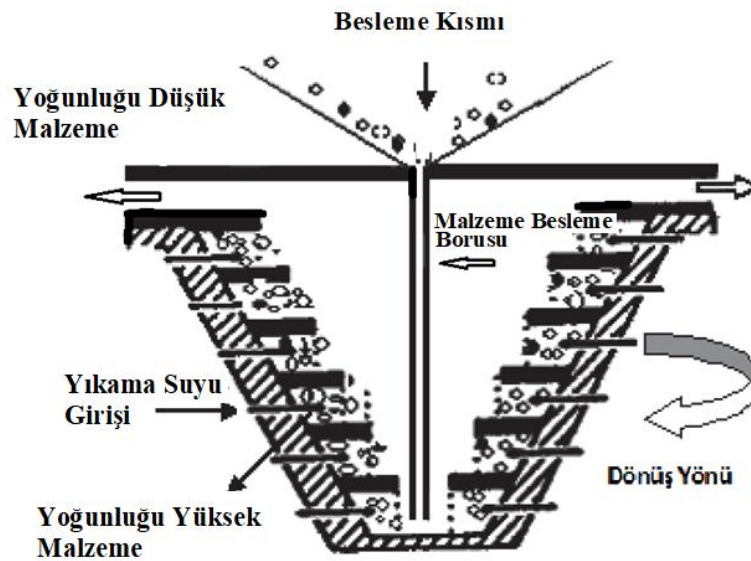
Şekil 3.8 Knelson Gravite Konsantratör çanağında malzeme yerleşmesinin şematik görünümü.
