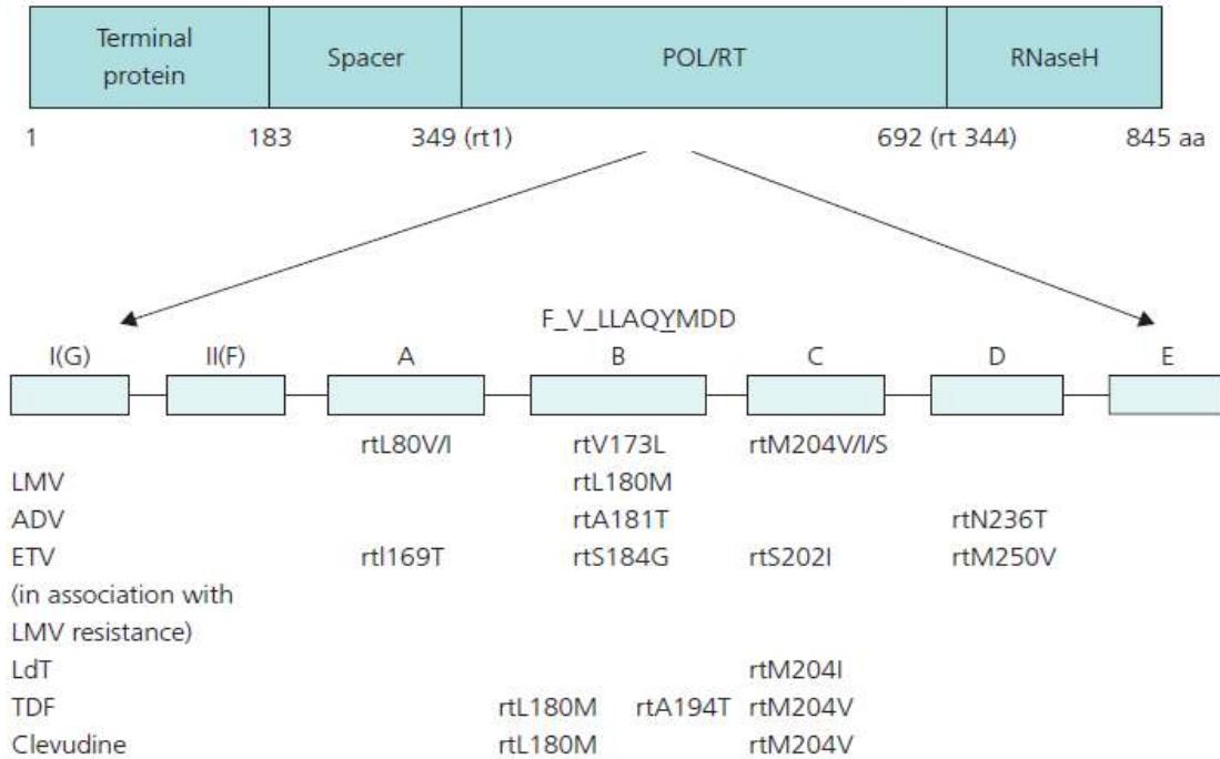
Şekil 8- HBV polimeraz majör gen mutasyon bölgeleri, Textbook of Gastroenterology, Yamada, Fifth Edition.
