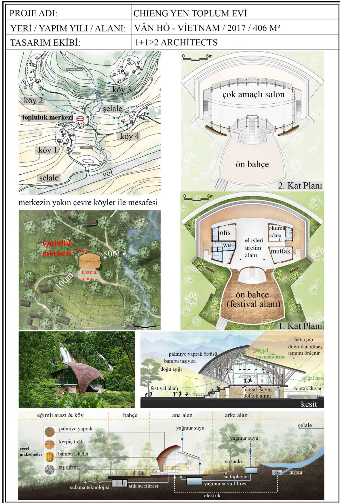
Şekil 2.43. Chieng Yen Toplum Evi, Vân Hồ, Vietnam (Anonim 2019d'den aktarılarak)
