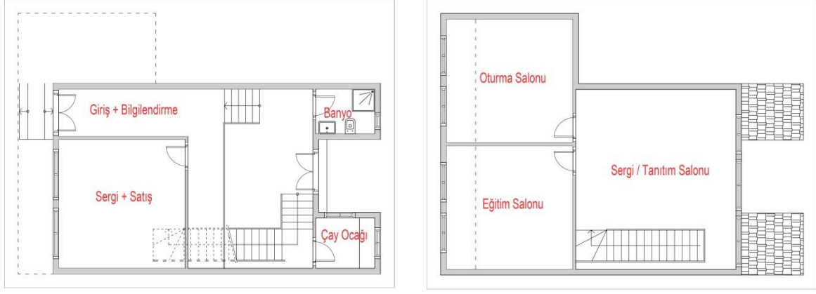
Şekil 3.55. Misi Köyü İpekevi zemin kat ve birinci kat plan şemaları
