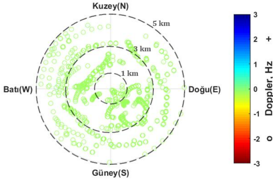
Şekil 6.24 Pruhanice, 17 Nisan 2011, saat 17:22 GS, önerilen teknik ile elde edilen Doppler haritasında yansıma noktalarının merkez noktası olan vericiye göre uzaklıkları (km).
