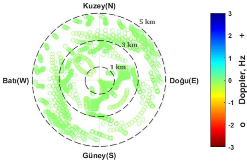
Şekil 6.20 Pruhanice, 17 Nisan 2011, saat 13:04 GS, önerilen teknik ile elde edilen Doppler haritasında yansıma noktalarının merkez noktası olan vericiye göre uzaklıkları (km).
