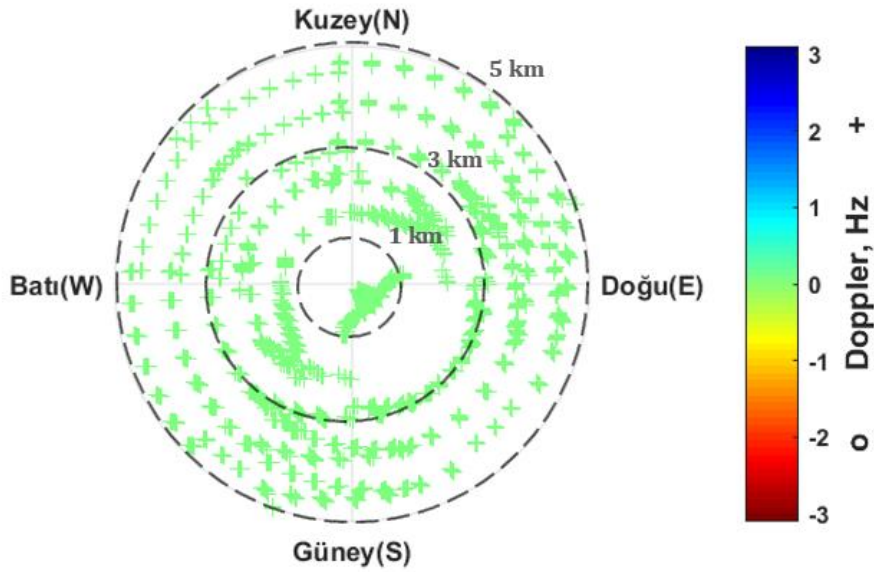
Şekil 6.12 Pruhanice, 17 Nisan 2011, saat 09:07 GS, önerilen teknik ile elde edilen Doppler haritasında yansıma noktalarının merkez noktası olan vericiye göre uzaklıkları (km).
