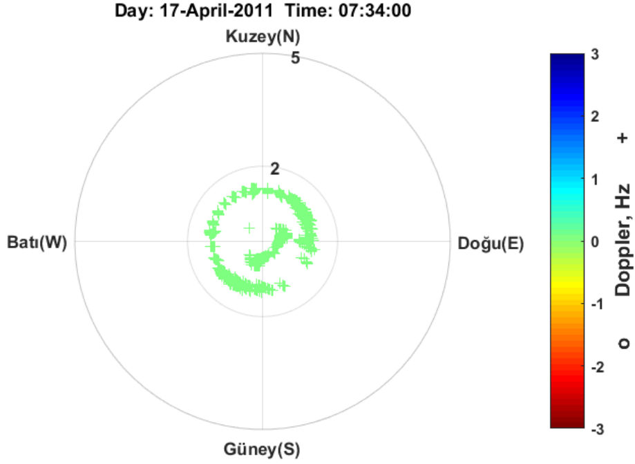
Şekil EK-1. 21 Pruhonice, 17 Nisan 2011, 07:34 GS, önerilen teknik ile elde edilen Doppler haritası
