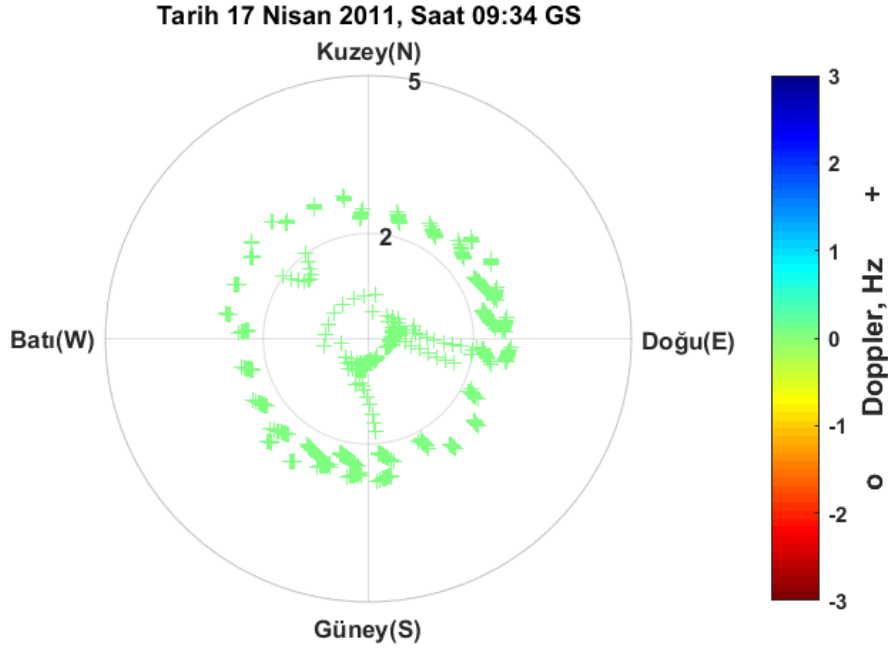
Şekil EK-1. 37 Pruhonice, 17 Nisan 2011, 09:34 GS, önerilen teknik ile elde edilen Doppler haritası
