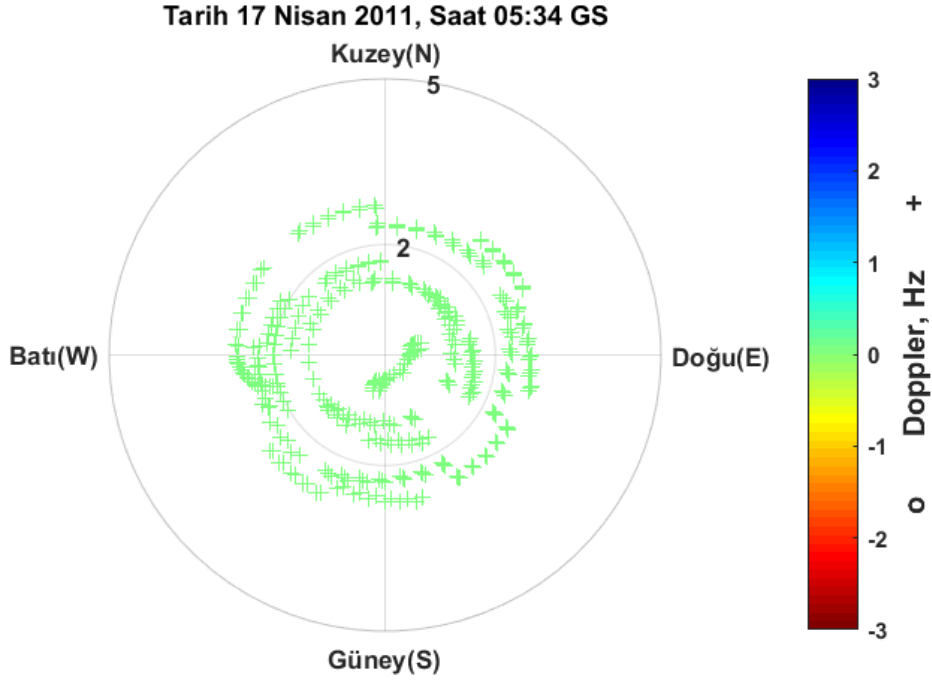
Şekil EK-1. 3 Pruhonice, 17 Nisan 2011, 05:34 GS, önerilen teknik ile elde edilen Doppler haritası
