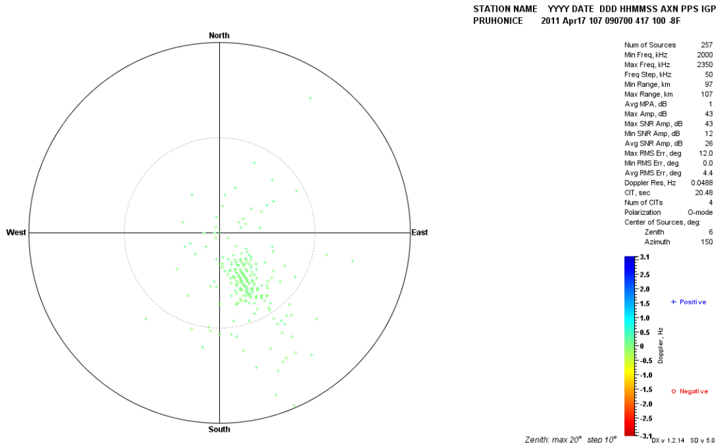
Şekil EK-1. 34 Pruhonice, 17 Nisan 2011, saat 09:07 GS, Drift Explorer yazılım aracı ile elde edilen Doppler haritası
