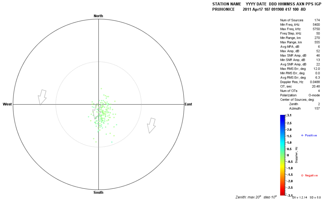
Şekil EK-1. 36 Pruhonice, 17 Nisan 2011, saat 09:19 GS, Drift Explorerer yazılım aracı ile elde edilen Doppler haritası
