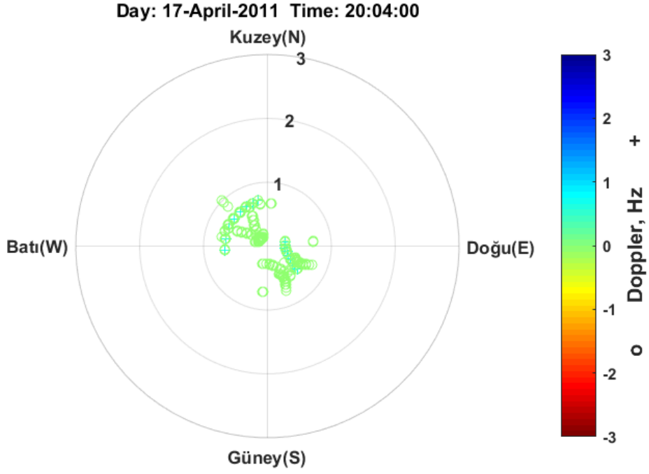
Şekil EK-1. 85 Pruhonice, 17 Nisan 2011, 20:04 GS, önerilen teknik ile elde edilen Doppler haritası
