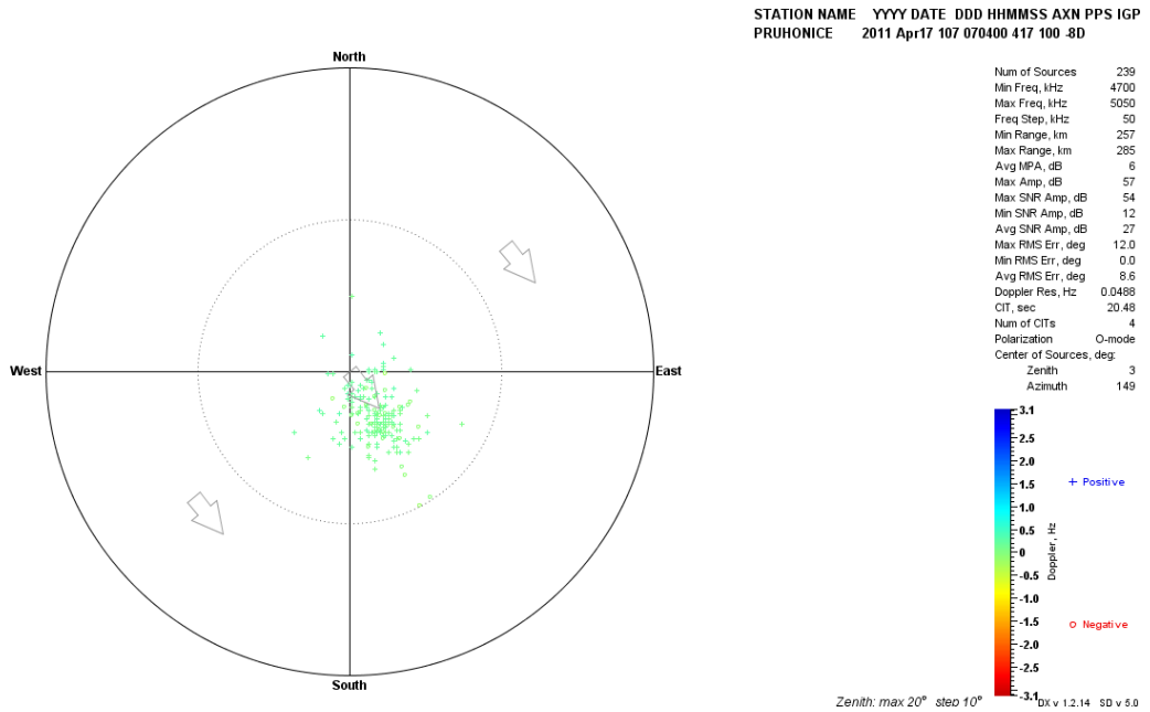
Şekil EK-1. 16 Pruhonice, 17 Nisan 2011, saat 07:04 GS, Drift Explorer yazılım aracı ile elde edilen Doppler haritası
