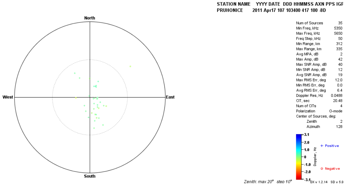
Şekil EK-1. 44 Pruhonice, 17 Nisan 2011, saat 10:34 GS, Drift Explorer yazılım aracı ile elde edilen Doppler haritası
