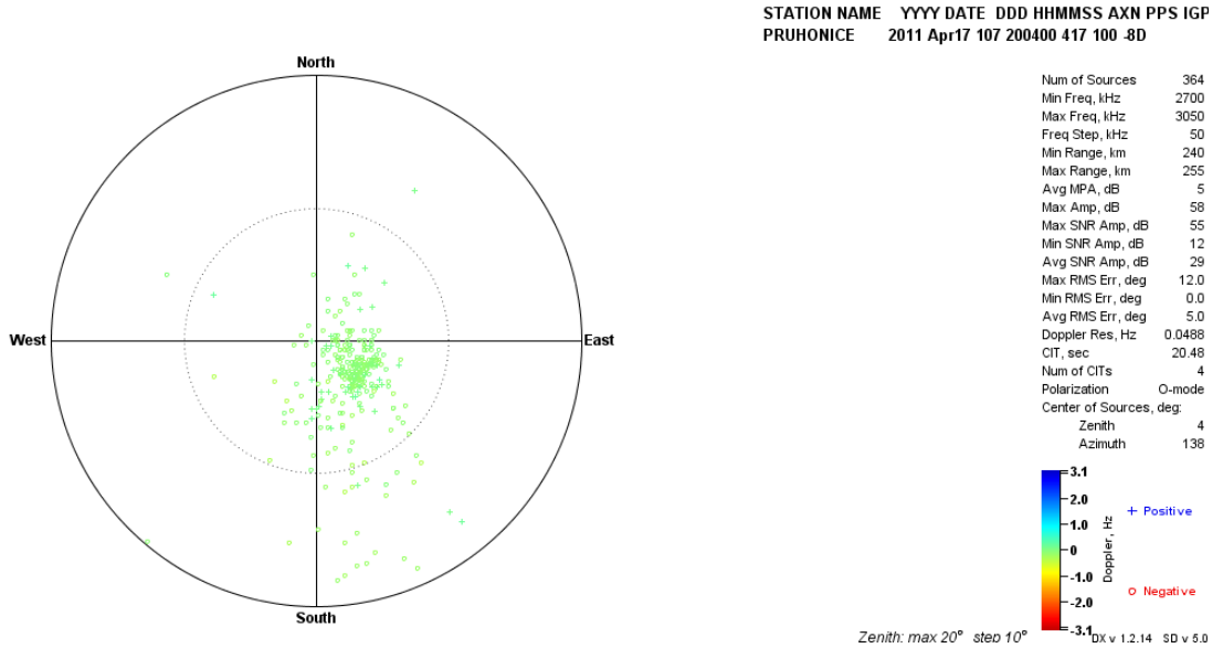
Şekil EK-1. 86 Pruhonice, 17 Nisan 2011, saat 20:04 GS, Drift Explorer yazılım aracı ile elde edilen Doppler haritası
