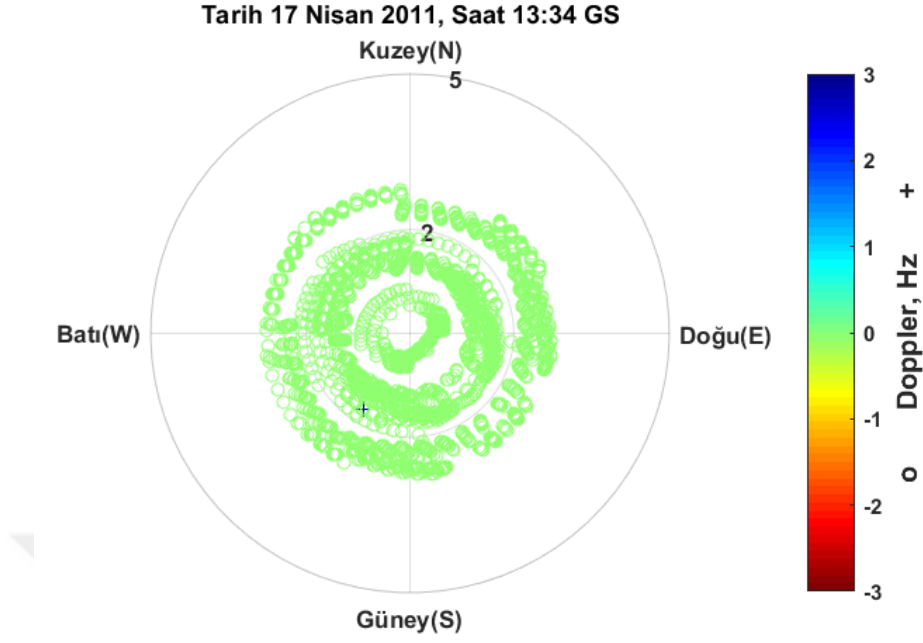
Şekil EK-1. 67 Pruhonice, 17 Nisan 2011, 13:34 GS, önerilen teknik ile elde edilen Doppler haritası
