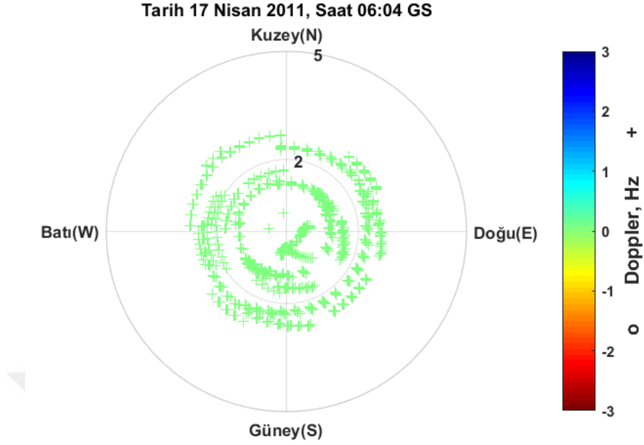
Şekil EK-1. 7 Pruhonice, 17 Nisan 2011, 06:04 GS, önerilen teknik ile elde edilen Doppler haritası
