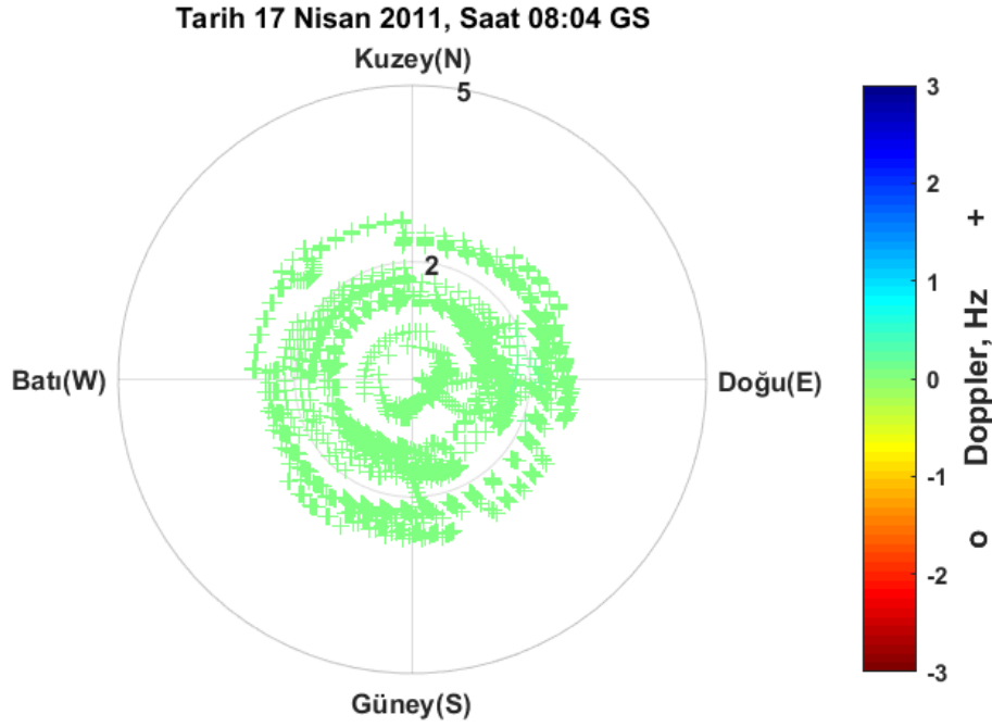
Şekil EK-1. 23 Pruhonice, 17 Nisan 2011, 08:04 GS, önerilen teknik ile elde edilen Doppler haritası
