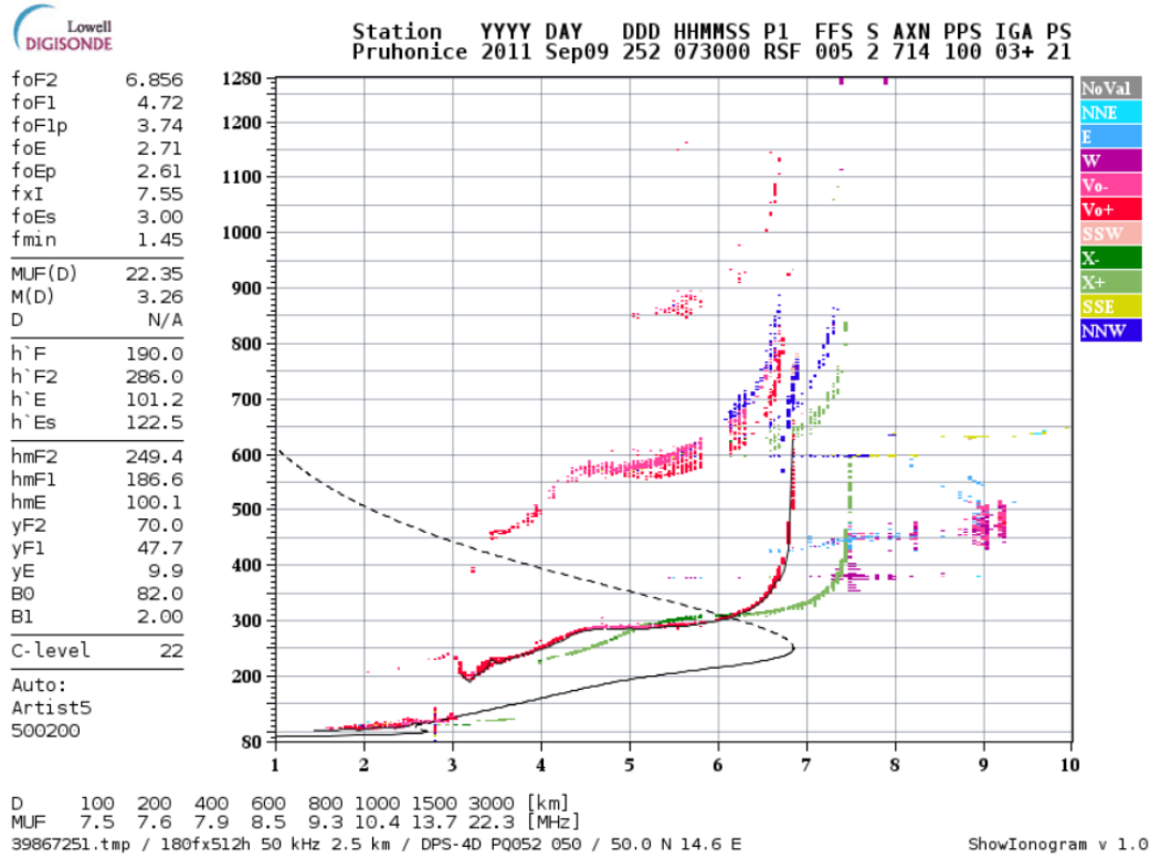
Şekil 3.4 Pruhonice İstasyonu, tarih 09 Eylül 2011, saat 07:30 GS için elde edilen Dijisonda ionogram grafiği.
