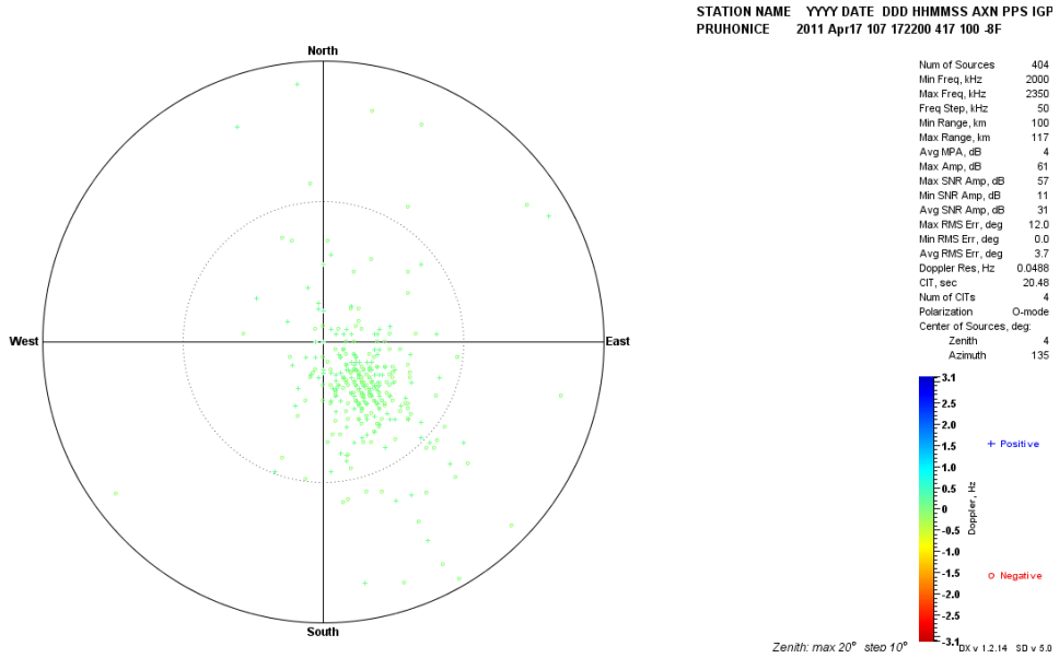
Şekil 6.23 Pruhonice, 17 Nisan 2011, saat 17:22 GS, Drift Explorer yazılım aracı ile elde edilen Doppler haritası
