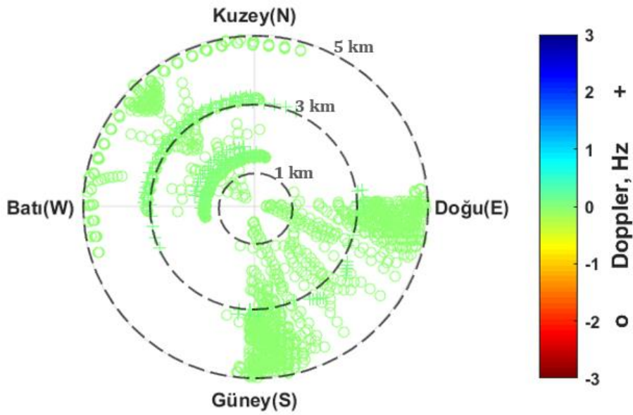
Şekil 6.16 Pruhanice, 17 Nisan 2011, saat 11:37 GS, önerilen teknik ile elde edilen Doppler haritasında yansıma noktalarının merkez noktası olan vericiye göre uzaklıkları (km).
