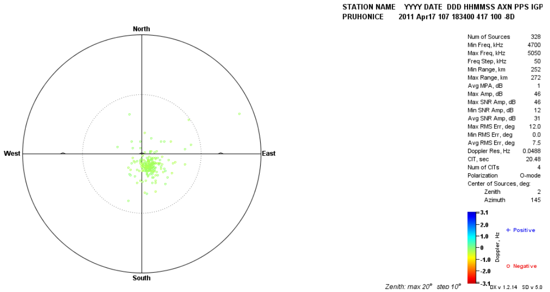
Şekil EK-1. 78 Pruhonice, 17 Nisan 2011, saat 18:34 GS, Drift Explorer yazılım aracı ile elde edilen Doppler haritası
