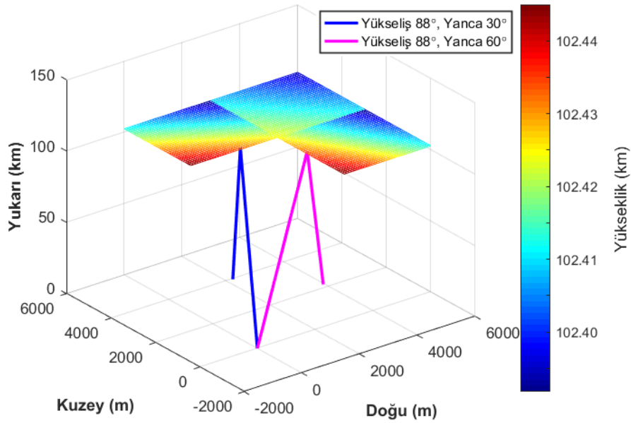
Şekil 6.4 Basitleştirilmiş ışın izleme tekniği ile düzlemsel dalgaların 15 dakika sonraki yayılımları, Pruhonice, 17 Nisan 2011, saat 11:19 GS, 3.20 MHz taşıyıcı frekansa sahip düzlemsel dalgaların 3.20 MHz plazma frekansına sahip iyonküre tabakalarından yansımaları.
