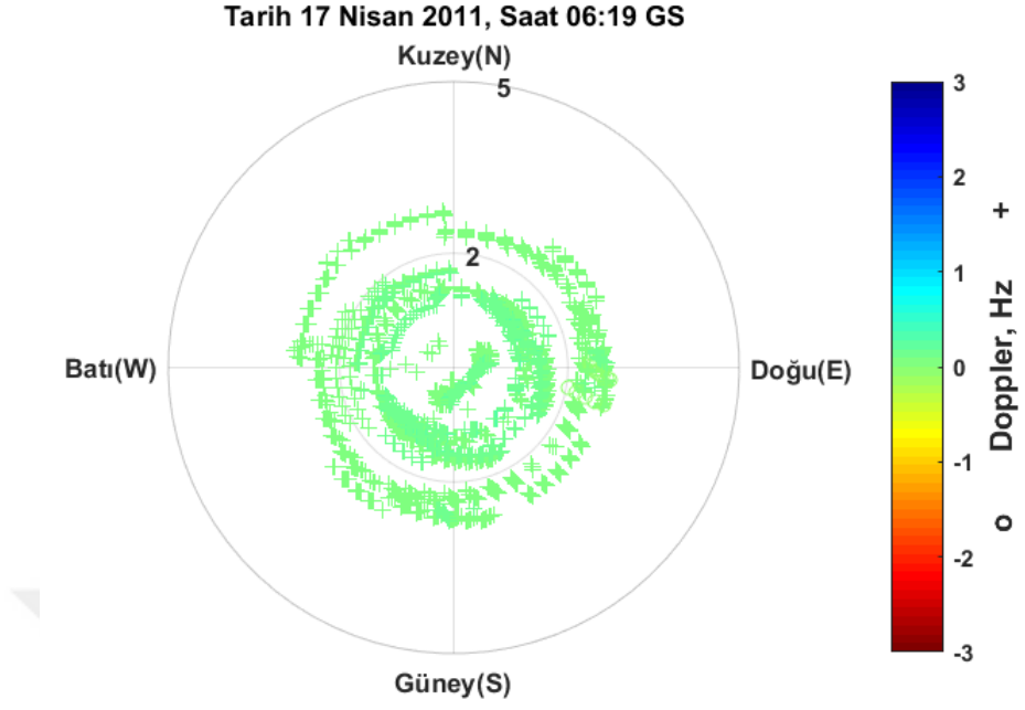
Şekil EK-1. 9 Pruhonice, 17 Nisan 2011, 06:19 GS, önerilen teknik ile elde edilen Doppler haritası
