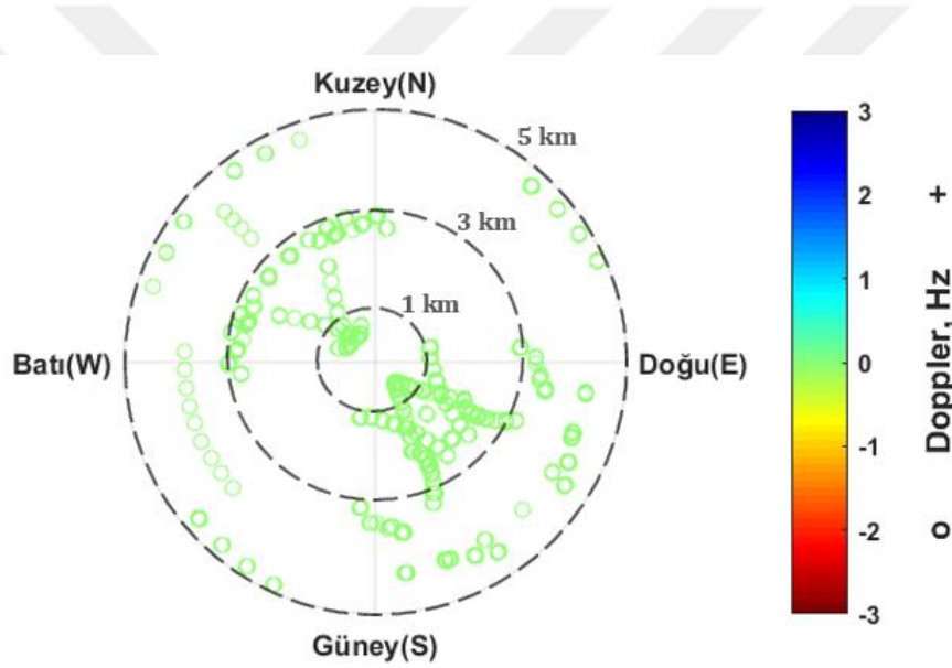
Şekil 6.28 Pruhanice, 17 Nisan 2011, saat 20:34 GS, önerilen teknik ile elde edilen Doppler haritasında yansıma noktalarının merkez noktası olan vericiye göre uzaklıkları (km).
