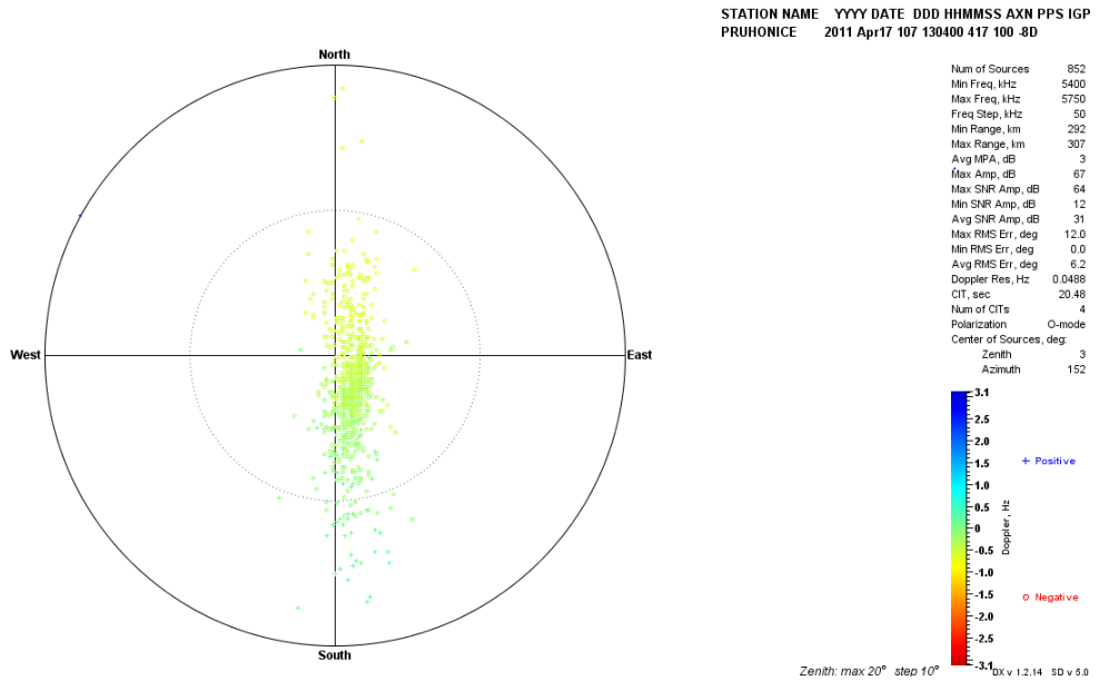
Şekil EK-1. 64 Pruhonice, 17 Nisan 2011, saat 13:04 GS, Drift Explorer yazılım aracı ile elde edilen Doppler haritası
