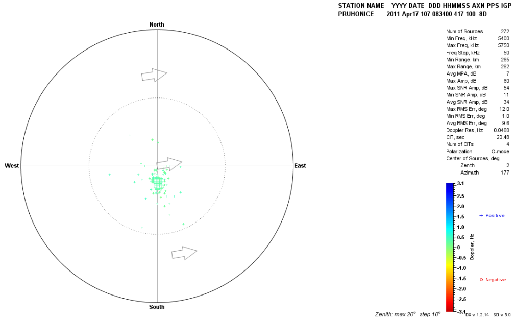
Şekil EK-1. 28 Pruhonice, 17 Nisan 2011, saat 08:34 GS, Drift Explorer yazılım aracı ile elde edilen Doppler haritası
