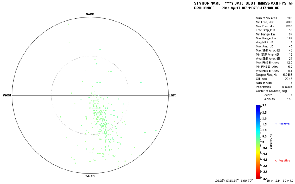
Şekil 6.15 Pruhonice, 17 Nisan 2011, saat 11:37 GS, Drift Explorerer yazılım aracı ile elde edilen Doppler haritası
