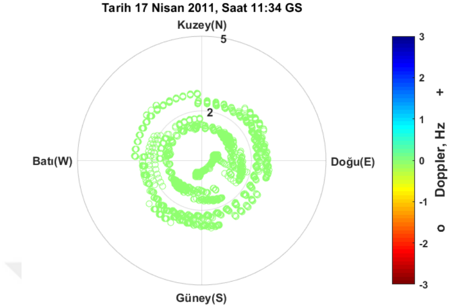
Şekil EK-1. 51 Pruhonice, 17 Nisan 2011, 11:34 GS, önerilen teknik ile elde edilen Doppler haritası
