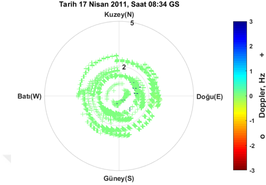
Şekil EK-1. 27 Pruhonice, 17 Nisan 2011, 08:34 GS, önerilen teknik ile elde edilen Doppler haritası
