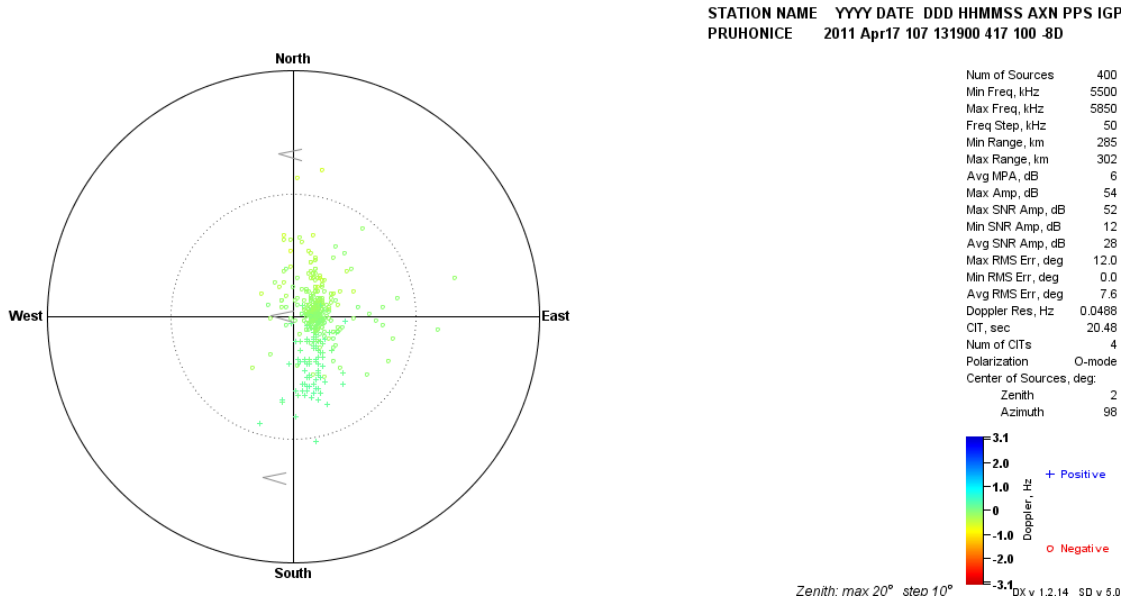
Şekil EK-1. 66 Pruhonice, 17 Nisan 2011, saat 13:19 GS, Drift Explorer yazılım aracı ile elde edilen Doppler haritası
