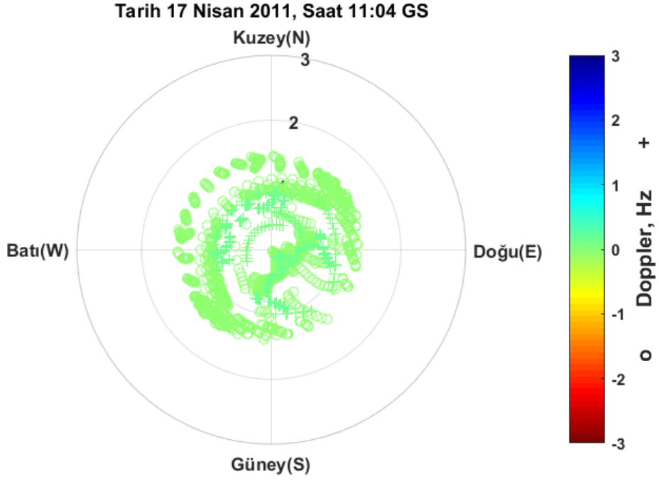
Şekil EK-1. 45 Pruhonice, 17 Nisan 2011, 11:04 GS, önerilen teknik ile elde edilen Doppler haritası
