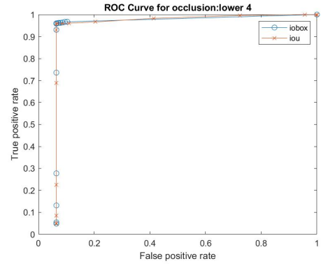
(d) ROC Curve for level 4 lower occlusion
