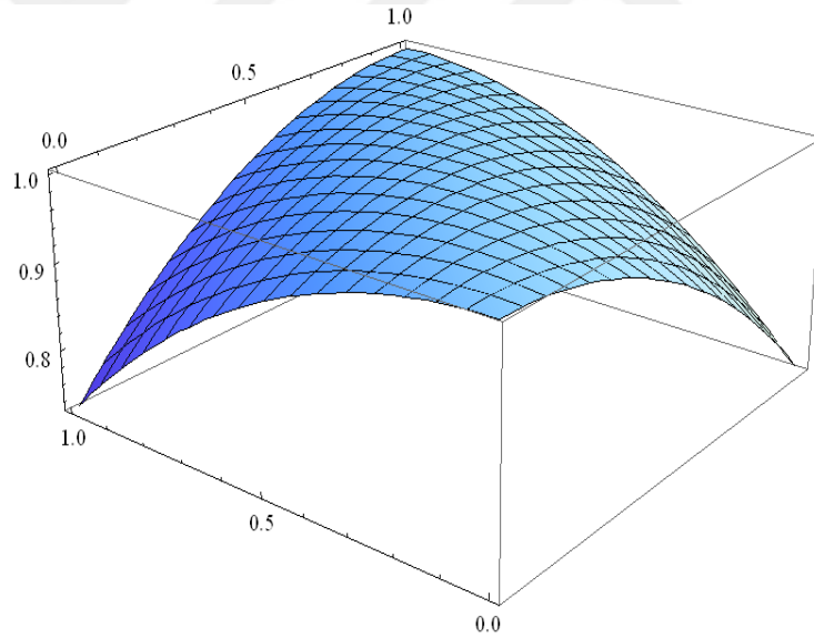
Şekil 1.6 u(x,t) = \cos^{\frac{1}{2}}(x-t) , 0 \leq x, t \leq 1 kompakton çözümün grafiği
