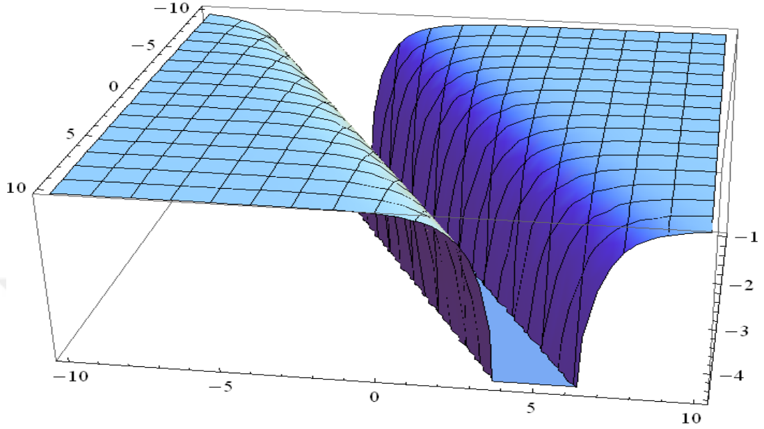
Şekil 3.3. u_3(x,t) ni grafiği
