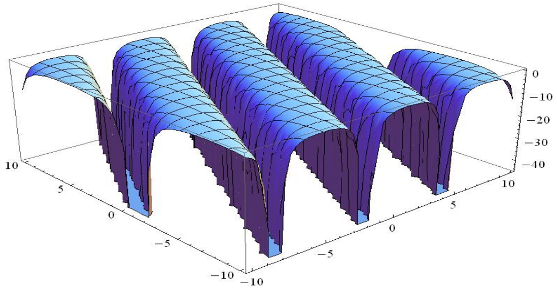
Şekil. 3.4 u_4(x,t) çözümünün grafiği
