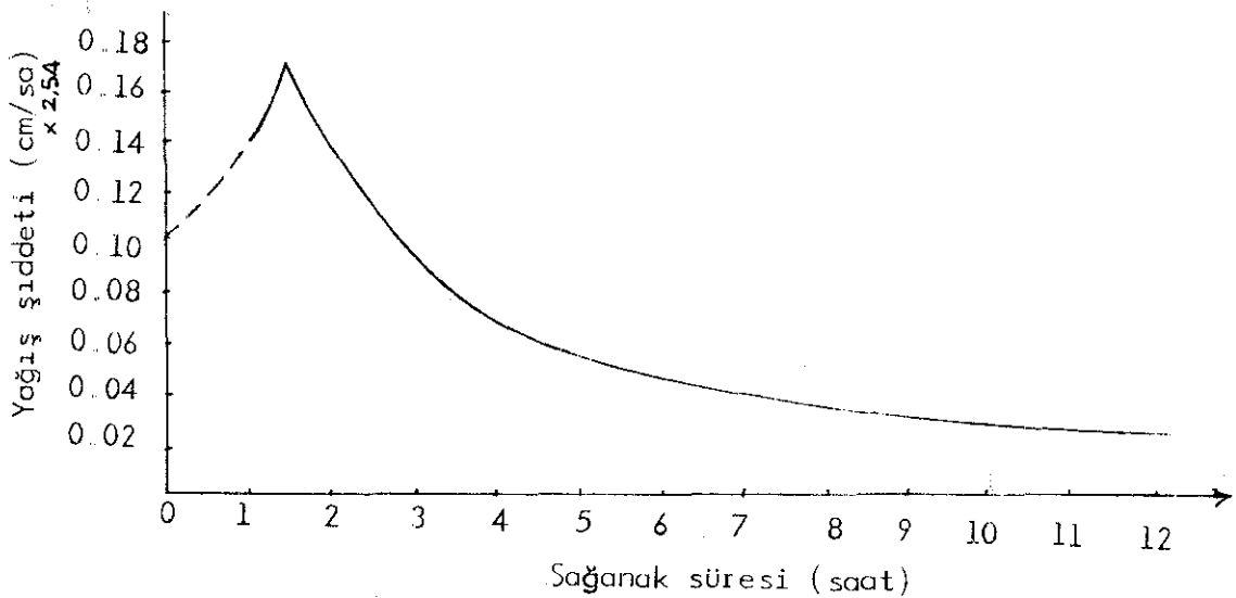
Şekil 3b. Amerika Meteorolojisi Bürosunun katsayılarının kullanıldığı yağış şiddeti-süre eğrisi
