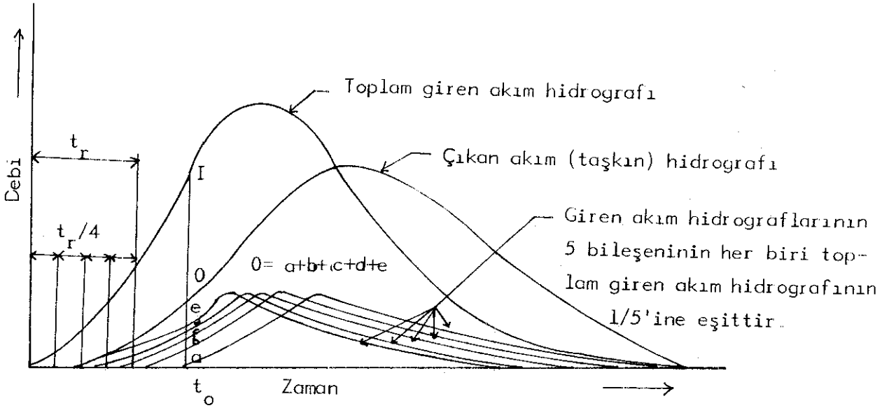
Şekil 18. Giren akım hidrograf bileşenlerinin grafik integrasyonu ile ana kanal boyunca ötelenmesi
