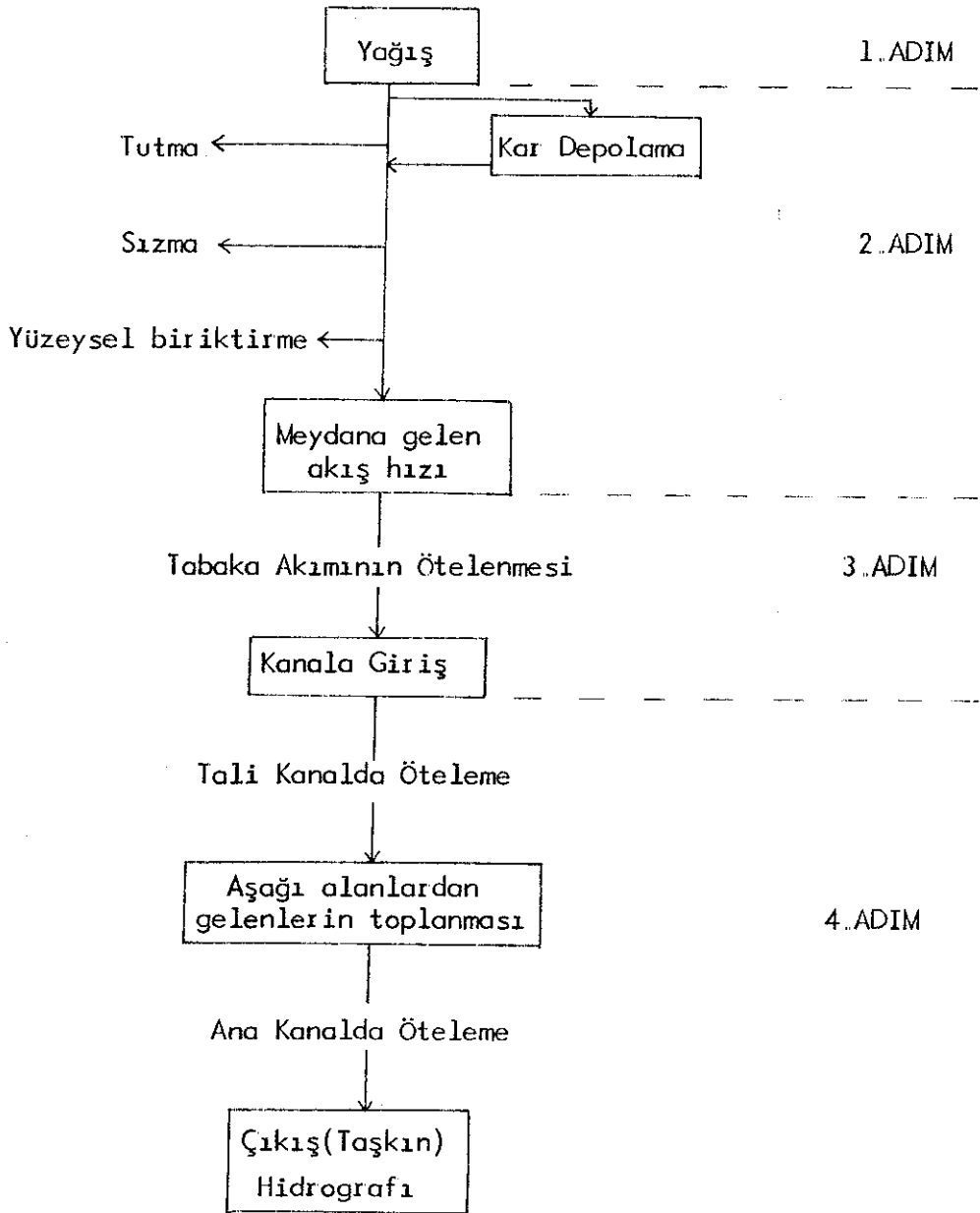
Şekil 1. Yüzey akış hidrografının analizinde küçük akarsu havzasının şematik görünümü
