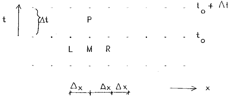
Şekil 14. Karakteristik düzlem üzerinde sonlu farklarla nokta ağı
