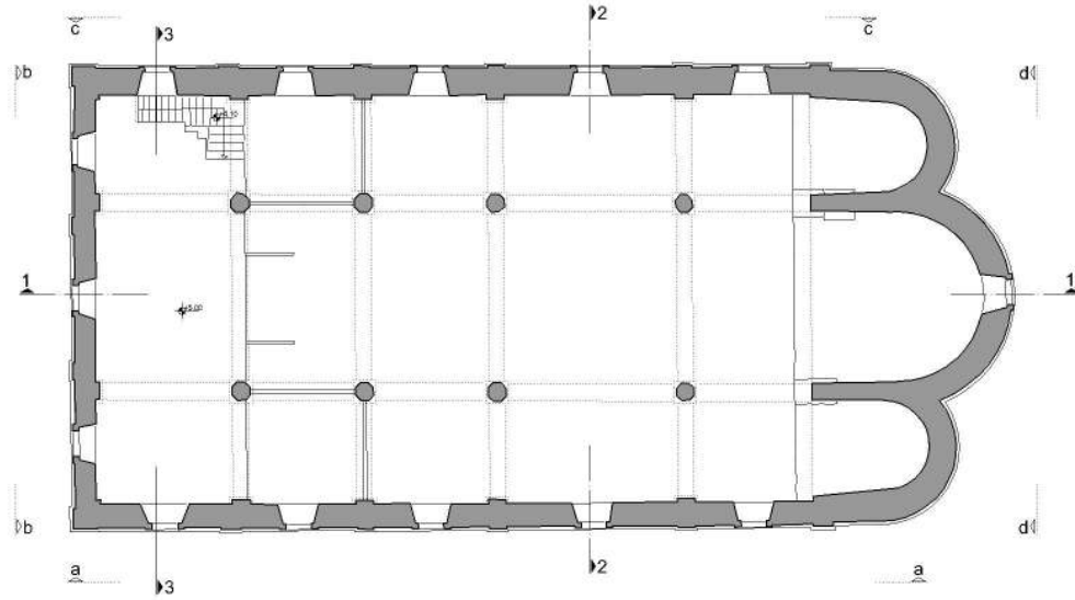
Şekil 4.24. Ordu Çok Amaçlı Salon rölöve projesi +6,50 kotu planı [KMDB arşivinden faydalanılarak Yusuf Seven tarafından yeniden çizilmiştir].
