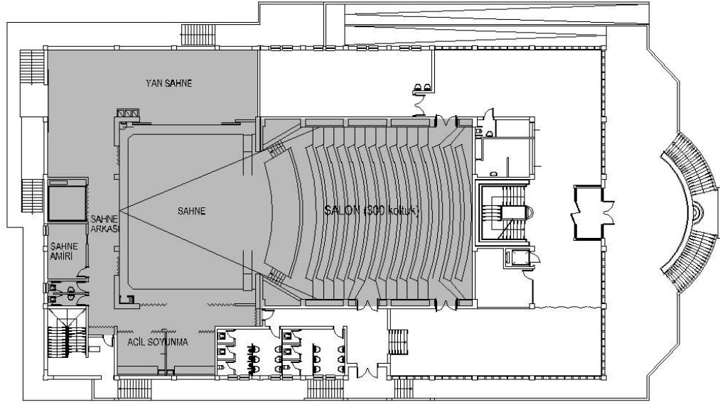
Şekil 3.3. Tip A1 KM zemin kat planı çok amaçlı salon gösterimi [KMDB arşivinden faydalanılarak Yusuf Seven tarafından yeniden düzenlenmiştir].
