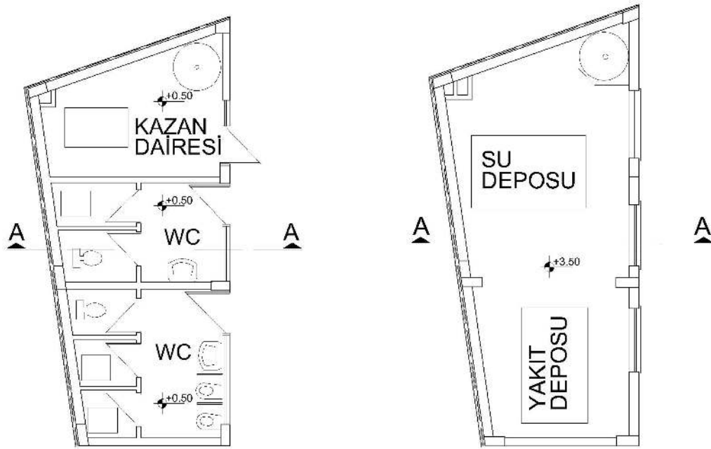
Şekil 4.43. Ordu Çok Amaçlı Salon teknik bina +0,50 ve +3,20 kotları planları [KMDB arşivinden faydalanılarak Yusuf Seven tarafından yeniden çizilmiştir].
