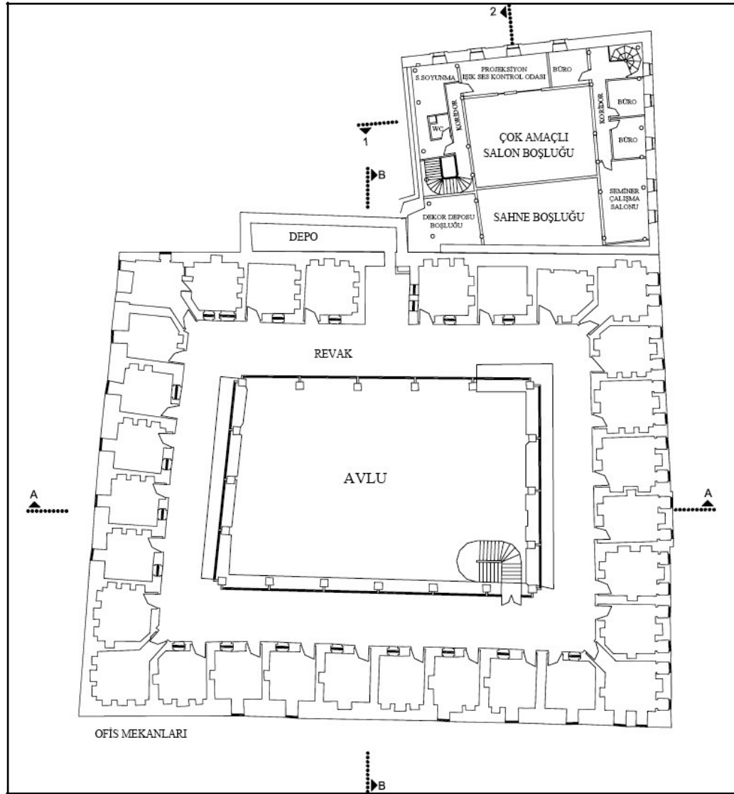
Şekil 4.6. Edirne Deveci Han 1. kat planı [Yılmaz, 2006].
