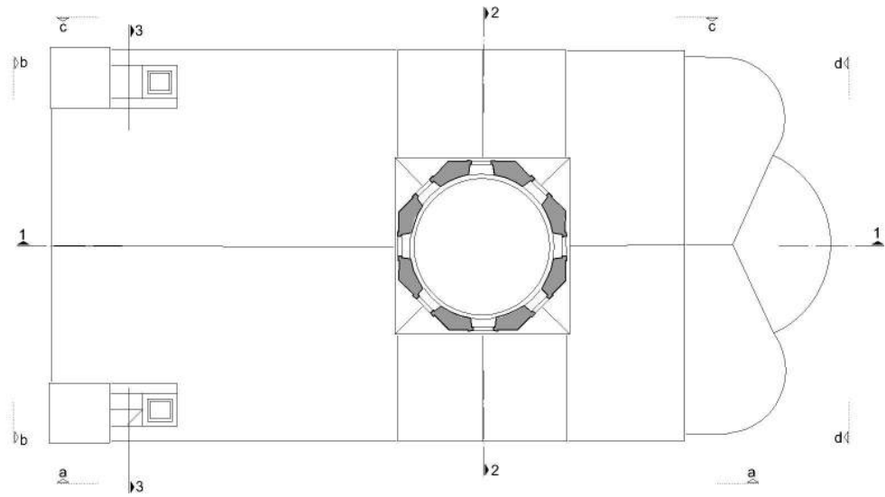
Şekil 4.25. Ordu Çok Amaçlı Salon rölöve projesi +15,00 kotu planı [KMDB arşivinden faydalanılarak Yusuf Seven tarafından yeniden çizilmiştir].
