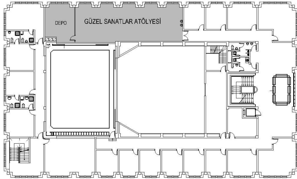
Şekil 3.10. Tip A1 KM 1. kat planı güzel sanatlar atölyesi gösterimi [KMDB arşivinden faydalanılarak Yusuf Seven tarafından yeniden düzenlenmiştir].
