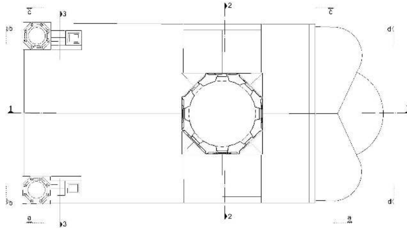
Şekil 4.35. Ordu Çok Amaçlı Salon restorasyon projesi +15,00 kotu planı [KMDB arşivinden faydalanılarak Yusuf Seven tarafından yeniden çizilmiştir].
