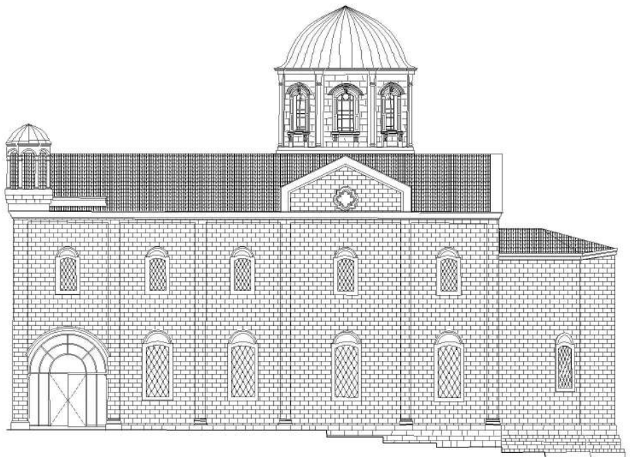
Şekil 4.39. Ordu Çok Amaçlı Salon restorasyon projesi a-a görünüşü [KMDB arşivinden faydalanılarak Yusuf Seven tarafından yeniden çizilmiştir].
