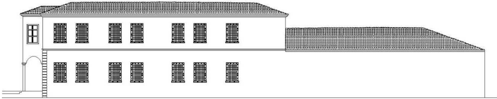
Şekil 4.16. Muğla Kültür Merkezi rölöve güney cephesi [KMDB arşivinden faydalanılarak Yusuf Seven tarafından yeniden çizilmiştir].
