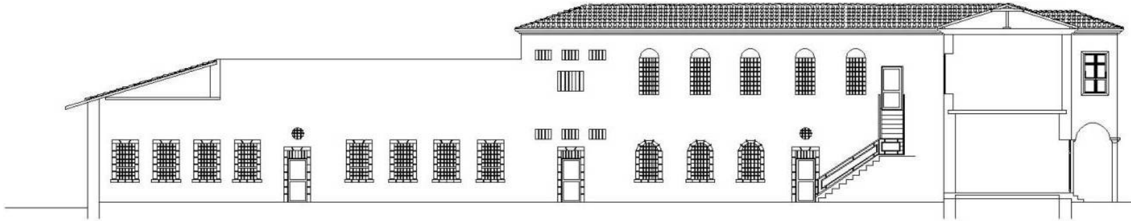
Şekil 4.13. Muğla Kültür Merkezi rölöve B-B kesiti [KMDB arşivinden faydalanılarak Yusuf Seven tarafından yeniden çizilmiştir].
