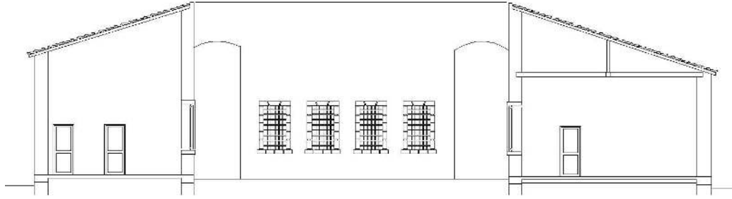
Şekil 4.14. Muğla Kültür Merkezi rölöve C-C kesiti [KMDB arşivinden faydalanılarak Yusuf Seven tarafından yeniden çizilmiştir].
