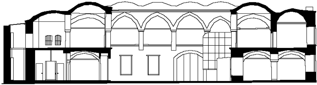
Şekil 4.7. Edirne Deveci Han B-B kesiti [Yılmaz, 2006].
