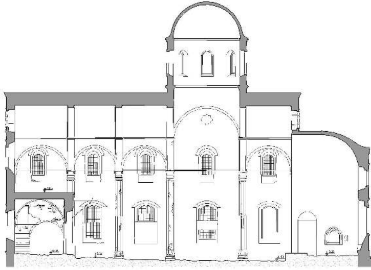
Şekil 4.26. Ordu Çok Amaçlı Salon rölöve projesi 1-1 kesiti [KMDB arşivinden faydalanılarak Yusuf Seven tarafından yeniden çizilmiştir].
