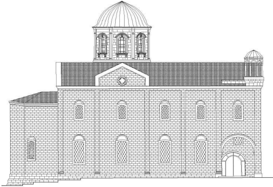
Şekil 4.40. Ordu Çok Amaçlı Salon restorasyon projesi d-d görünüşü [KMDB arşivinden faydalanılarak Yusuf Seven tarafından yeniden çizilmiştir].
