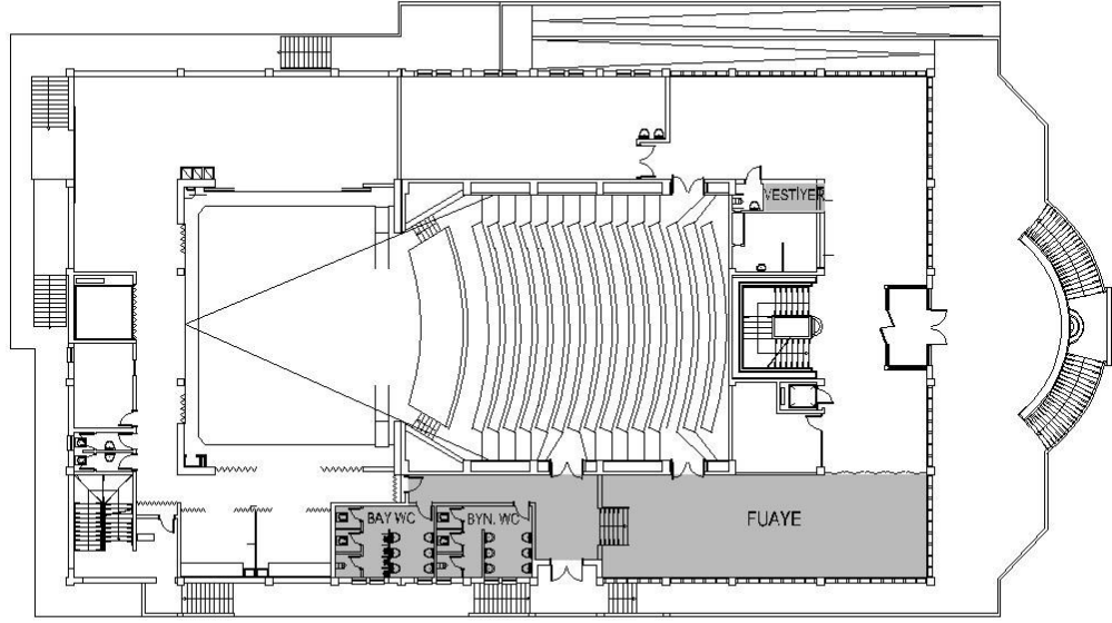
Şekil 3.2. Tip A1 KM zemin kat planı fuaye gösterimi [KMDB arşivinden faydalanılarak Yusuf Seven tarafından yeniden düzenlenmiştir].
