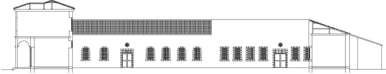
Şekil4.12. Muğla Kültür Merkezi rölöve A-A kesiti [KMDB arşivinden faydalanılarak Yusuf Seven tarafından yeniden çizilmiştir].
