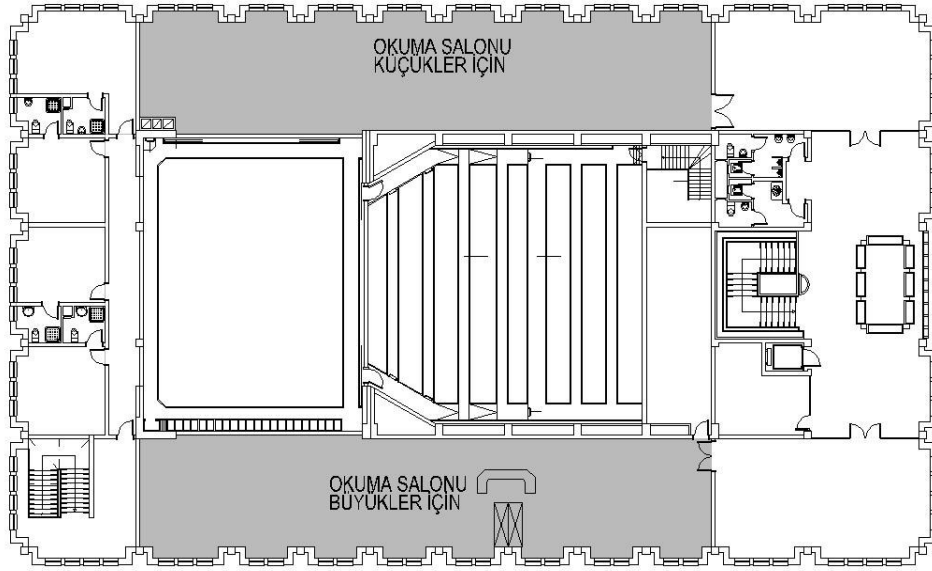
Şekil 3.11. Tip A1 KM 2. kat planı okuma salonları gösterimi [KMDB arşivinden faydalanılarak Yusuf Seven tarafından yeniden düzenlenmiştir].
