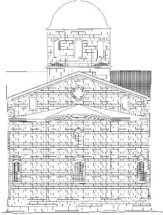
Şekil 4.32. Ordu Çok Amaçlı Salon rölöve projesi d-d görünüşü [KMDB arşivinden faydalanılarak Yusuf Seven tarafından yeniden çizilmiştir].
