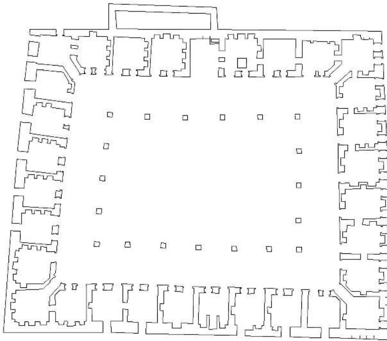
Şekil 4.2. Edirne Deveci Han 1. kat rölöve planı [KMDB arşivinden faydalanılarak Yusuf Seven tarafından yeniden çizilmiştir].
