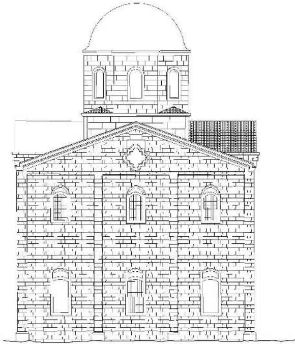
Şekil 4.31. Ordu Çok Amaçlı Salon rölöve projesi b-b görünüşü [KMDB arşivinden faydalanılarak Yusuf Seven tarafından yeniden çizilmiştir].
