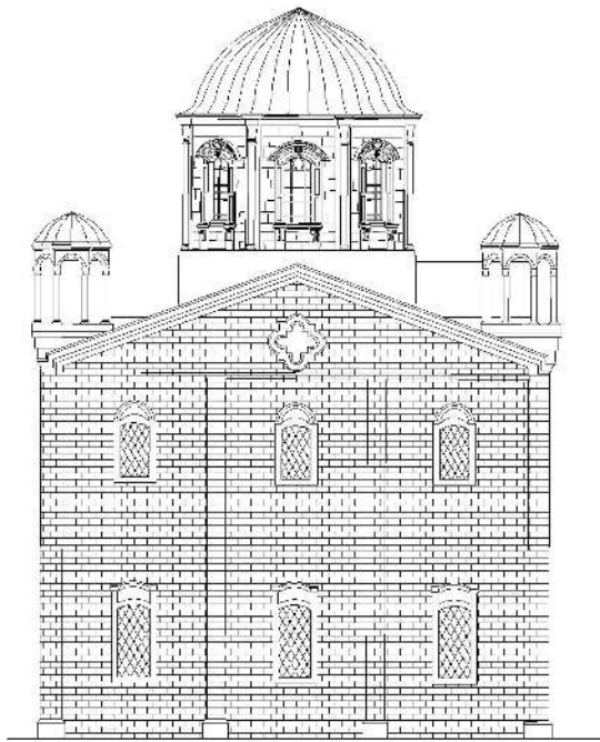
Şekil 4.41. Ordu Çok Amaçlı Salon restorasyon projesi b-b görünüşü [KMDB arşivinden faydalanılarak Yusuf Seven tarafından yeniden çizilmiştir].
