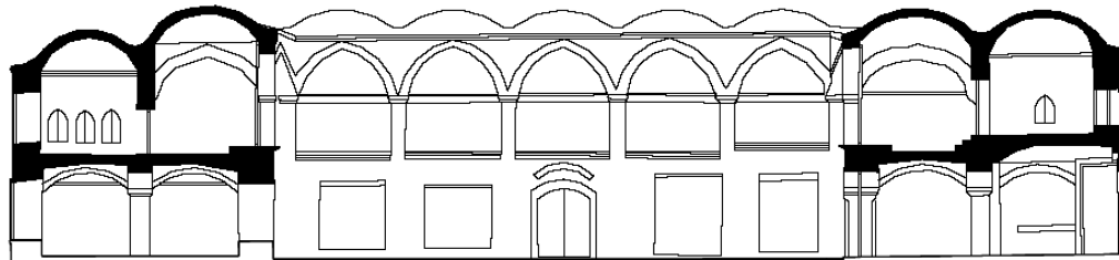
Şekil 4.5. Edirne Deveci A-A kesiti [Yılmaz, 2006].
