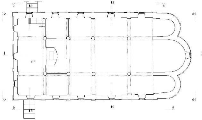
Şekil 4.34. Ordu Çok Amaçlı Salon restorasyon projesi +6,50 kotu planı [KMDB arşivinden faydalanılarak Yusuf Seven tarafından yeniden çizilmiştir].
