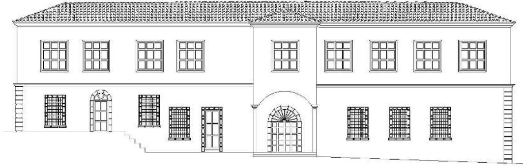
Şekil 4.15. Muğla Kültür Merkezi rölöve batı (giriş) cephesi [KMDB arşivinden faydalanılarak Yusuf Seven tarafından yeniden çizilmiştir].
