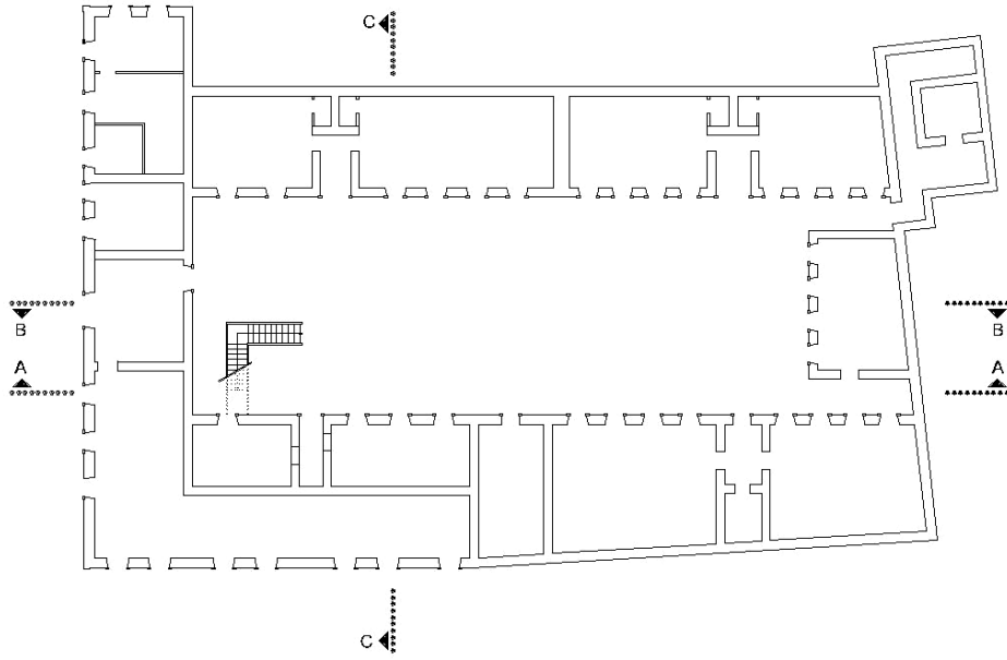
Şekil 4.10. Muğla Kültür Merkezi zemin kat rölöve planı [KMDB arşivinden faydalanılarak Yusuf Seven tarafından yeniden çizilmiştir].
