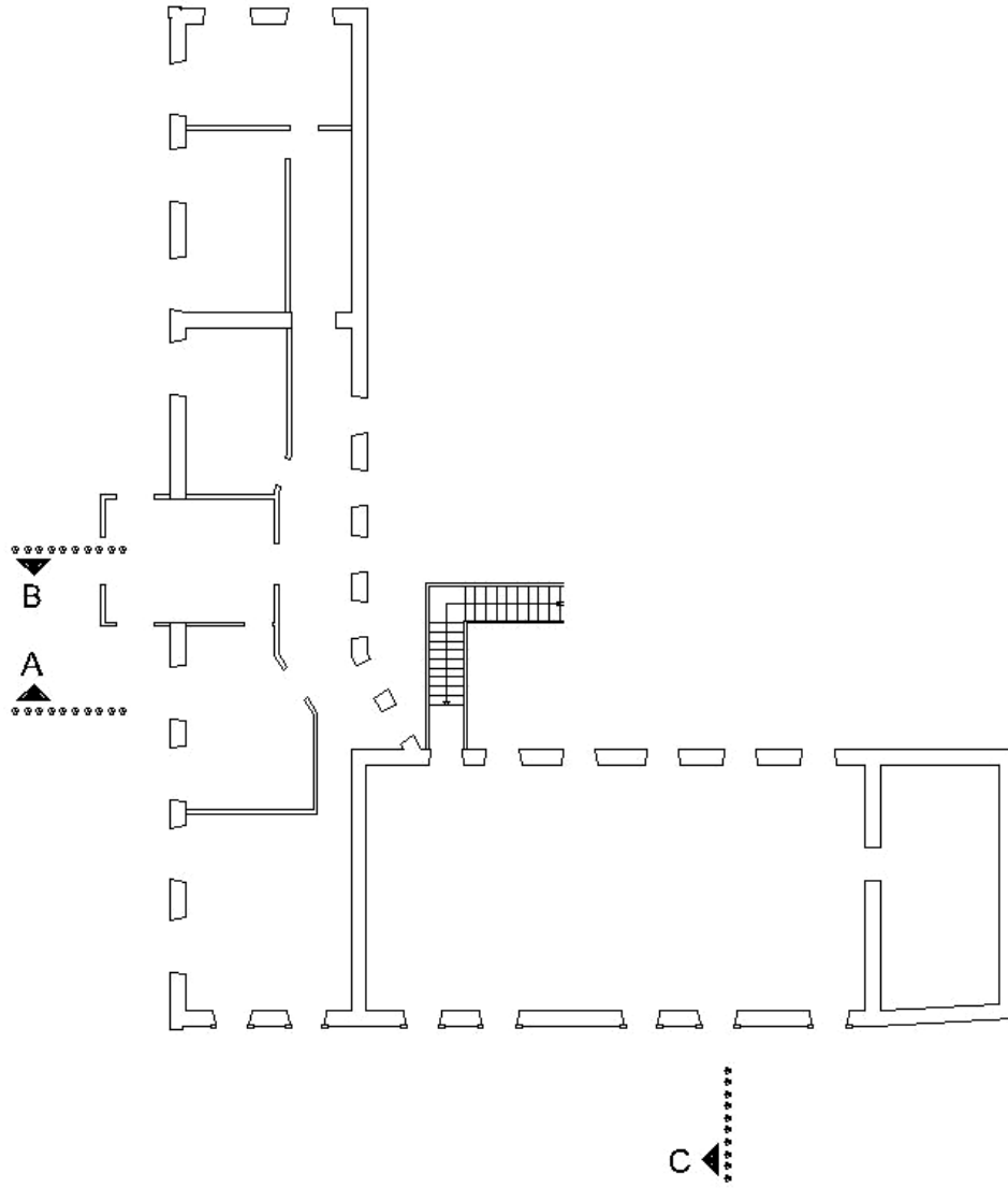
Şekil 4.11. Muğla Kültür Merkezi 1. kat rölöve planı [KMDB arşivinden faydalanılarak Yusuf Seven tarafından yeniden çizilmiştir].
