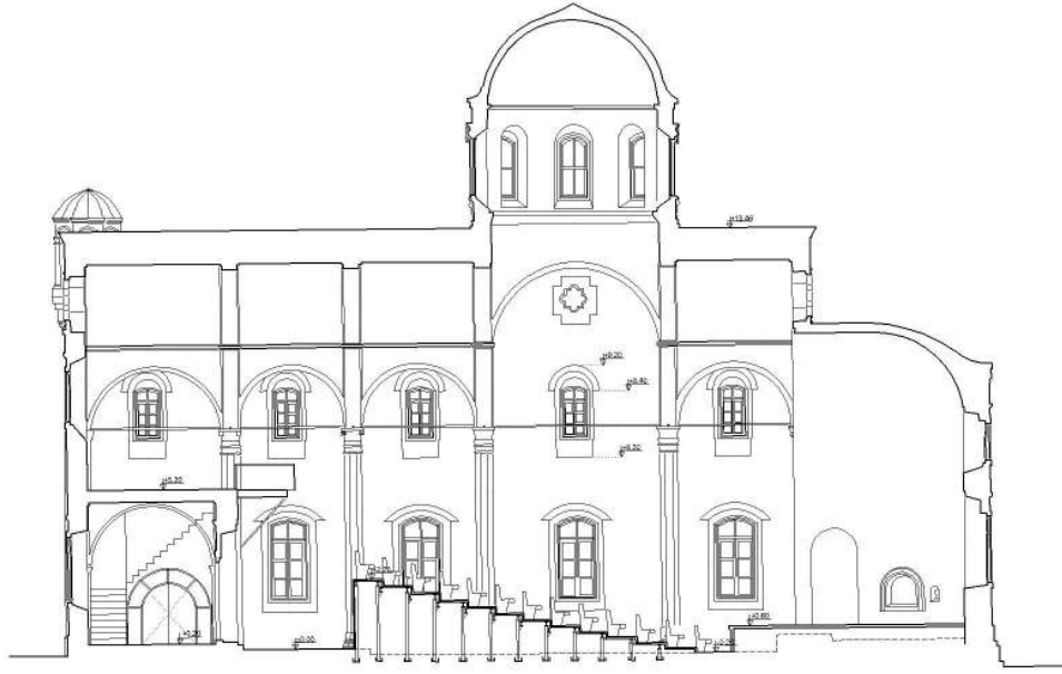
Şekil 4.36. Ordu Çok Amaçlı Salon restorasyon projesi 1-1 kesiti [KMDB arşivinden faydalanılarak Yusuf Seven tarafından yeniden çizilmiştir].
