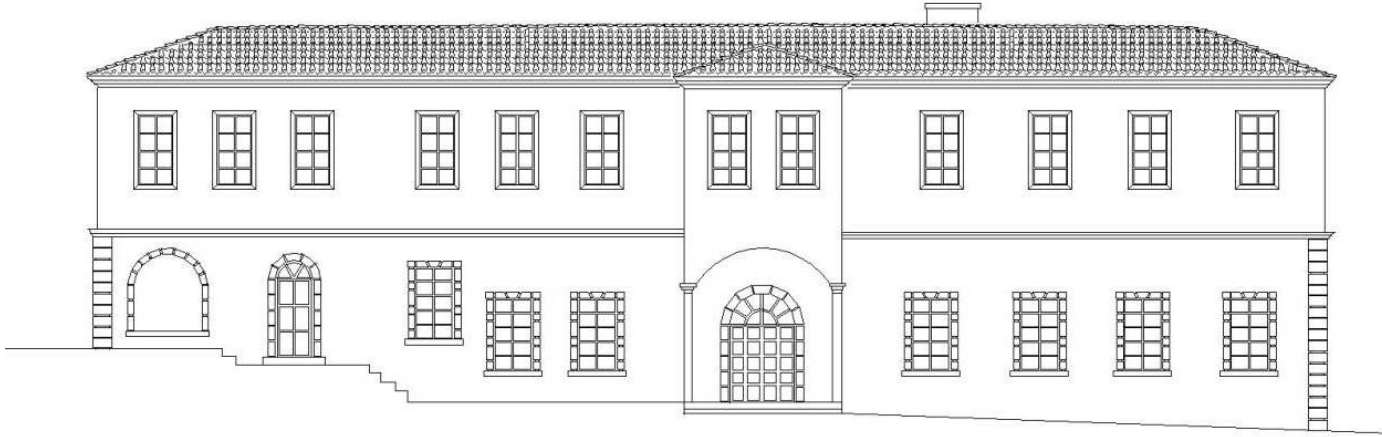
Şekil 4.21. Muğla KM batı cephesi [KMDB arşivinden faydalanılarak Yusuf Seven tarafından yeniden çizilmiştir].
