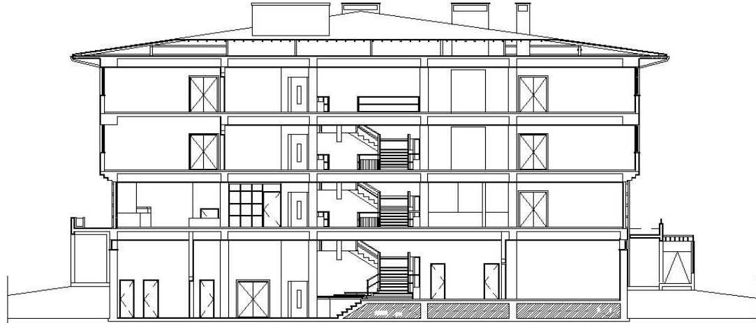
Şekil 3.18. Tip A1 KM B-B kesiti [KMDB arşivinden faydalanılarak Yusuf Seven tarafından yeniden düzenlenmiştir].
