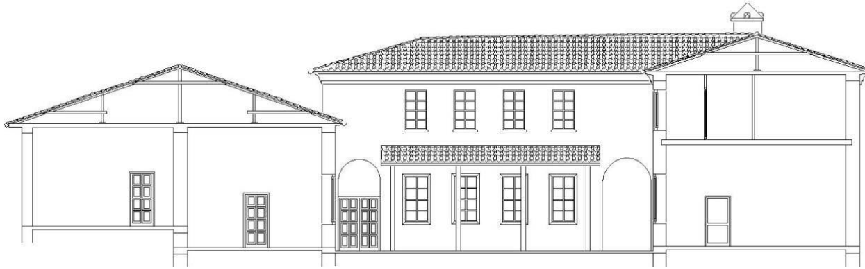
Şekil 4.20. Muğla Kültür Merkezi B-B kesiti [KMDB arşivinden faydalanılarak Yusuf Seven tarafından yeniden çizilmiştir].
