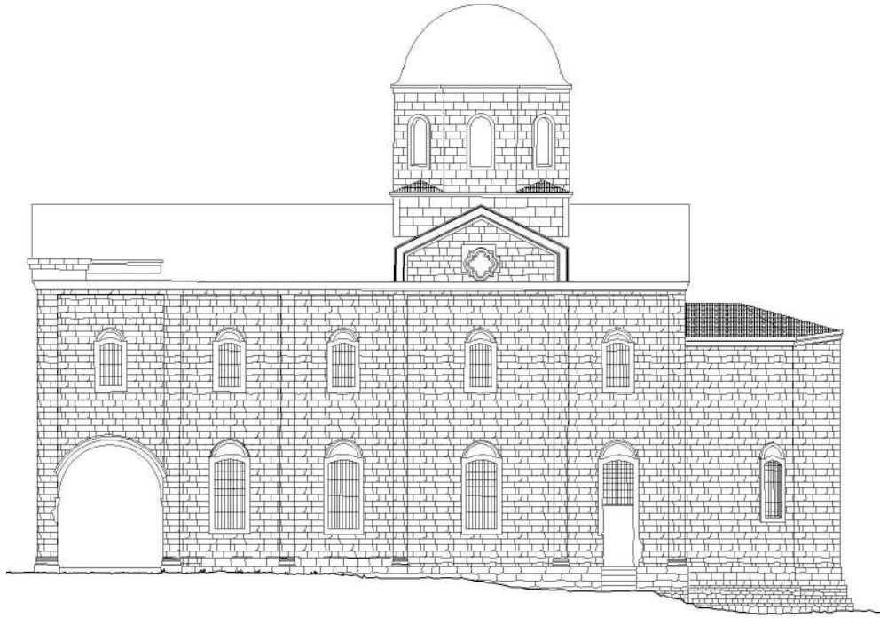
Şekil 4.29. Ordu Çok Amaçlı Salon rölöve projesi a-a görünüşü [KMDB arşivinden faydalanılarak Yusuf Seven tarafından yeniden çizilmiştir].
