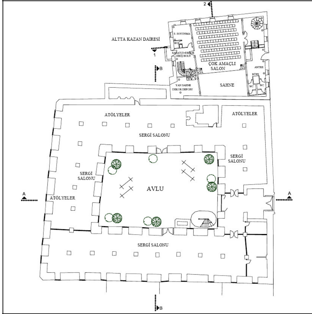
Şekil 4.4. Edirne Deveci Han zemin kat planı [Yılmaz, 2006]
