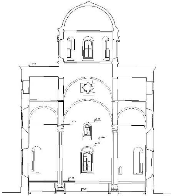
Şekil 4.37. Ordu Çok Amaçlı Salon restorasyon projesi 2-2 kesiti [KMDB arşivinden faydalanılarak Yusuf Seven tarafından yeniden çizilmiştir].
