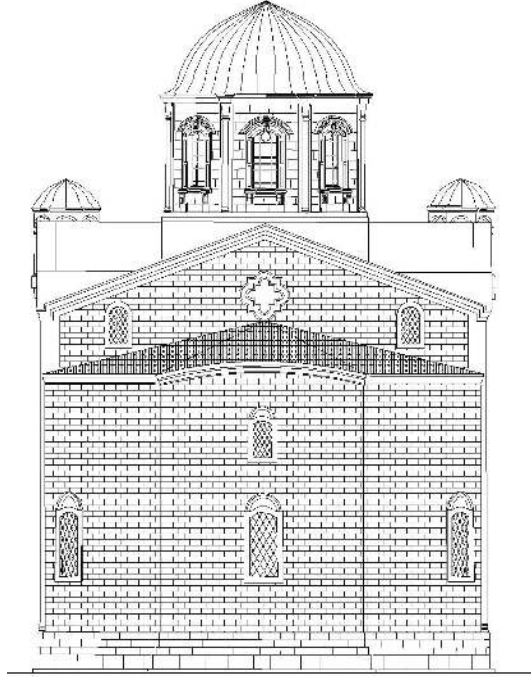
Şekil 4.42. Ordu Çok Amaçlı Salon restorasyon projesi c-c görünüşü [KMDB arşivinden faydalanılarak Yusuf Seven tarafından yeniden çizilmiştir].
