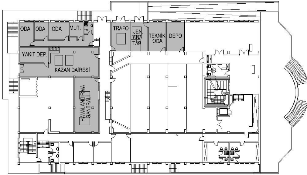
Şekil 3.16. Tip A1 KM bodrum kat planı teknik mekanlar gösterimi (KMDB arşivinden faydalanılarak Yusuf Seven tarafından yeniden düzenlenmiştir.)
