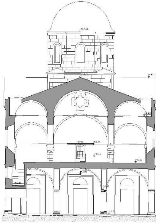
Şekil 4.28. Ordu Çok Amaçlı Salon rölöve projesi 3-3 kesiti [KMDB arşivinden faydalanılarak Yusuf Seven tarafından yeniden çizilmiştir].
