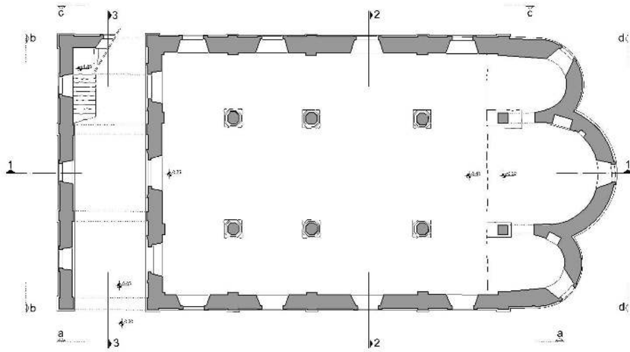
Şekil 4.23. Ordu Çok Amaçlı Salon rölöve projesi +2,00 kotu planı [KMDB arşivinden faydalanılarak Yusuf Seven tarafından yeniden çizilmiştir].
