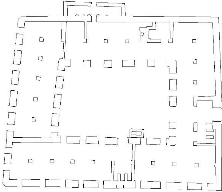
Şekil 4.1. Edirne Deveci Han zemin kat rölöve planı [KMDB arşivinden faydalanılarak Yusuf Seven tarafından yeniden çizilmiştir].
