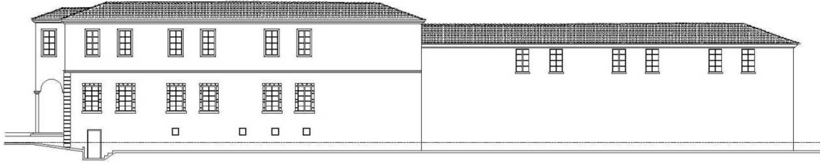
Şekil 4.22. Muğla KM güney cephesi [KMDB arşivinden faydalanılarak Yusuf Seven tarafından yeniden çizilmiştir].
