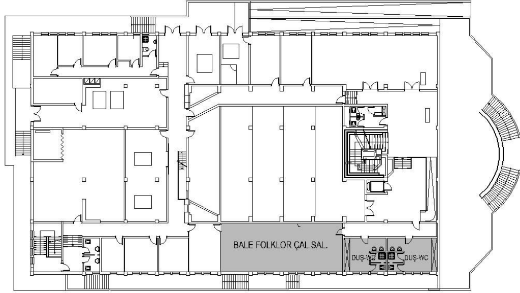
Şekil 3.7. Tip A1 KM bodrum kat planı bale folklor çalışma salonu gösterimi [KMDB arşivinden faydalanılarak Yusuf Seven tarafından yeniden düzenlenmiştir].
