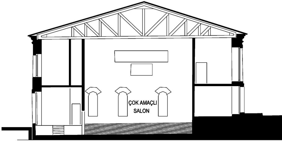
Şekil 4.8. Edirne Deveci Han 1-1 kesiti [Yılmaz, 2006].
