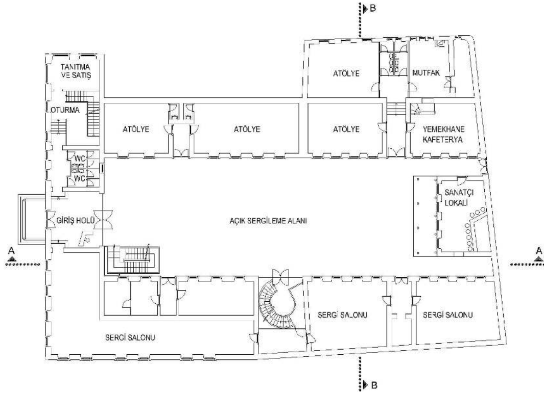
Şekil 4.17. Muğla Kültür Merkezi zemin kat planı [KMDB arşivinden faydalanılarak Yusuf Seven tarafından yeniden çizilmiştir].
