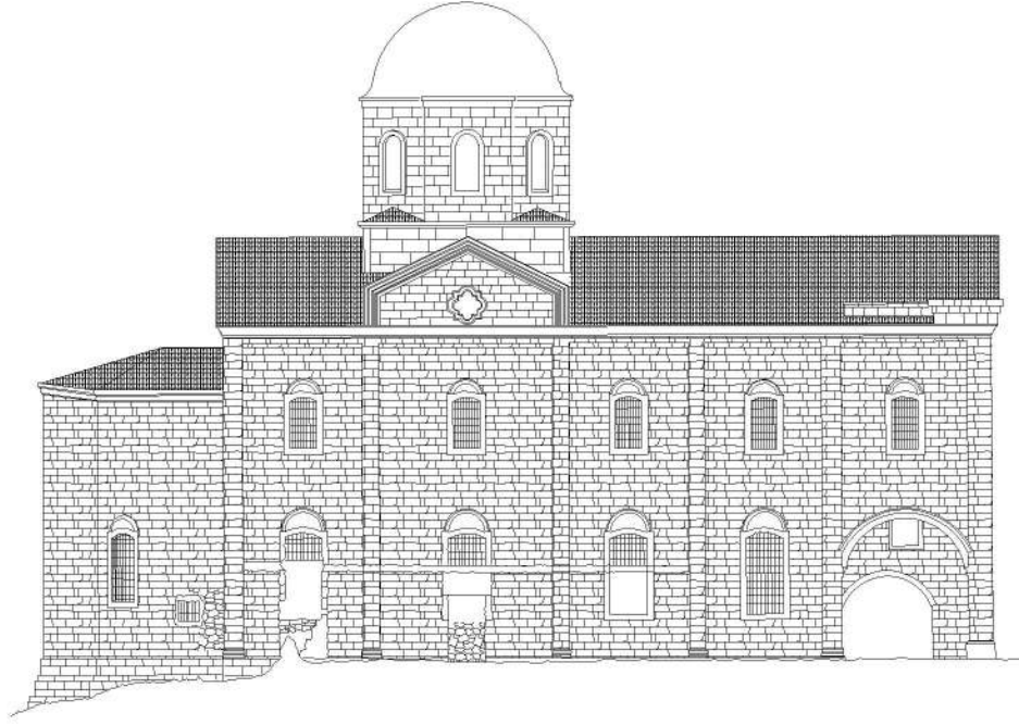
Şekil 4.30. Ordu Çok Amaçlı Salon rölöve projesi d-d görünüşü [KMDB arşivinden faydalanılarak Yusuf Seven tarafından yeniden çizilmiştir].
