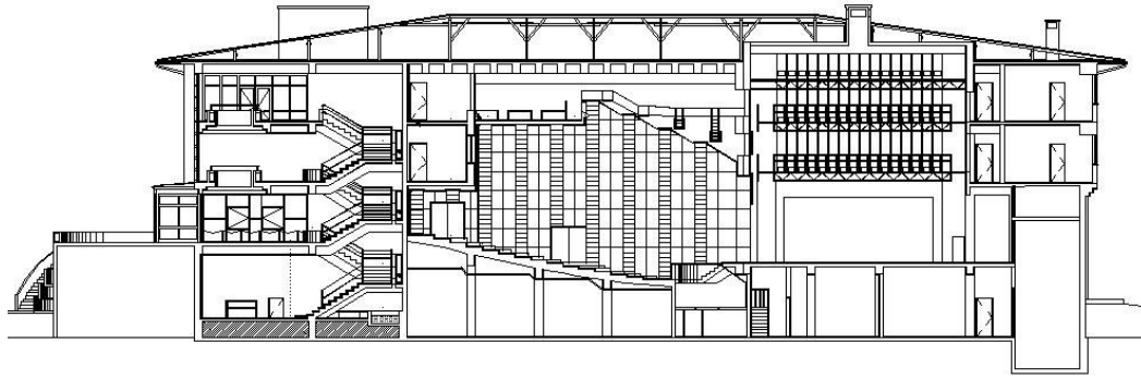
Şekil 3.17. Tip A1 KM A-A kesiti [KMDB arşivinden faydalanılarak Yusuf Seven tarafından yeniden düzenlenmiştir].
