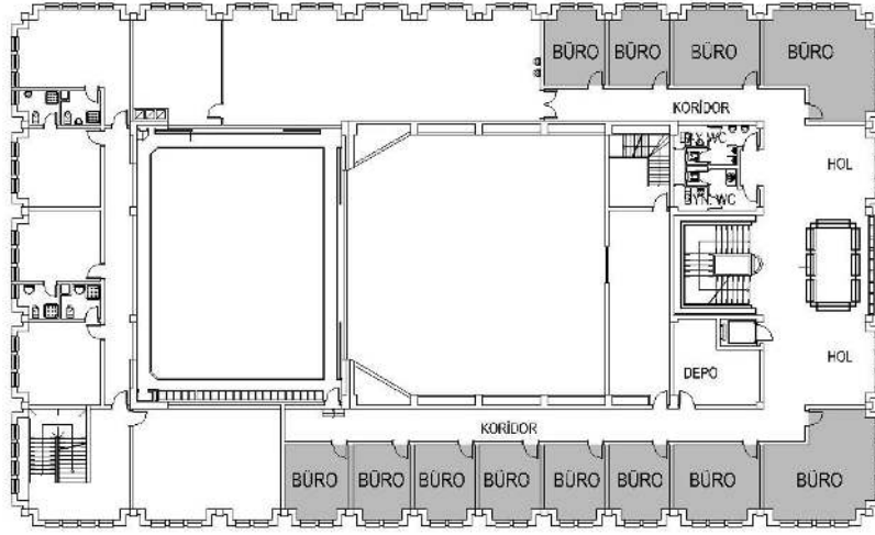
Şekil 3.12. Tip A1 KM 1. kat planı idari birimler gösterimi [KMDB arşivinden faydalanılarak Yusuf Seven tarafından yeniden düzenlenmiştir].
