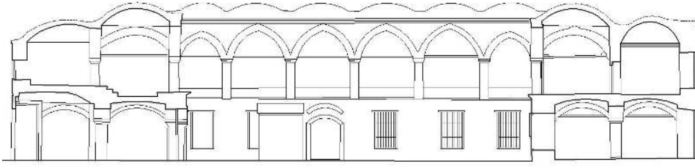
Şekil 4.3. Edirne Deveci Han rölöve kesiti [KMDB arşivinden faydalanılarak Yusuf Seven tarafından yeniden çizilmiştir].
