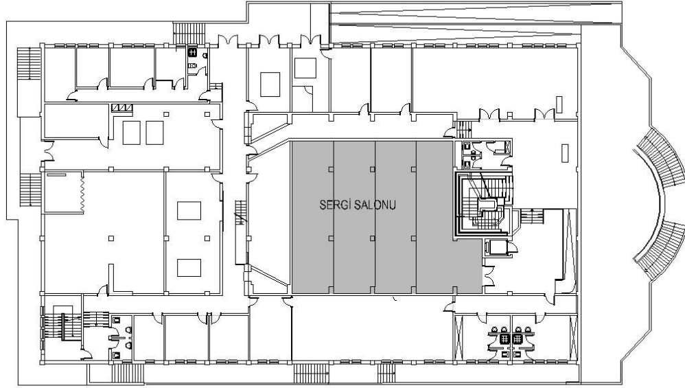
Şekil 3.8. Tip A1 KM bodrum kat planı sergi salonu gösterimi [KMDB arşivinden faydalanılarak Yusuf Seven tarafından yeniden düzenlenmiştir].
