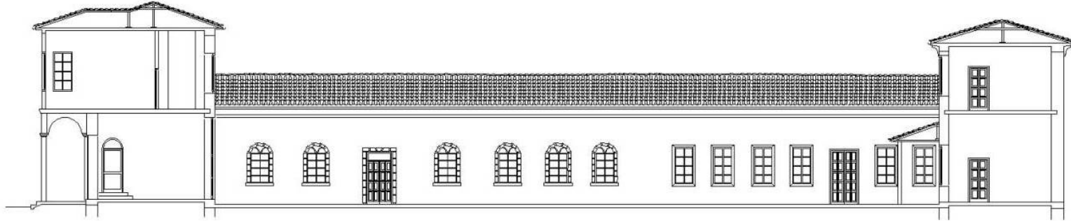
Şekil 4.19. Muğla Kültür Merkezi A-A kesiti [KMDB arşivinden faydalanılarak Yusuf Seven tarafından yeniden çizilmiştir].
