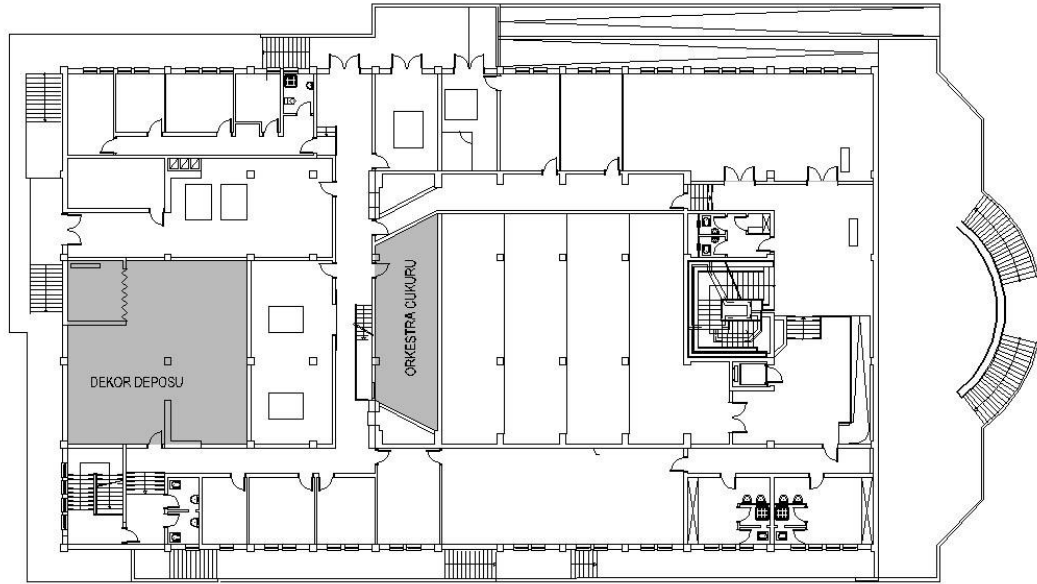
Şekil 3.5. Tip A1 KM bodrum kat planı dekor deposu ve orkestra çukuru gösterimi [KMDB arşivinden faydalanılarak Yusuf Seven tarafından yeniden düzenlenmiştir].
