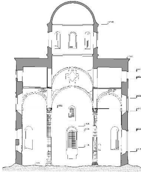
Şekil 4.27. Ordu Çok Amaçlı Salon rölöve projesi 2-2 kesiti [KMDB arşivinden faydalanılarak Yusuf Seven tarafından yeniden çizilmiştir].
