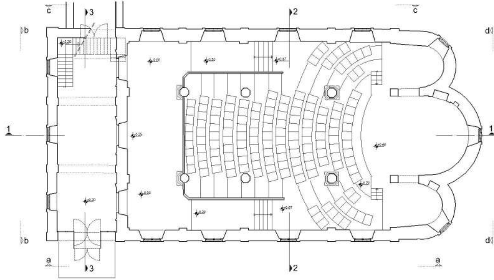
Şekil 4.33. Ordu Çok Amaçlı Salon restorasyon projesi +2,00 planı [KMDB arşivinden faydalanılarak Yusuf Seven tarafından yeniden çizilmiştir].
