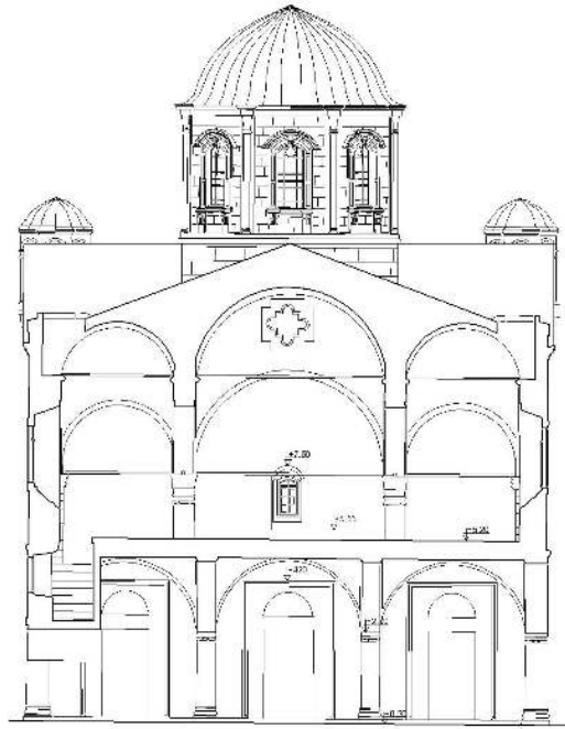
Şekil 4.38. Ordu Çok Amaçlı Salon restorasyon projesi 3-3 kesiti [KMDB arşivinden faydalanılarak Yusuf Seven tarafından yeniden çizilmiştir].
