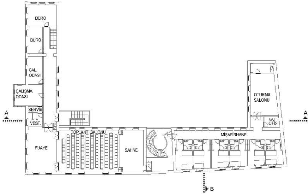
Şekil 4.18. Muğla Kültür Merkezi 1. kat planı [KMDB arşivinden faydalanılarak Yusuf Seven tarafından yeniden çizilmiştir].
