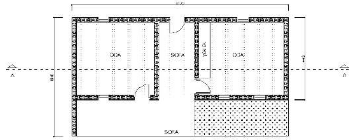
ZEMİN KAT PLANI
