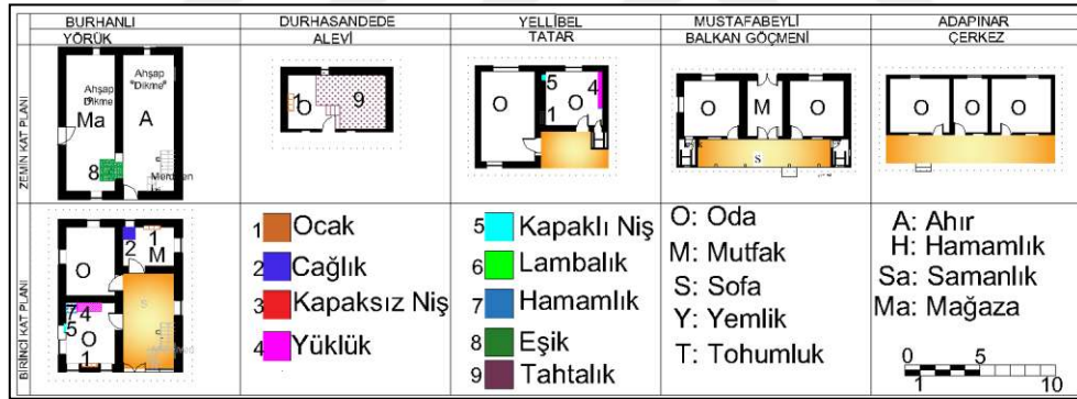
Şekil 6.62. Kat Planları Açısından Değerlendirme
