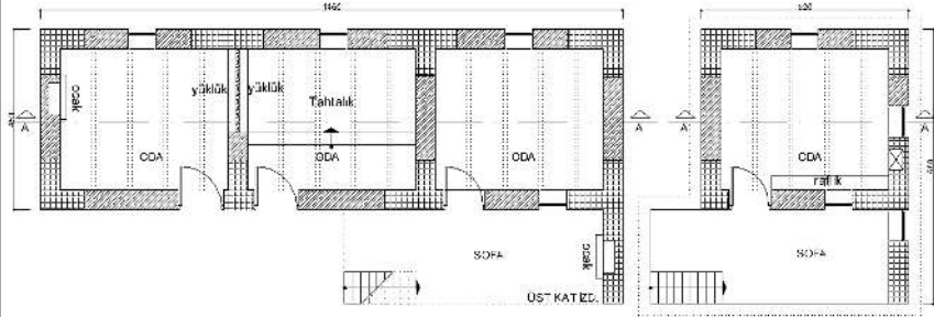
ZEMİN KAT PLANI
