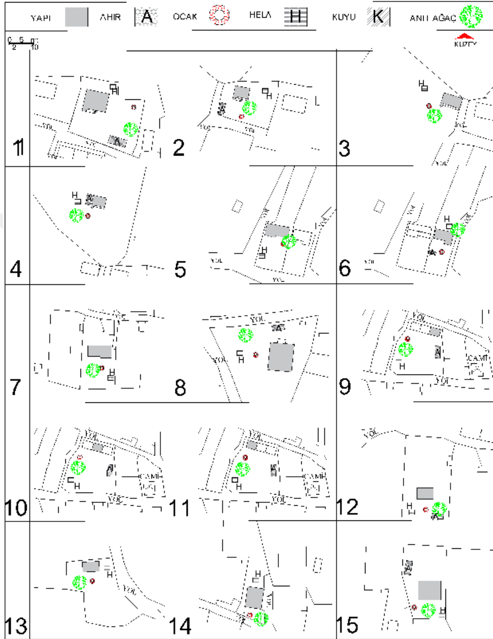
Şekil 6.32. Yellibel Köyünde Çalışma Yapılan Evlerin Vaziyet Planları
