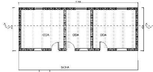
ZEMİN KAT PLANI
