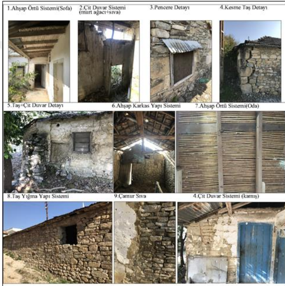
Şekil 6.36. Yelibel Köyündeki Yapım Sistemleri ve Malzemeleri (Yazarın arşivi)
