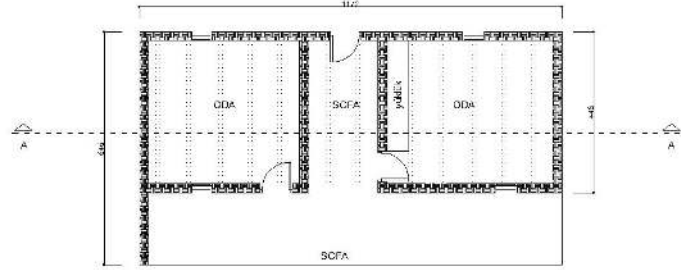
ZEMİN KAT PLANI
