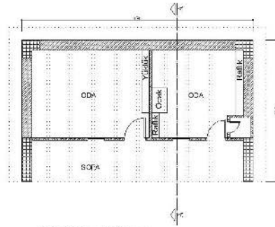
Kerpiç Eklenti Yapı Moloz Taş ZEMİN KAT PLANI Kesme Taş Çit Duvar
