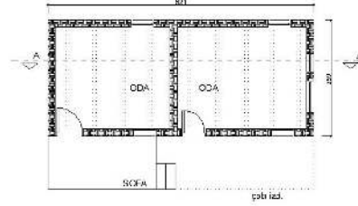
ZEMİN KAT PLANI
