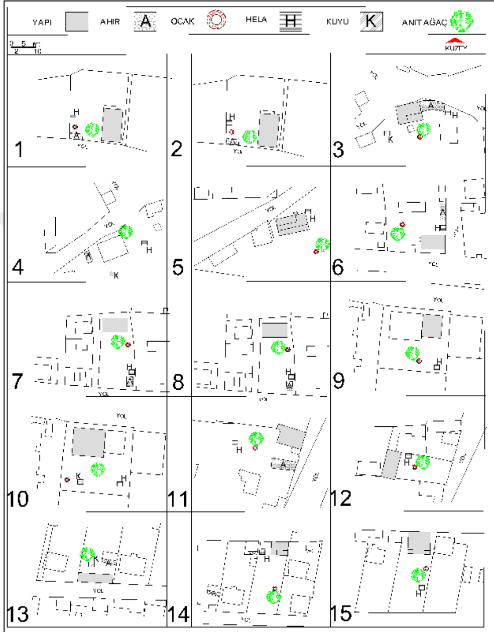
Şekil 6.43. Mustafabeyli Köyünde Çalışma Yapılan Evlerin Vaziyet Planları
