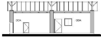
AA KESİTİ
