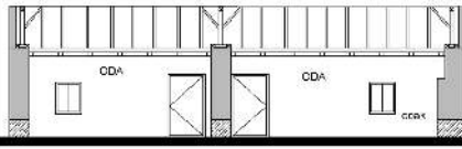
AA KESİTİ
