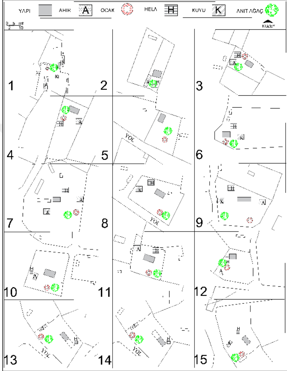
Şekil 6.53. Adapınar Köyünde Çalışma Yapılan Evlerin Vaziyet Planları
