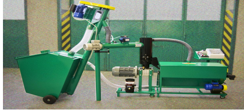
Şekil 3.3. Gübre işleme-Pelletleme
