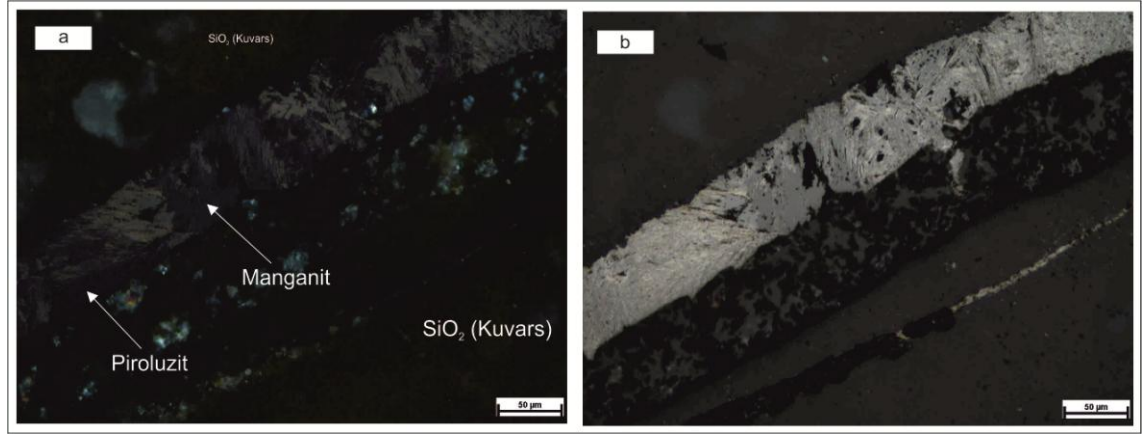
Şekil 4.13. Çift (a) ve tek (b) nikolde silisli matriks içerisinde damar halinde bulunan manganit ve piroluzit görünüşleri
