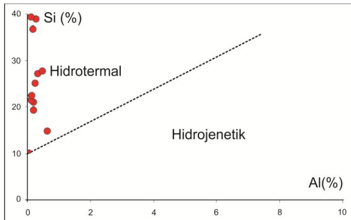
Şekil 4.24. Örneklere ait Si-Al diyagramı (Toth 1980)
