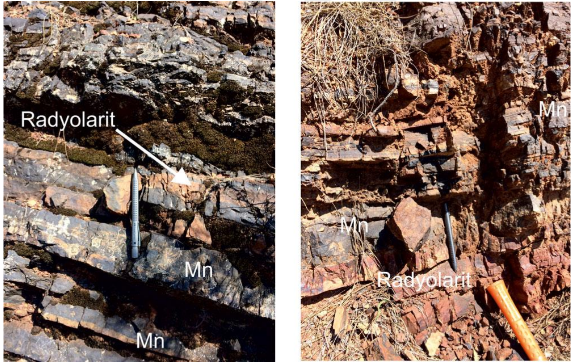
Şekil 4.1. Belen mevkinde mangan cevherleşme şekillerinin görünümü
