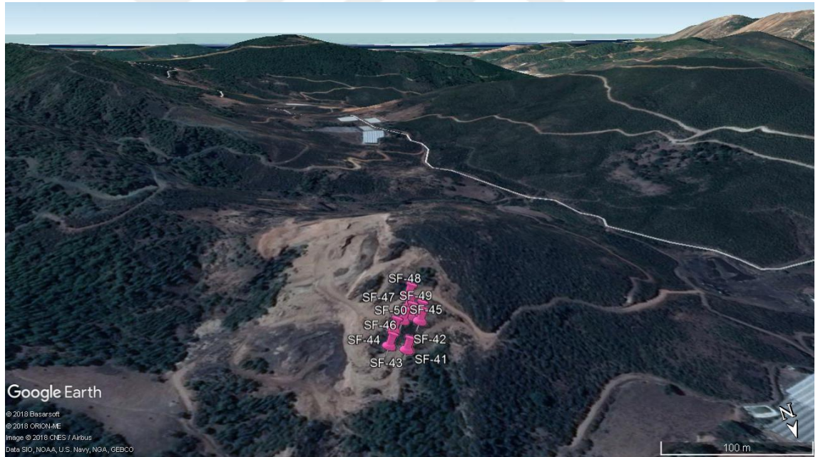
Şekil 3.4. Kumluca-Altınyaka yolu üzerindeki Asmad madenciliğe ait manganez ocağından alınan numunelerin uydu görüntüsü
