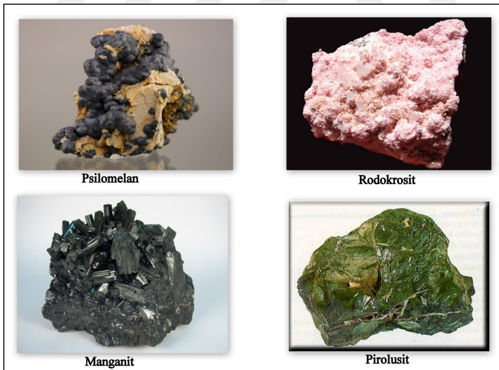
Şekil 1.5. Önemli mangan cevher mineralleri
