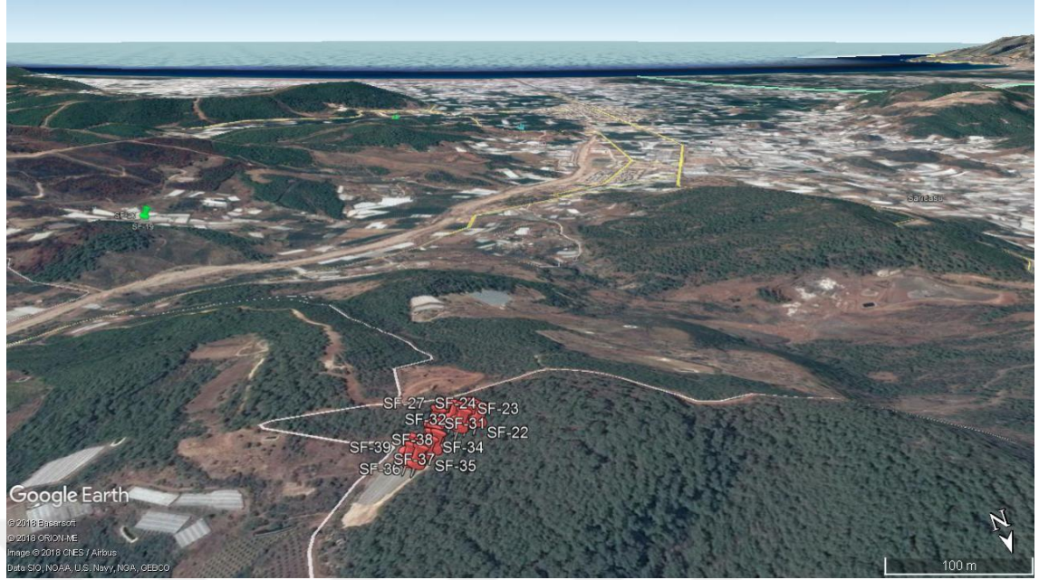
Şekil 3.3. Kumluca-Altınyaka yolu üzerindeki eski hafriyat ocağından alınan numunelerin uydu görüntüsü
