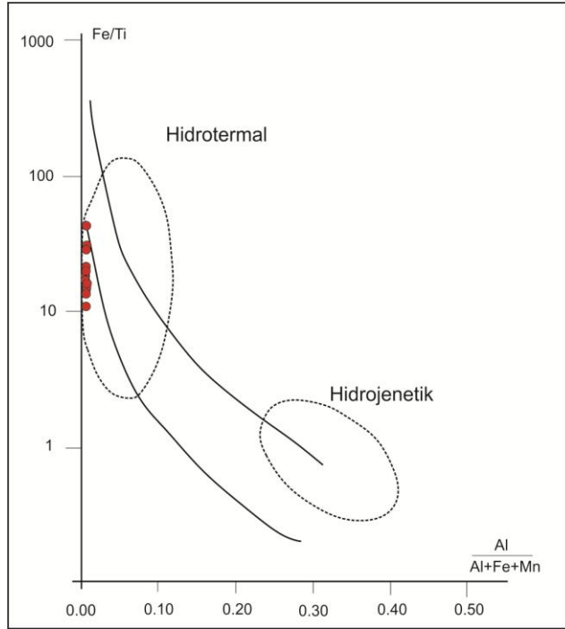
Şekil 4.27. Pelajik çökellerdeki malzemenin kökensel karşılaştırılması (Boström 1970)
