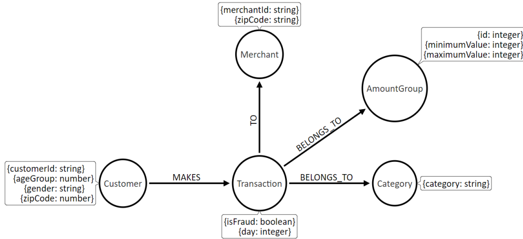
Şekil 6.2. Önerilen çizge veritabanı modeli.
