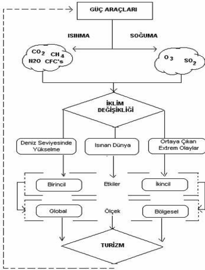
Şekil 4.18. İklim değişiklikleri ile turizm arasındaki ilişki (Giles Andrew ve Perry Allen, 1998).
