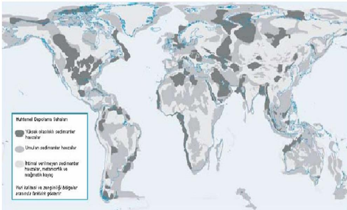
Şekil 4.26. Karbon depolamada kullanılabilecek uygun tuz formasyonları, petrol veya gaz arazileri ya da kömür yataklarının bulunabileceği sedimanter havzalardaki muhtemel bölgeler (Ecosystem,
