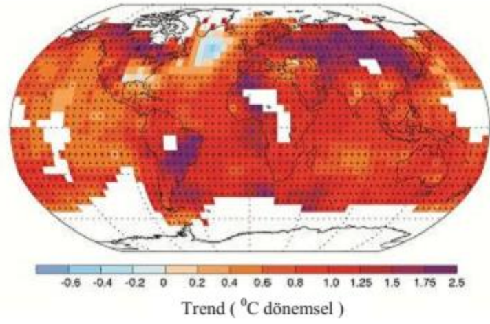
Şekil 2.1.b. 1901-2012 ortalama yüzey sıcaklığında gözlenmiş değişim (IPCC, 2013).
