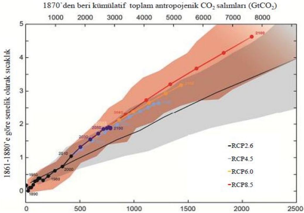
Şekil 2.9. CO 2 'nin kümülatif yayılımlarının küresel yüzey ısınmasına etkisi (IPCC, 2013).
