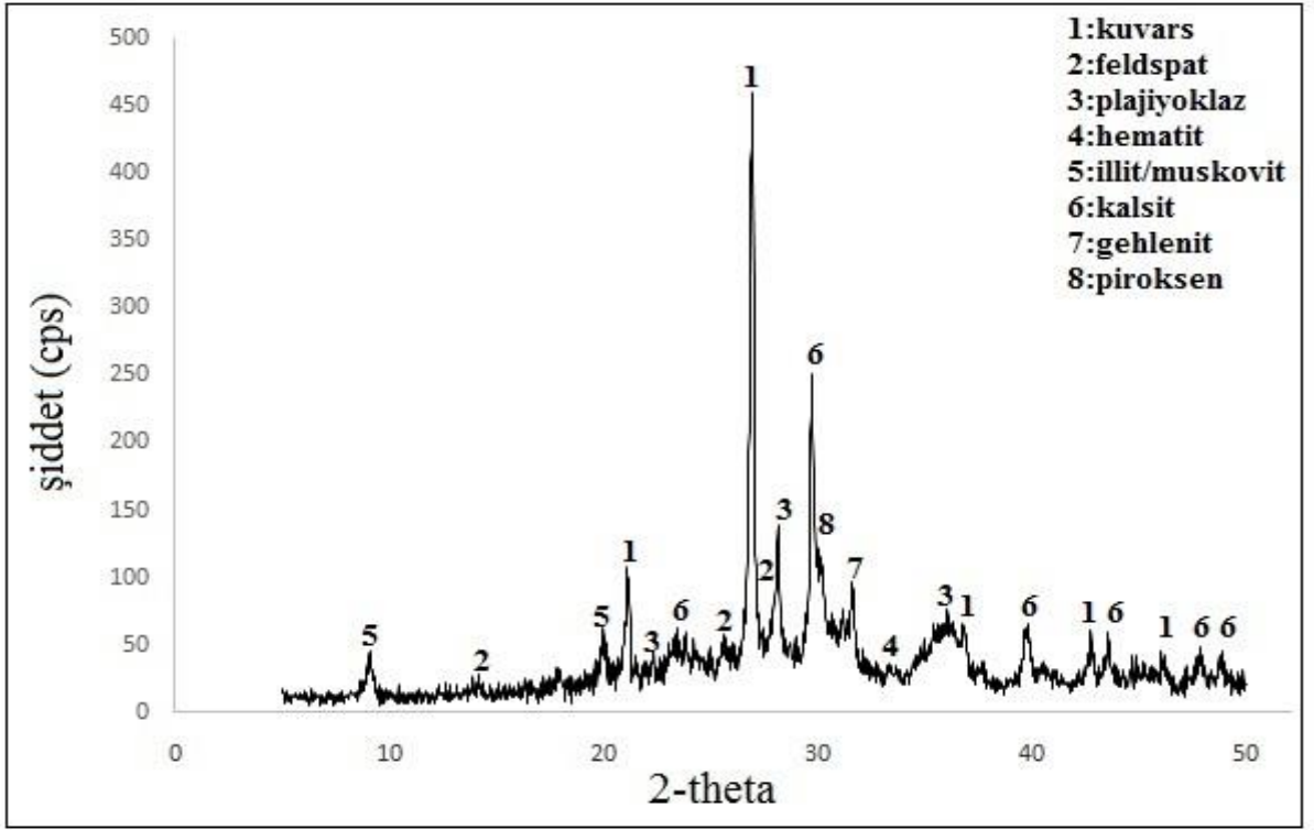
Şekil 4. 3. MA-3 kodlu seramiğe ait XRD paterni.
