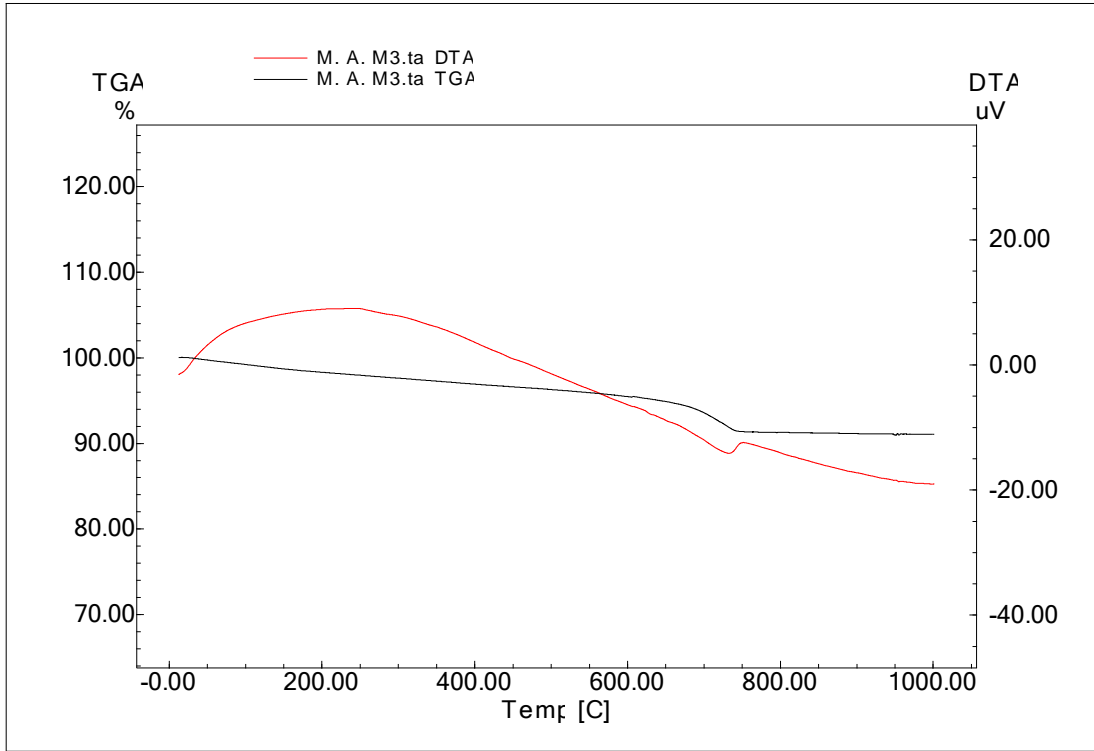
Şekil 4. 25. MA-3 kodlu seramiğe ait TG-DTA diyagramı
