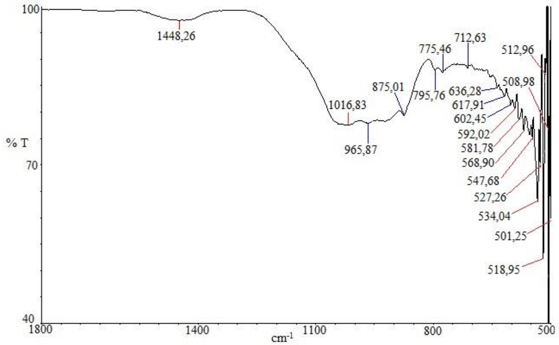
Şekil 4. 45. MA-1 kodlu seramik örneğe ait FTIR spektrumu
