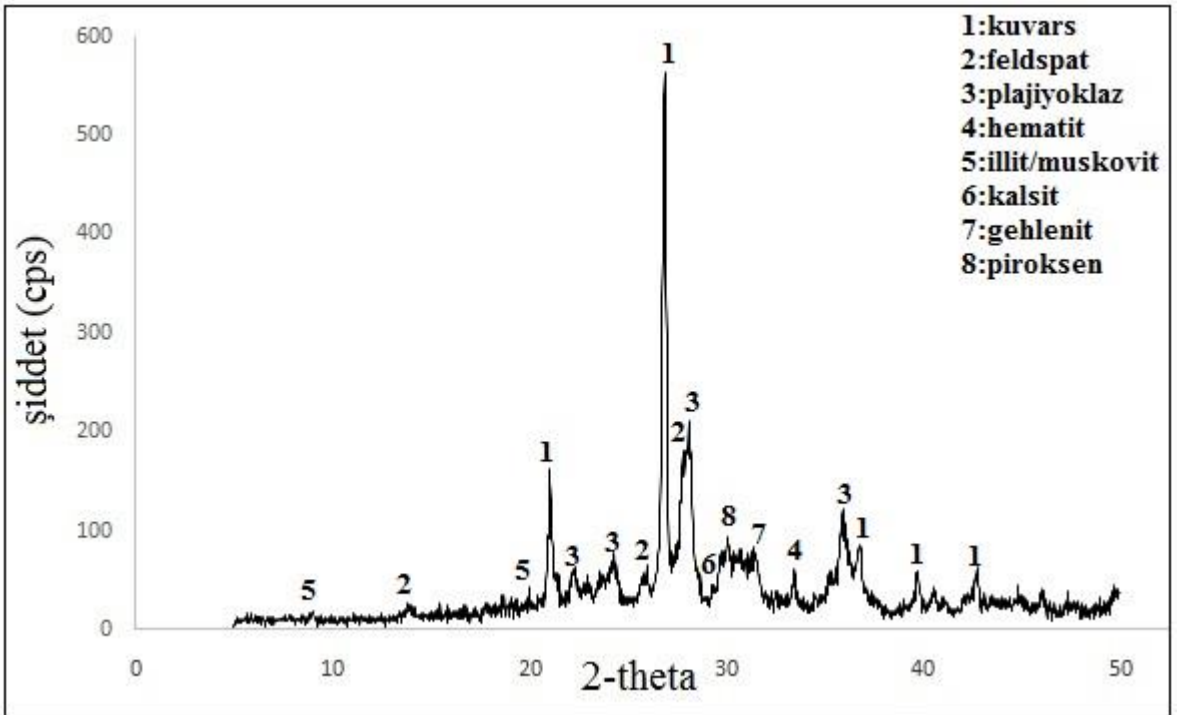
Şekil 4. 12. MA-12 kodlu seramiğe ait XRD paterni
