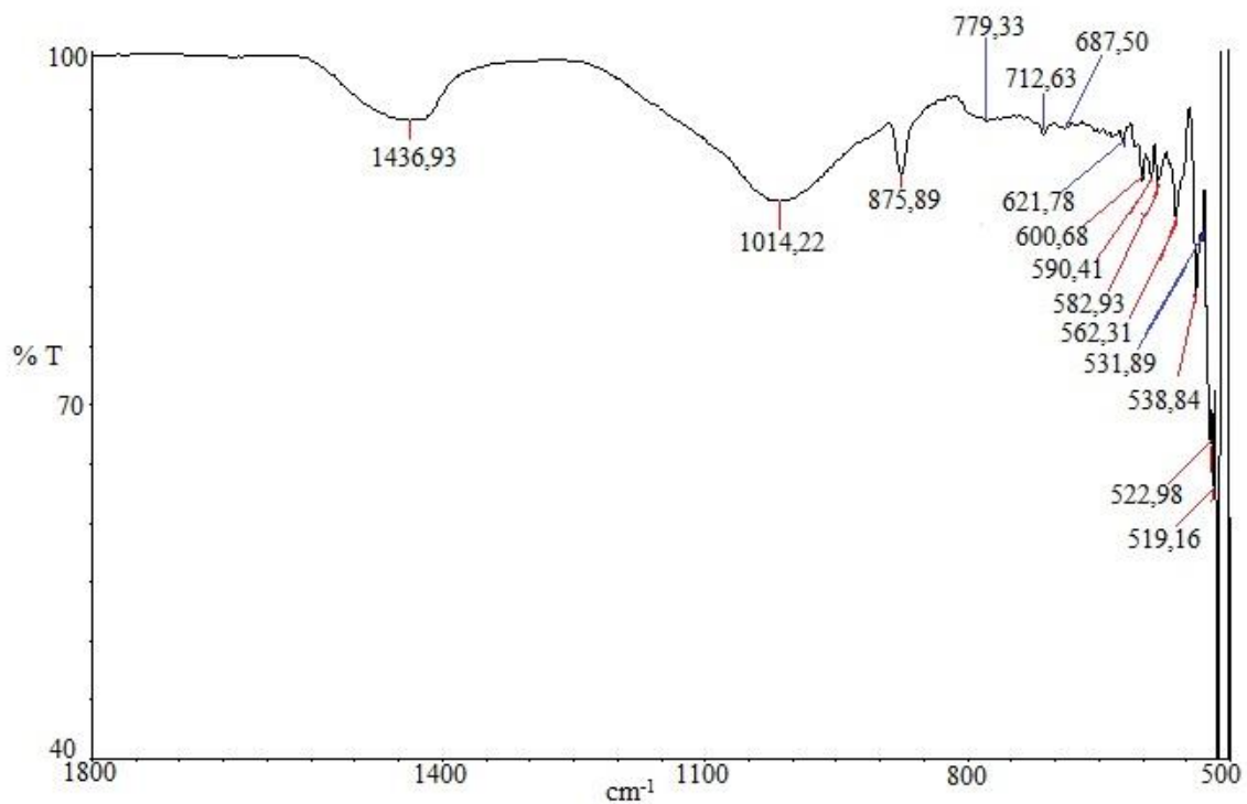
Şekil 4. 46. MA-2 kodlu seramik örneğe ait FTIR spektrumu
