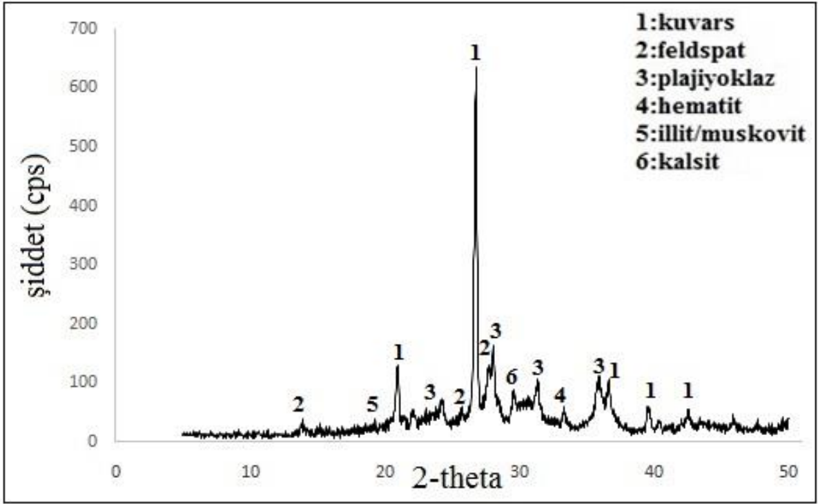
Şekil 4. 15. MA-15 kodlu seramiğe ait XRD paterni
