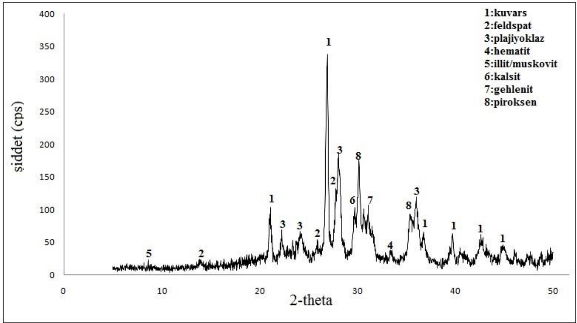
Şekil 4. 1. MA-1 kodlu seramiğe ait XRD paterni
