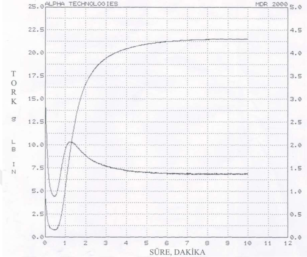
Şekil 4.1. Rheometre eğrisi
