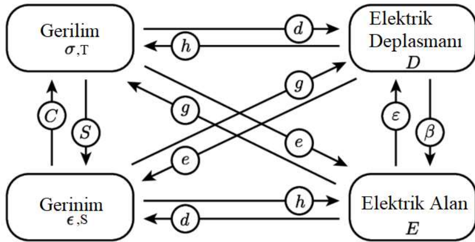
Şekil 2.12. Elastik, piezoelektrik ve dielektrik ilişkiler (Tholander, 2014'ten değiştirilerek alınmıştır)
