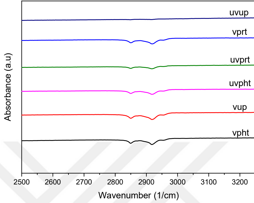
Şekil 4.10. 2500-3200 cm -1 dalga sayısı aralığında transmittans FTIR sonuçları
