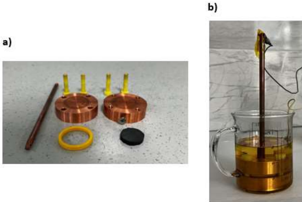
Şekil 3.4. Polarizasyon aparatı a) Aparatın parçaları b) Aparatın montajlı hali
