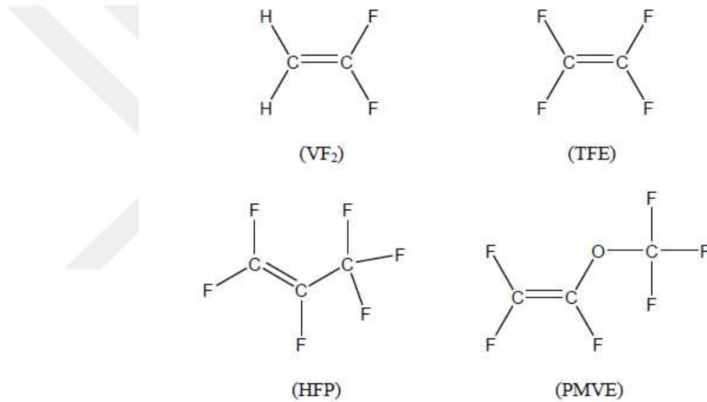
Şekil 2.27. FKM tiplerinin içerdiği bazı monomerler (Hiltz, 2009)
