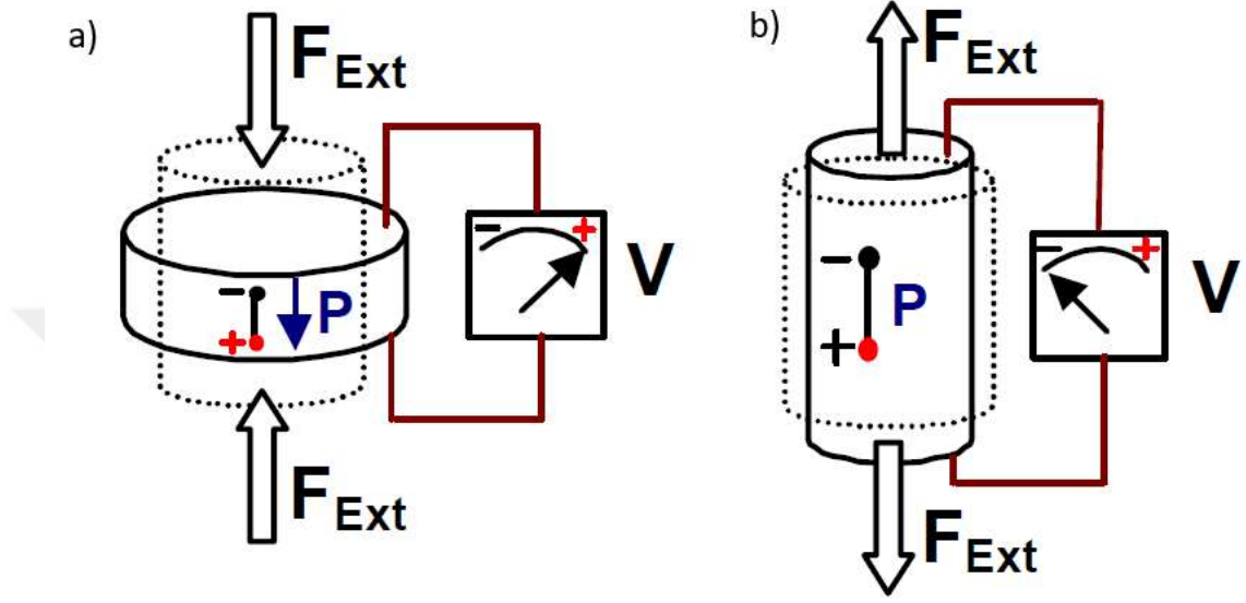
Şekil 2.4. Direkt piezoelektrik etkinin şematik gösterimi a) Basma yönünde kuvvet uygulandığında b) çekem yönünde kuvvet uygulandığında (Carazo, 2002)
