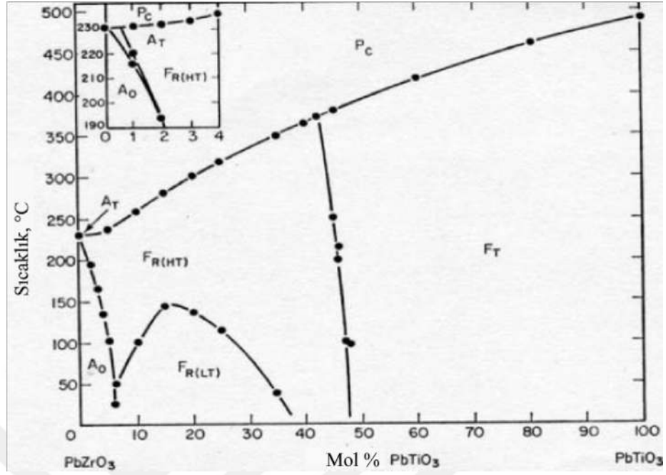
Şekil 2.18. PZT faz diyagramı (Panda ve Sahoo, 2015)
