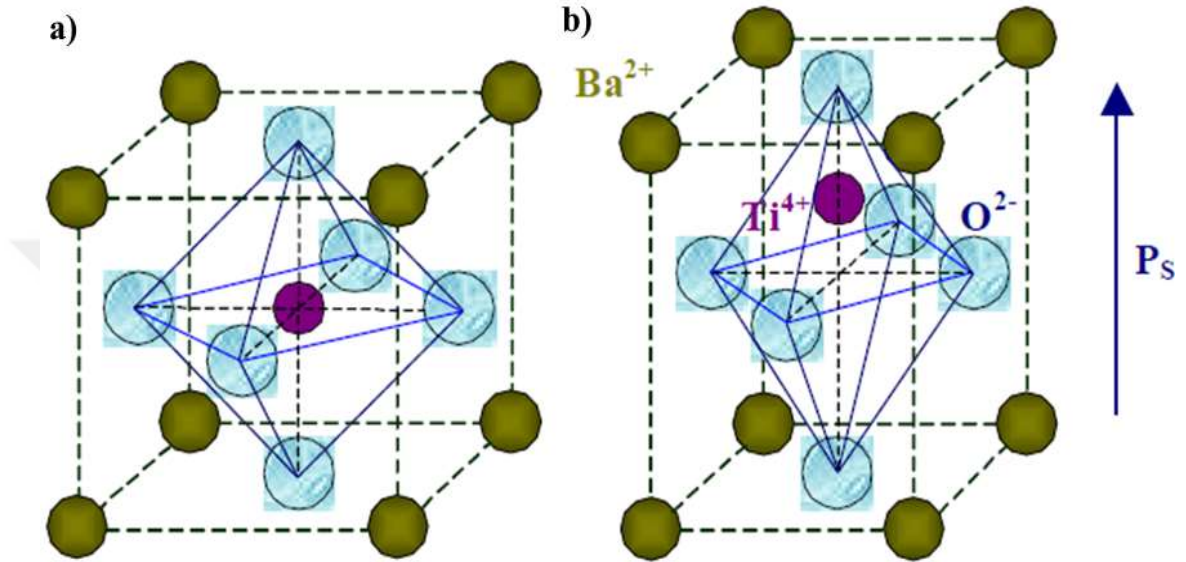
Şekil 2.8. Baryum titanatın kristal yapısının küri sıcaklığı ile değişimi a) Küri sıcaklığının üzerinde b) Küri sıcaklığının altında (Carazo, 2002)
