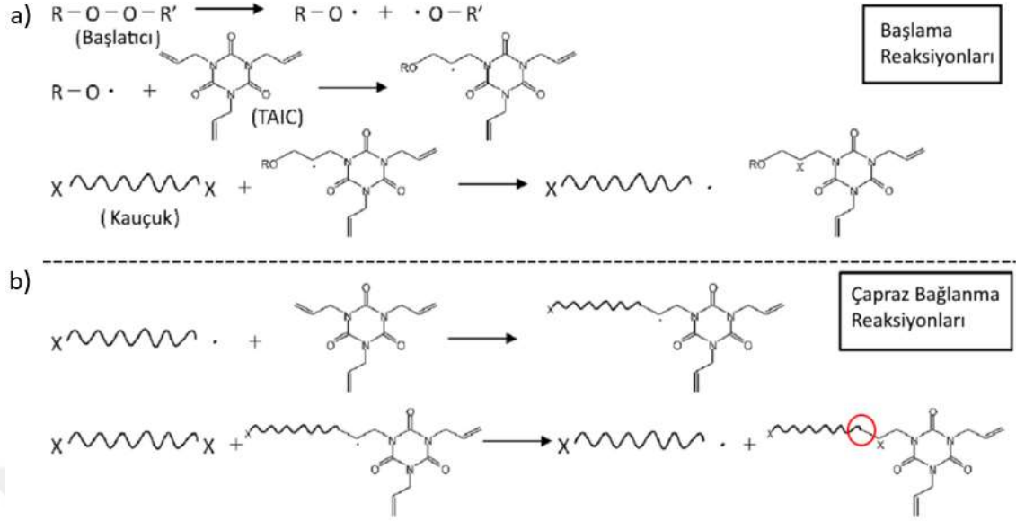
Şekil 4.9. TAIC ve peroksit pişirici istemli FKM'nin vulkanizasyon reaksiyonları a) Başlama reaksiyonları b) Çapraz bağlanma reaksiyonları (Muroga ve diğerleri, 2021'den değiştirilerek alınmıştır)
