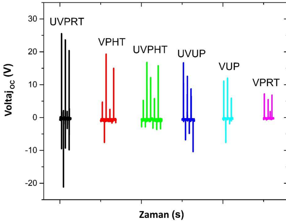
Şekil 4.5. Açık devre voltajı ölçüm sonuçlarının karşılaştırılması
