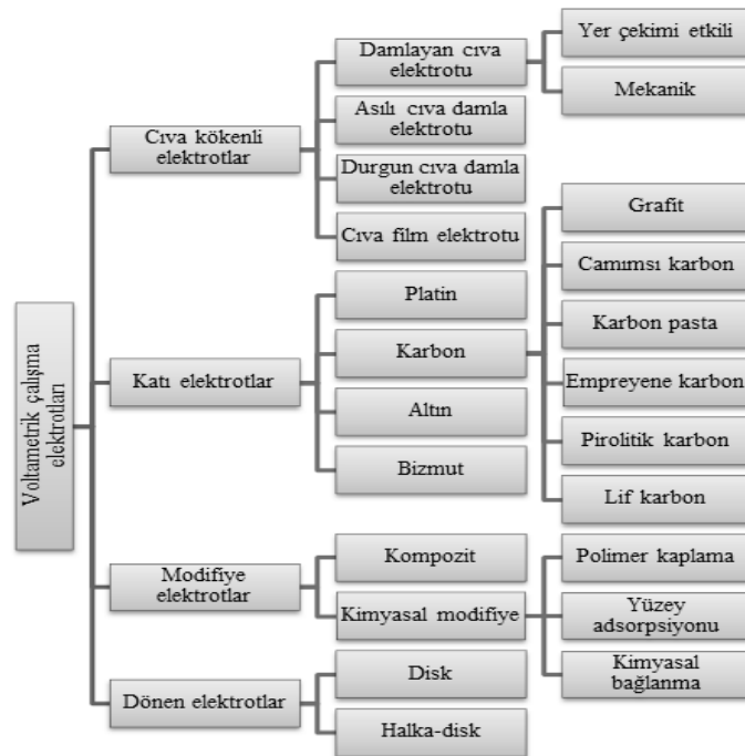
Şekil 2.12. Voltametrde kullanılan çalışma elektrotları
