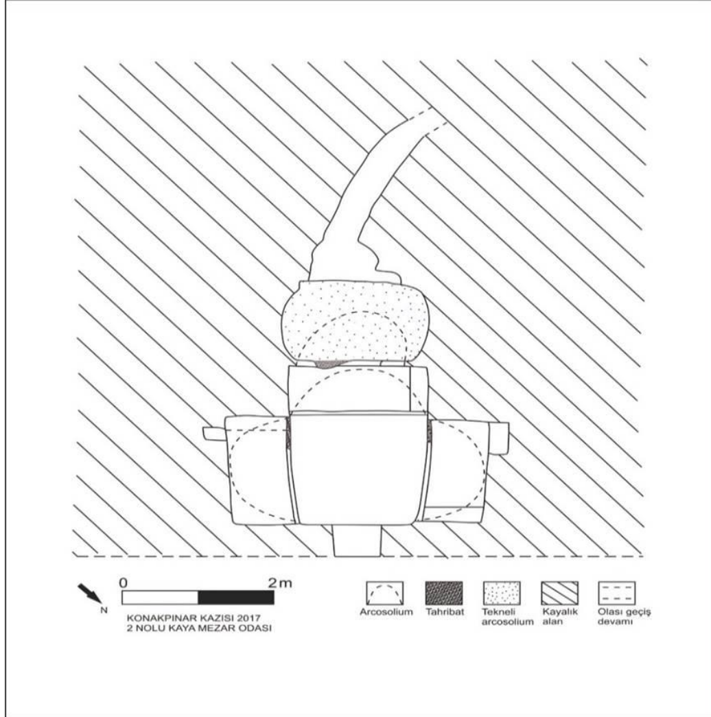
Şekil 3.10: 2 No.lu kaya mezarı planı (Kemal ATAĞ tarafından çizilmiştir.)
