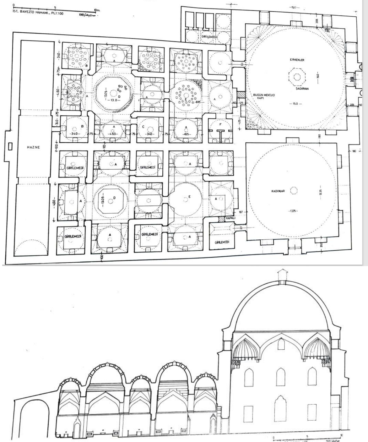
Şekil 1.7. Hamam Planı (Kaynak: Yüksel, İ. A. (1983). Osmanlı Mimârisinde II. Bâyezid Yavuz Selim Devri, V., s. 212-213)
