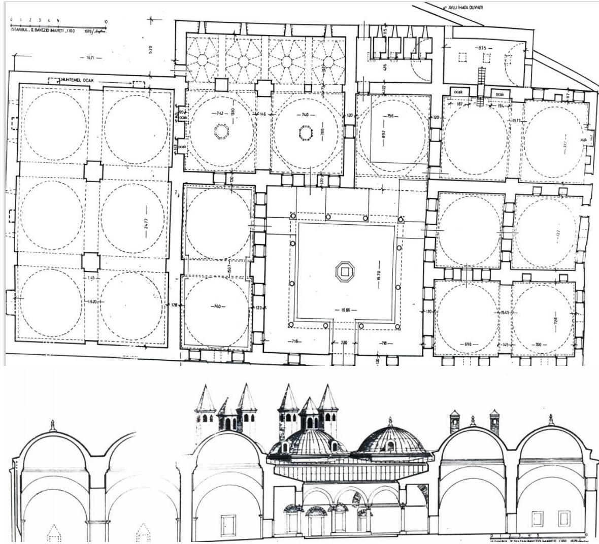
Şekil 1.5. İmâret Planı (Kaynak: Yüksel, İ. A. (1983). Osmanlı Mimârisinde II. Bâyezid Yavuz Selim Devri, V., s. 208-209)
