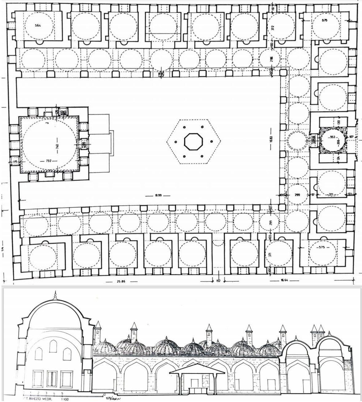
Şekil 1.4. Medrese Planı (Kaynak: Yüksel, İ. A. (1983). Osmanlı Mimârisinde II. Bâyezid Yavuz Selim Devri, V., s. 205)
