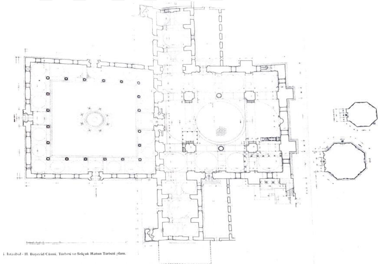
Şekil 1.2. II. Bâyezid Camii, Türbesi ve Selçuk Sultan Türbesi planı (Kaynak: Yüksel, İ. A. (1983). Osmanlı Mimârisinde II. Bâyezid Yavuz Selim Devri, V., s. 188-189)
