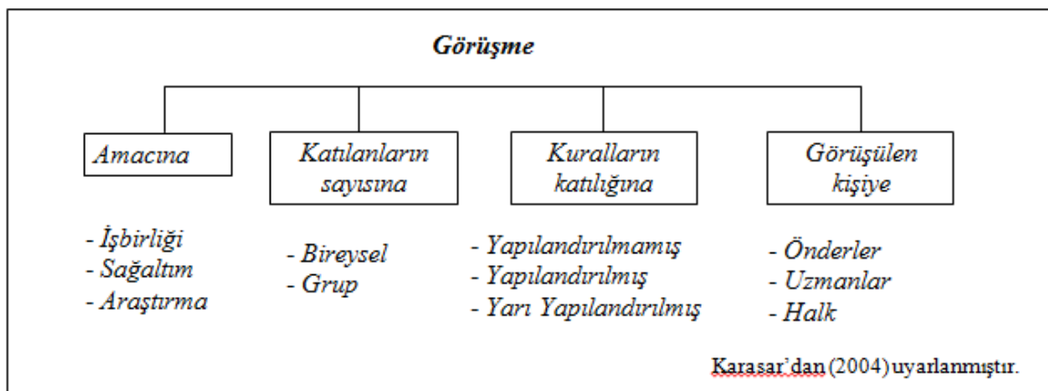
Şekil 3.1 Görüşme Türleri
