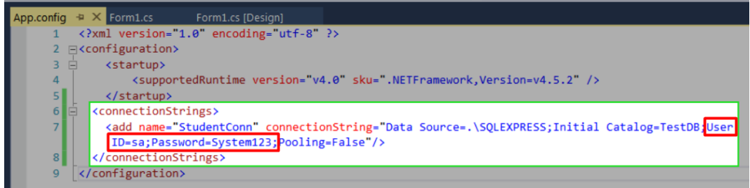
Şekil 3.19. Bir Asp.NET uygulamasında veritabanı bilgilerinin yapılandırma dosyasında düz metin olarak tutulması
