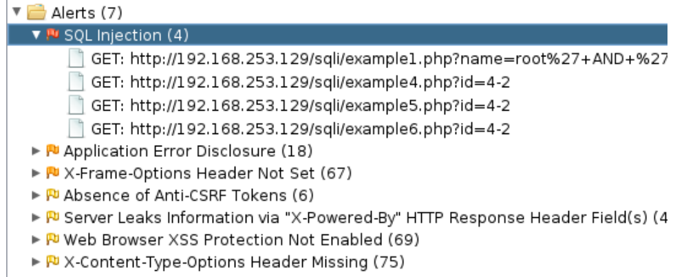
Şekil 4.7. SQL Injection ile kullanıcı bilgilerinin elde edilmesi
