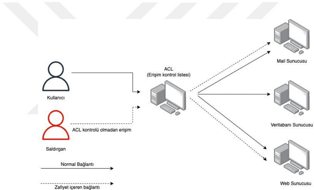
Şekil 2.6. Kırık kimlik doğrulama
