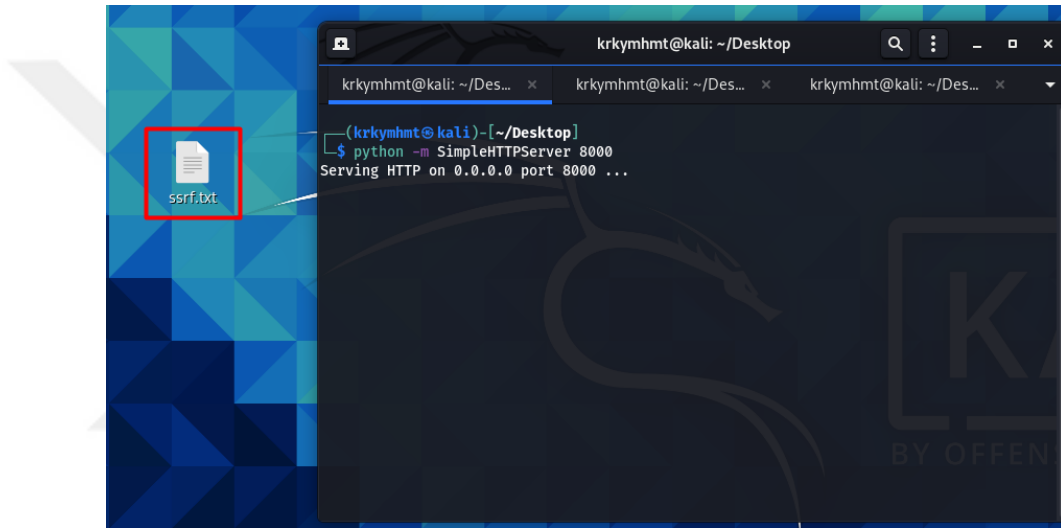
Şekil 3.50. Kali Linux üzerinde Python kullanılarak sunucu ve ssrf.txt dosyasının oluşturulması
