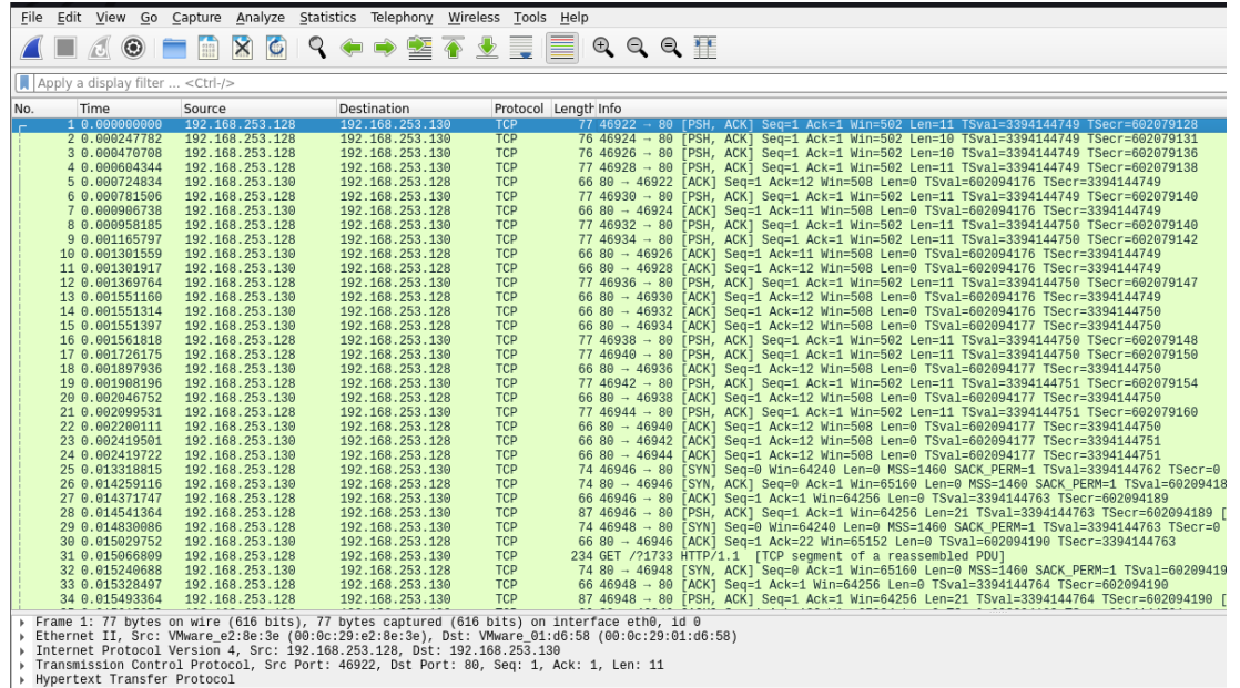
Şekil 4.18. Wireshark ile DDoS saldırı paketlerinin incelenmesi
