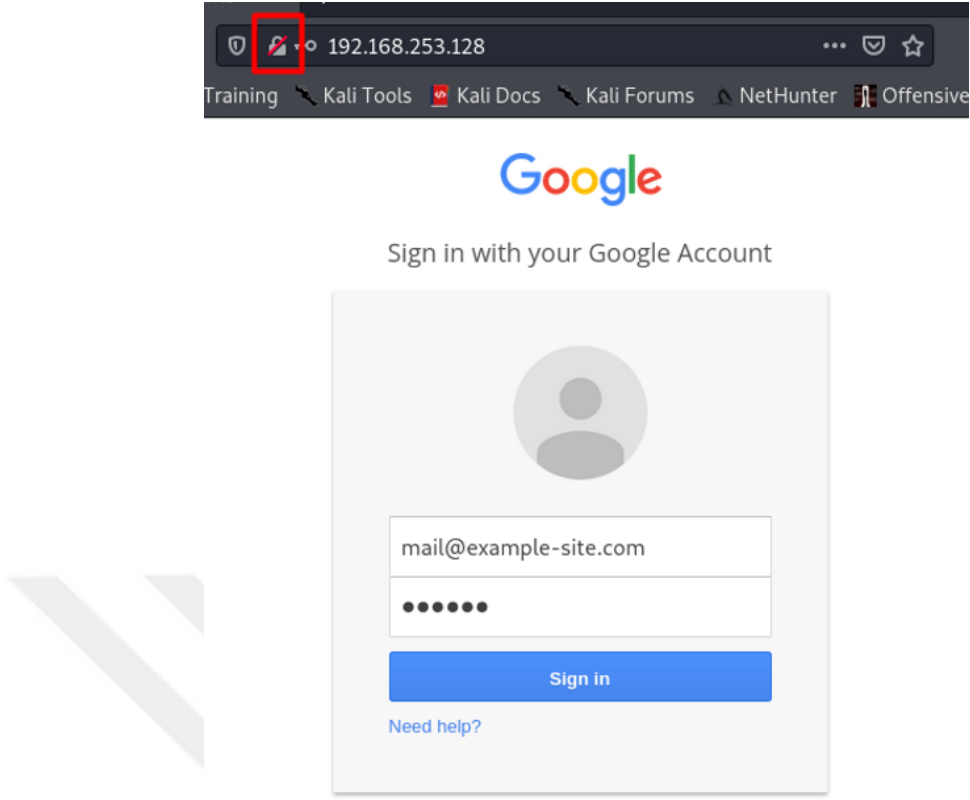
Şekil 3.35. Oltalama için kullanılan örnek bir giriş sayfası
