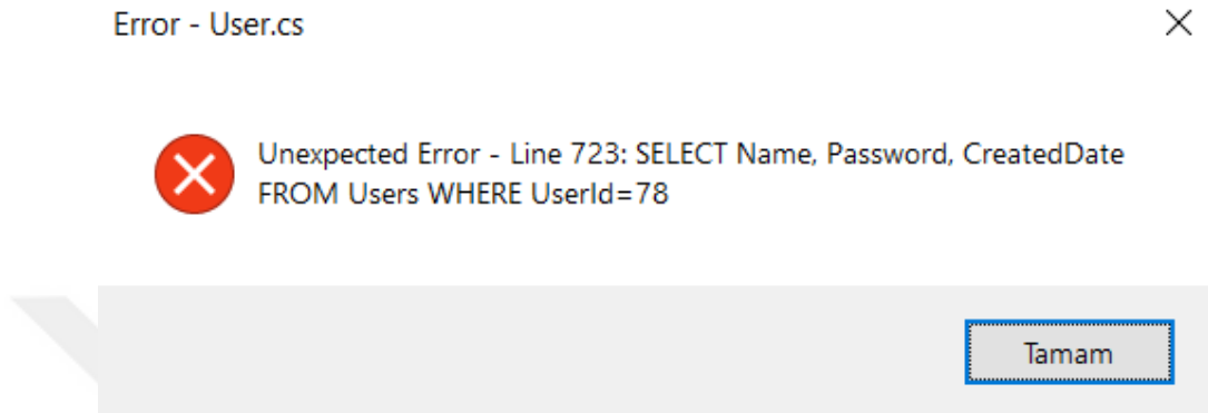
Şekil 3.22. Kritik bilgi barındıran bir hata mesajı örneği
