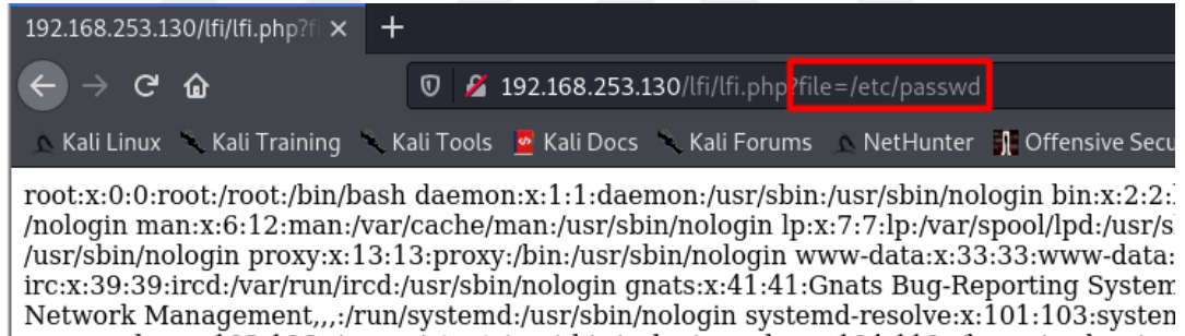
Şekil 3.42. URL üzerinden sunucuda bulunan diğer dosyalara erişilmesi
