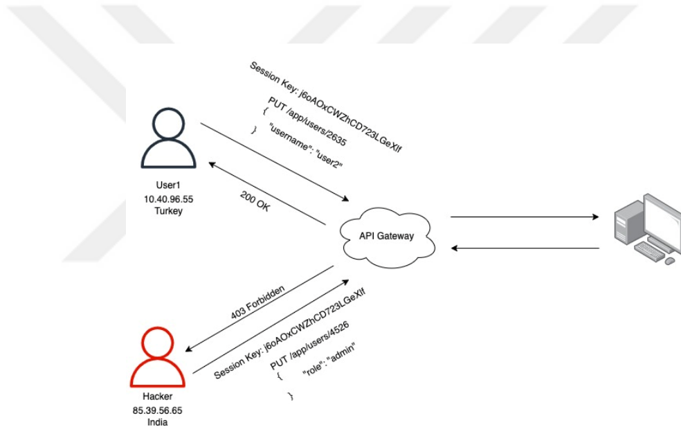
Şekil 2.7. Sunucu tarafı istek sahteciliği
