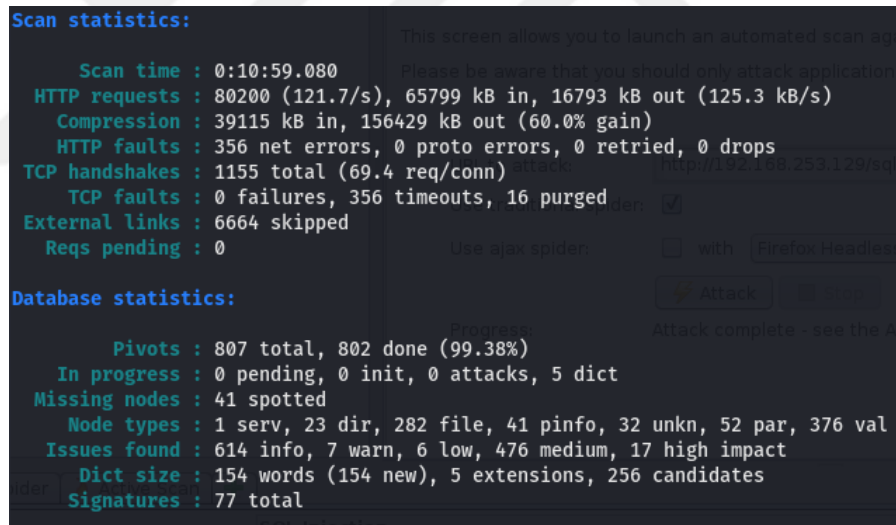
Şekil 4.8. Skipfish tarama sonucu
