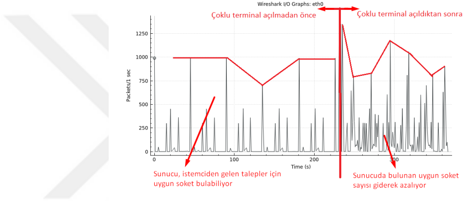
Şekil 4.19. DDoS saldırısının birden fazla terminal üzerinden yapılması durumunda sunucuya giden network trafiği
