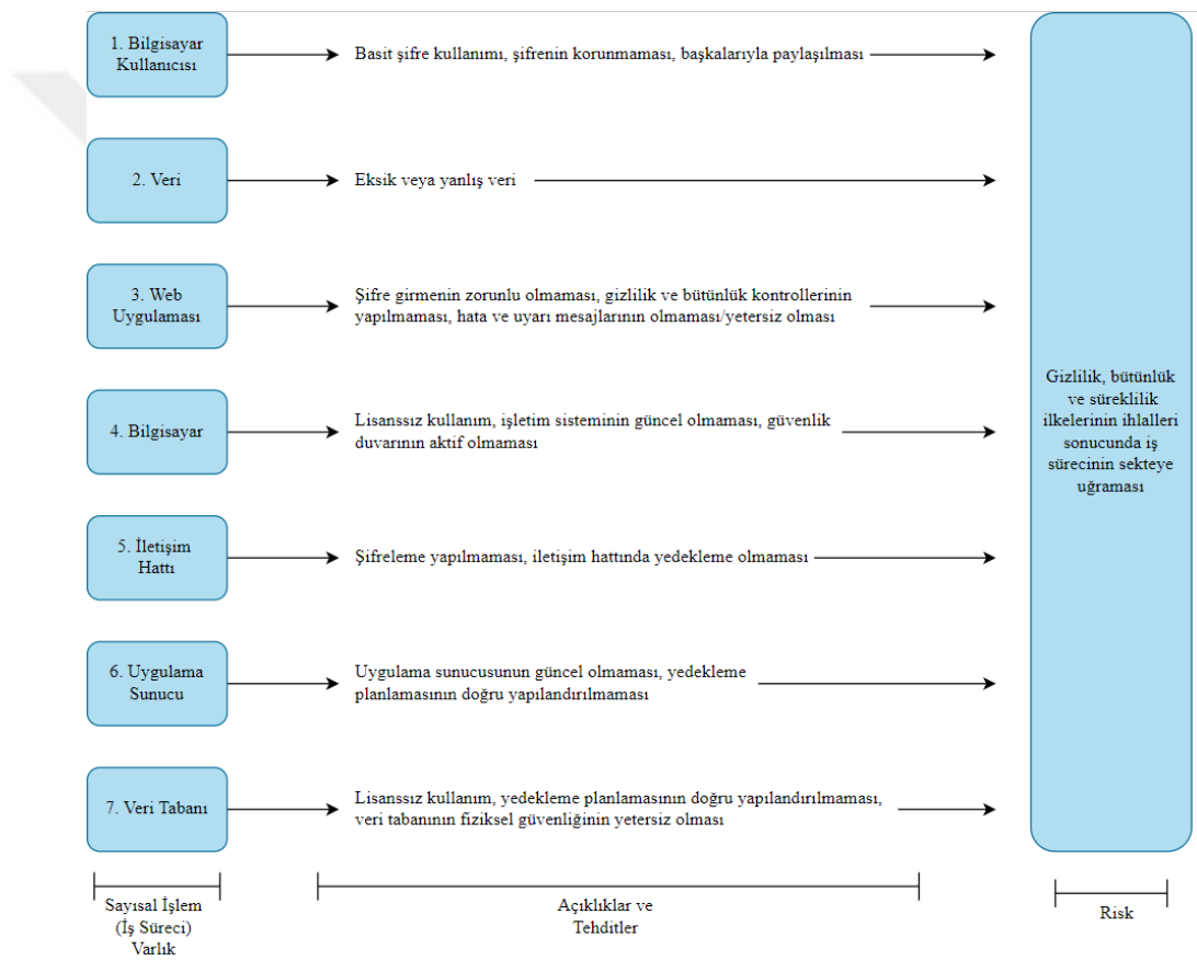
Şekil 2.3. Örnek bir süreç modeli ve modelin kullanılarak risk analizi yapılması [15].
