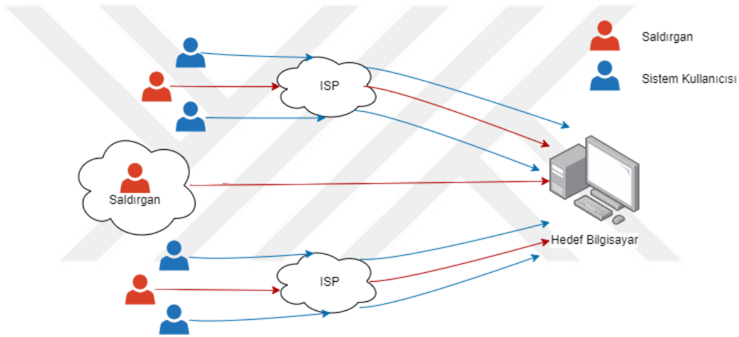
Şekil 4.14. DDoS Saldırı Şeması
