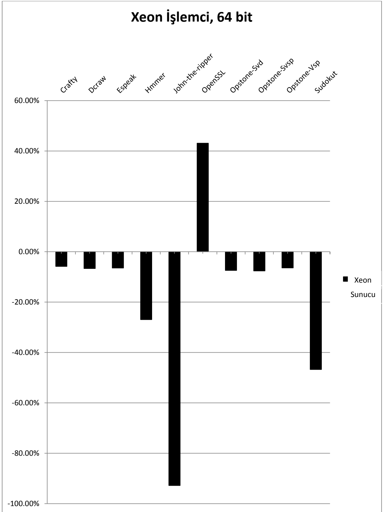
Şekil 8. İleri Düzey Özel Bulutun, Halk Bulut Performansına Göre Yüzdelik Değerleri
