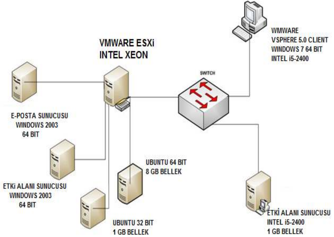
Şekil 5. Xeon İşlemcili Sunucu Test Topolojisi
