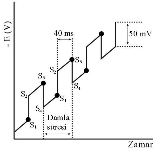
Şekil 2.13. Diferansiyel puls polarografisinde uyarma sinyalleri
