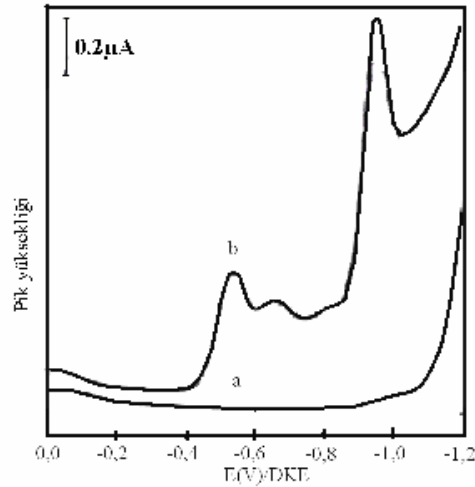
Şekil 4.1. Kuşburnu numunesinin pH=2 HCl ortamındaki polarogramı (a) 10 mL pH= 2 HCl çözeltisi; (b) a + 0,2 mL numune
