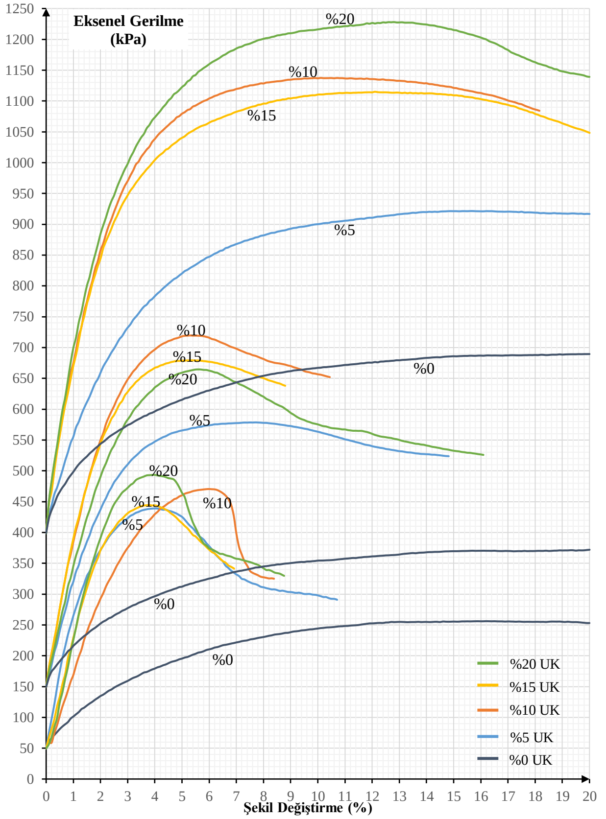
Şekil 4.5: 32 gün kürde bekletilmiş karışımların Eksenel gerilme - Şekil değişirme eğrileri.
