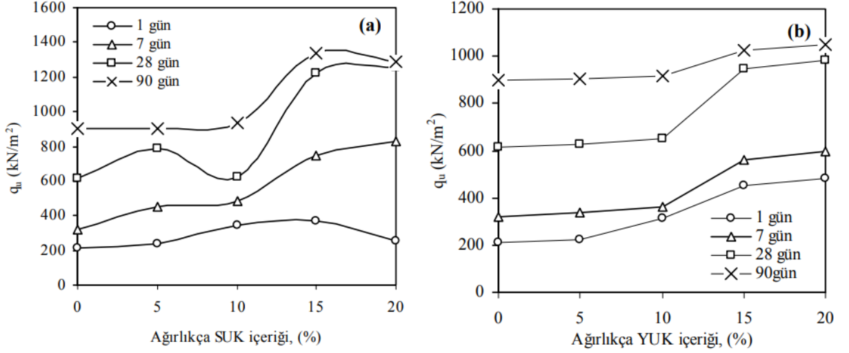
Şekil 1.2: Uçucu kül içeriği ile serbest basınç dayanımı değişimi (a: Soma, b: Yatağan) (İnan vd., 2005).
