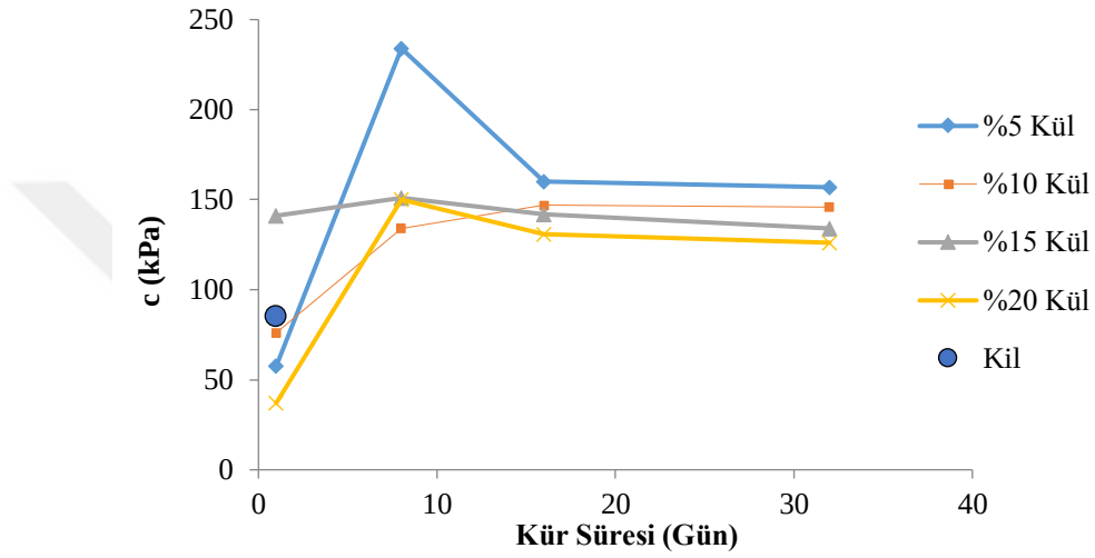
Şekil 4.3: Kohezyon değerlerinde gözlenen değişimler.
