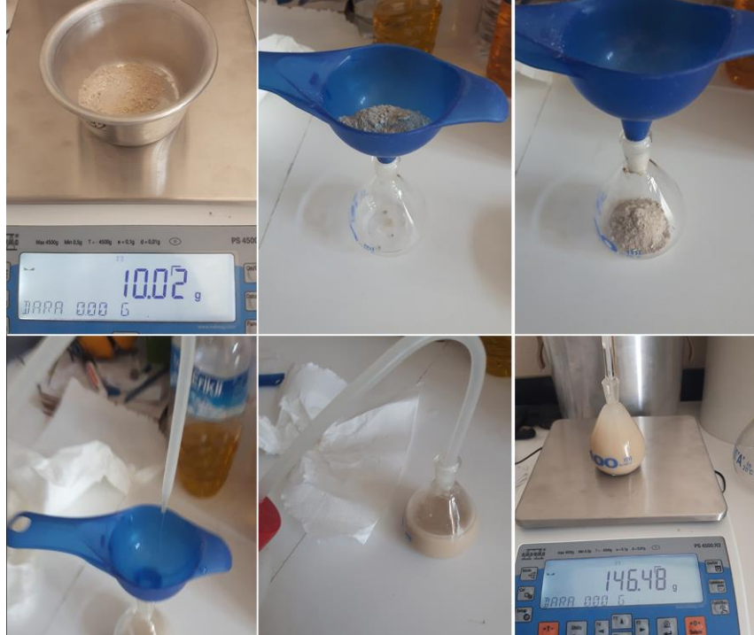
Şekil 3.6: Piknometre deney görüntüleri.
