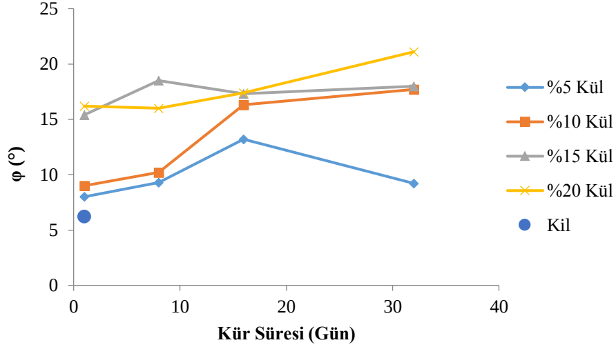
Şekil 4.4: Kayma direnci açısında gözlenen değişimler.
