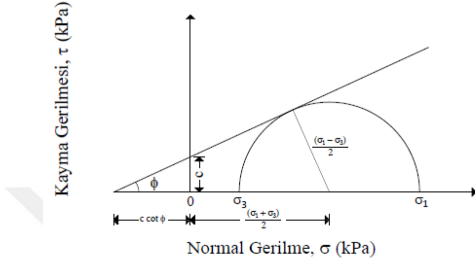
Şekil 2.7: Aşırı konsolide kil zeminde kırılma zarfına ait tipik ilişkiler (Das, 1983).
