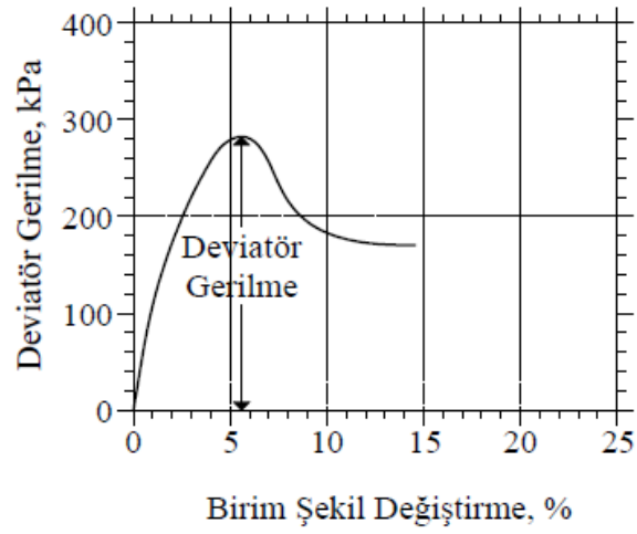
Şekil 2.2: Doruk değerın küçük birim deformasyon değerlerinde görülmesi durumuna ait örnek grafik.
