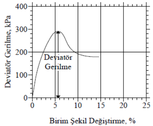
Şekil 2.3: Maksimum deviator gerilmeye ulaşmadan gerilme oranının pik yaptığı duruma ait örnek grafik.
