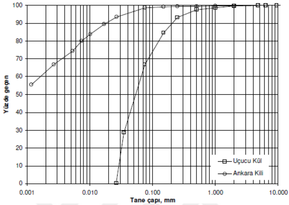
Şekil 1.4: Ankara Çukurambar killi zemin numunesi ve Çayırhan Termik Santrali uçucu külüne ait dane boyutu dağılım eğrileri (Yılmaz ve Sevensan, 2010).
