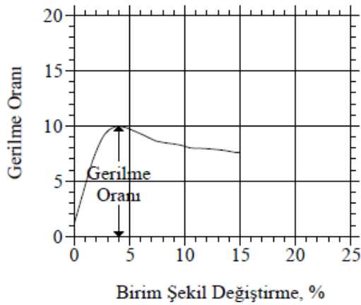
Şekil 2.3: Maksimum deviator gerilmeye ulaşmadan gerilme oranının pik yaptığı duruma ait örnek grafik.
