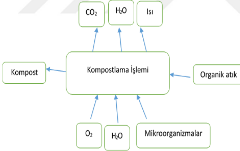
Şekil 1.3. Kompostlama işlemi
