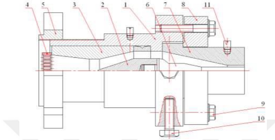
Şekil 2.29. Boru kalıbı (Milli Eğitim Bakanlığı, 2012)
