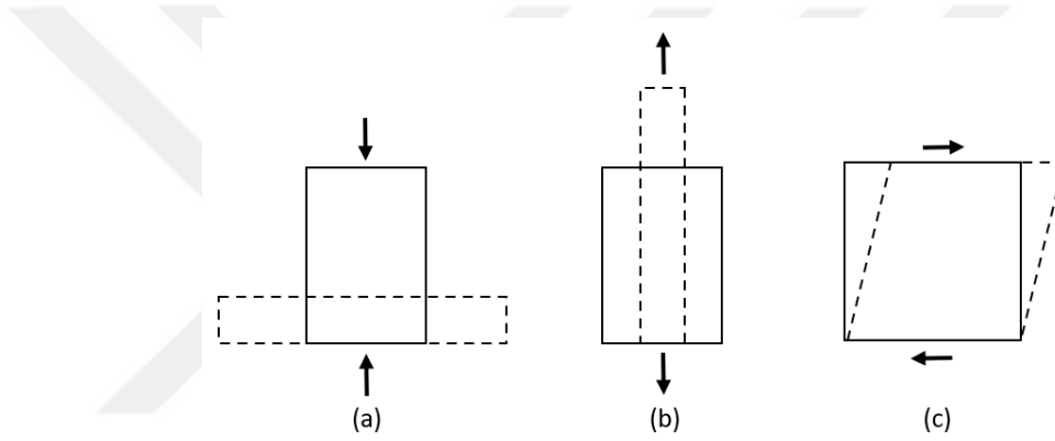
Şekil 2.1. (a) Basma (b) Çekme (c) Kayma (Çakır, 2011)
