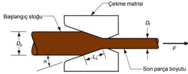
Şekil 2.5. Tel ve çubuk çekme yöntemi (Demirkol, 2010)
