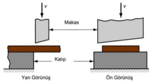
Şekil 2.6. Giyotin kesme (Kayaoğlu, 2019)
