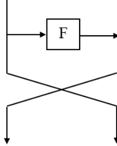
Şekil 3.3. Feistel yapı.
