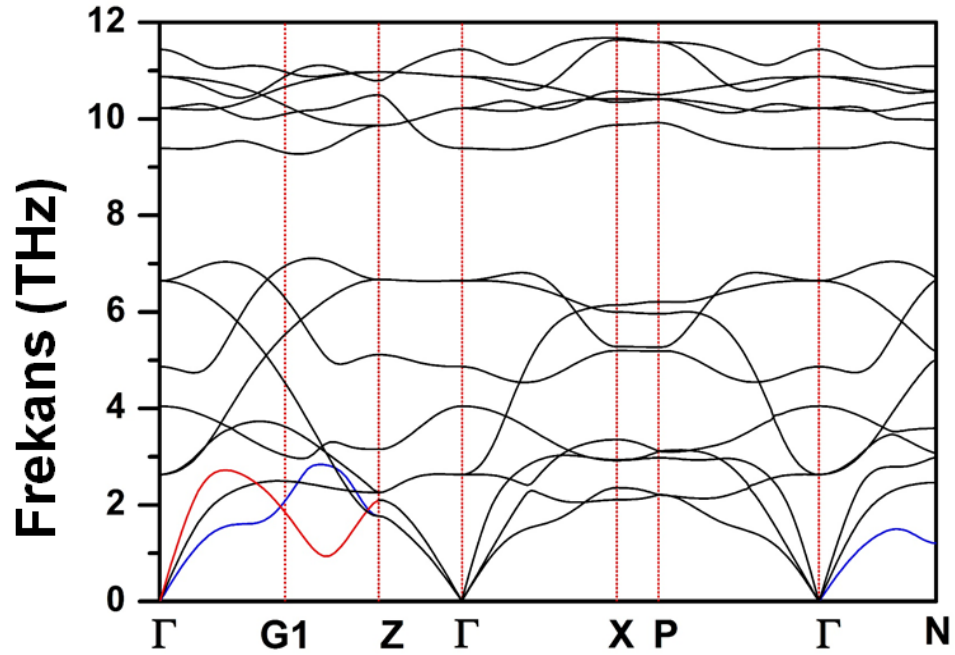
Şekil 5.5. Titreşim modlarının farklı yüksek simetri doğrultularında dağılımlarının gösterilmesi.
