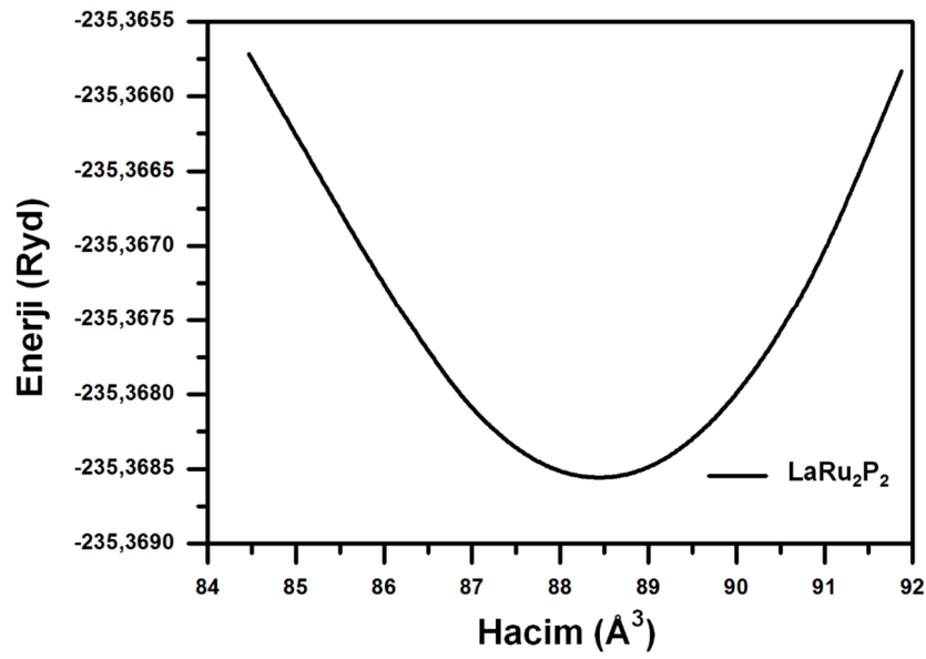
Şekil 5.2. \text{LaRu}_2\text{P}_2 malzemesinin hesaplamalar sonucu elde edilen enerji-hacim grafiği.
