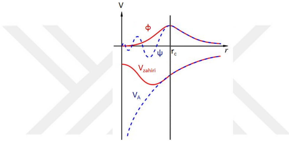
Şekil 3.3. Zahiri potansiyel ve zahiri dalga fonksiyonunun gösterimi.
