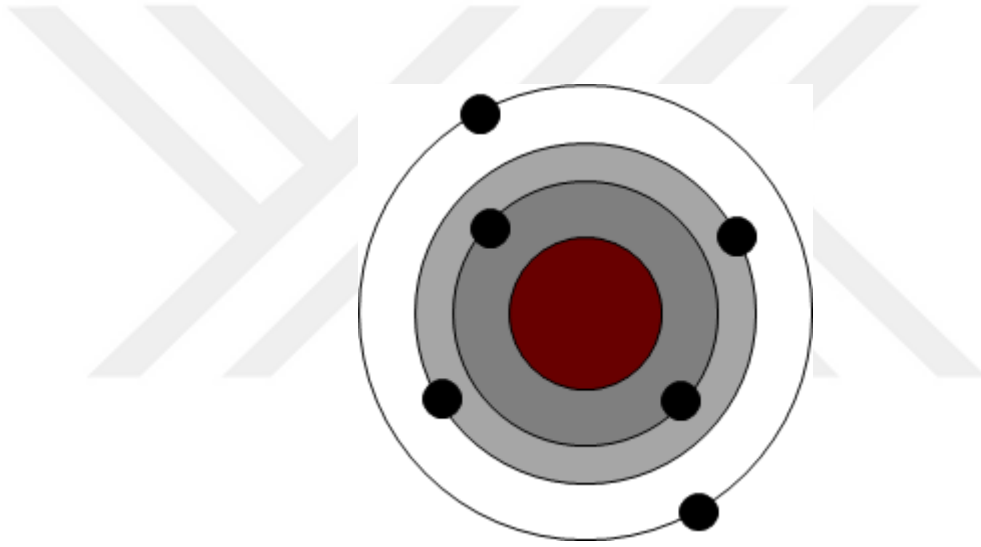
Şekil 3.2. Çekirdek, kor elektronları ve değerlik elektronlarından oluşmuş bir atom. Taralı bölge kor bölgesini göstermektedir.
