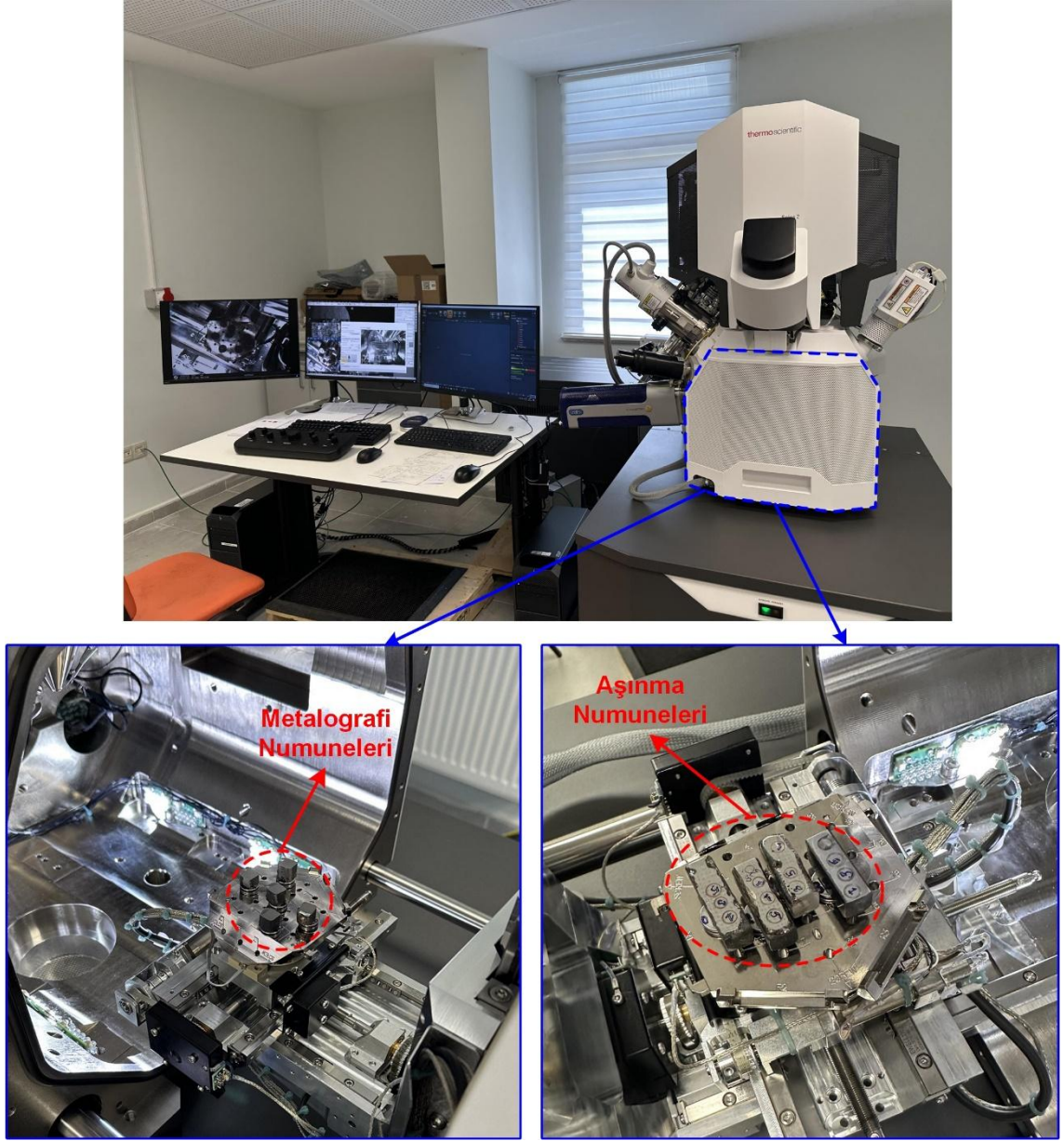
Şekil 3.11. Taramalı elektron mikroskobu
