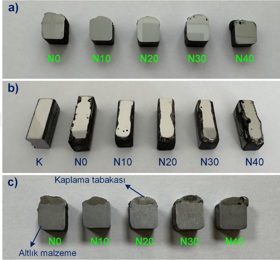
řekil 3.9. Metalografi numuneleri (a), ařınma numuneleri (b) ve dađlama sonrası metalografi numuneleri (c)
