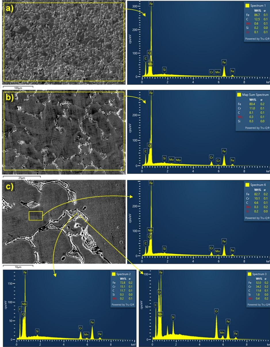
Şekil 4.13. N0 numunesinin EDS analizi; a) altlık malzeme, b) kaplama tabakası, c) kaplama matrisi ve karbür çökeltileri
