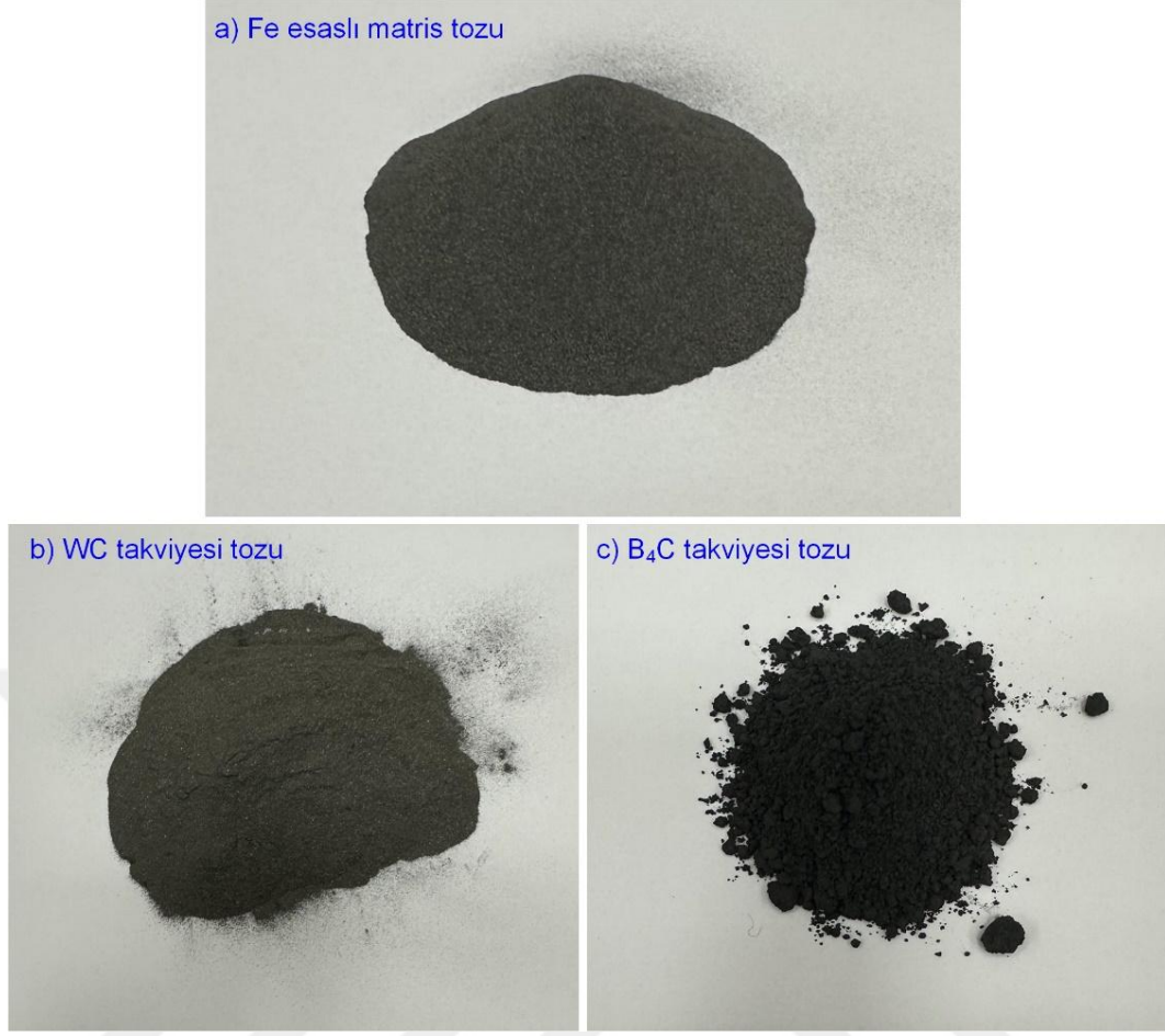
Şekil 3.2. Kaplama tozları
