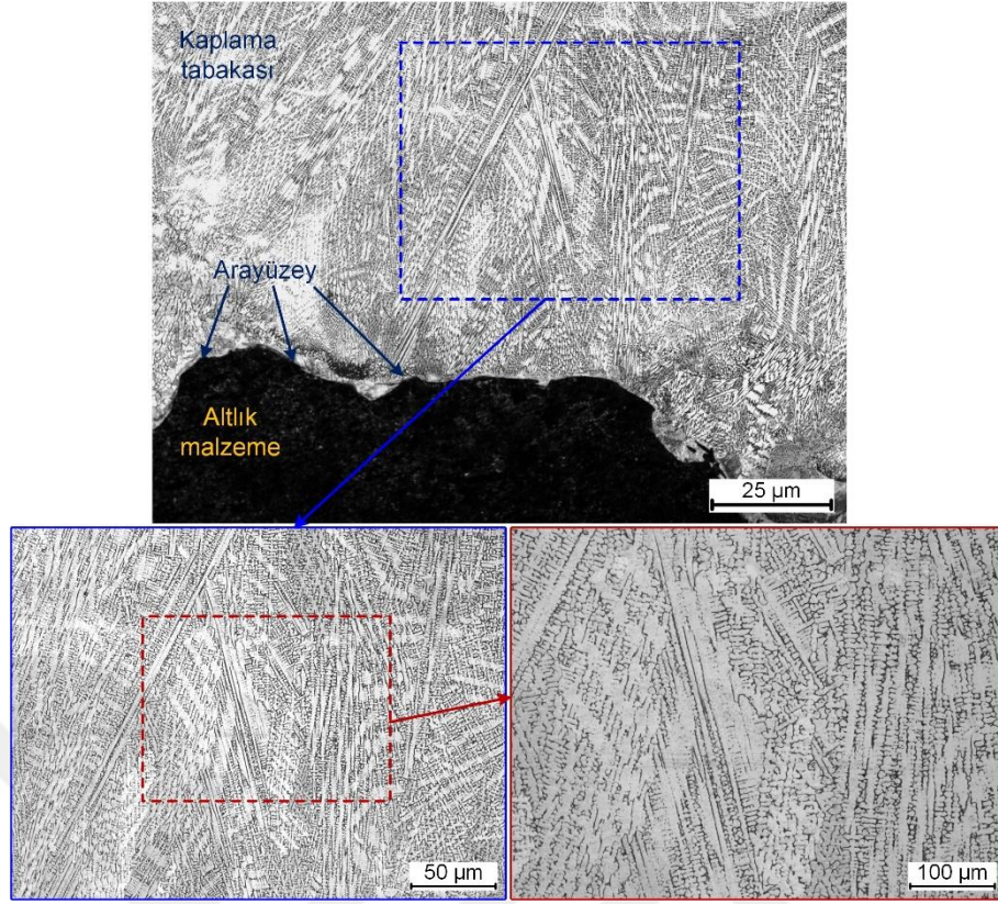
Şekil 4.1. N0 numunesinin OM görüntüleri
