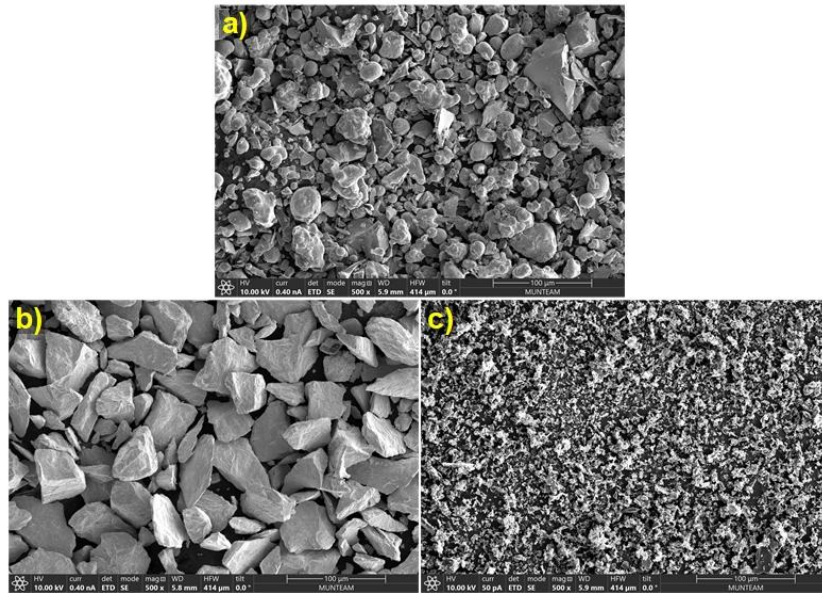
Şekil 4.6. Kaplama tozlarının SEM görüntüleri; a) matris tozu, b) WC tozu, c) B 4 C tozu
