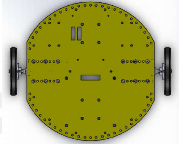
Şekil 5.2. Bu çalışma için tasarlanan sürüş sisteminin çizimi
