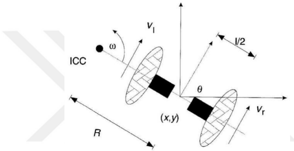
Şekil 5.4. Mobil robot için diferansiyel sürüş kinematik görseli
