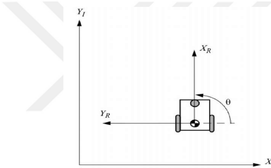
Şekil 3.1. İki boyutlu koordinat düzlemine oturtulmuş olan diferansiyel sürüş sistemine sahip bir robotun pozisyonu
