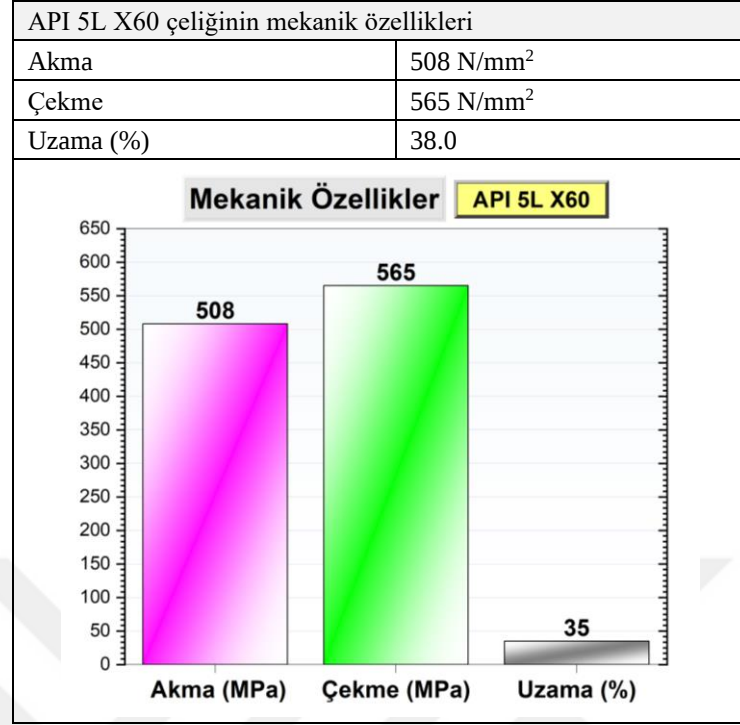
Çizelge 3.2. API 5L X60 çeliğinin mekanik özellikleri
