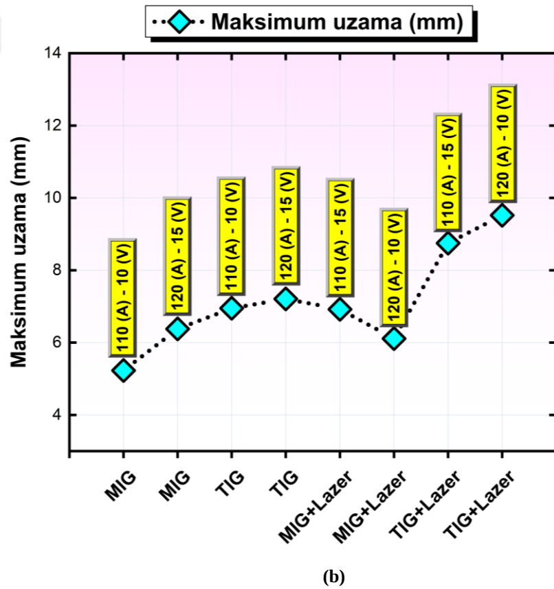
Şekil 4.5. (a) maksimum çekme kuvvetleri ve (b) maksimum uzama değerleri
