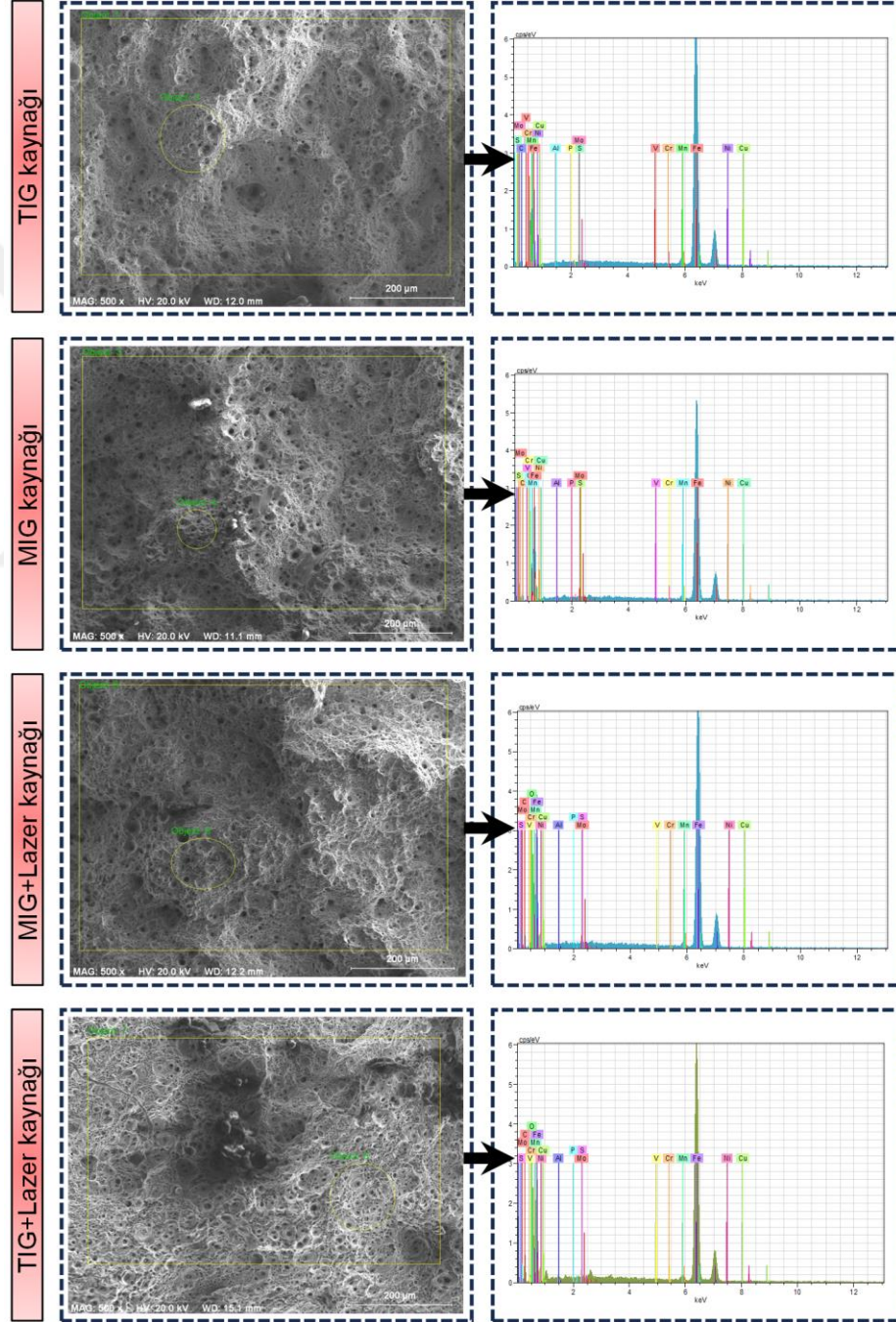
Şekil 4.12. Kırılma yüzeylerinin elementel analizleri
