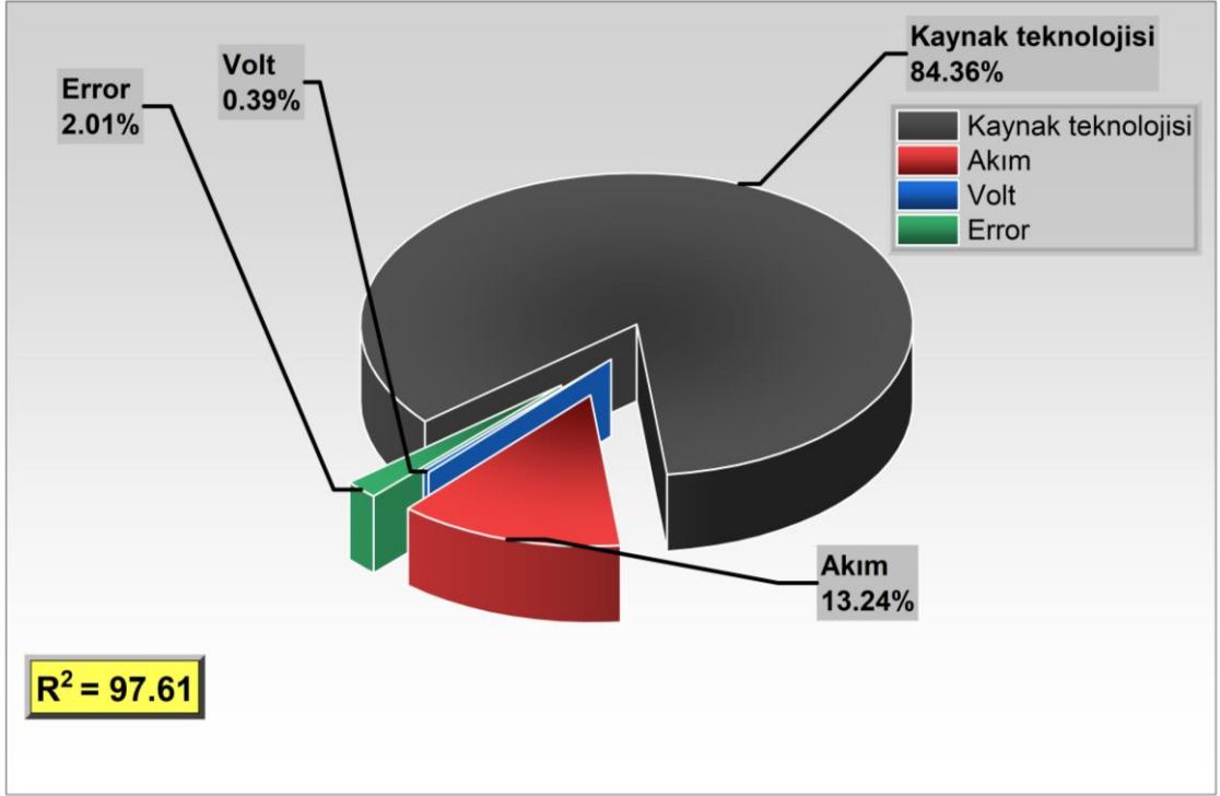
Şekil 4.10. Maksimum çekme kuvvetleri için ANOVA yüzde katkı analizi sonuçları
