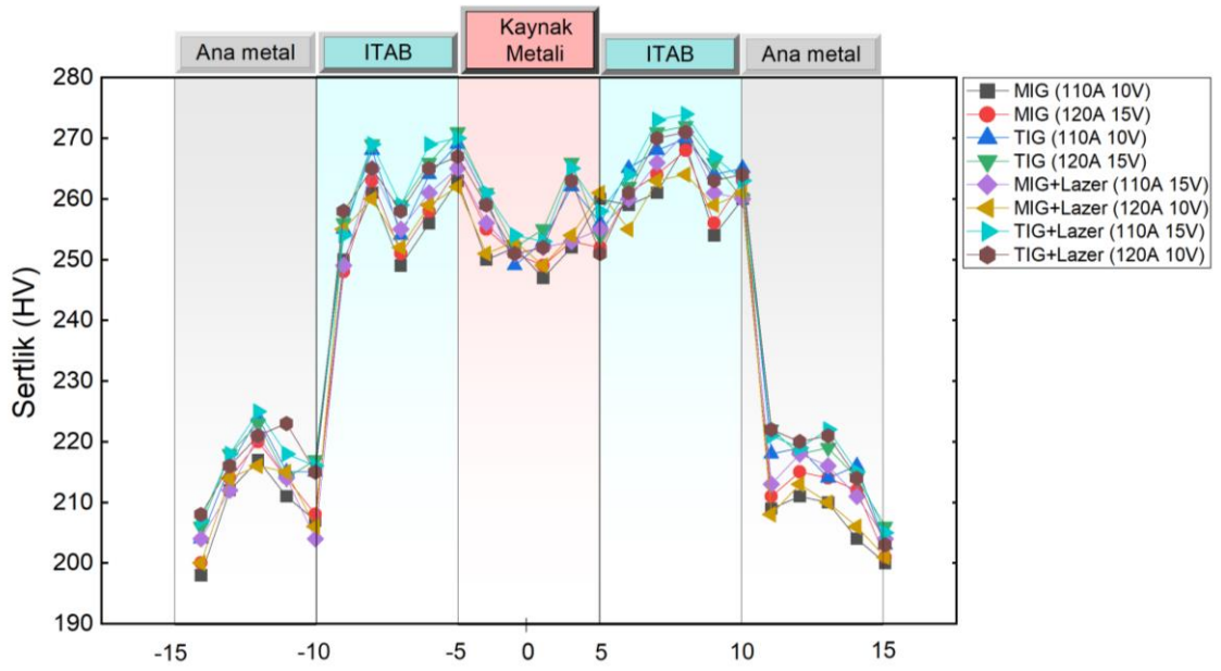
Şekil 4.14. Mikrosertlik ölçümleri
