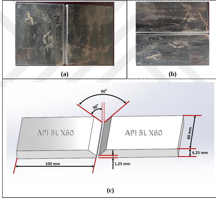
Şekil 3.6. (a ve b) Kaynak ağzı açılan numunelerin görüntüleri ve (c) 3D ölçeklendirilmiş resmi
