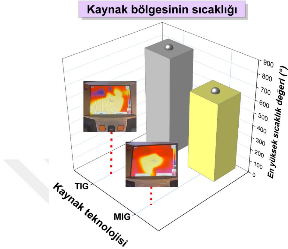
Şekil 4.8. MIG ve TIG kaynağı işlemleri sırasında ölçülen en yüksek sıcaklık değerleri
