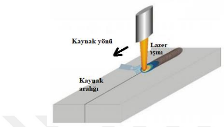
Şekil 1.2. Lazer kaynağı gösterimi (Fetita, 2023)
