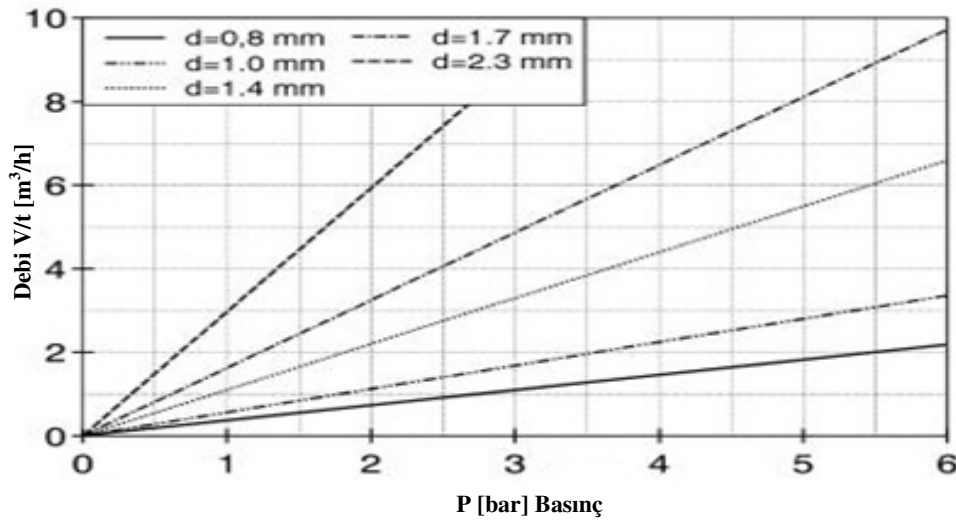
řekil 1.29 6 bar'a kadar oksijenle kesimde kesme gazı tknetimi [d nozul apı]
