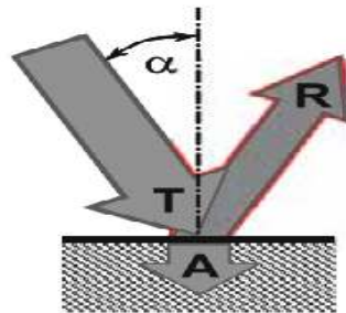
Şekil 1.18 Lazer ışının absorbesi ve yansıması
