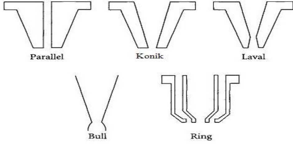
Şekil 1.35 Nozul Çeşitleri
