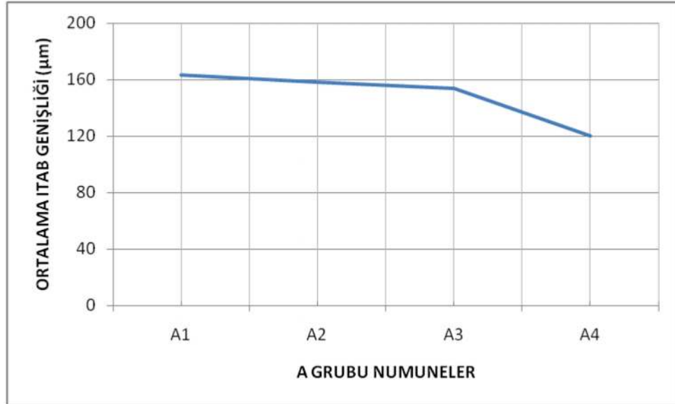
Şekil 3.3 A grubu numuneler; kesme basıncı ve lazer ışını odak noktası sabit, hız kademeli olarak arttırılmış numunelerin hız artışına bağlı olarak ITAB değişimi
