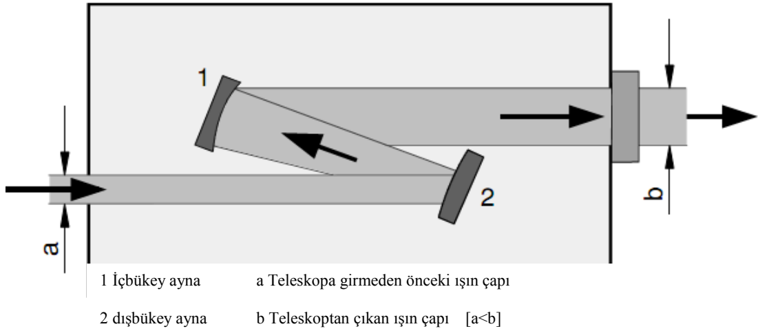
Şekil 1.34 ışın teleskopu içerisinde ışığın genişlemesinin şematik gösterimi
