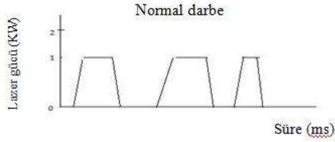
Şekil 1.24 Normal darbeli çalışma
