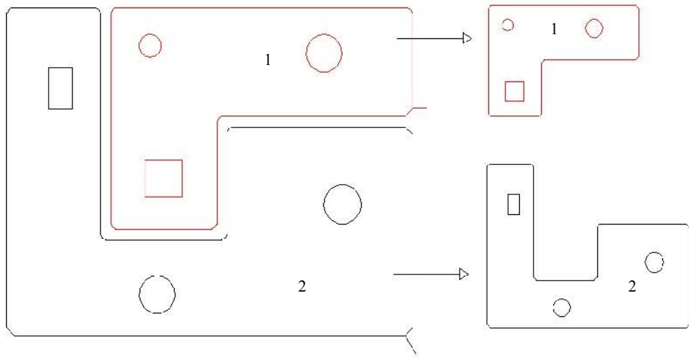
Şekil 5.2 Lazer kesimde parça konumları
