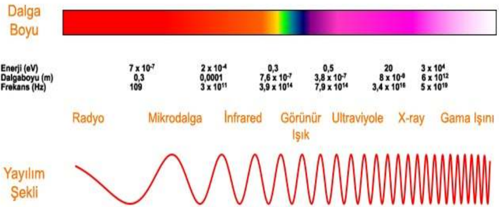
Şekil 1.7 Elektromanyetik spektrum
