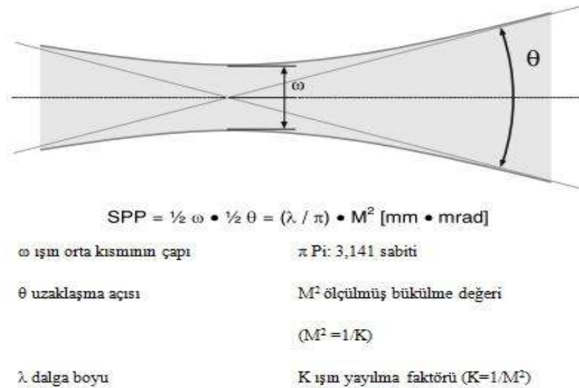
Şekil 1.8 Işın uzaklaşma açısı
