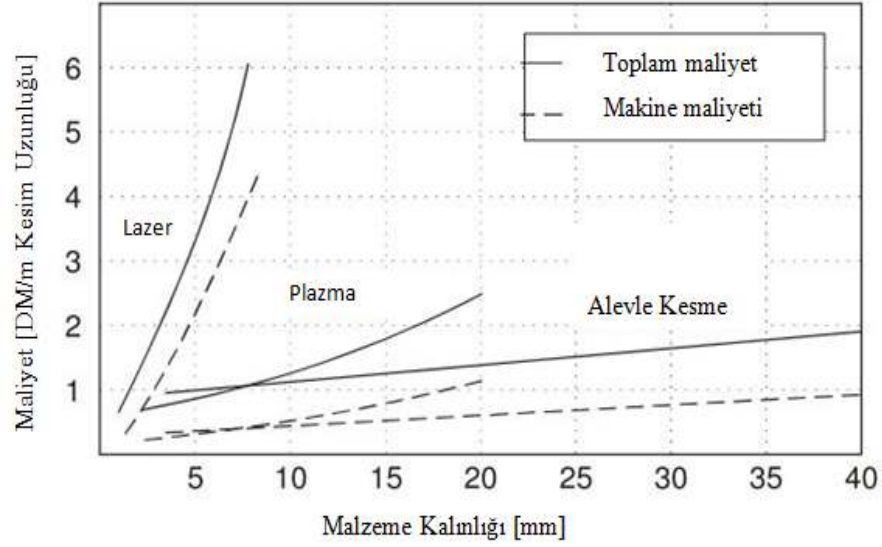
Şekil 5.3 Termik kesme yöntemleri makine maliyeti ve toplam maliyeti
