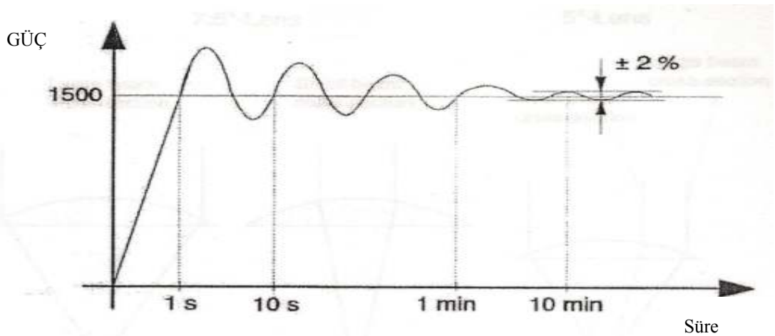
Şekil 1.31 Lazer güç değişimi
