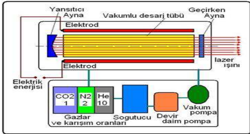
Şekil 1.21 CO 2 lazer sistemi şematik gösterimi
