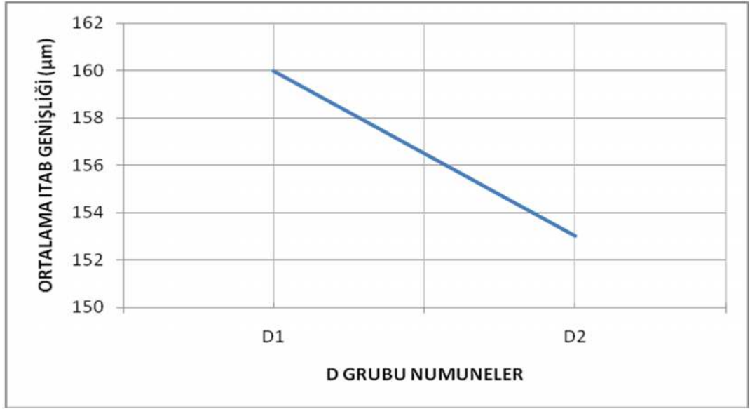
Şekil 3.15 B grubu numuneler; kesme basıncı ve lazer ışını odak noktası sabit, hız kademeli olarak arttırılmış numunelerin hız artışına bağlı olarak ITAB değişimi
