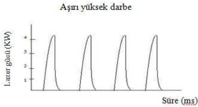
Şekil 1.25 Aşırı yüksek darbeli çalışma
