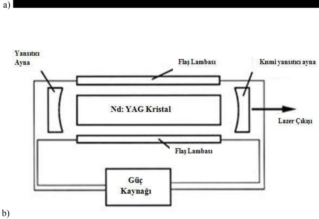
Şekil 1.2 a) Ruby lazer sistemi b) Nd: YAG Lazer sistemi şematik gösterimleri
