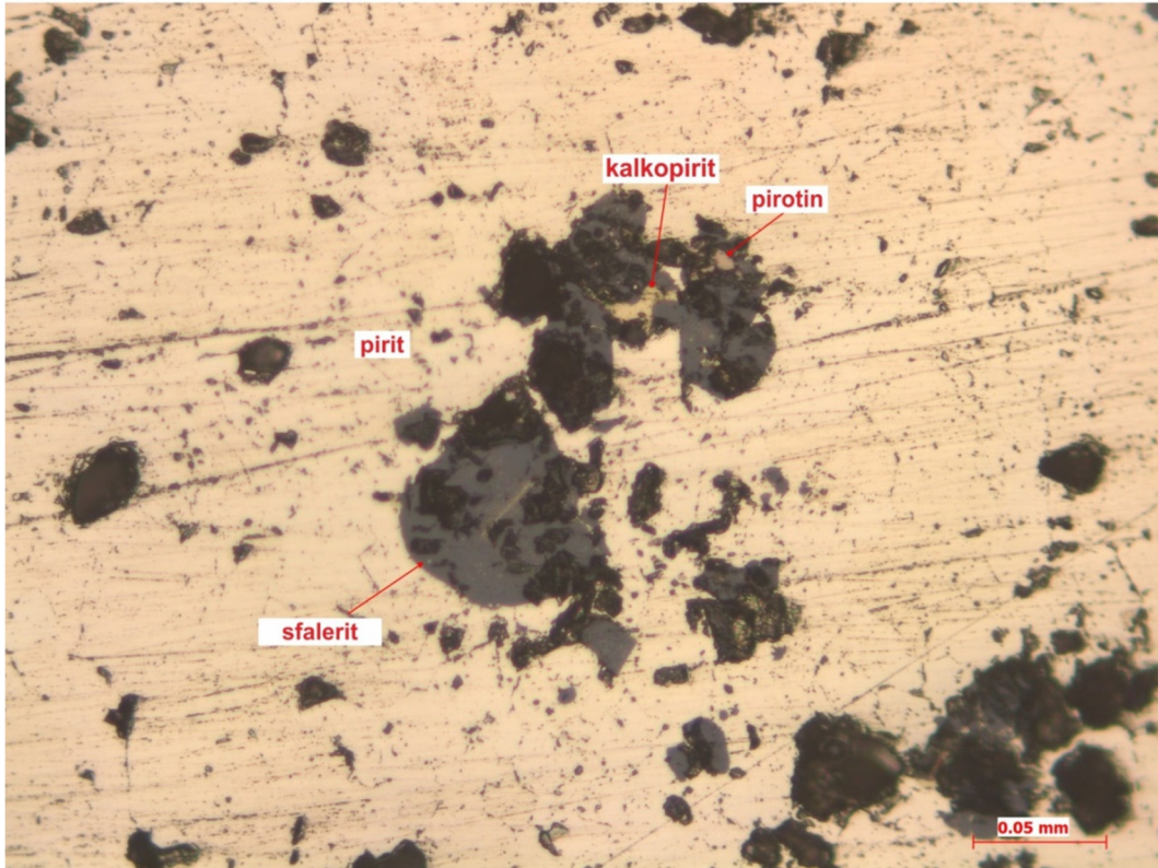
Şekil 2.41. MSC10 örneğinin cevher mikroskopisi incelemesinde gözlenen; masif piritin boşluklarında gelişmiş kalkopiritin kovellin tarafından ornatılması (üstte), masif pirit içerisinde kalkopirit ayrılmaları ve piritin pirotine dönüşümü (altta).
