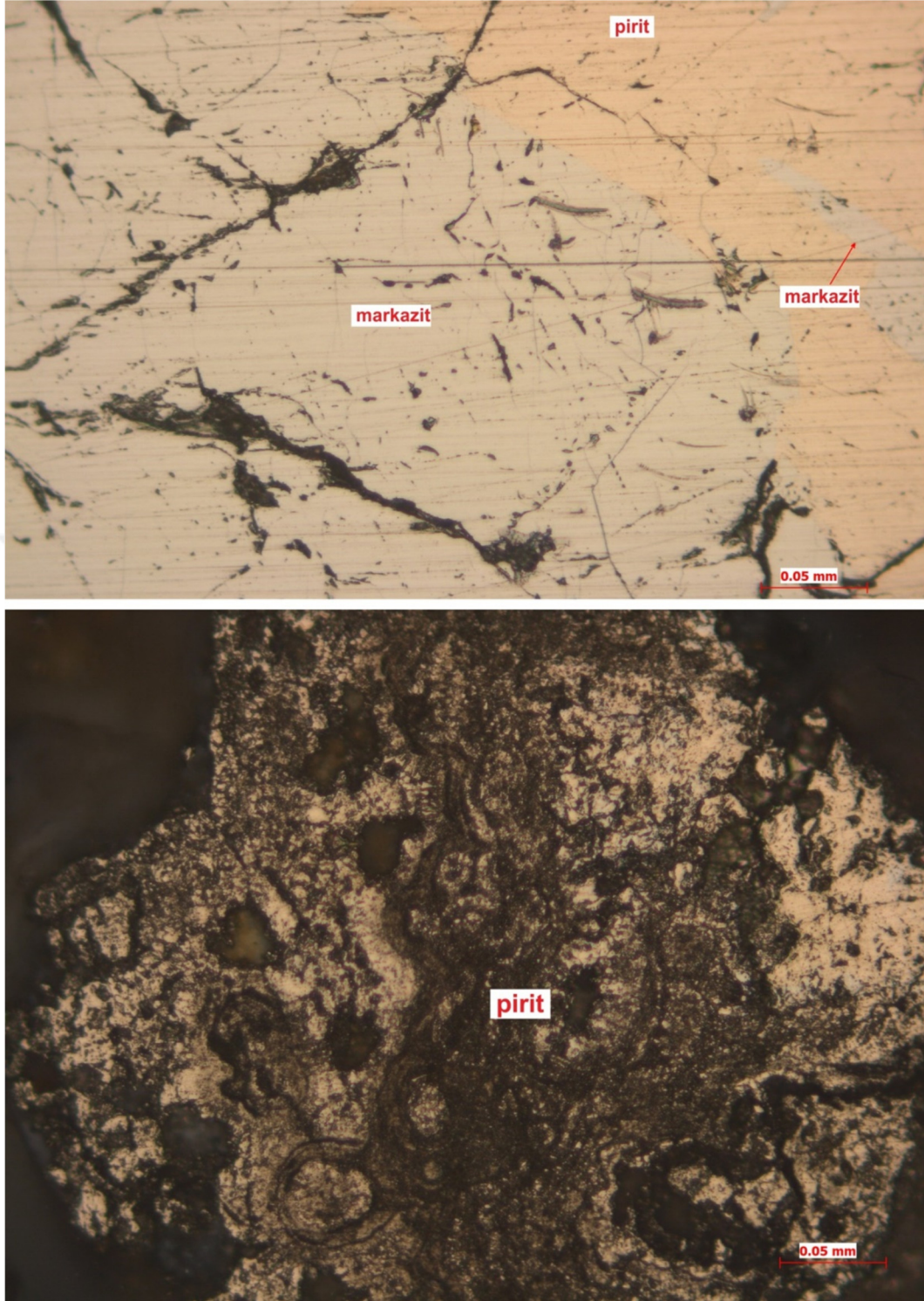
Şekil 2.37. MSC9A örneği cevher mikroskobisi incelemesinde gözlenen; markazitin piriti ornatımı (üstte), kolloform dokulu, yer yer boşluklar içeren pirit (altta).
