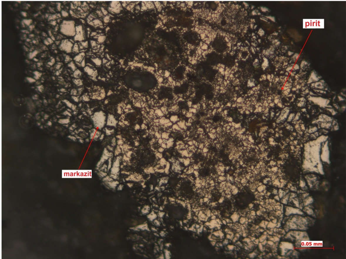
Şekil 2.34. MSC9A örneği cevher mikroskobisi incelemesinde gözlenen; özşekilsiz, bol kırık ve çatlaklı pirit tanesinin kenarlarından itibaren markazite dönüşümü.
