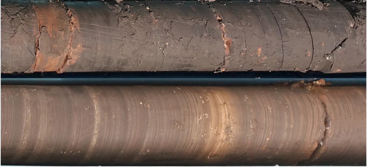
Şekil 2.10. Uंबर seviyelerine ait karot fotoğrafları (kuyu adı: MD-18, karot çapı: 6,35 cm)
