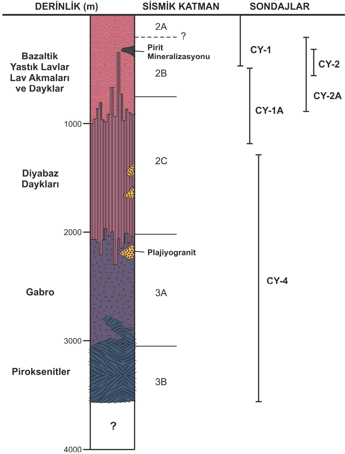
Şekil 1.7. Troodos Masifi'nde yapılan derin sondajlar sonucunda oluşturulan, Troodos okyanusal kabuğuna ait basitleştirilmiş stratigrafik kesit ([18]'den değiştirilerek)
