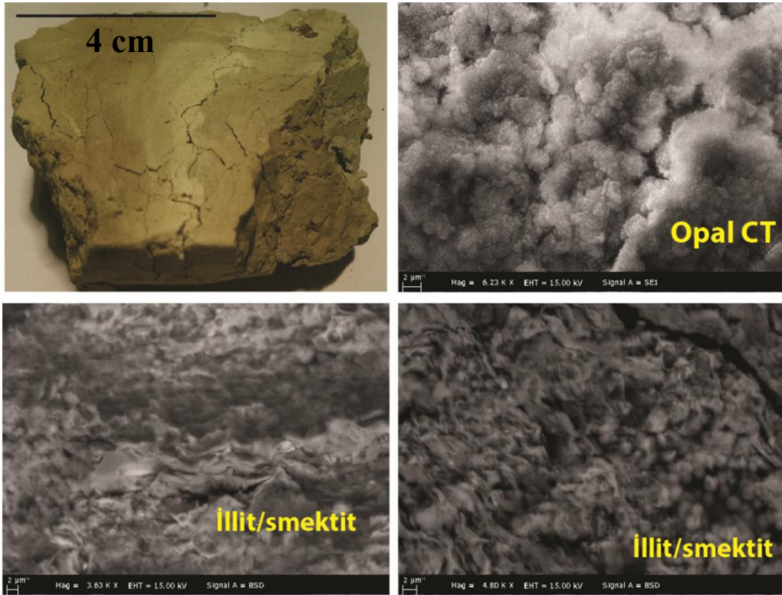
Şekil 2.8. MP-11 el örneği ile opal CT ve illit/smektit minerallerine ait SEM mikrografları
