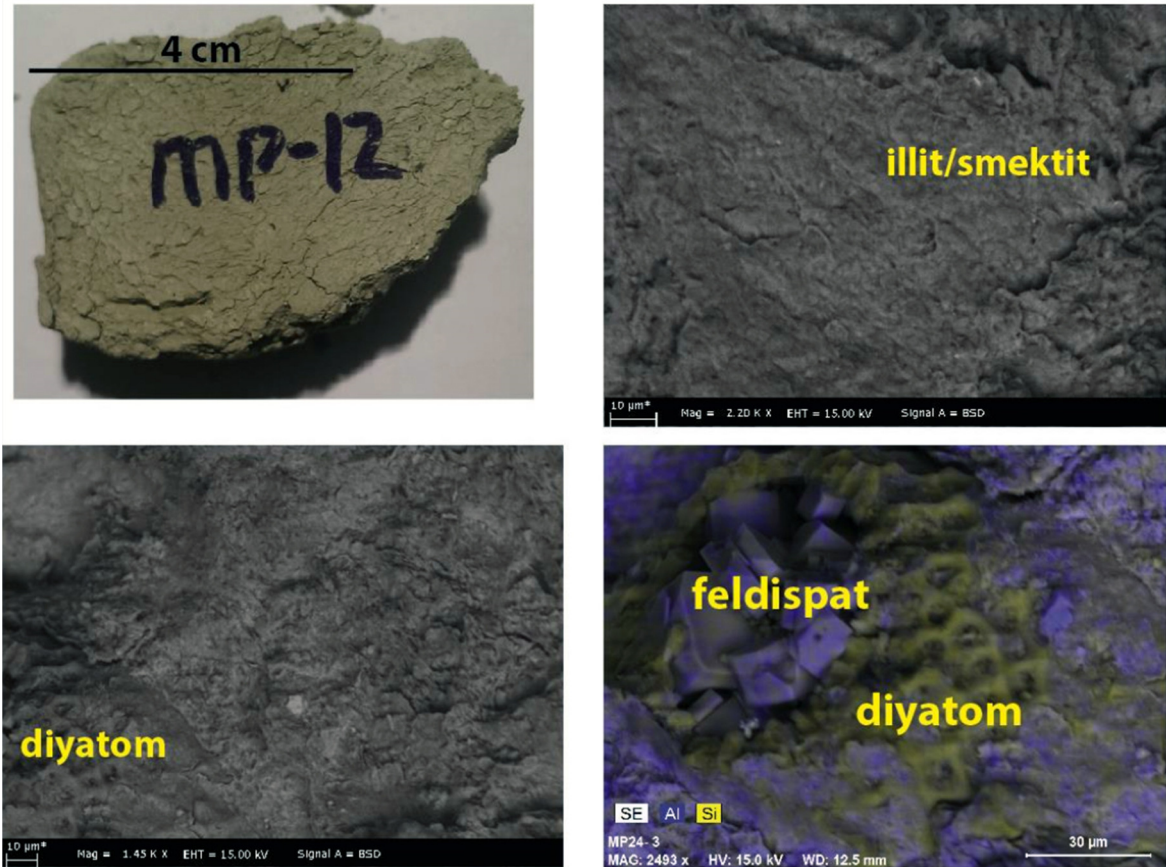
Şekil 2.9. MP-12 el örneği ve SEM mikrografları
