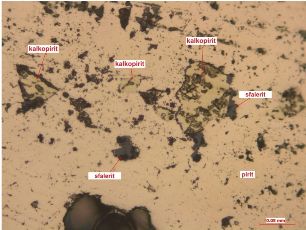
Şekil 2.42. MSC10 örneğinin cevher mikroskobisi incelemesinde gözlenen; masif piritin boşluklarında yer alan kalkopirit ve eser miktarda sfalerit (üstte ve altta), kalkopiritin kenarlarından itibaren bornit tarafından ornatılması (üstte).
