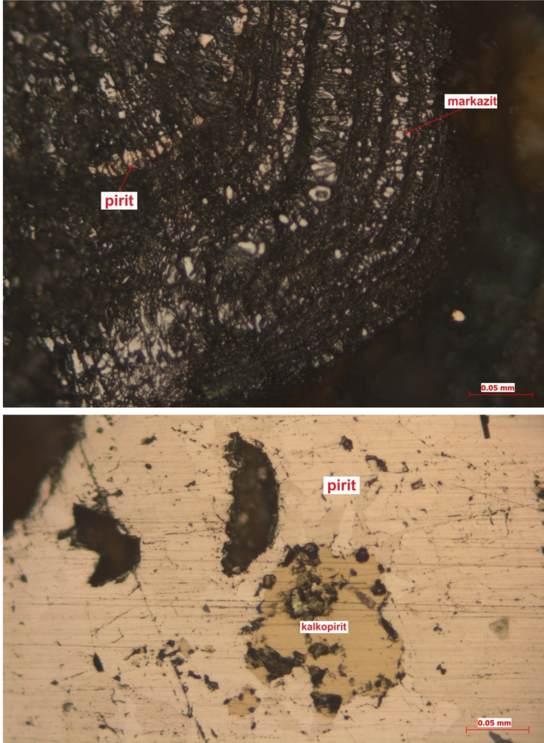
Şekil 2.38. MSC9A örneği cevher mikroskobisi incelemesinde gözlenen; ışınsal dizilişli, ince taneli topluluklar şeklinde markazitler ve merkeze yakın bölümle korunmuş piritler (üstte), masif pirit çakılının boşluklarında gelişen kalkopiritler (altta).
