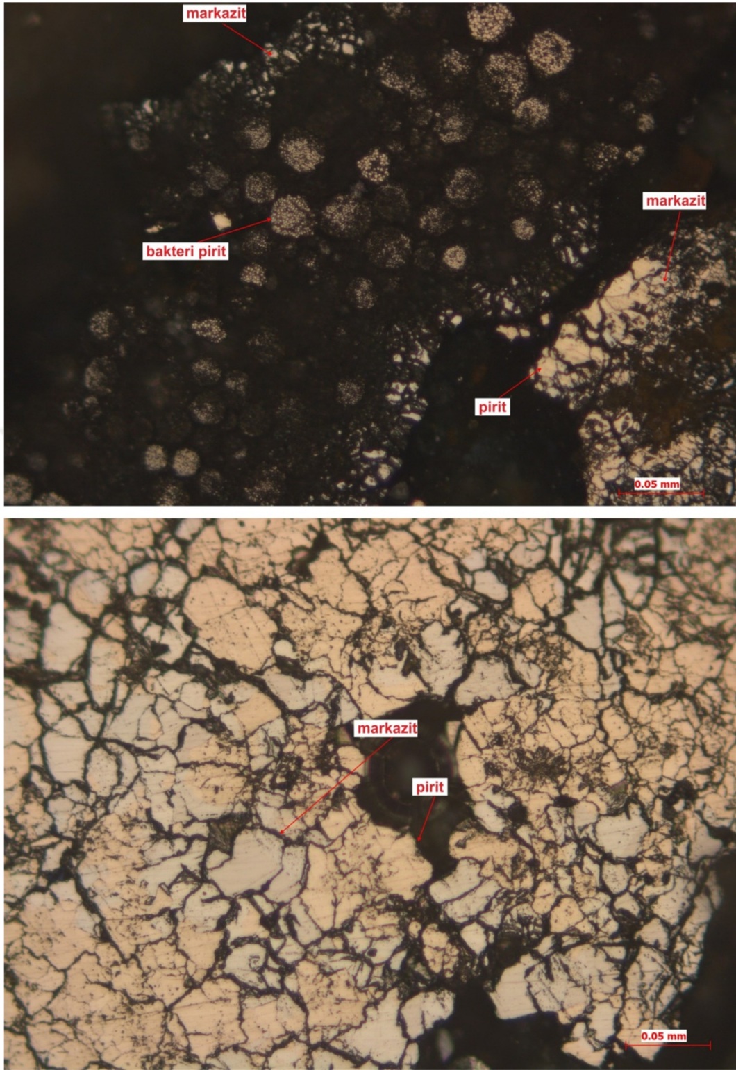
Şekil 2.36. MSC9A örneği cevher mikroskobisi incelemesinde gözlenen; framboidal piritlerin etrafında ince taneli topluluklar şeklinde markazitler (üstte), özşekilsiz piritin görece geniş çatlaklar boyunca markazite dönüşümü (altta).
