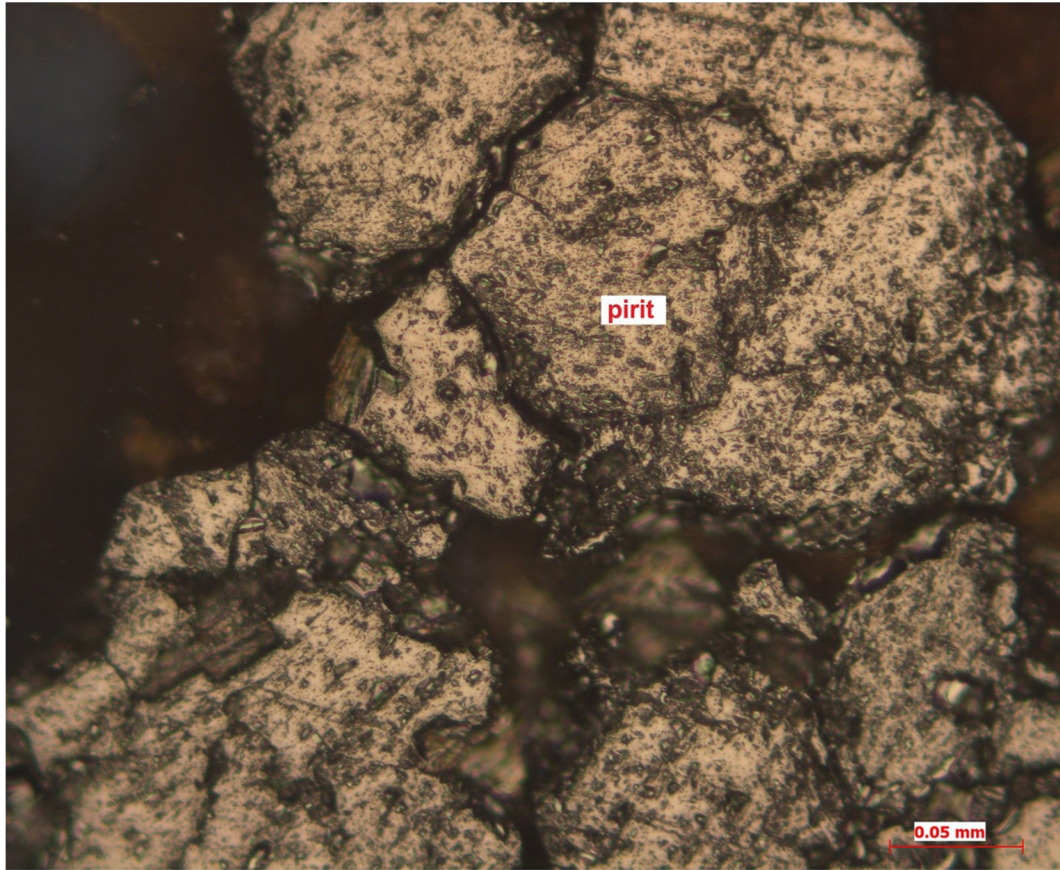
Şekil 2.33. MSC9 örneği cevher mikroskobisi incelemesinde gözlenen; özşekli piritin çevresinde gelişen kalkopiritlerin büyük oranda kovelline dönüşümü (üstte), özşekilsiz jel piritler (altta).
