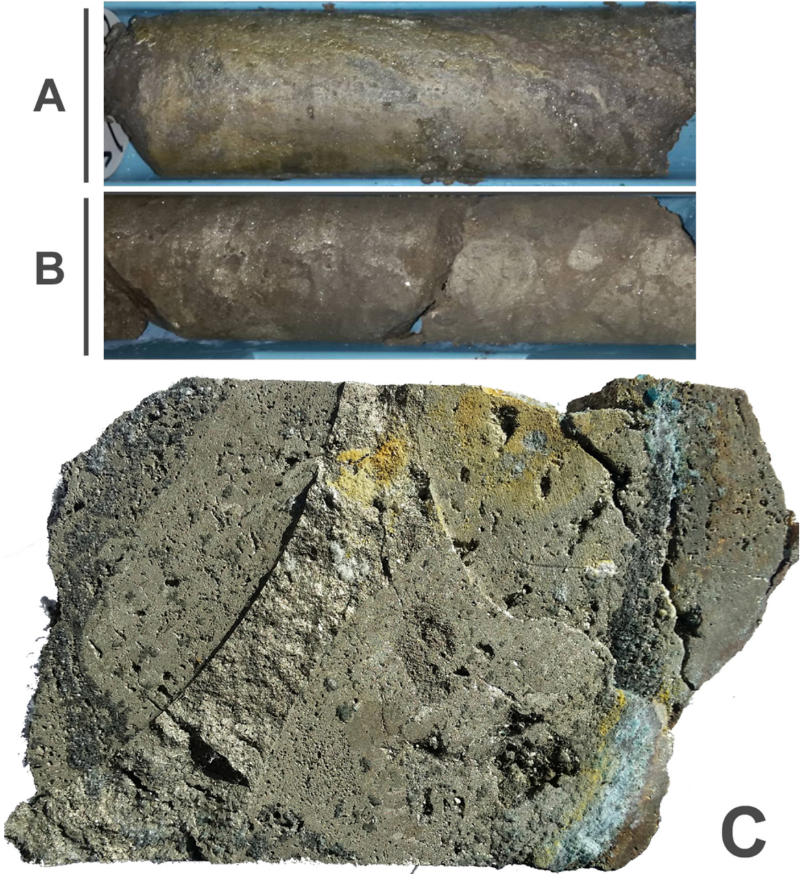
Şekil 2.39. A: MD-4 sondajından masif sülfite bloğu. B: MD-4 sondajından sülfite bloklu cevher (A ve B karot çapı: 6,35 cm). C: MD-11 sondajından yarılanmış masif sülfite bloğu karot görüntüsü. Mavi ve sarı renklerde görülen bakır ve demir sülfatlar, karot kesimi sonrası atmosferik koşullar etkisiyle gelişmiştir. (C karot çapı: 8,5 cm)
