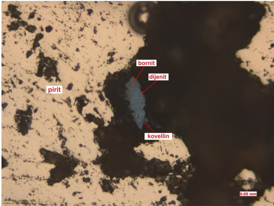
Şekil 2.45. MSC10 örneğinin cevher mikroskobisi incelemesinde gözlenen; kalkopiritlerin bornite ve dijenite ornatılması (üstte), tamamen kovelline ornatılmış serbest kalkopirit tanesinin, bornite ve dijenite ornatılması (altta).
