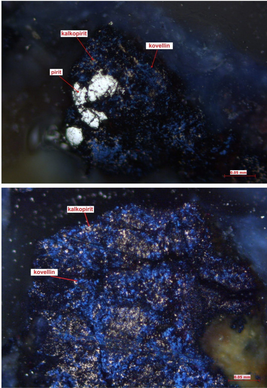
Şekil 2.32. MSC9 örneği cevher mikroskobisi incelemesinde gözlenen; kırık ve çatlaklı özşekilsiz piriti çevreleyen, ince tanecikler şeklindeki kalkopiritlerin büyük oranda kovelline dönüşümü (üstte), kalkopiritlerin kovelline dönüşümü (altta)
