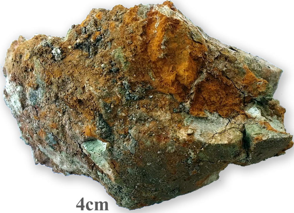
Şekil 2.25. MSC7 el örneği.
