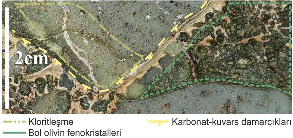
Şekil 2.21. MP-1 karot görüntüsü ve olivin fenokristallerinin yakın çekim görüntüsü (kuyu adı: MD-11, karot çapı: 8,5 cm)
