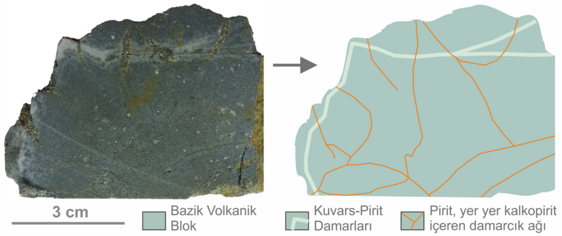
Şekil 2.62. MD-18 nolu sondajda kesilen polimiktik breş cevher zonu içerisinde tanımlanan kök/ağsal damarcıklı zona ait blok.
