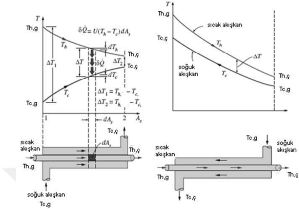
Şekil 4.16. Paralel ve çapraz akışlı eşanjörlerde sıcaklık fark grafiği (Çengel, 2002)
