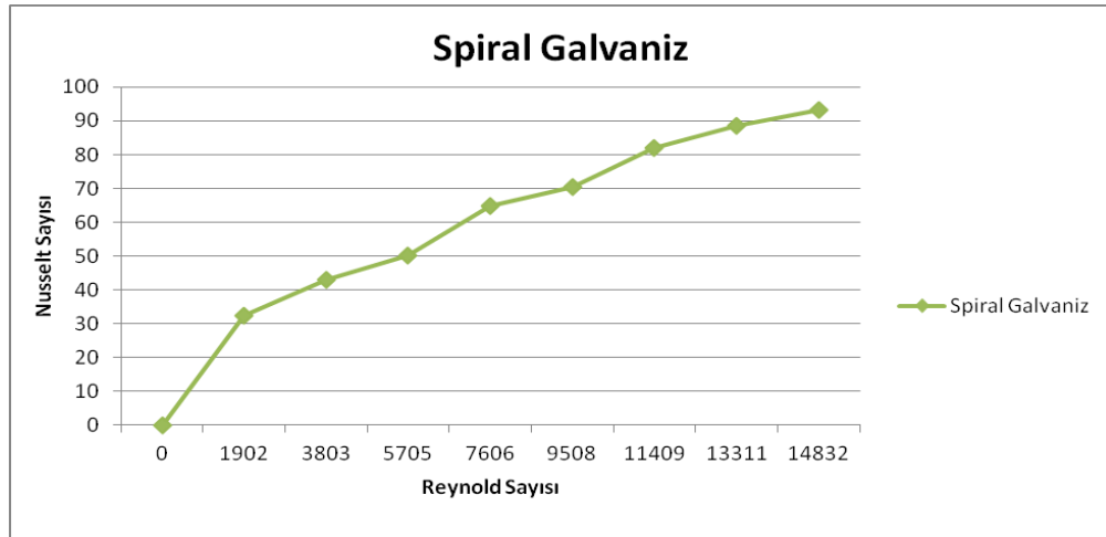
Şekil 5.6. Deney sistemi spiral galvaniz levha boru Nusselt Sayısı-Reynolds Sayısı grafiği
