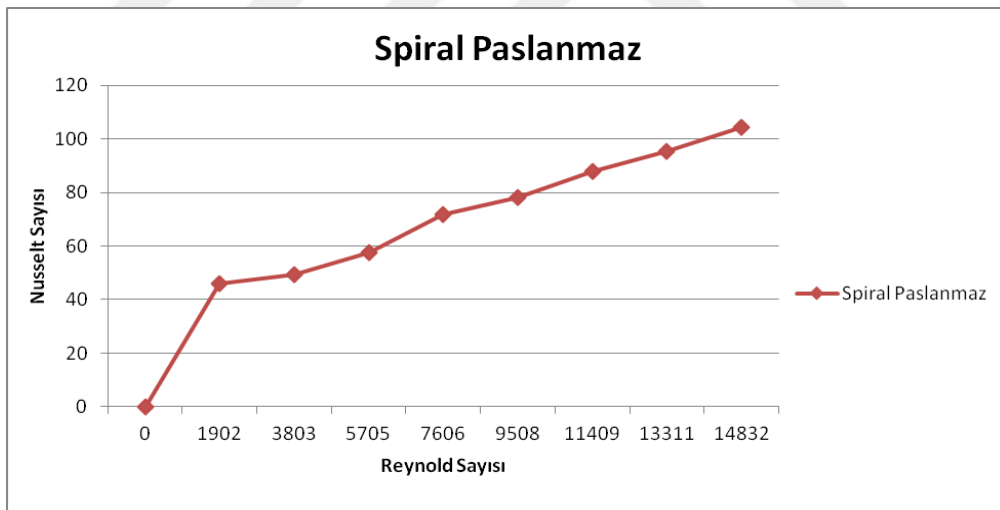
Şekil 5.7. Deney sistemi spiral paslanmaz çelik levha boru Nusselt Sayısı-Reynolds Sayısı grafiği
