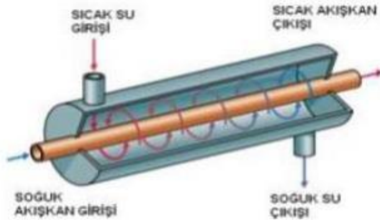
Şekil 3.1. Düz borulu ısı değıştircisi (Bozkula, 2016)
