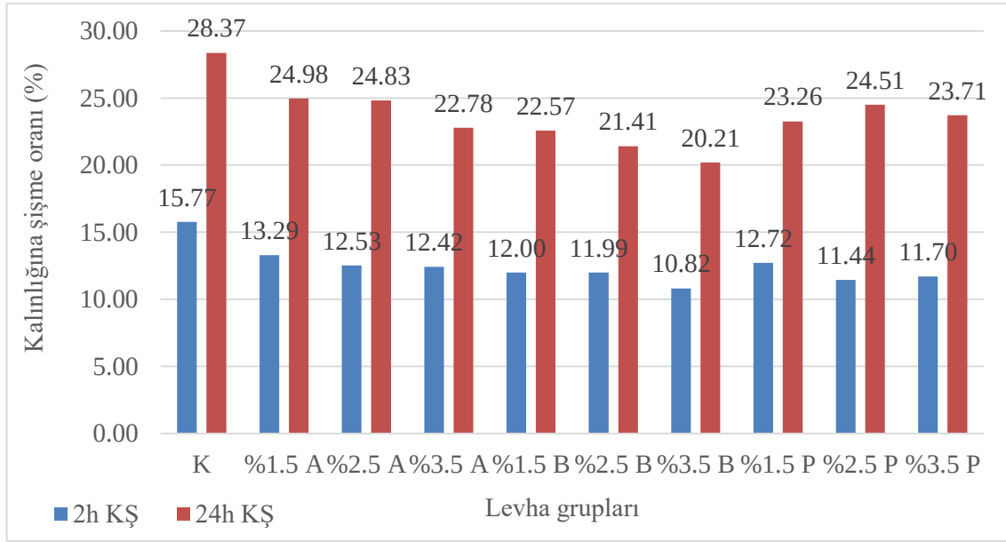
Şekil 3.1: Levha gruplarının 2 ve 24 saat kalınlığına şişme değerleri.
