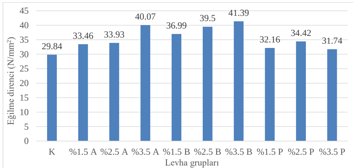
Şekil 3.4: Levha gruplarının eğilme direnci değerleri
