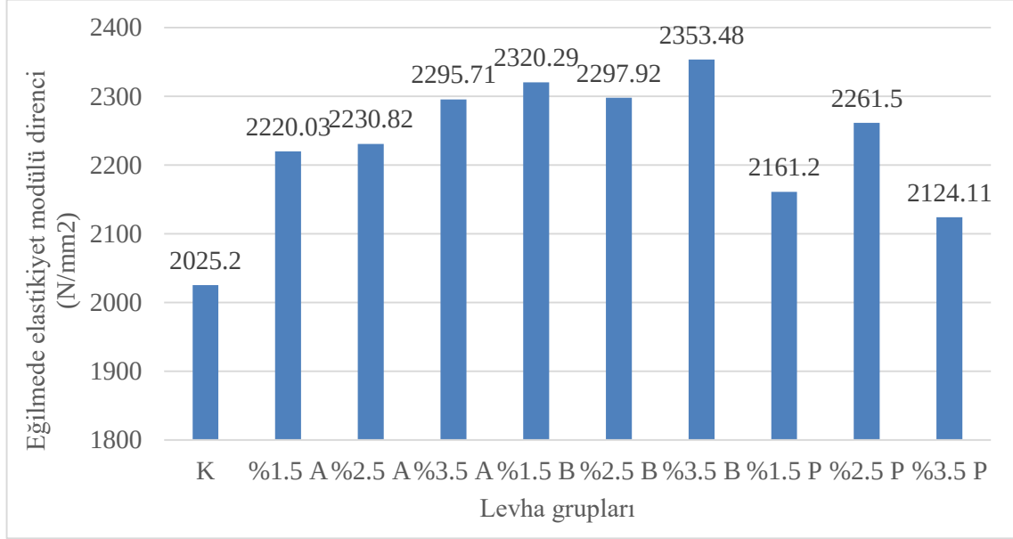
Şekil 3.5. Levha gruplarının eğilme elastikiye modülü direnci değerleri.
