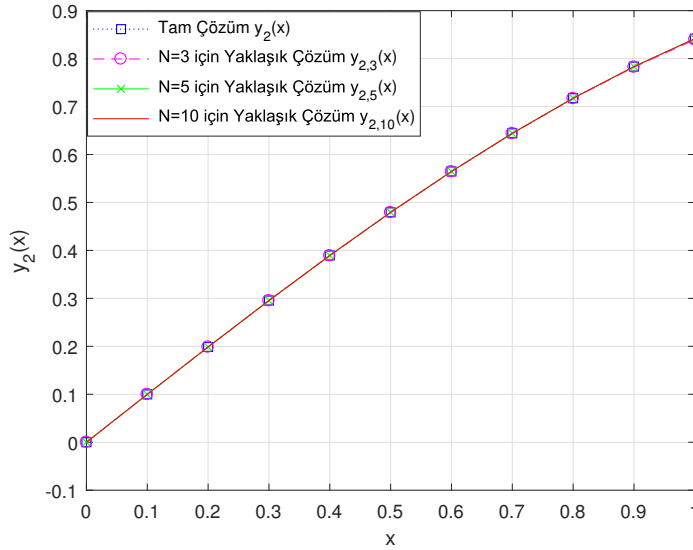
Şekil 4.31. Örnek 4.5'te y_2(x) tam çözümü ve N = 3, 5, 10 için yaklaşık çözümleri
