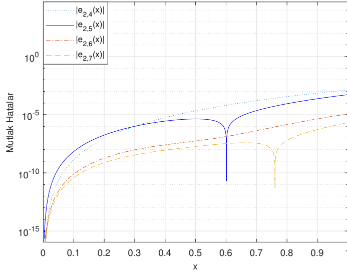
Şekil 4.24. Örnek 4.4 için e_{2,N}(x) gerçek hatasının çeşitli N değerleri için elde edilen gerçek mutlak hata fonksiyonları
