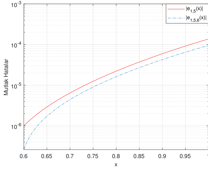
Şekil 4.28. Örnek 4.4'ün y_1(x) çözümü için N = 5 ve M = 6 olarak alındığında elde edilen gerçek ve tahmini mutlak hata fonksiyonlarının karşılaştırılması
