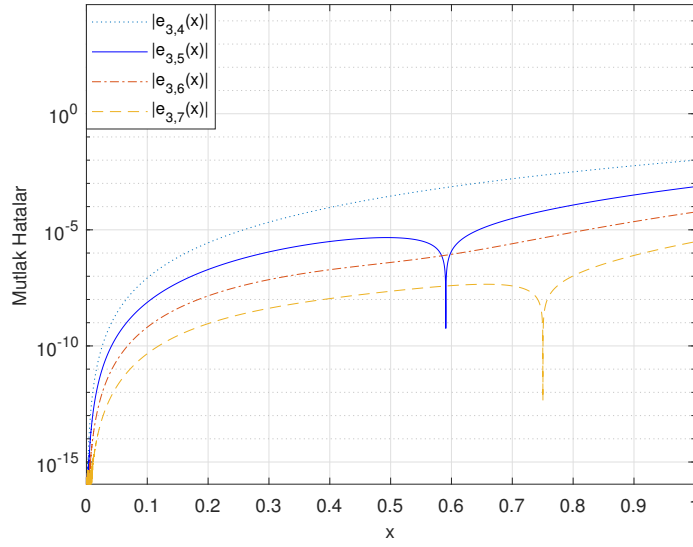
Şekil 4.25. Örnek 4.4 için e_{3,N}(x) gerçek hatasının çeşitli N değerleri için elde edilen gerçek mutlak hata fonksiyonları
