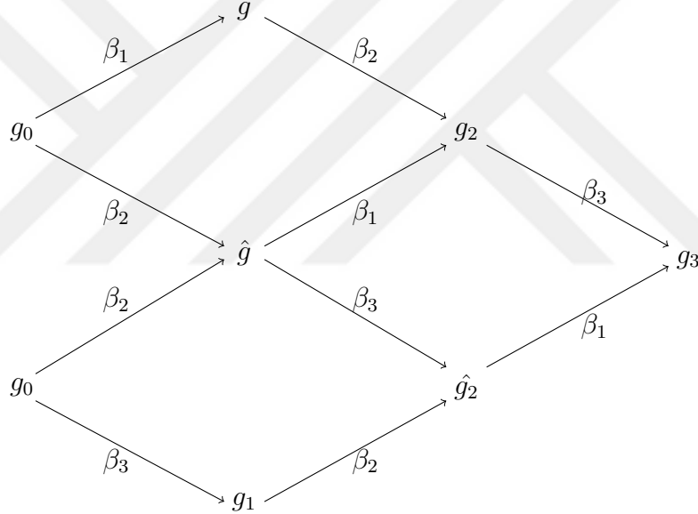
Şekil 10: KdV denkleminin bilineer formla elde 3-soliton çözümü için Bianchi diyagramı
