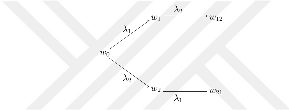
Şekil 4: KdV denklemi için Bianchi diyagramı
