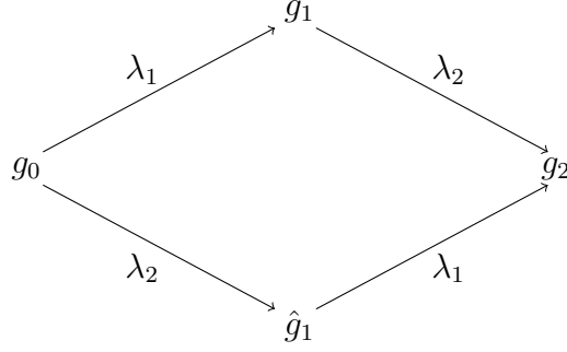
Şekil 8: KdV denklemleri için bilineer formdaki süperpozisyon formülünün komütatif Bianchi diyagramı
