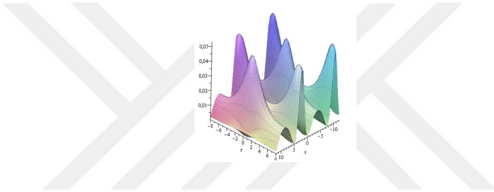
Şekil 11: Boussinesq denkleminin periyodik breather tip dalga çözümü
