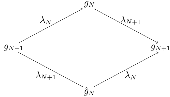
Şekil 9: KdV denklemi için bilineer formdaki süperpozisyon formülünün genelleştirilmiş komütatif Bianchi diyagramı
