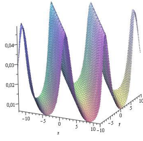
Şekil 12: Boussinesq denkleminin periyodik dalga çözümü
