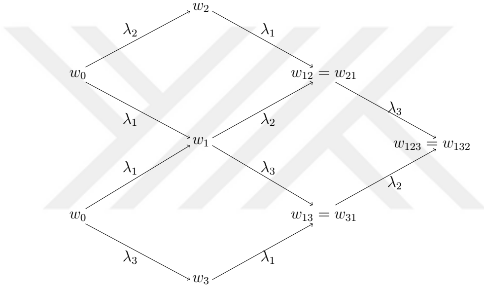
Şekil 7: KdV denkleminin 3-soliton çözümünün Bianchi diyagramı
