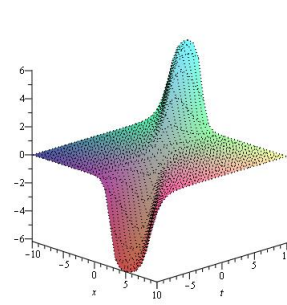
Şekil 14: Sine-Gordon denkleminin kink-antikink etkileşimini ifade eden çözümü
