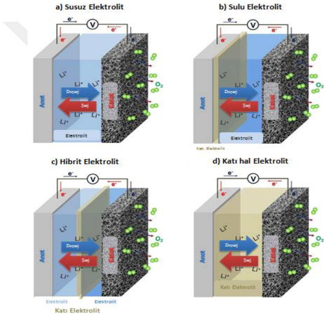
Şekil 3.6. Lityum hava pillerinde kullanılan elektrolit tipleri [34].
