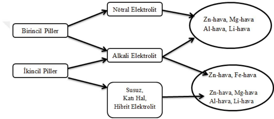
Şekil 2.5. Metal hava pil çeşitleri [15].
