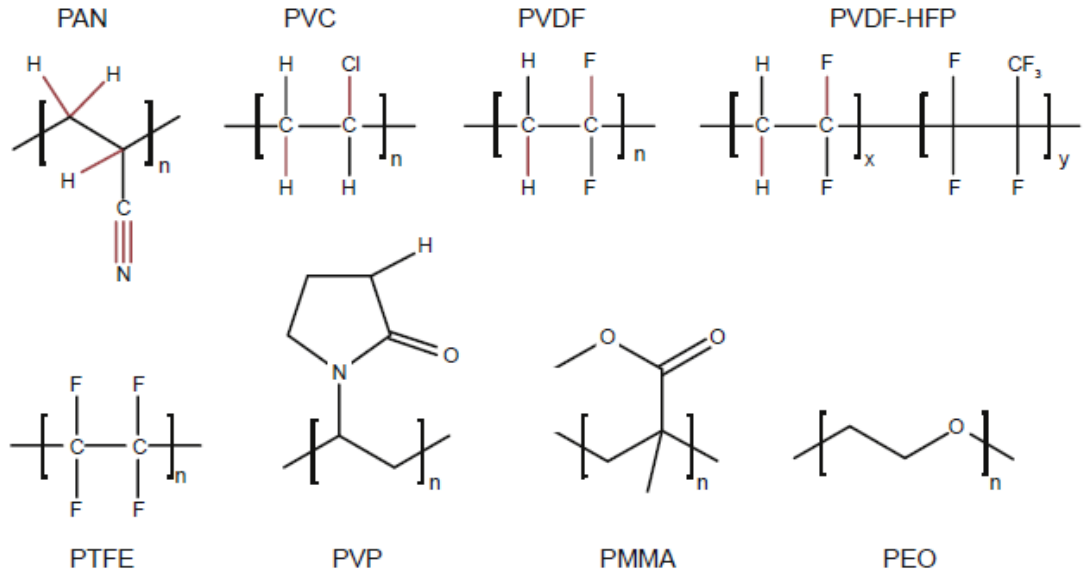
Şekil 3.7. Yaygın olarak kullanılan polimerlerin yapısal formülleri. Kırmızı çizgiler \text{Li}_2\text{O}_2 ile reaksiyona girdiğinde tercihen ayrılan bağları göstermektedir [61].
