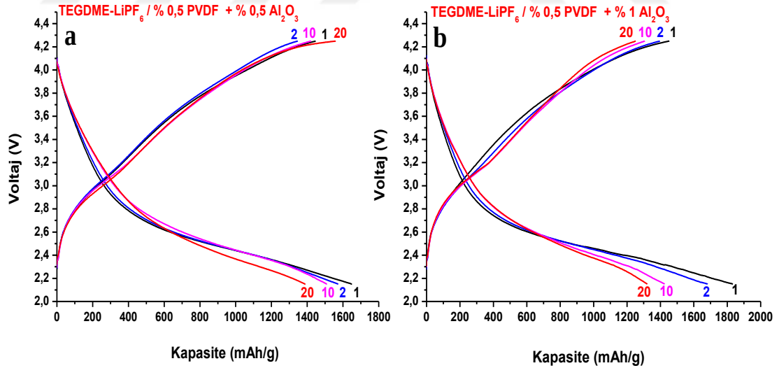
Şekil 7.4. PVDF ve nanoseraamik partikül ilaveli elektrolitlere ait kapasite-voltaj eğrileri.
