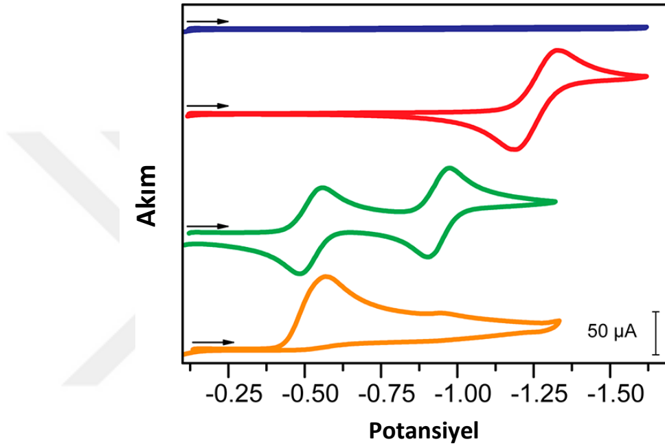
Şekil 6.4. Literatürdeki bazı çalışmalara ait CV eğrisi örnekleri [125].
