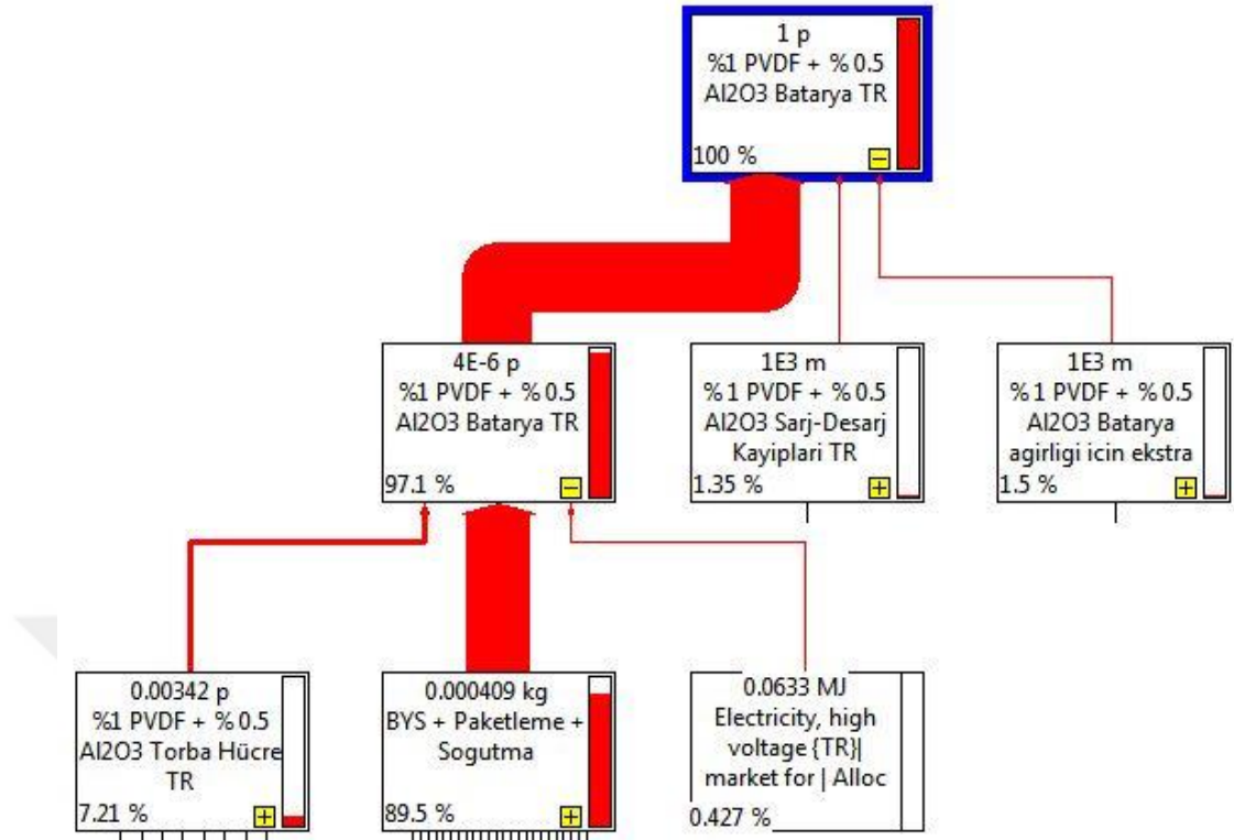
Şekil 7.15. %1 PVDF + %0,5 Al 2 O 3 batarya AKTP sonuçlarına proses katkıları (kg Sb-eş/km).
