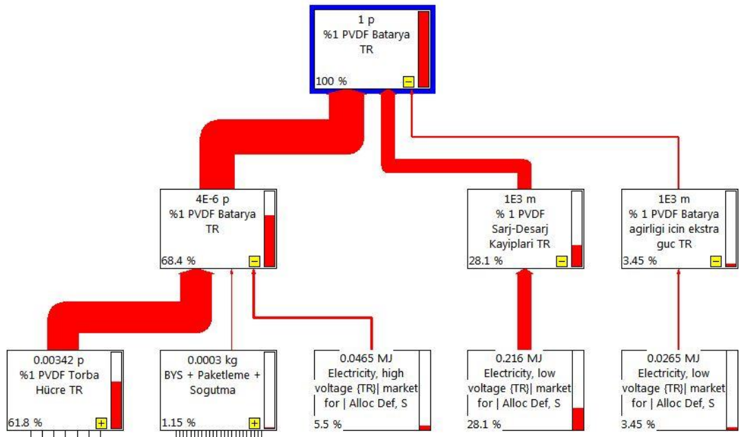
Şekil 7.11. %1 PVDF batarya KIP sonuçlarına proses katkıları (kg CO 2 -eş/km).
