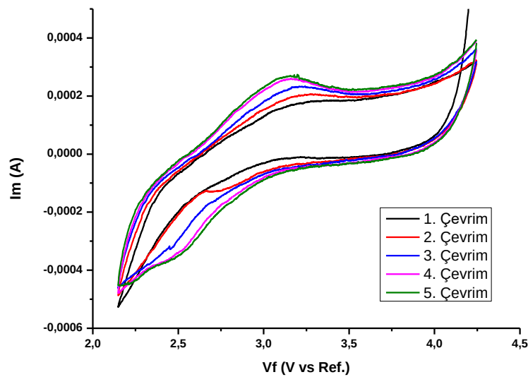
Şekil 7.1. İlavesiz TEGDME-LiPF 6 elektrolitine ait 5 çevrimlik CV değerleri.
