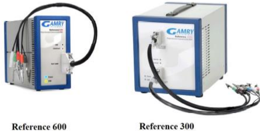
Şekil 6.6. Gamry marka Reference 600 ve Reference 3000 model potensiyostat/galvanostat cihazları.
