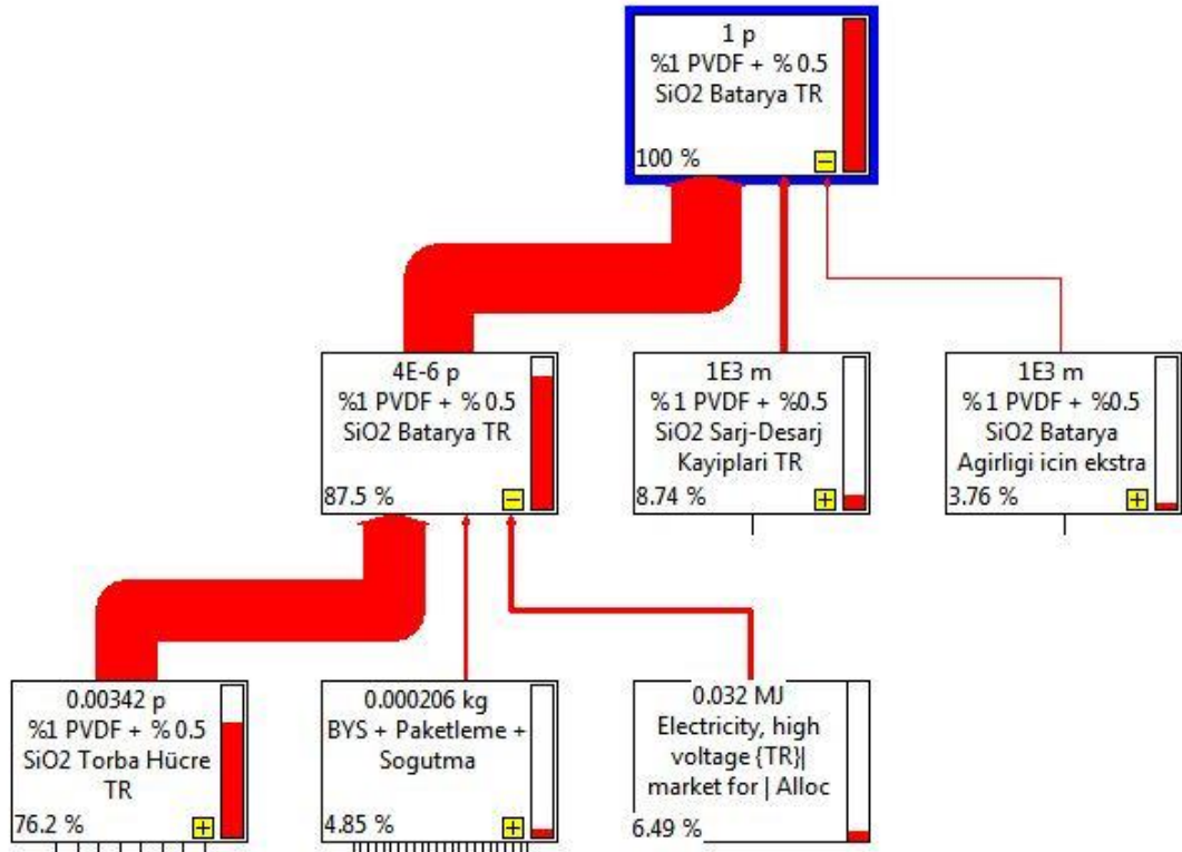
Şekil 7.22. %1 PVDF + %0,5 SiO 2 batarya insan toksisitesi - kanser etki grafiği.
