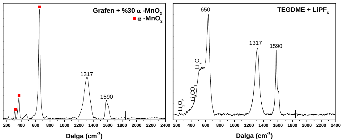
Şekil 7.9. Grafen / % 30 \alpha - \text{MnO}_2 katot çevrim öncesi ve çevrim sonrası Raman spektrum grafiği.
