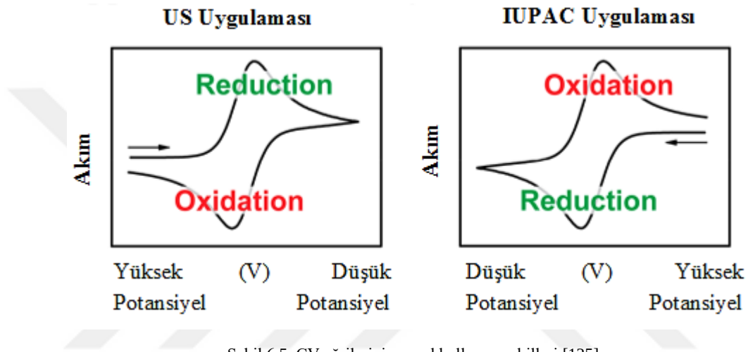
Şekil 6.5. CV eğrilerinin genel kullanım şekilleri [125].
