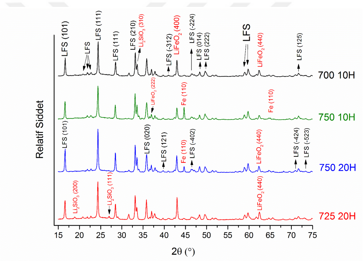
Şekil 4. 3. Sıcaklık ve süreye bağlı olarak istenen ve istenmeyen fazlarının karşılaştırılması
