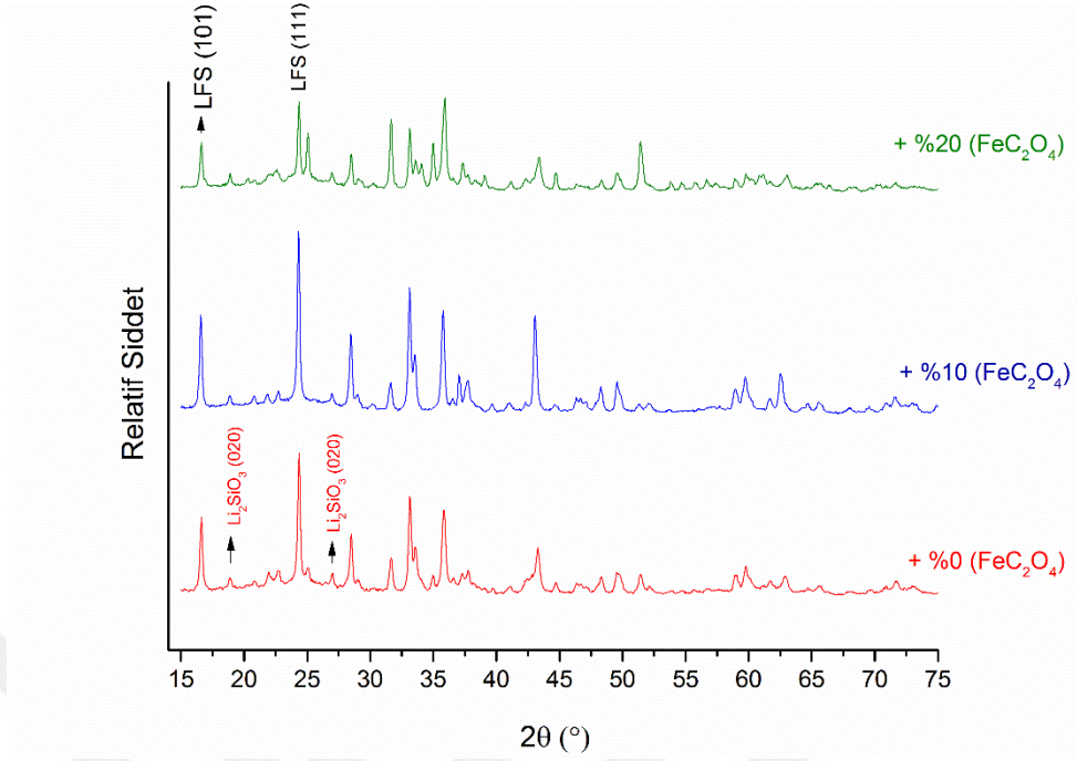
Şekil 4. 7. Kütlece %0, %10 ve %20 fazlardan Fe (II) Okzalat İlavesi ile sentezlenen LFS tozuna ait XRD patternleri
