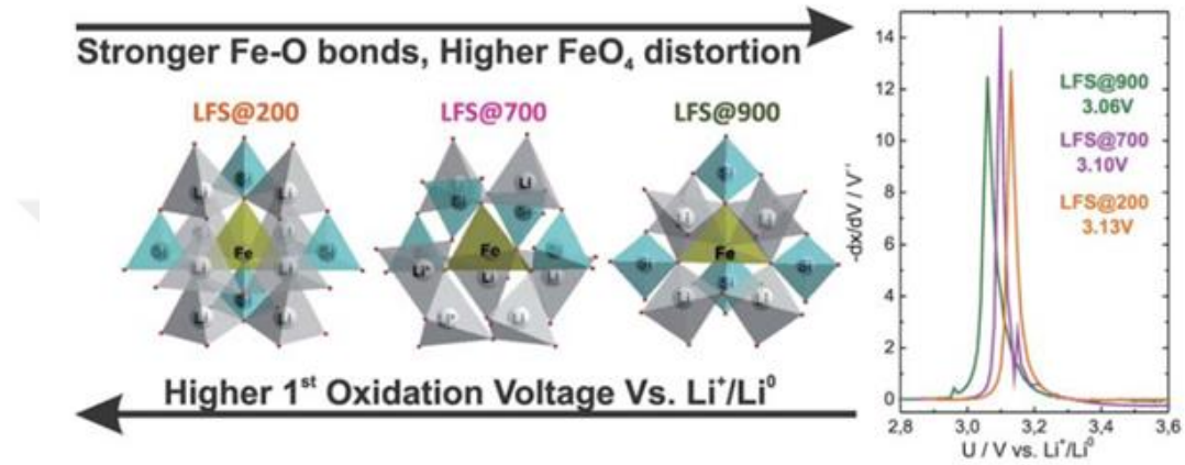
Şekil 2. 8. Farklı sıcaklıklarda (200, 700 ve 900°C) tavlama görmüş LFS kristal yapısının değişimi
