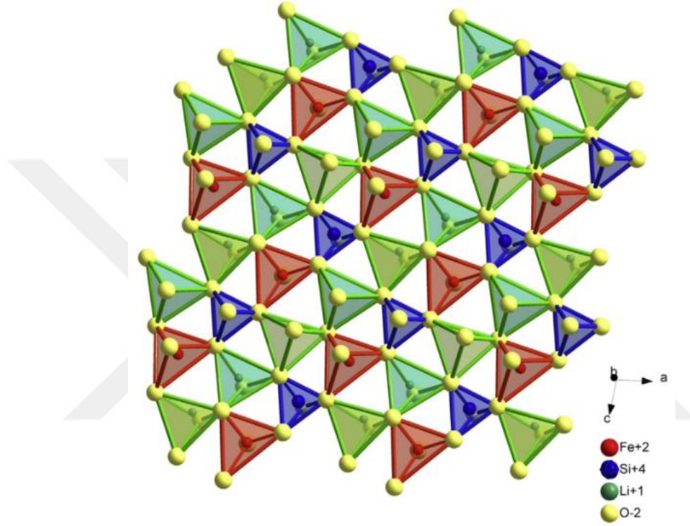
Şekil 2. 10. b-ekseni yönünde \text{Li}_2\text{FeSiO}_4 kristal yapısı.
