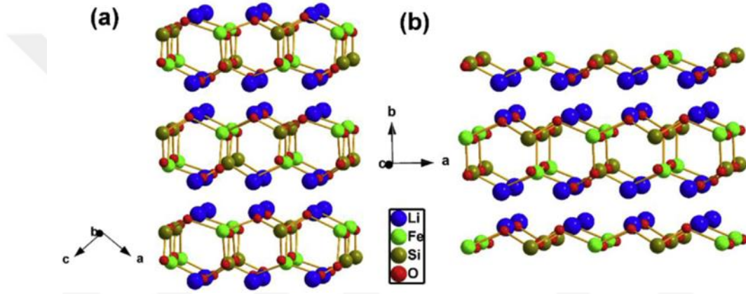
Şekil 2.7. Monoklinik (a) ve ortorombik (b) LFS kristal yapılarının şematik gösterimi. Her iki kristal yapıda da Li iyonları FeO 4 -SiO 4 tetrahedraları arasına girmektedir
