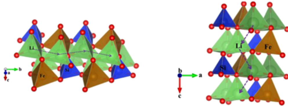
Şekil 2. 9. LFS ( \text{Pmn}2_1 ) uzay düzlemine göre Li iyonlarının difüzyonu sırasında takip ettiği 2 farklı yön
