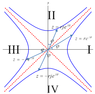
Şekil 4.1. Lorentz düzleminde hareket
