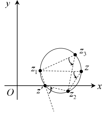
Şekil 2.3c Üç noktadan geçen çember
