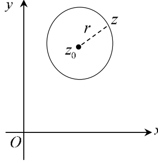
Şekil 2.3b z_0 merkezli r yarıçaplı çember
