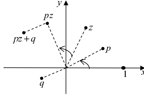
Şekil 2.5. Z noktasının z' noktasına hareketi
