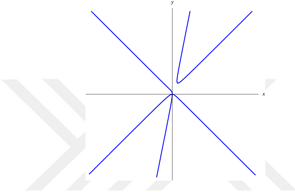
Şekil 4.3. Lorentz düzleminde a_3 = 2 ve b_3 = 1 için cp eğrisi
