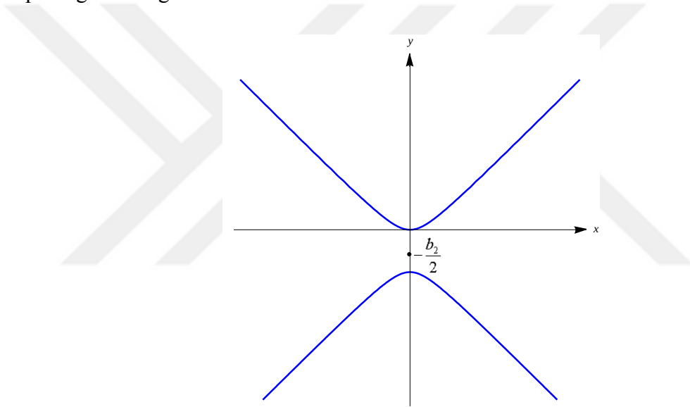
Şekil.4.2. Lorentzian büküm çemberi
