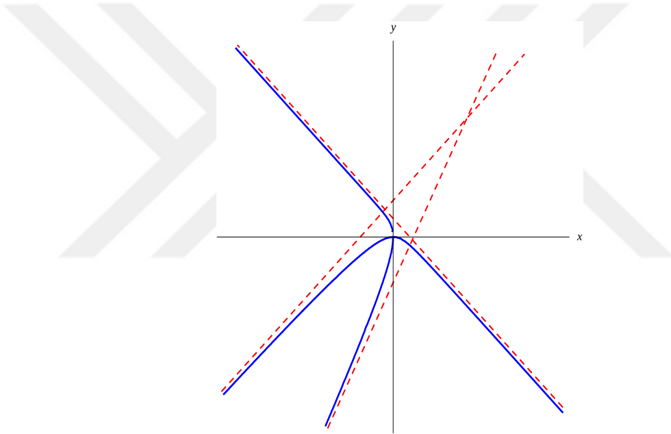
Şekil 4.8. Lorentz düzleminde cp ve c\tilde{p} eğrileri ile asimptotları
