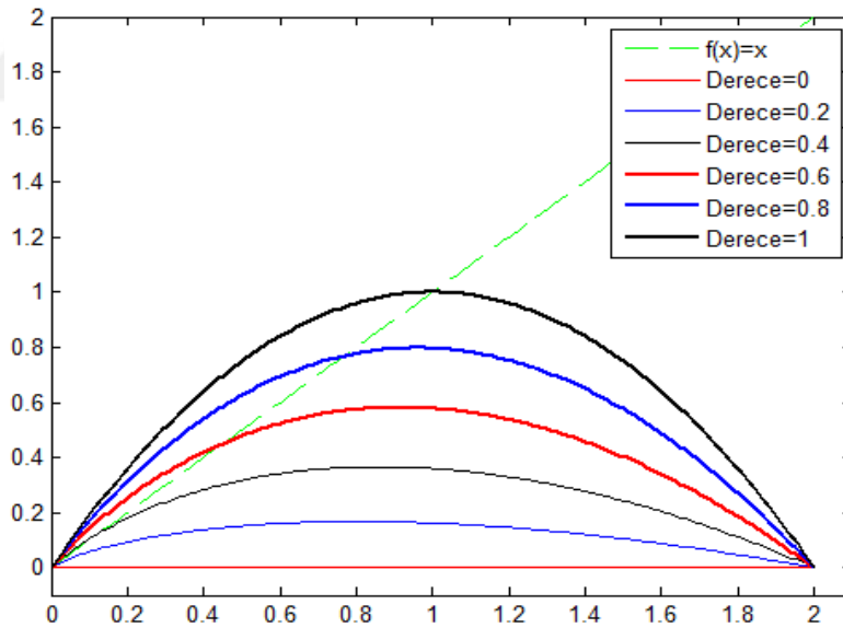
Şekil 3.1 f(x) = x fonksiyonu Riemann-Liouville kesirli dereceli türevleri
