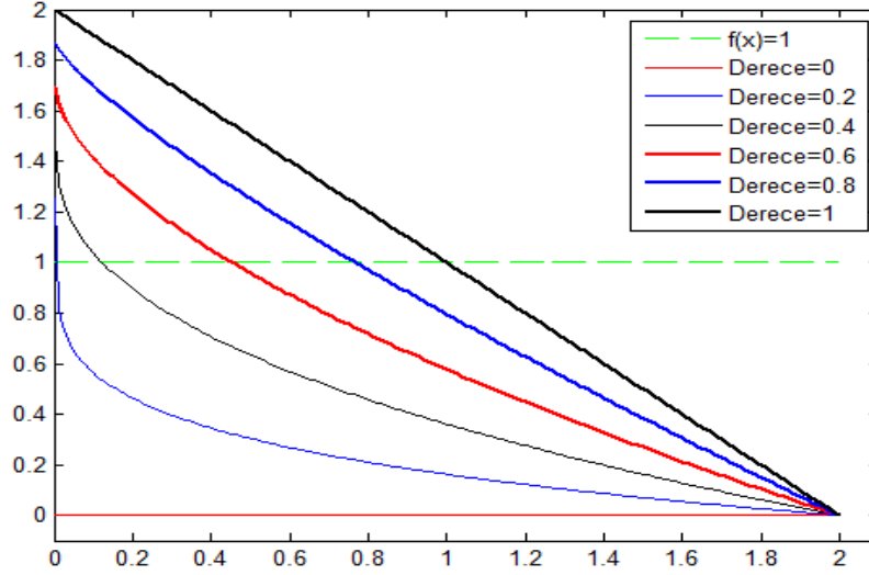
Şekil 3.2 f(x)=1 fonksiyonu Riemann-Liouville kesir dereceli türevleri
