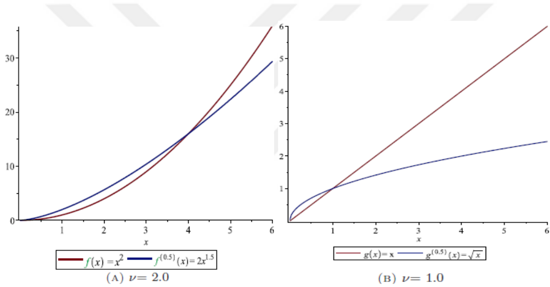
Şekil 3.3 f(x) = x^\nu kuvvet fonksiyonunun 1/2 merteben Katugampola kesirli türevleri
