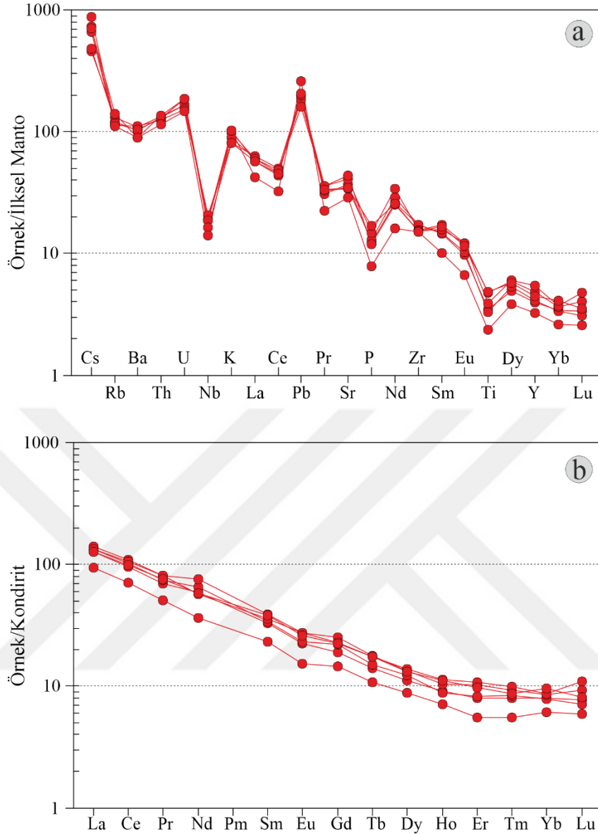
Şekil 3.12. Volkanik kayaların iz element dağılım diyagramları, (a) İlksel manto (Sun ve McDonough, 1989) (b) Kondirite (Boynton, 1984) göre normalize edilmiş nadir toprak element dağılımları.
