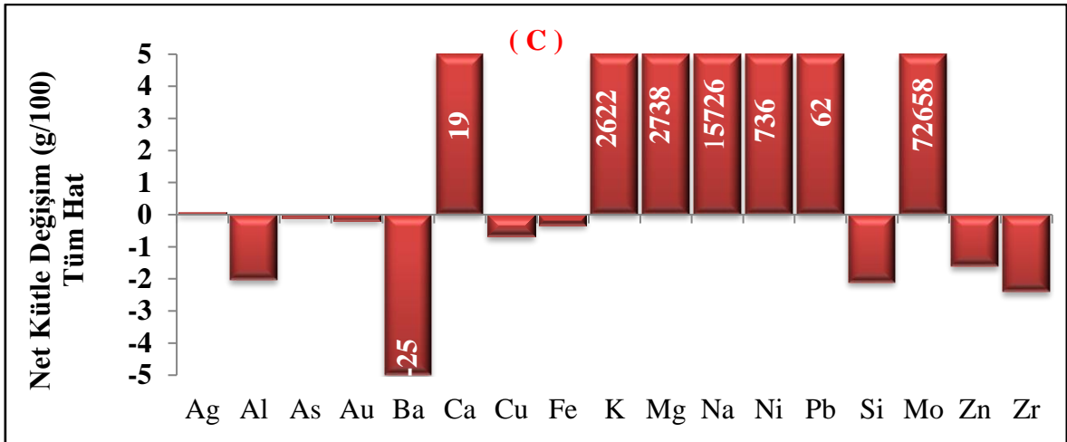
Şekil 3.24. Alterasyon zonunda hesaplanan net kütle değişim diyagramları a) propilitik alterasyon zonu, b) cevherli zon, c) tüm hat.
