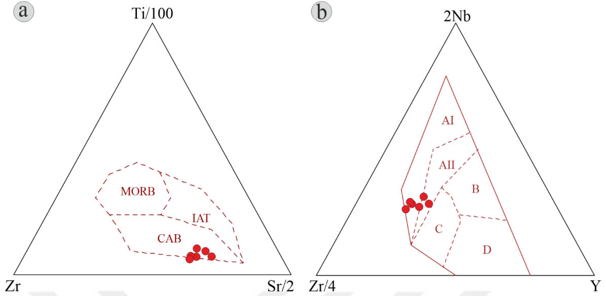
Şekil 3.13. Volkanik kayaların tektonik ayırtman grafikleri A) Ti/100-Zr-Sr/2 diyagramı (MORB: Okyanus tabanı bazaltı, CAB: Kalk-alkali bazaltı, IAT: Adayayı toleyitik bazaltı), (Pearce ve Cann, 1973), B) Zr-Nb-Y diyagramı (AI: Plaka içi alkali bazalt, AII: Plaka içi alkali bazalt/toleyit, B: E-tipi MORB, C: Plaka içi toleyit/volkanik yay bazaltı, D: N-tipi MORB/volkanik-yay bazaltı), (Meschede, 1986).
