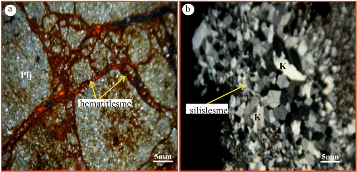
Şekil 3.21. Üst Kretase yaşlı Andezitlerde, ayrışmaların mikroskop altında çapraz nikeldeki görünüşleri. (a) Hematitleşme, Örnek no: M12, (b) Silisleşme, Örnek no: M13. (Plj: Plajiyoklas; K: Kuvars)
