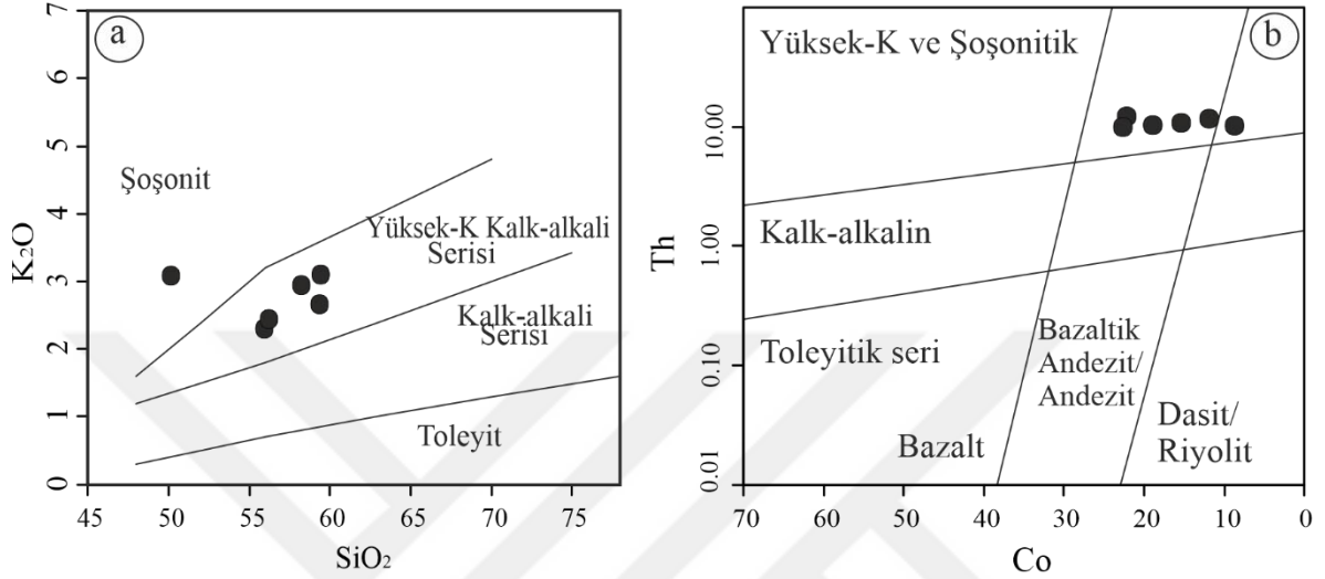
Şekil 3.11. Volkanik kayaların (a) SiO 2 (%)'ye karşı K 2 O (%) ve (b) Co karşı Th diyagramı.
