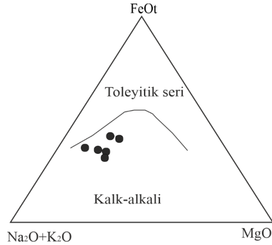
Şekil 3.10. Volkanik kayalarının AFM üçgen diyagramı (toleyitik-kalk-alkali ayırım eğrisi Irvine ve Baragar, 1971'den alınmıştır).
