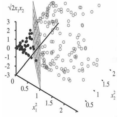
b.) 3 boyuta taşındıktan sonra doğrusal olarak ayrılabilen veriler
