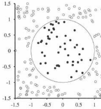
a.) 2 boyutta doğrusal olarak ayıramayan veriler
