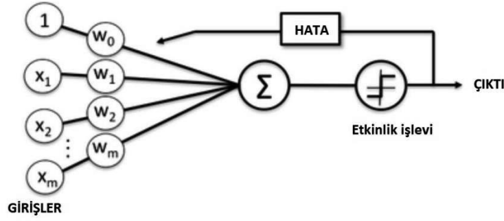
Şekil 2-8 Perceptron örneği
