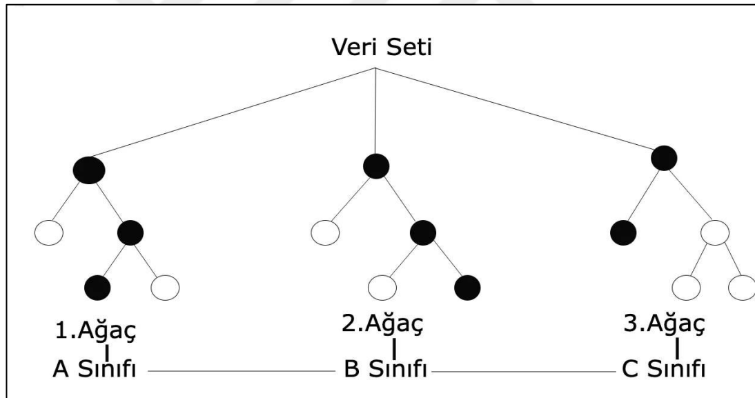
Şekil 3.6 Rastgele orman (Tafralı, 2022)
